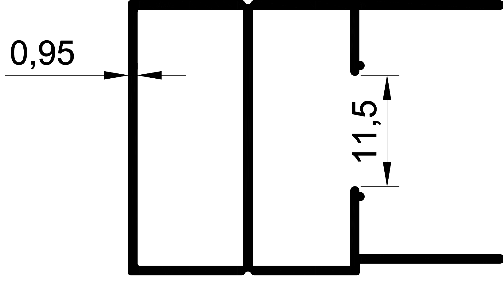
EKOL 1142 0,374 gr/m. PİLELİ SİNEKLİK KASA
