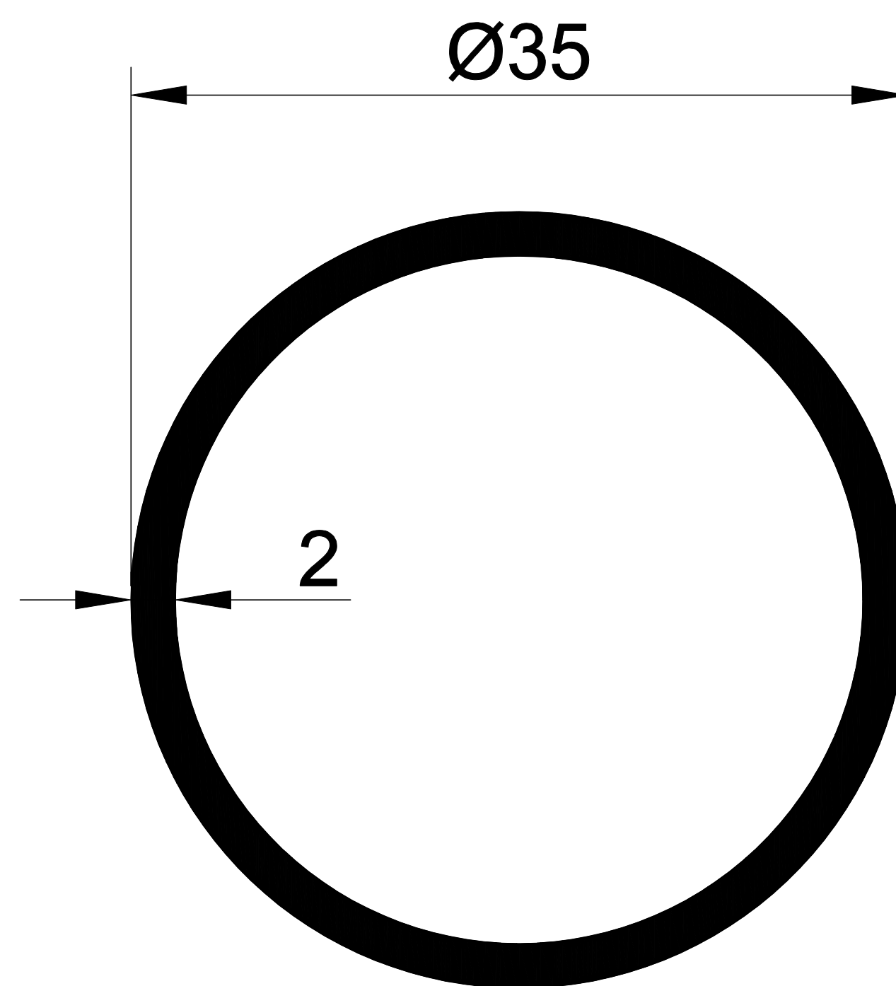
EKOL 1070-B 0,561 gr/m.
