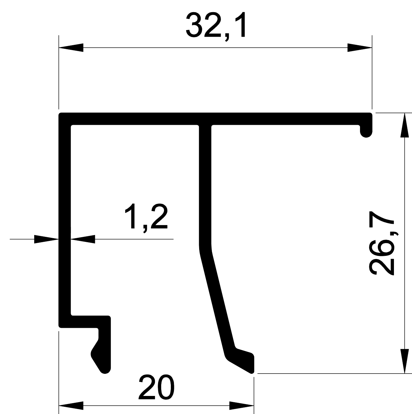
EKOL 1404 0,297 gr/m. BİM ISI CAM ÇİTASI
