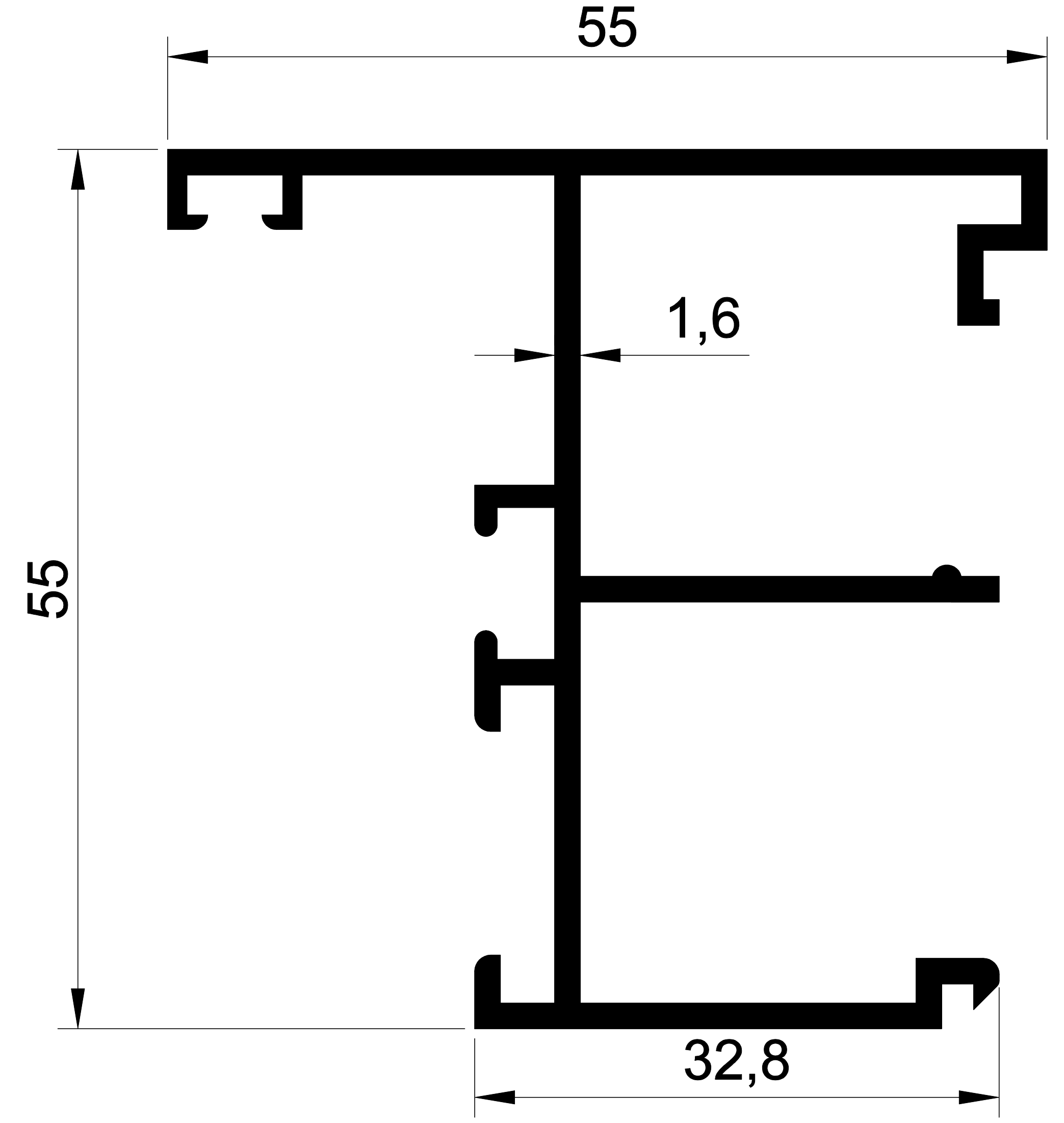
EKOL 1354 0,915 gr/m. SİSTEM ÇİFT KAPI ADAPTÖRÜ
