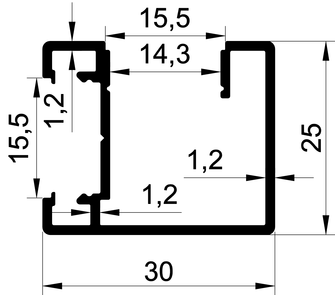
1462 0,357 gr/m 30*25 GEMİCİ
