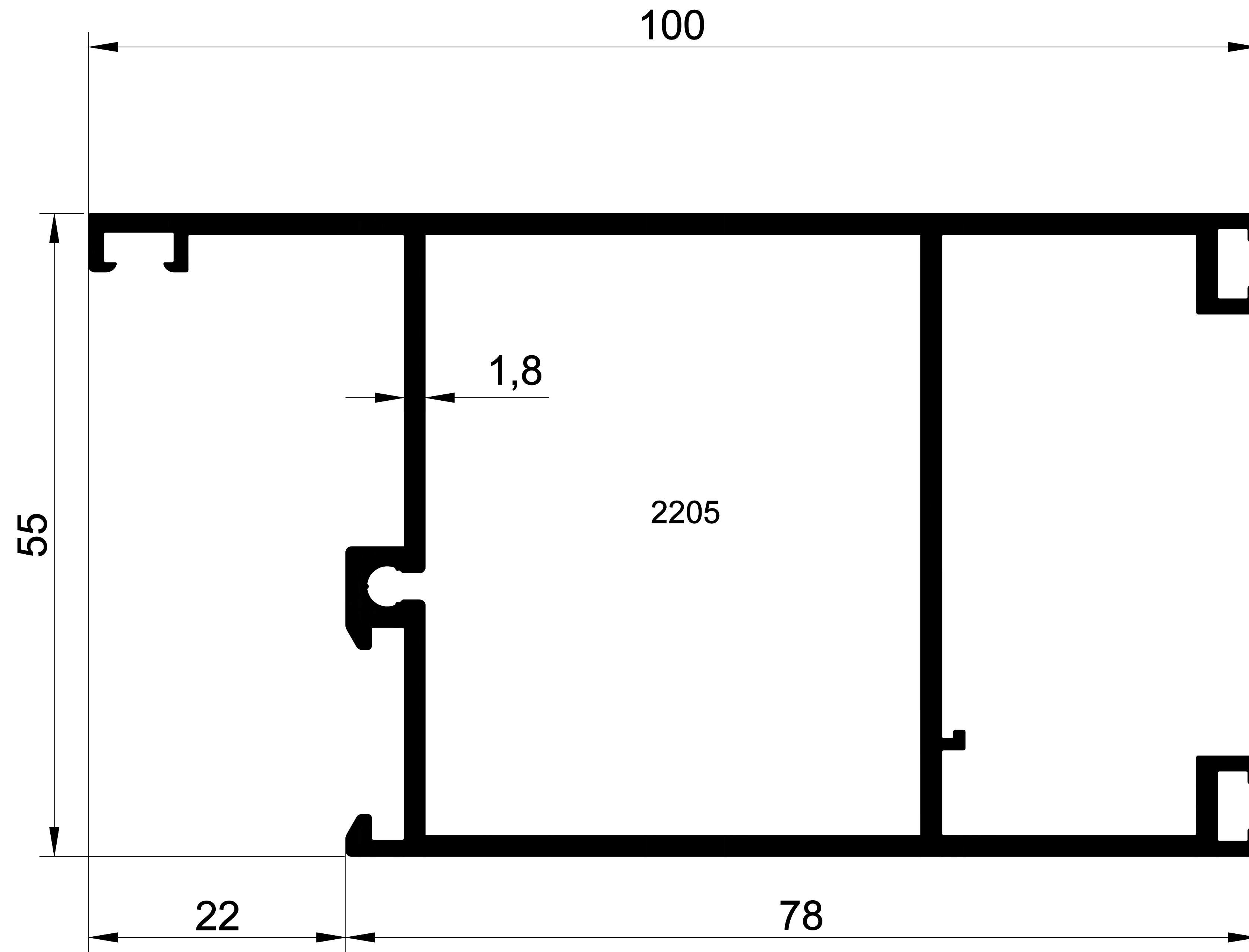
EK-55- 2205 1,561 gr/m
