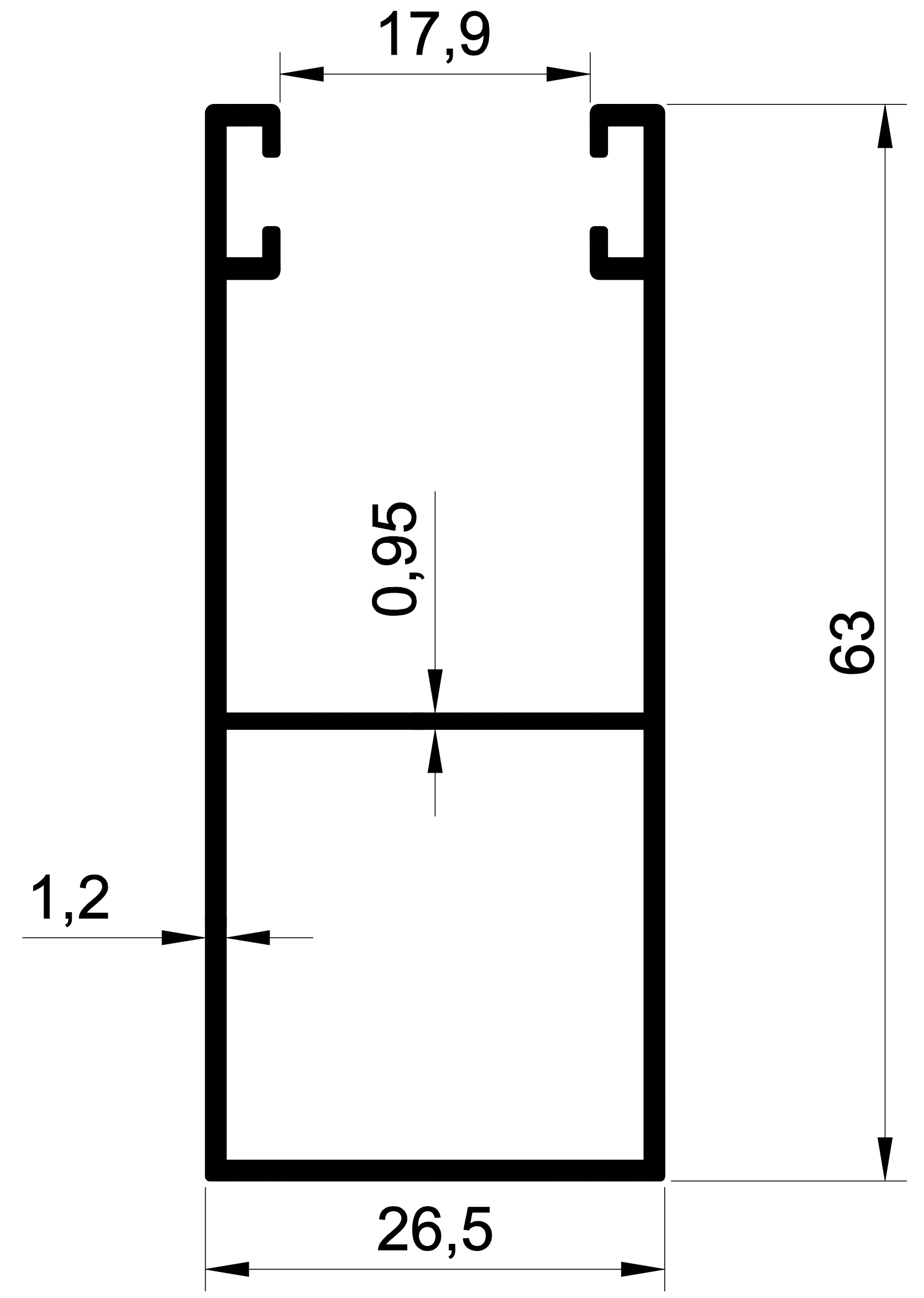
EKOL 1308 0,604 gr/m. 63'LÜK DİKME
