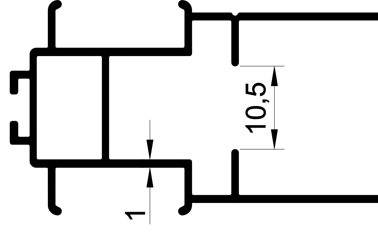
EKOL 1143 0,409 gr/m. PİLELİ SİNEKLİK KANAT
