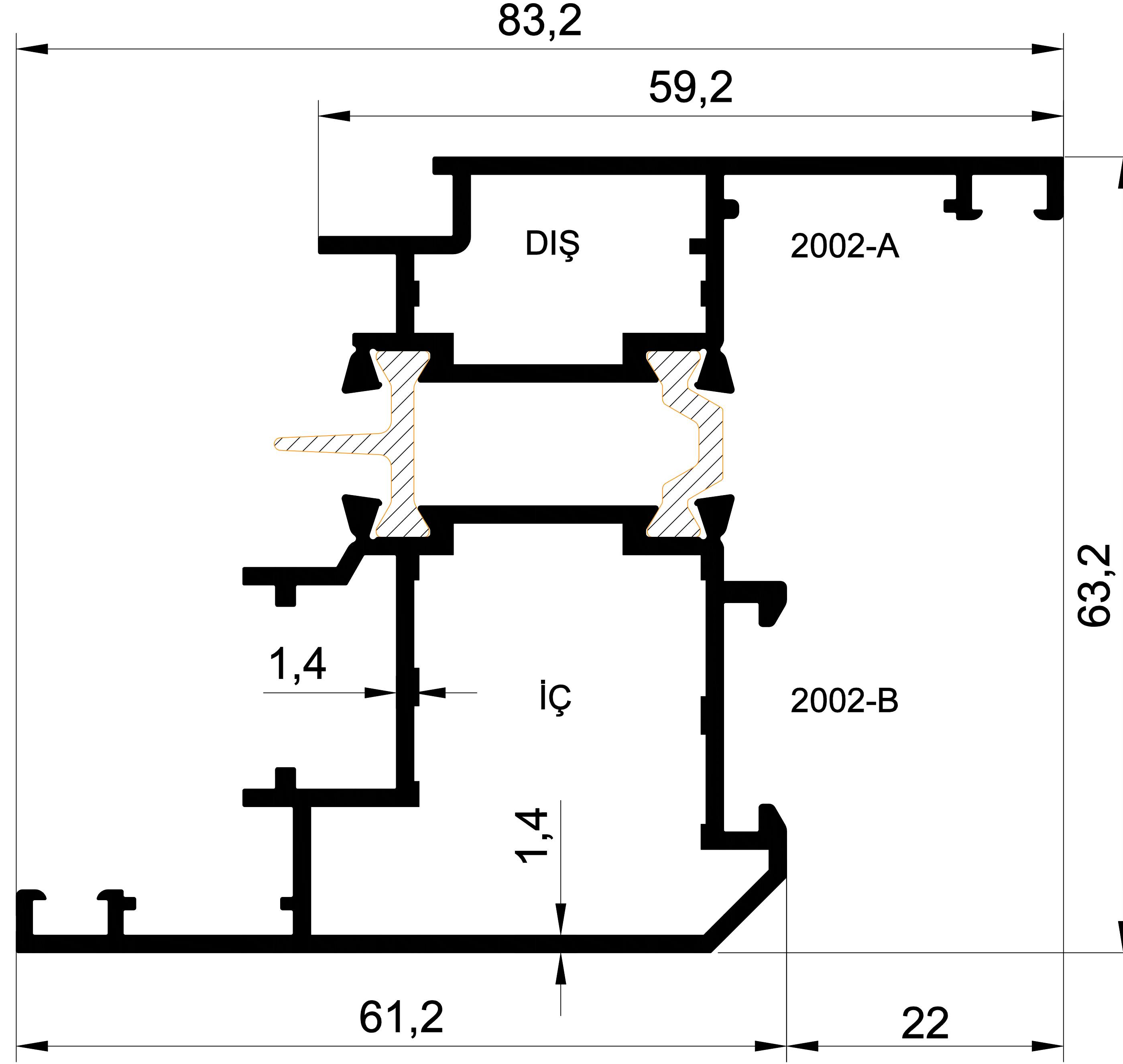
EKL-55- 2002 1,386 gr/m SİSTEM 55 ISI YALITIM KANAT
