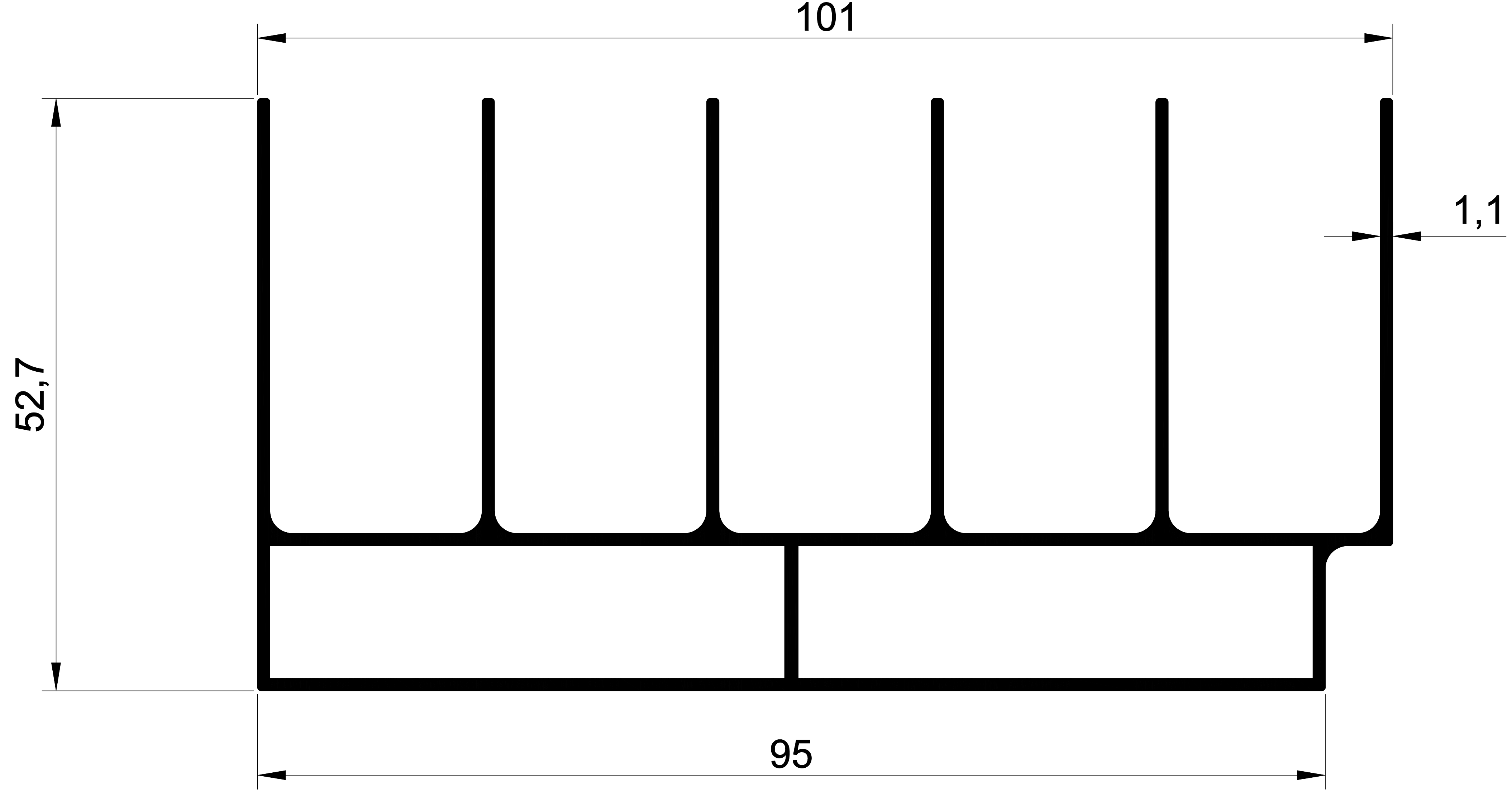
EKOL 1165 1,410 gr/m. SÜRME KASA
