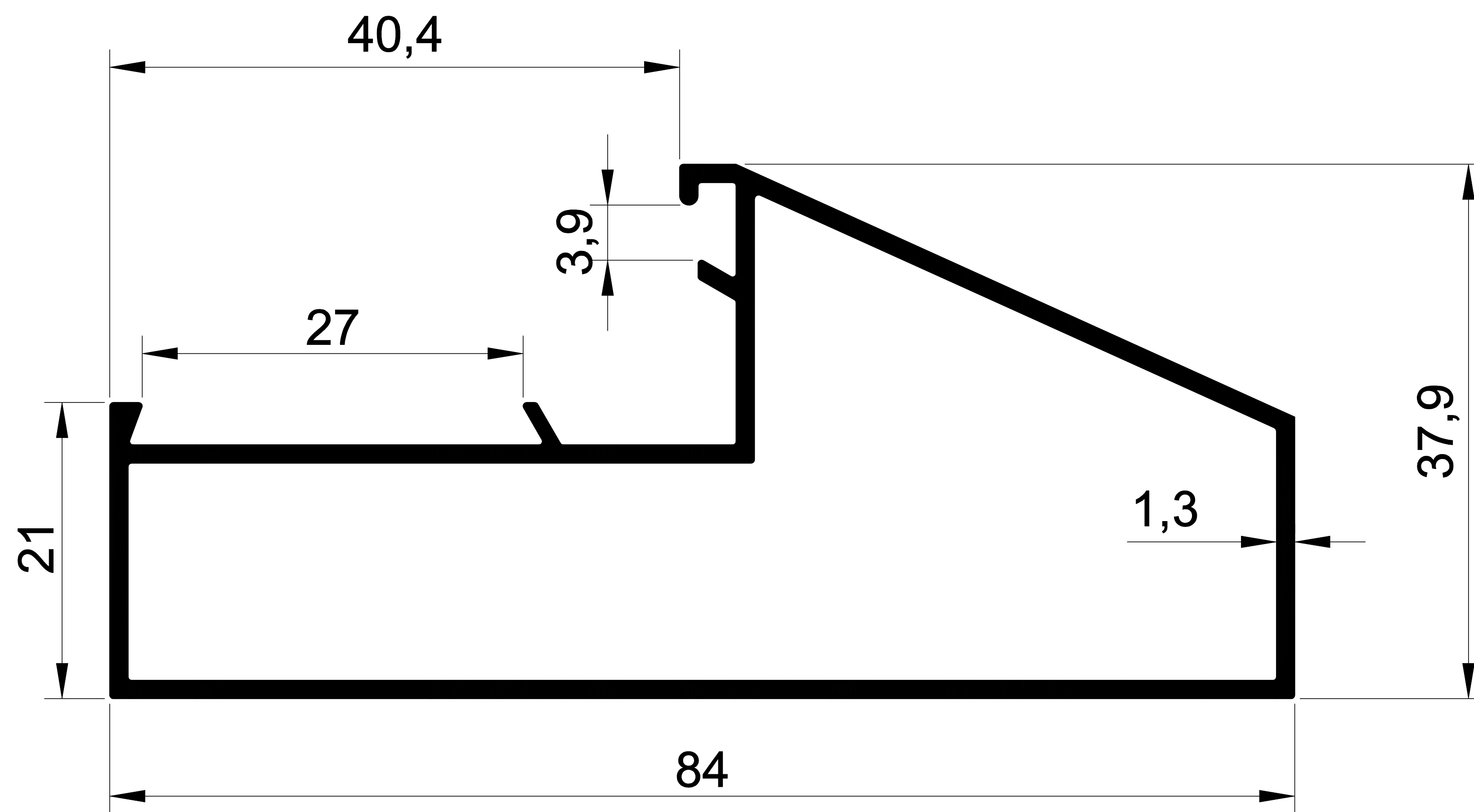
EKOL 1415 0,846 gr/m. JALUZİ OFİS BÖLME KAPI KASASI
