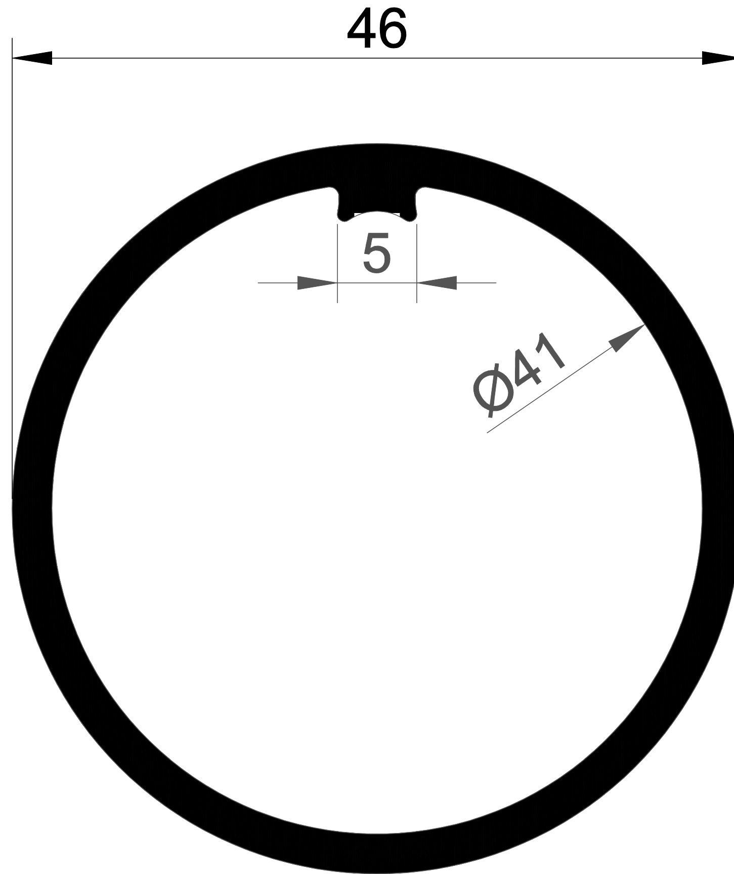
EKOL 1018-B 0,954 gr/m.
