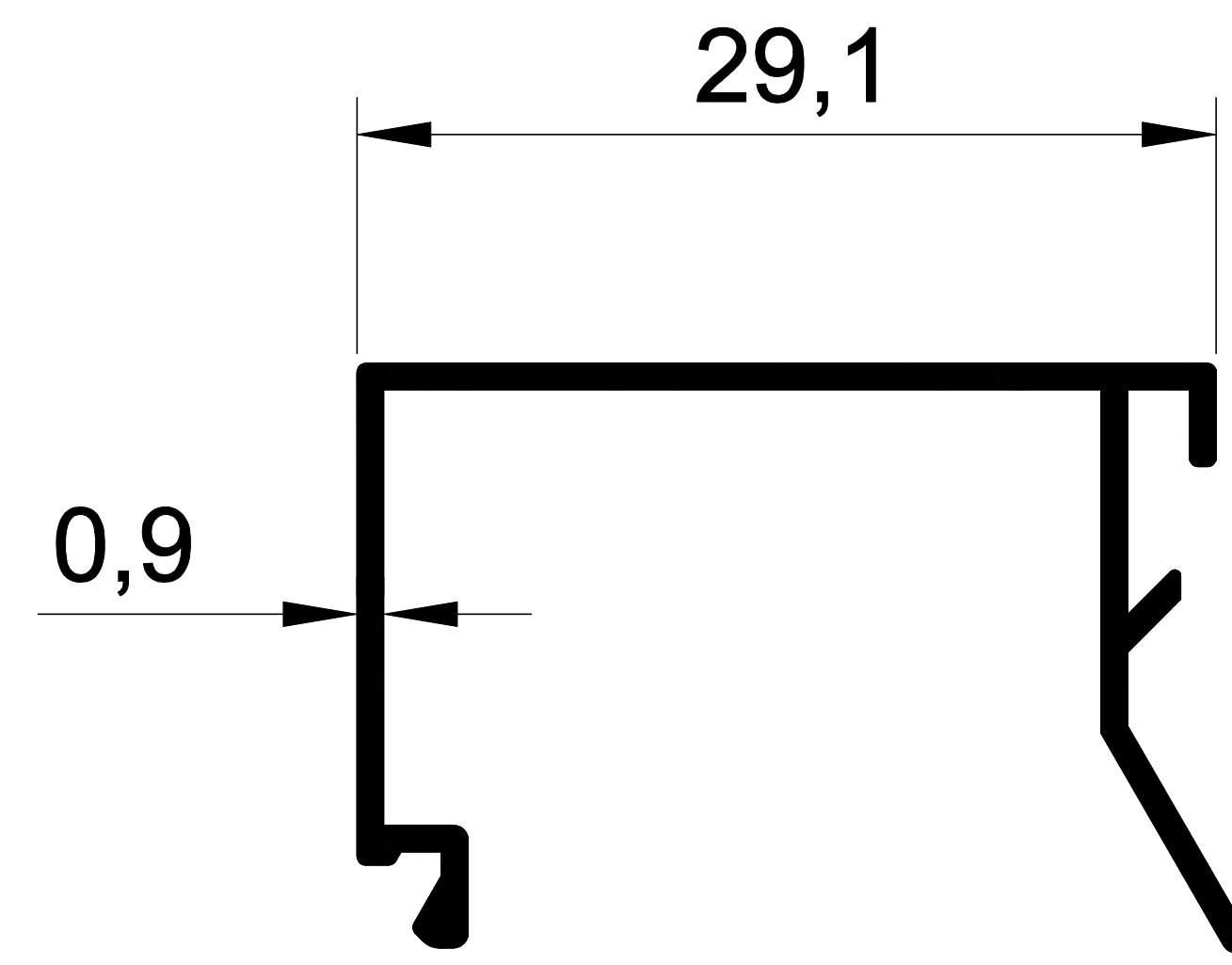
EKOL 1090 0,191 gr/m ALDOKS TEK CAM ÇİTASI
