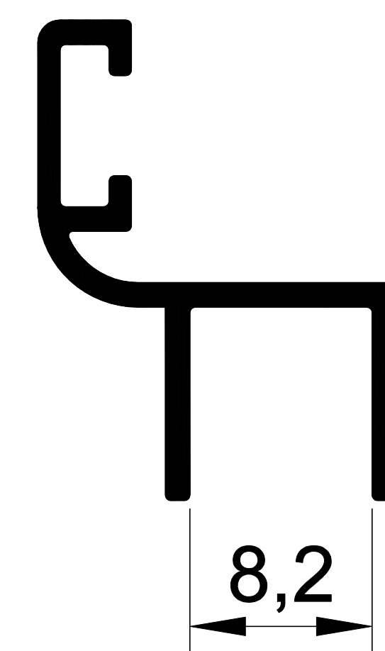
EKOL 1170 0,152 gr/m. CAM H
