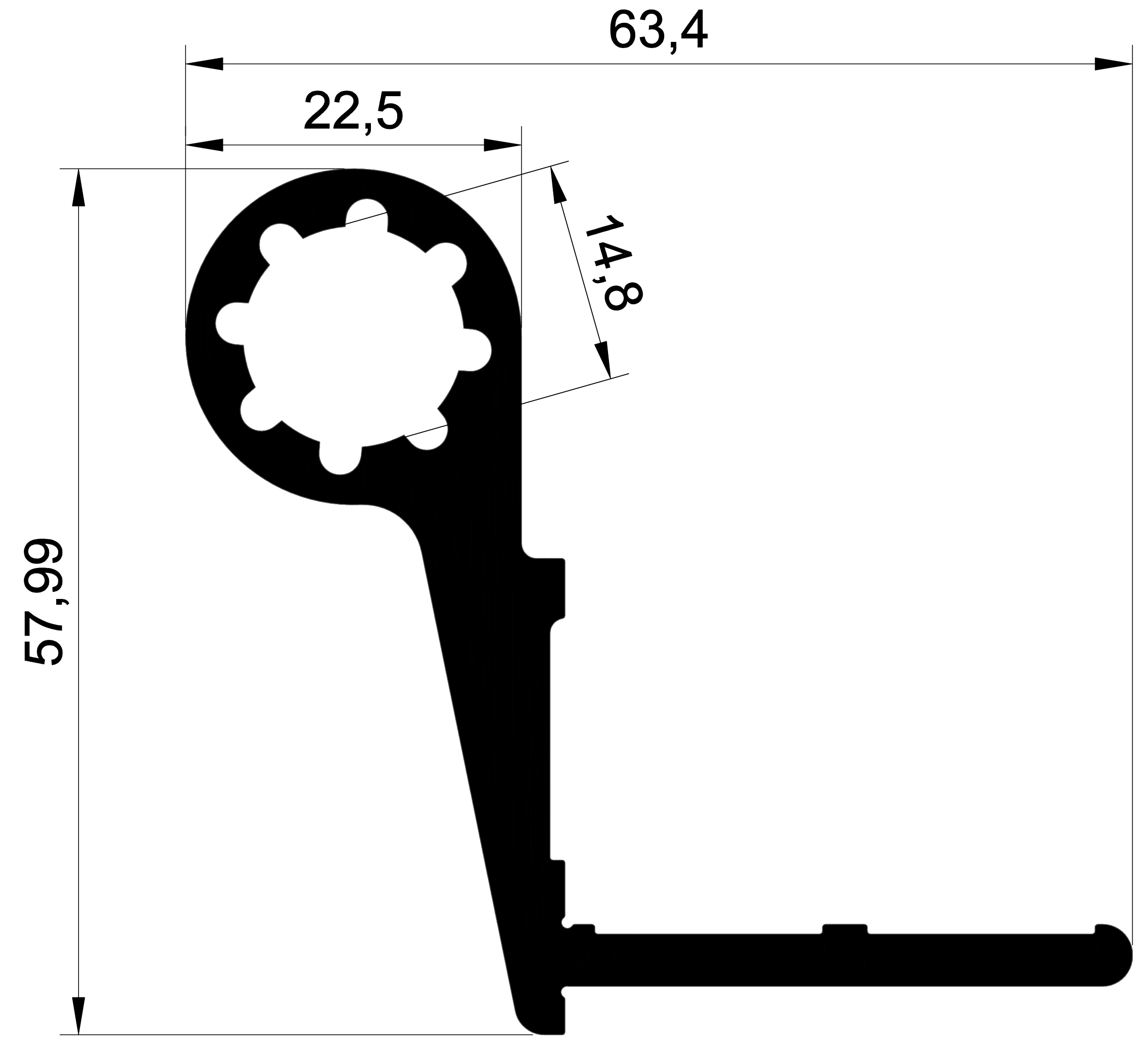
EKOL 1011-B 1,521 gr/m.
