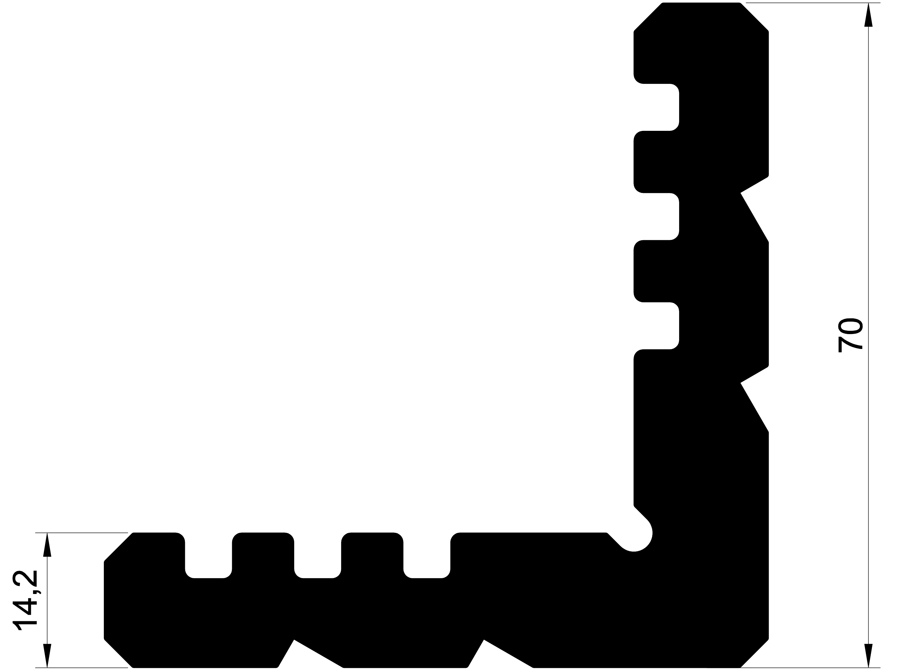
EKOL 1402 1,402 gr/m. 14'LÜK CEPHE KÖŞE
