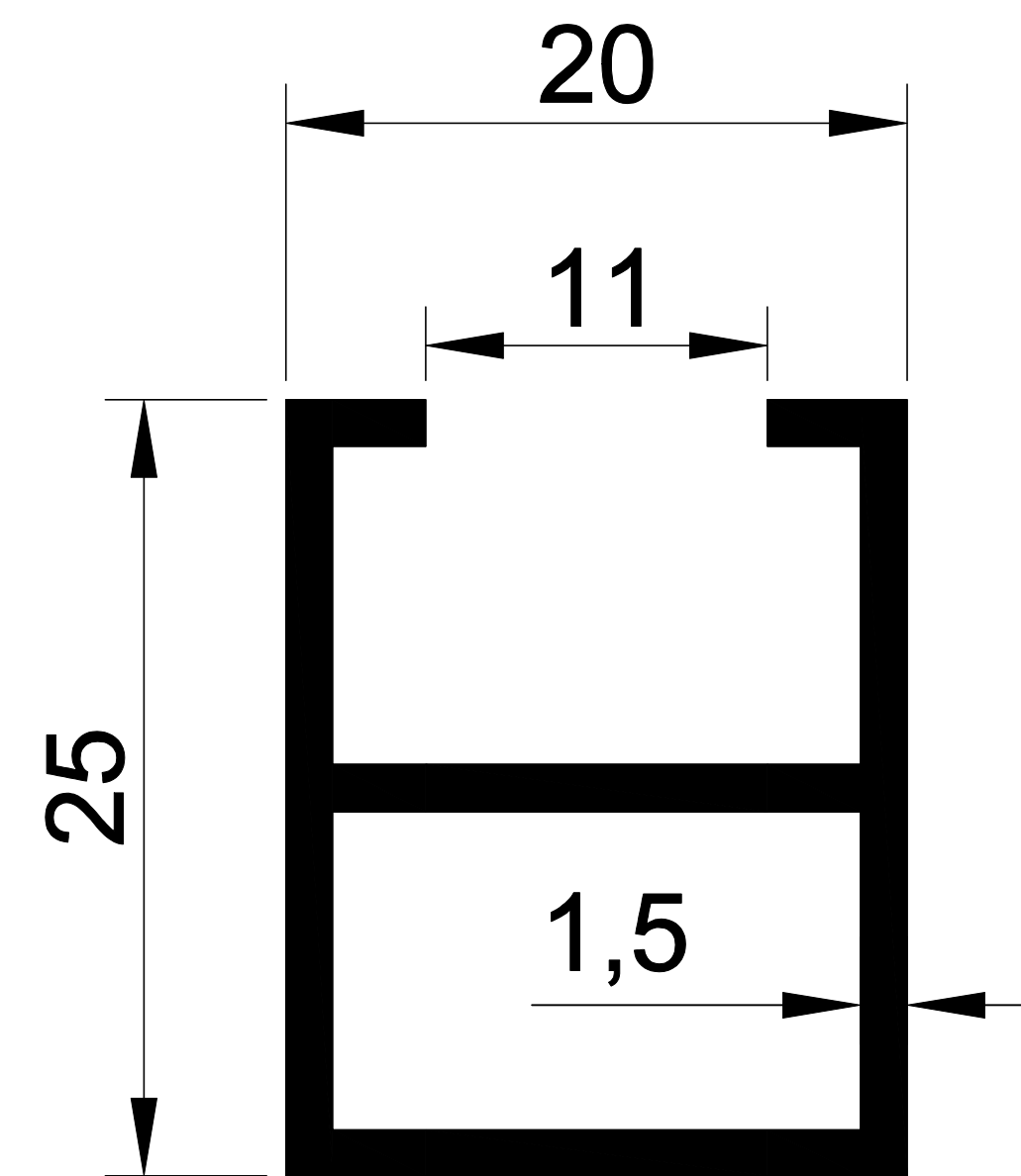
EKOL 1141 0,366 gr/m. MİNİ GEMİCİ
