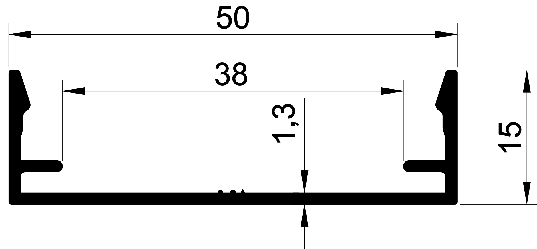
EKOL 1397 0,324 gr/m. 15 MM CEPHE KAPAK
