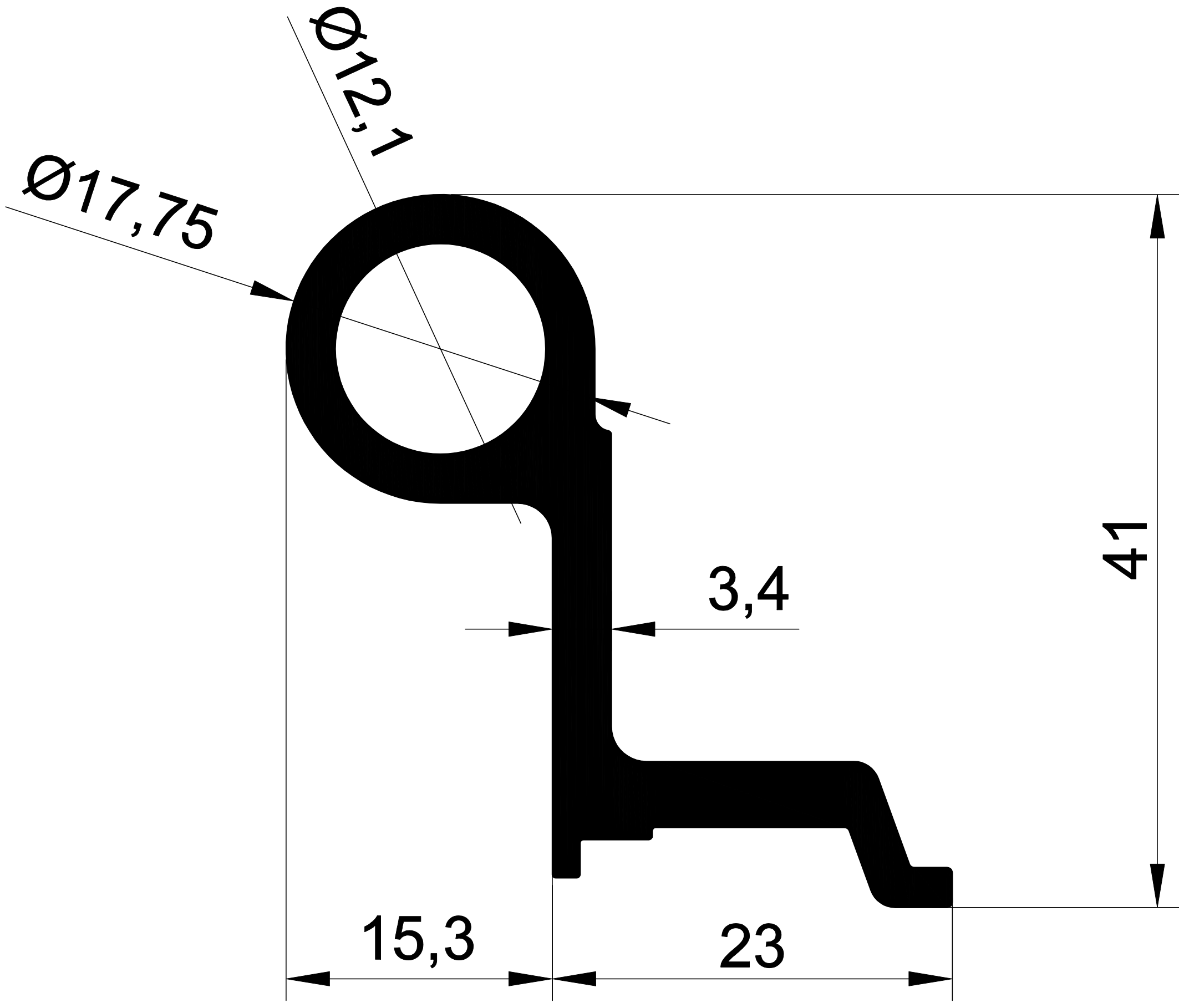
EKOL 1463 0,819 gr/m
