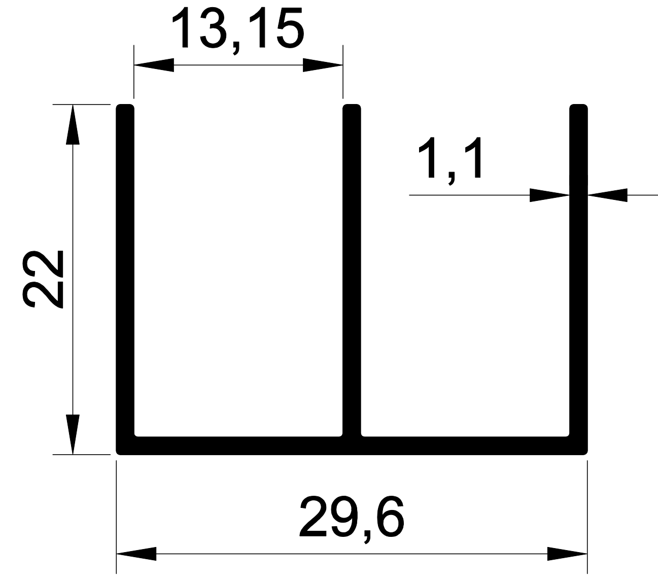
EKOL 1408 0,275 gr/m. MOBİLYA E PROFİLİ
