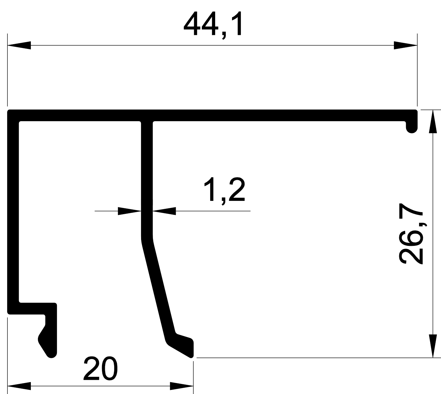
EKOL 1405 0,336 gr/m. BİM TEK CAM ÇİTASI
