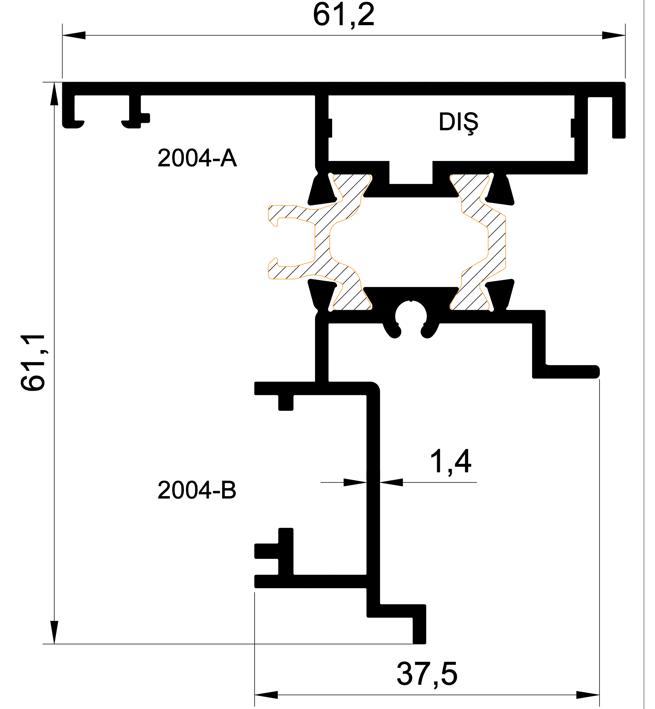
EKL-55- 2004 1,039 gr/m SİSTEM 55 ISI YALITIM ÇİFT KANAT ADAPTÖR
