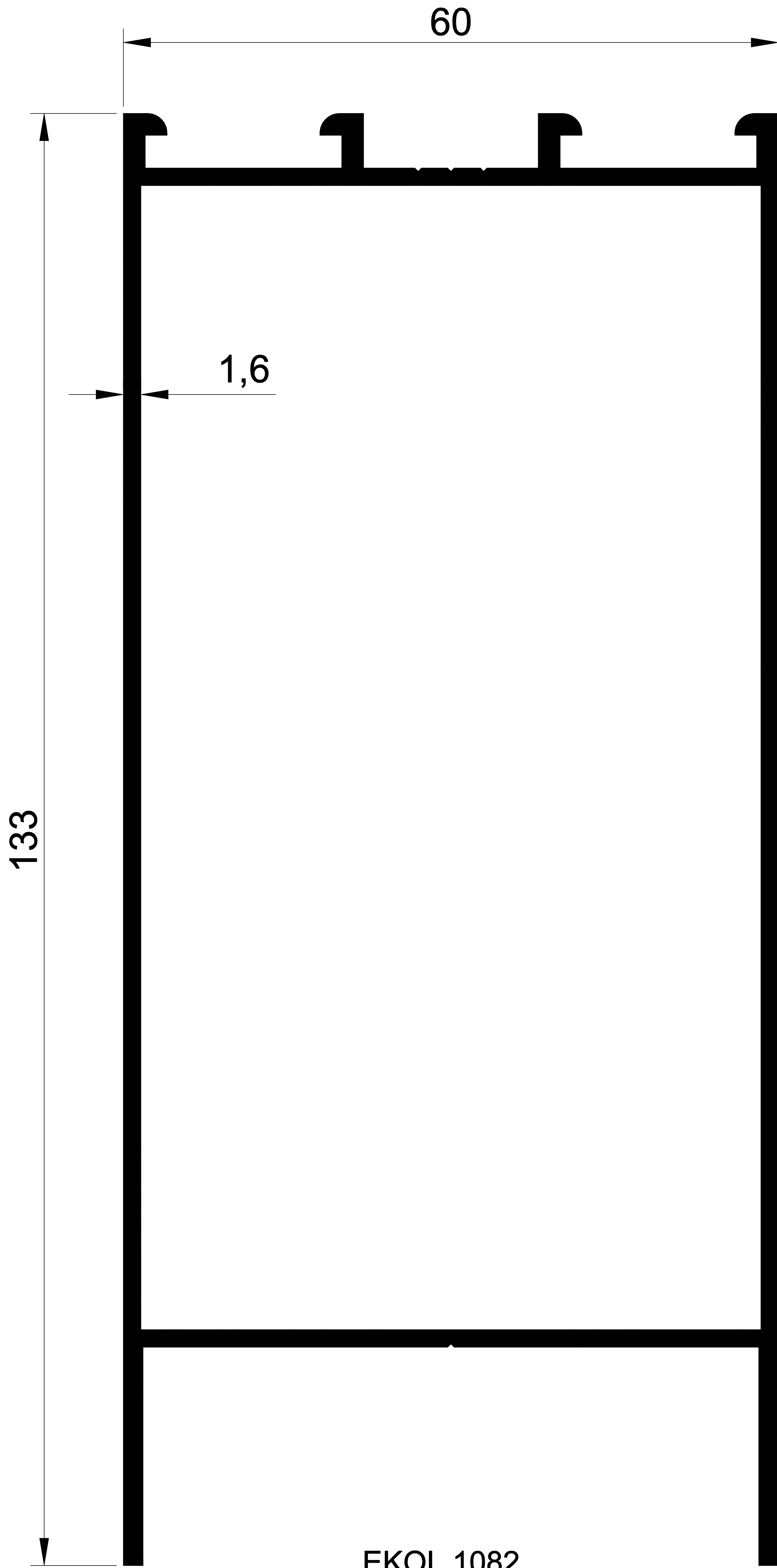
EKOL 1082 1,767 gr/m. C-60 ETEK
