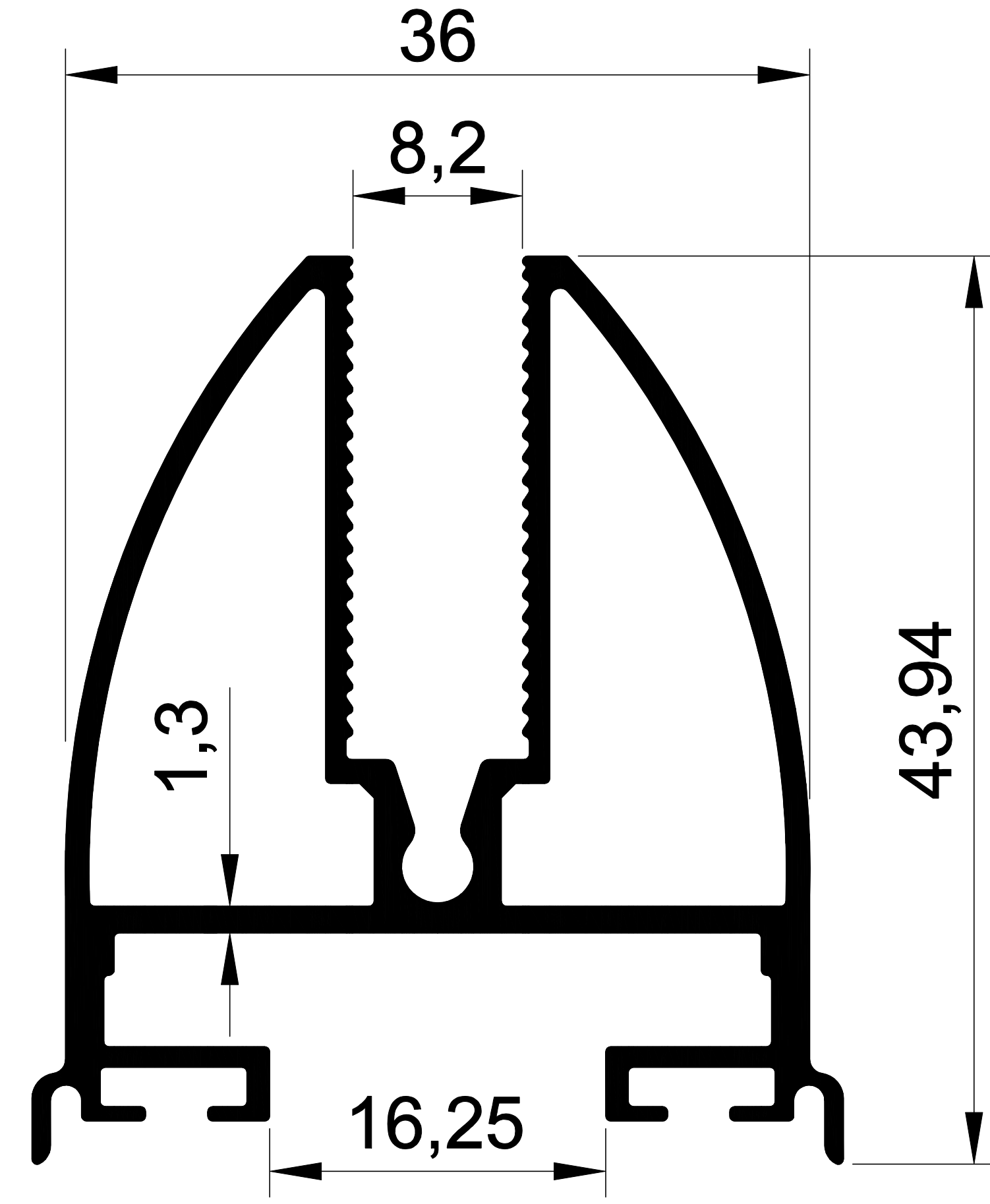
EKOL 1186 0,756 gr/m. BKS KANAT
