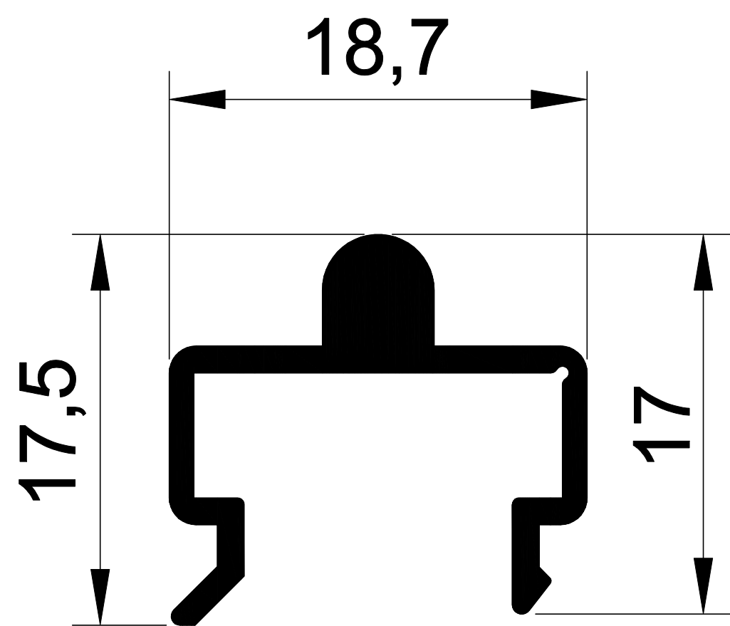
EKOL 1193 0,203 gr/m DAR TUBA RAY
