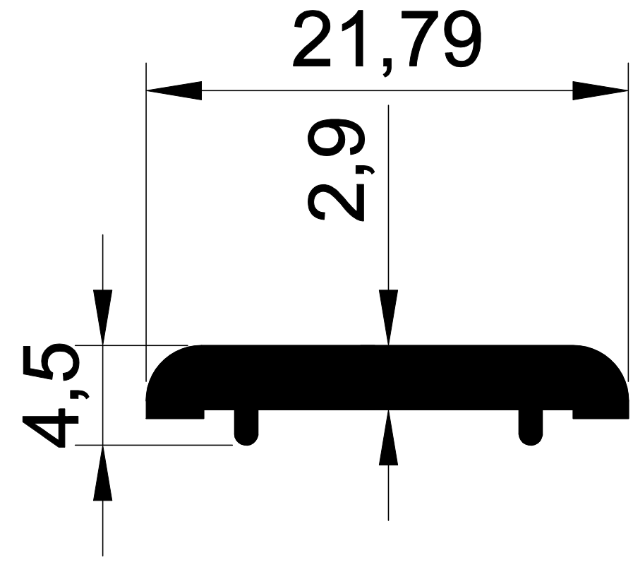
EKOL 1276 0,179 gr/m.
