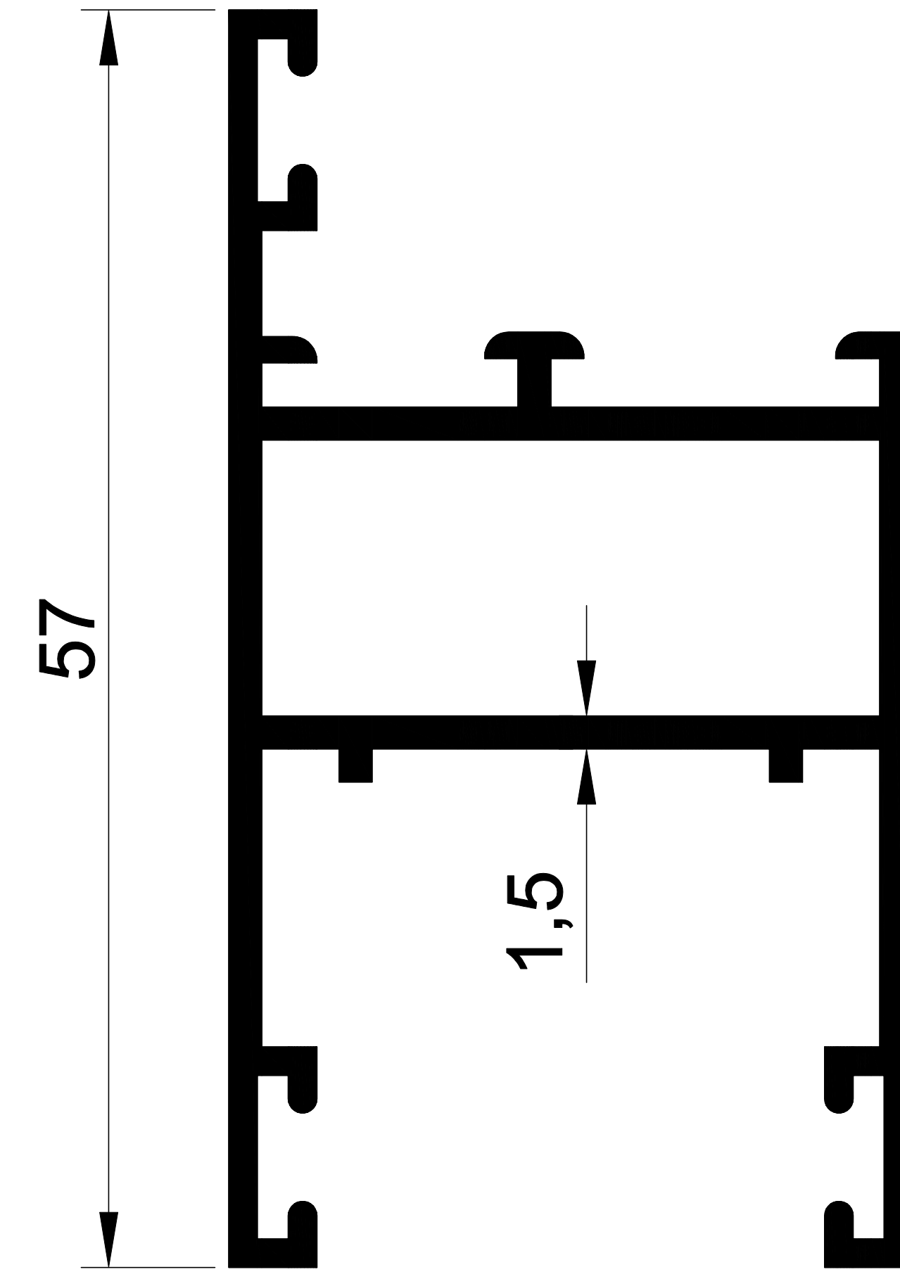
EKOL 1196 0,753 gr/m DAR TUBA KANAT
