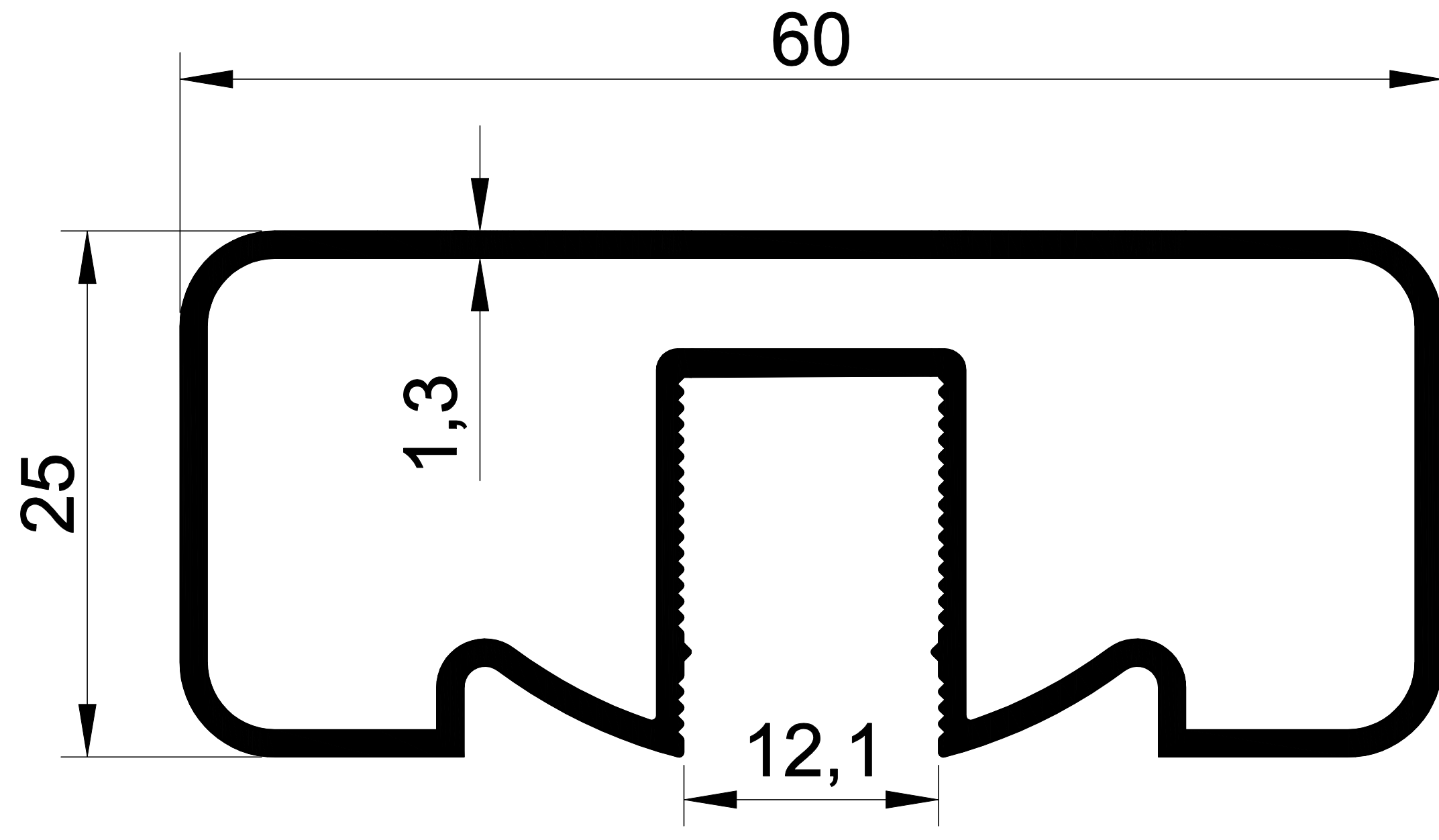
EKOL 1129 0,706 gr/m. 25X60 ORTADAN CAMLI
