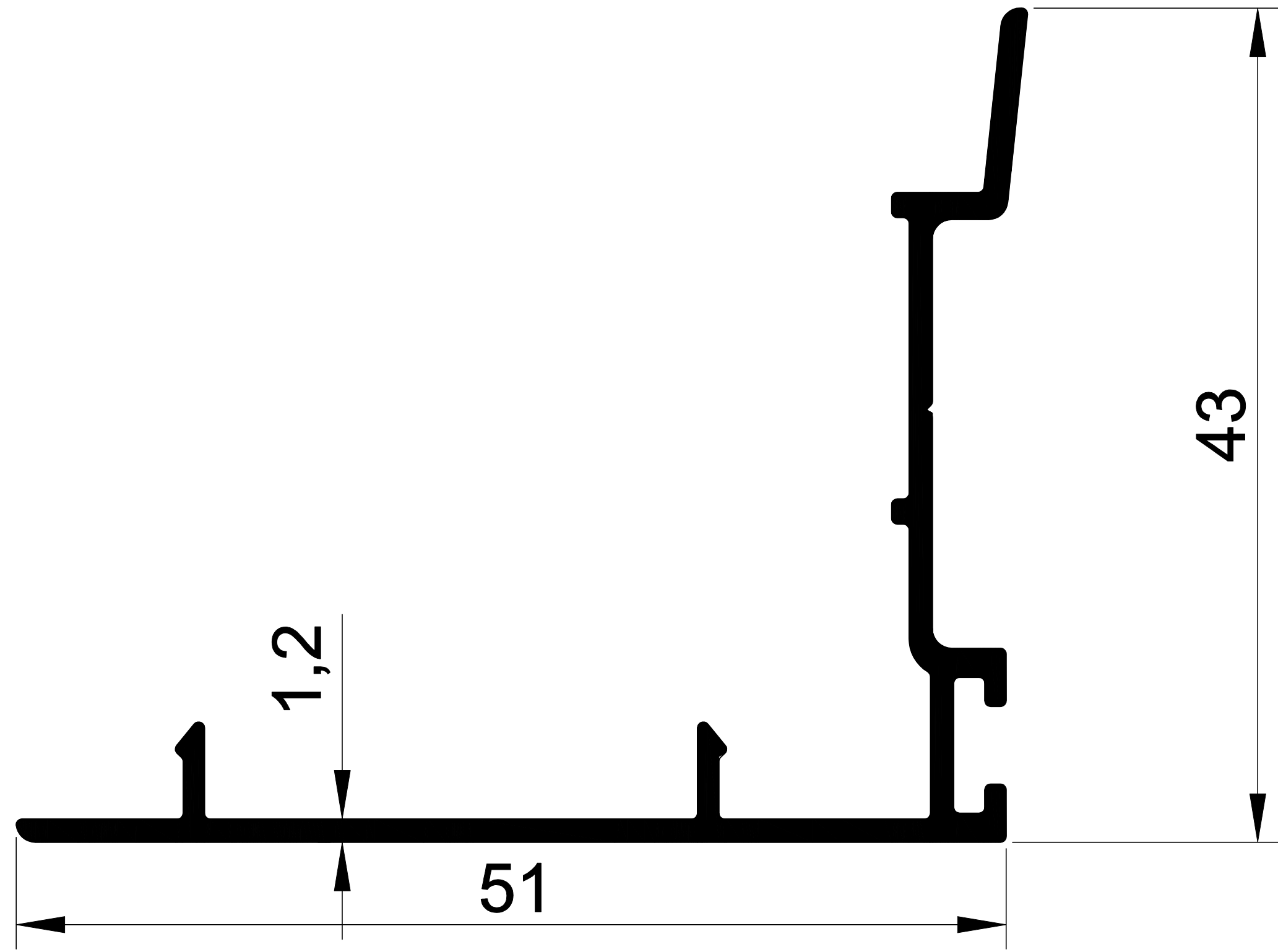
EKOL 1387 0,379 gr/m. 100'LÜK TUBA KENET
