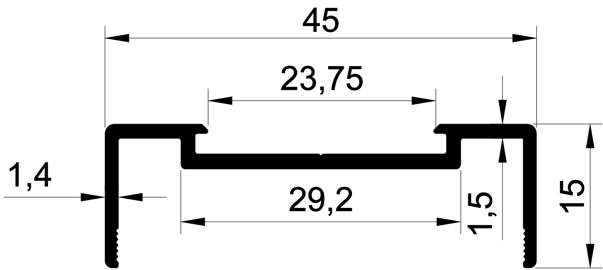
EKOL 1419 0,320 gr/m. MS-AHŞAP KANAT ÇERÇEVESİ
