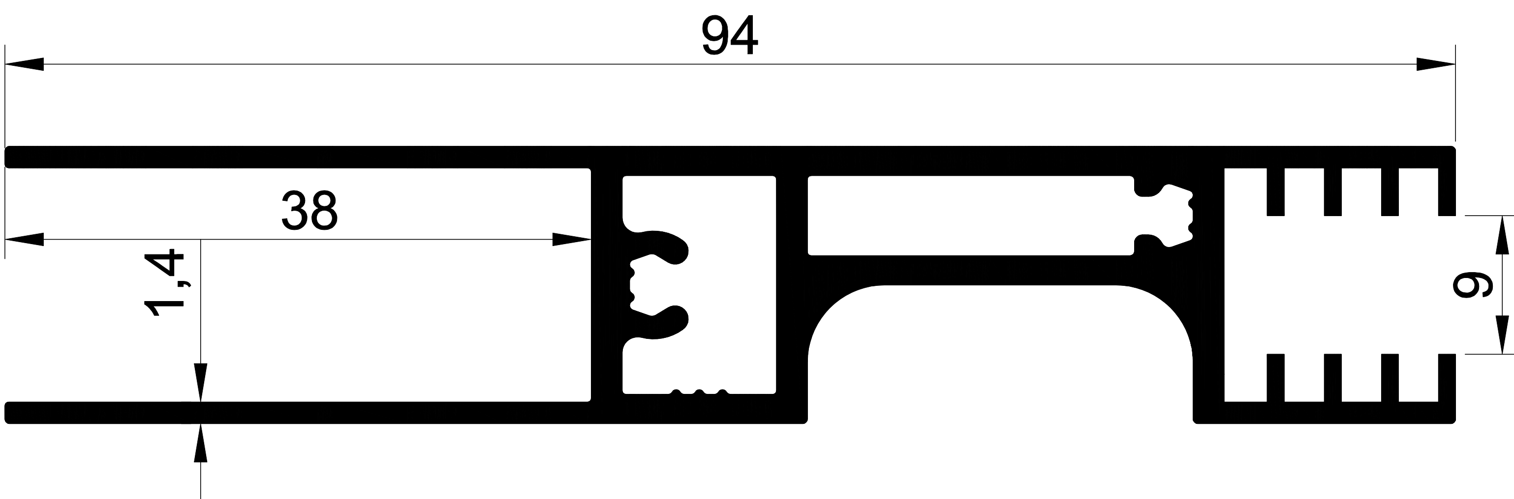
EKOL 1167 1,225 gr/m. SÜRME ALT KANAT
