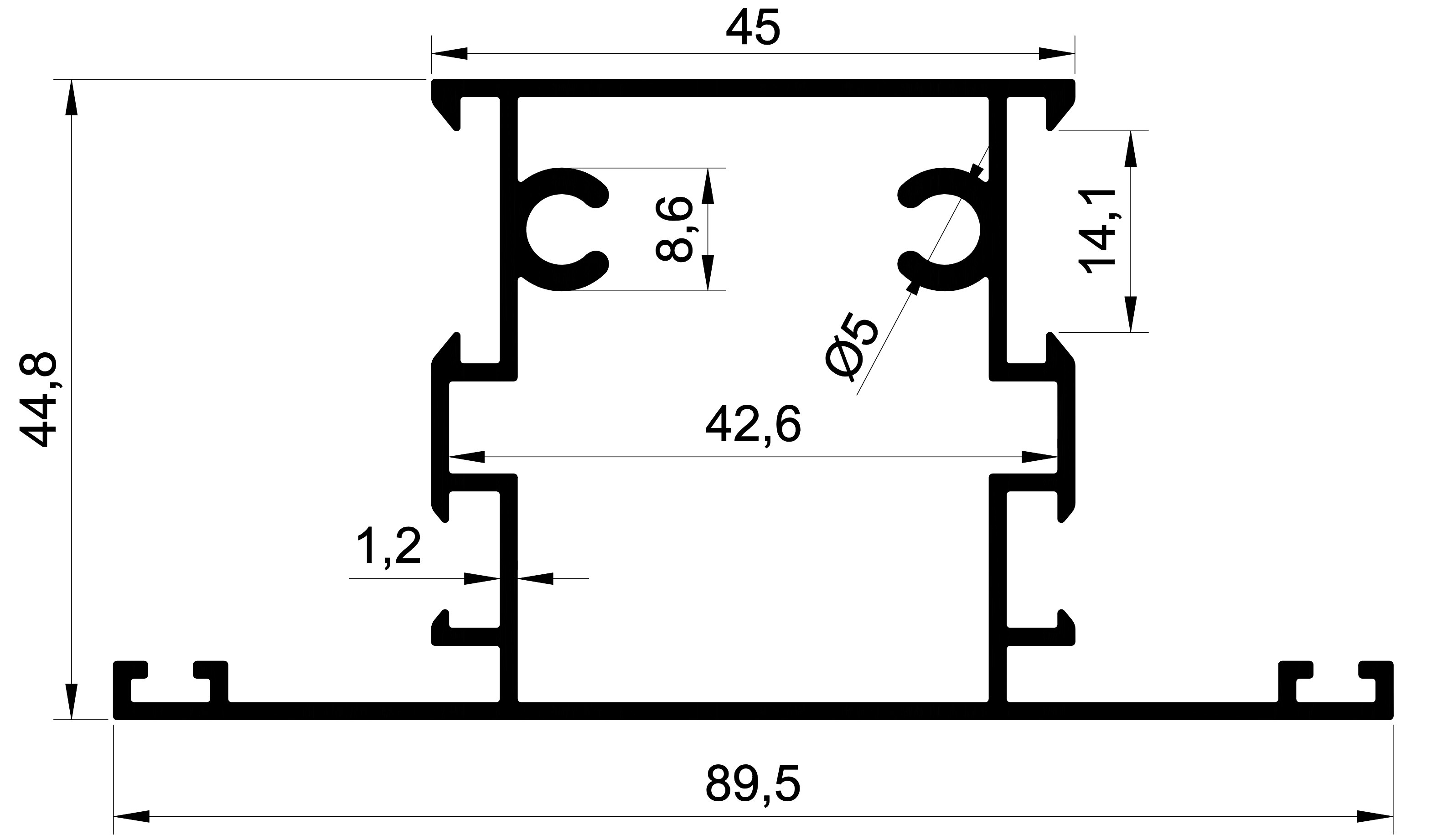
EKOL 1372 1,054 gr/m. OVAL ORTA
