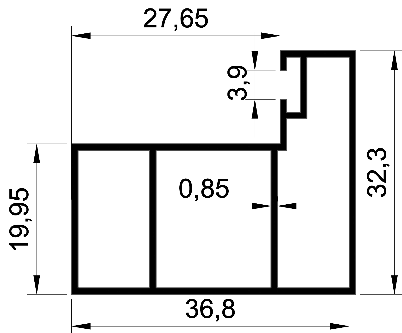
EKOL 1450 0,411 gr/m. BKS DİKME
