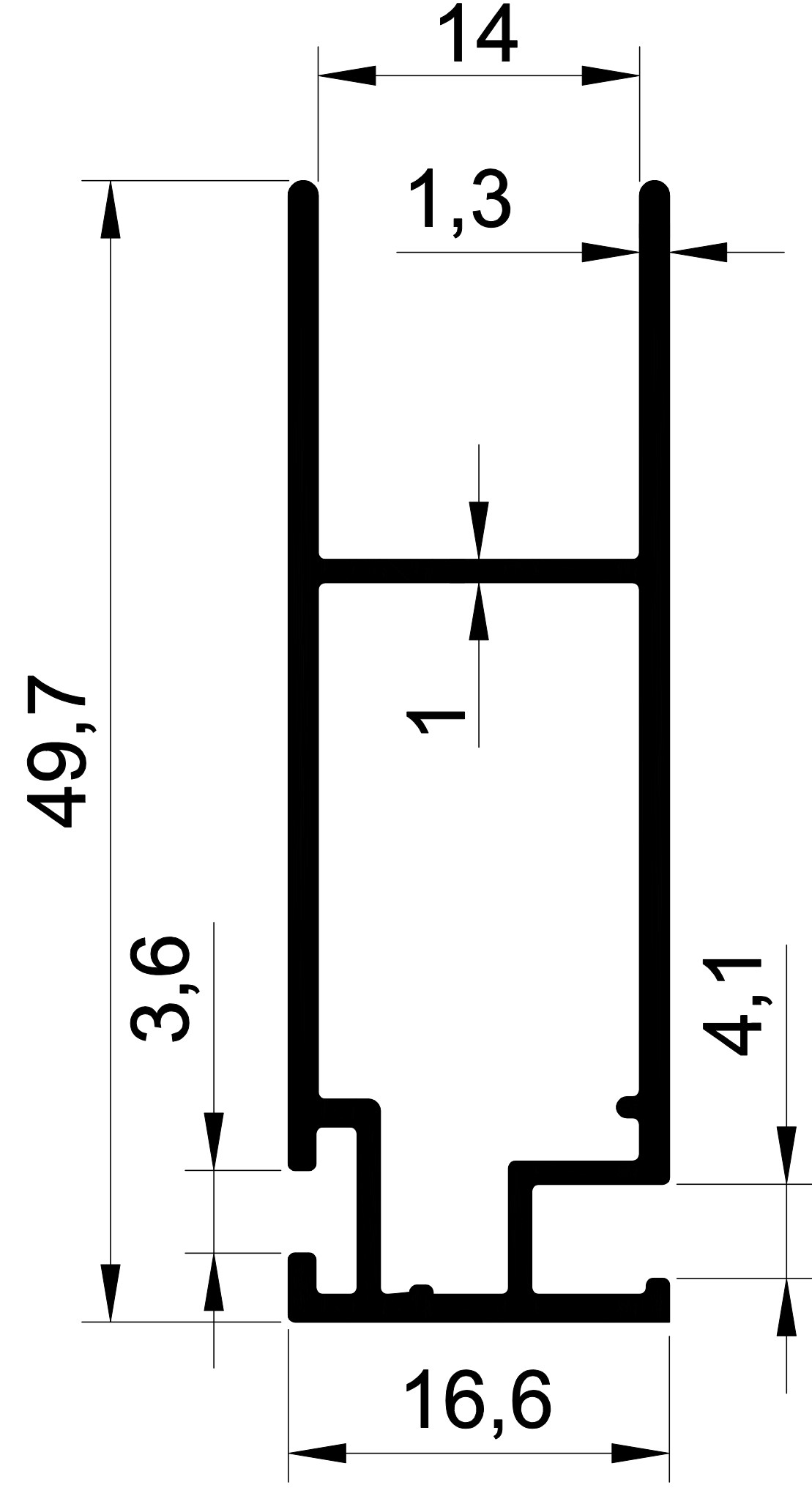
EKOL 1373 0,464 gr/m. AYKİM KANAT
