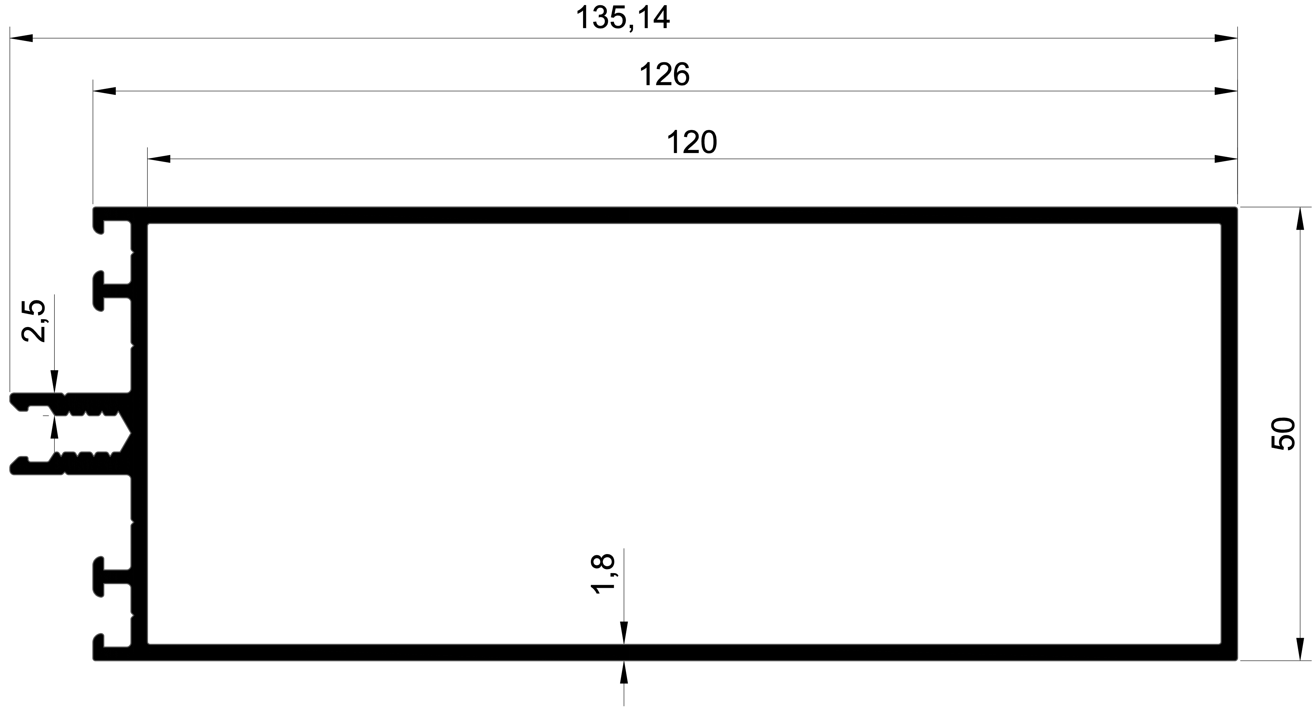
EKOL 1446 1,894 gr/m. 126'LIK CEPHE PROFİLİ
