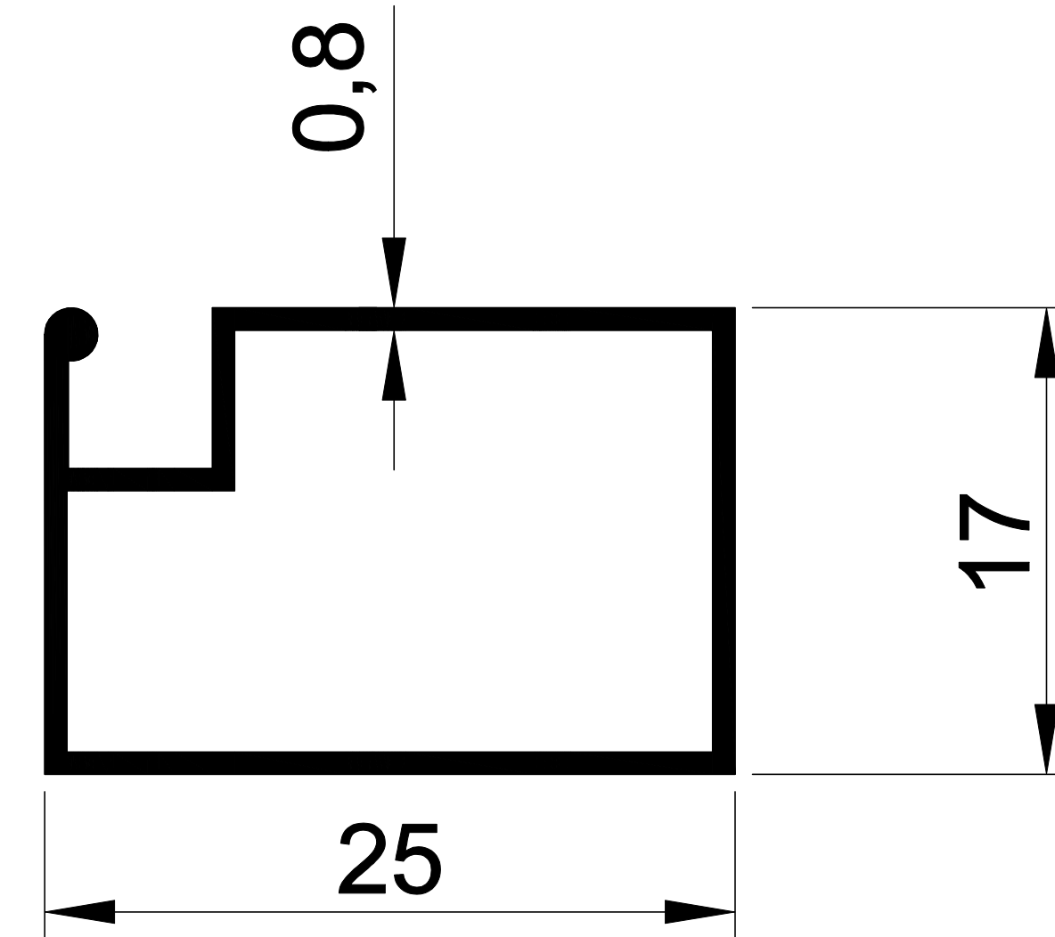
EKOL 1072 0,169 gr/m. 17*25 SİNEKLİK
