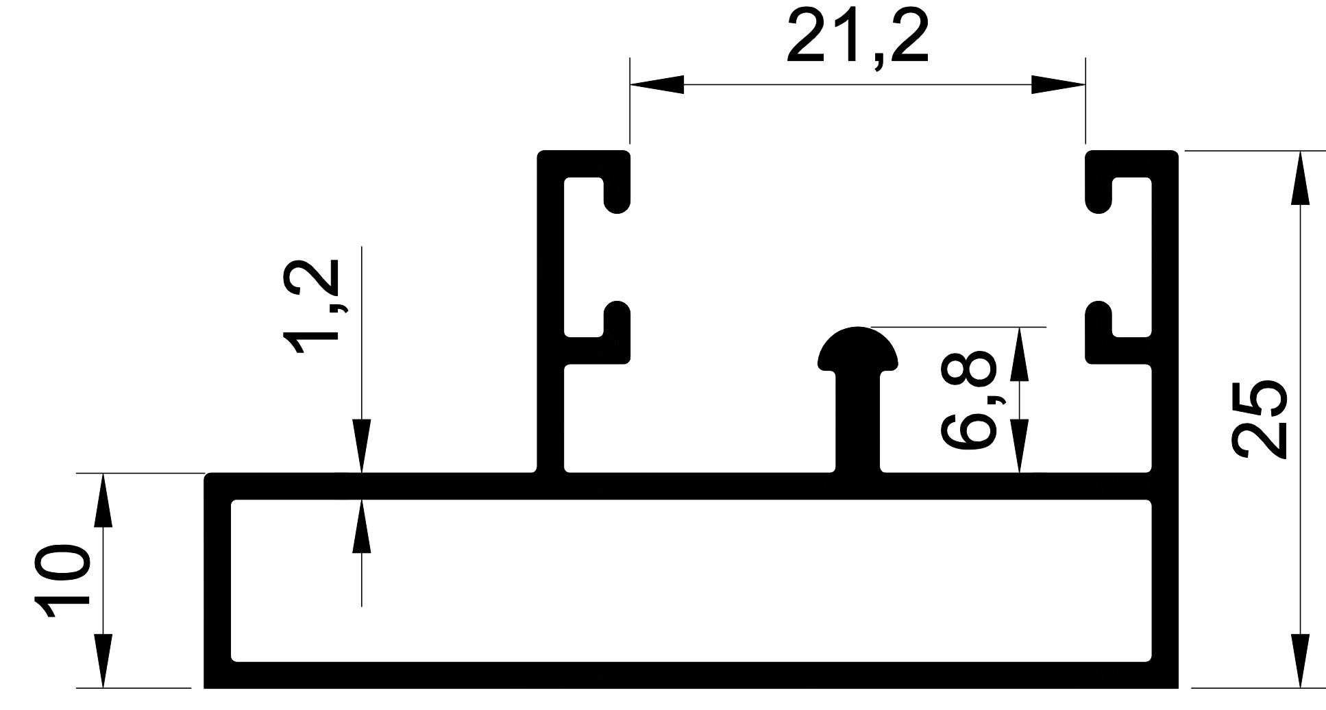
EKOL 1374 0,545 gr/m. AYKİM KASA
