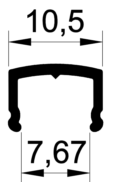
EKOL 1437 0.070 gr/m. ÖZEL DİKME KAPAĞI
