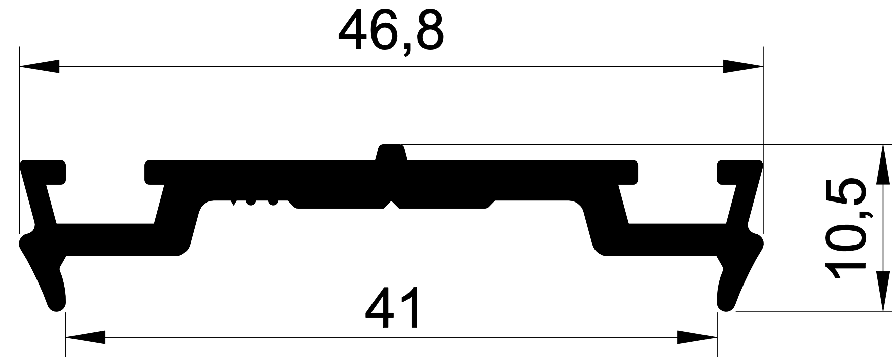
EKOL 1395 0,428 gr/m. CEPHE KAPAK ALTI
