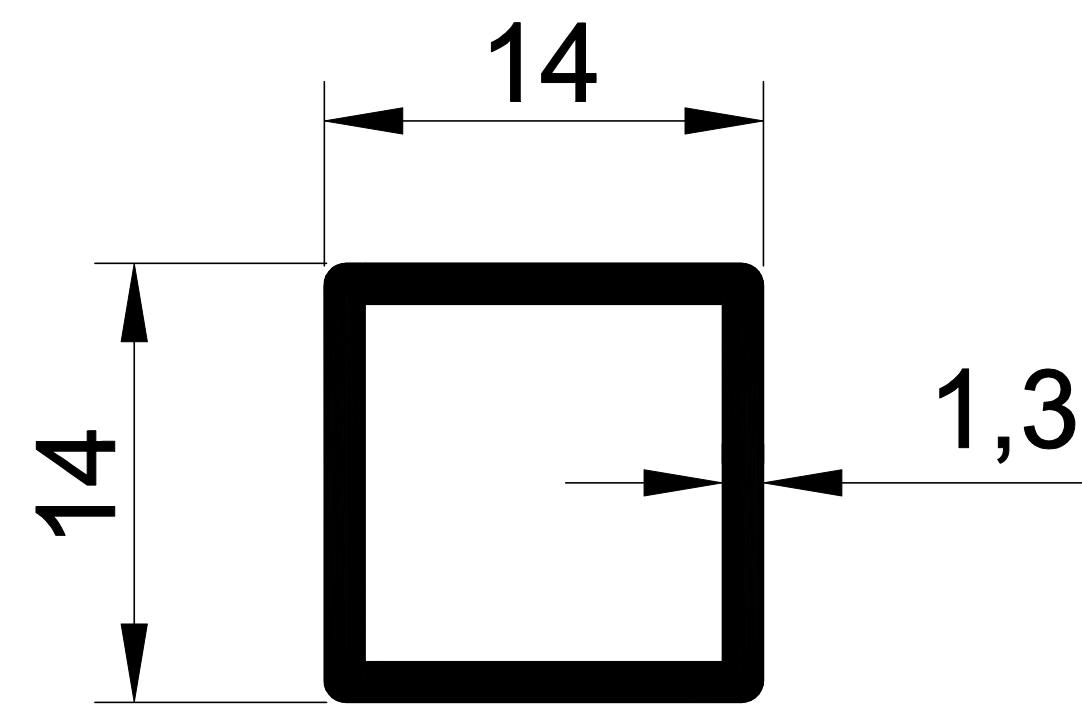
EKOL 1131 0,179 gr/m. 14X14 BARIYER
