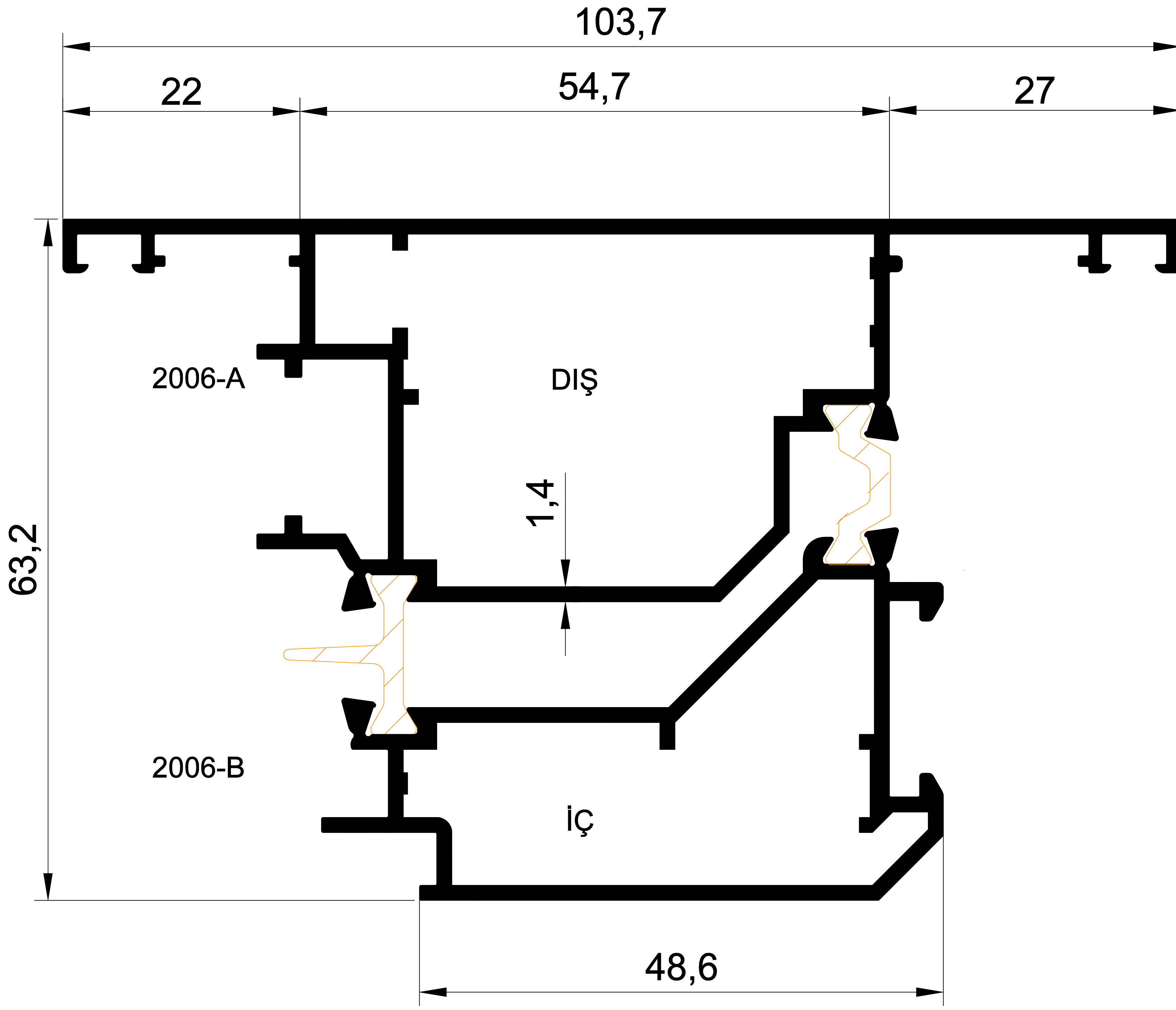
EKL-55- 2006 1,794 gr/m SİSTEM 55 ISI YALITIM DIŞA AÇILIR KAPI
