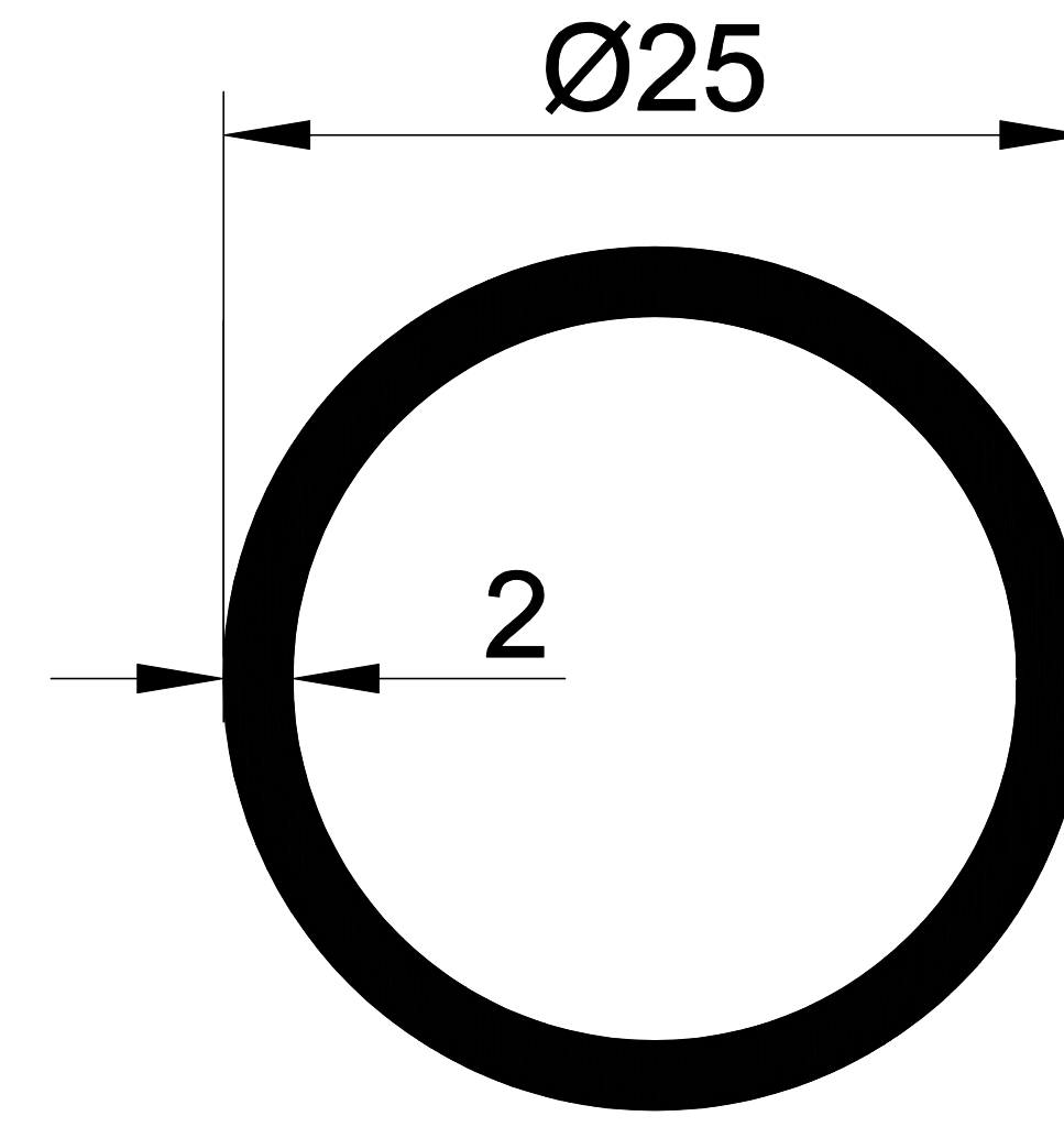
EKOL 1287 0,393 gr/m.
