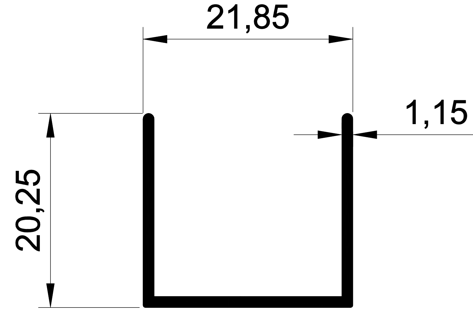
EKOL 1158 0,187 gr/m. 20 mm U PROFİL (KOMBİ U'SU)
