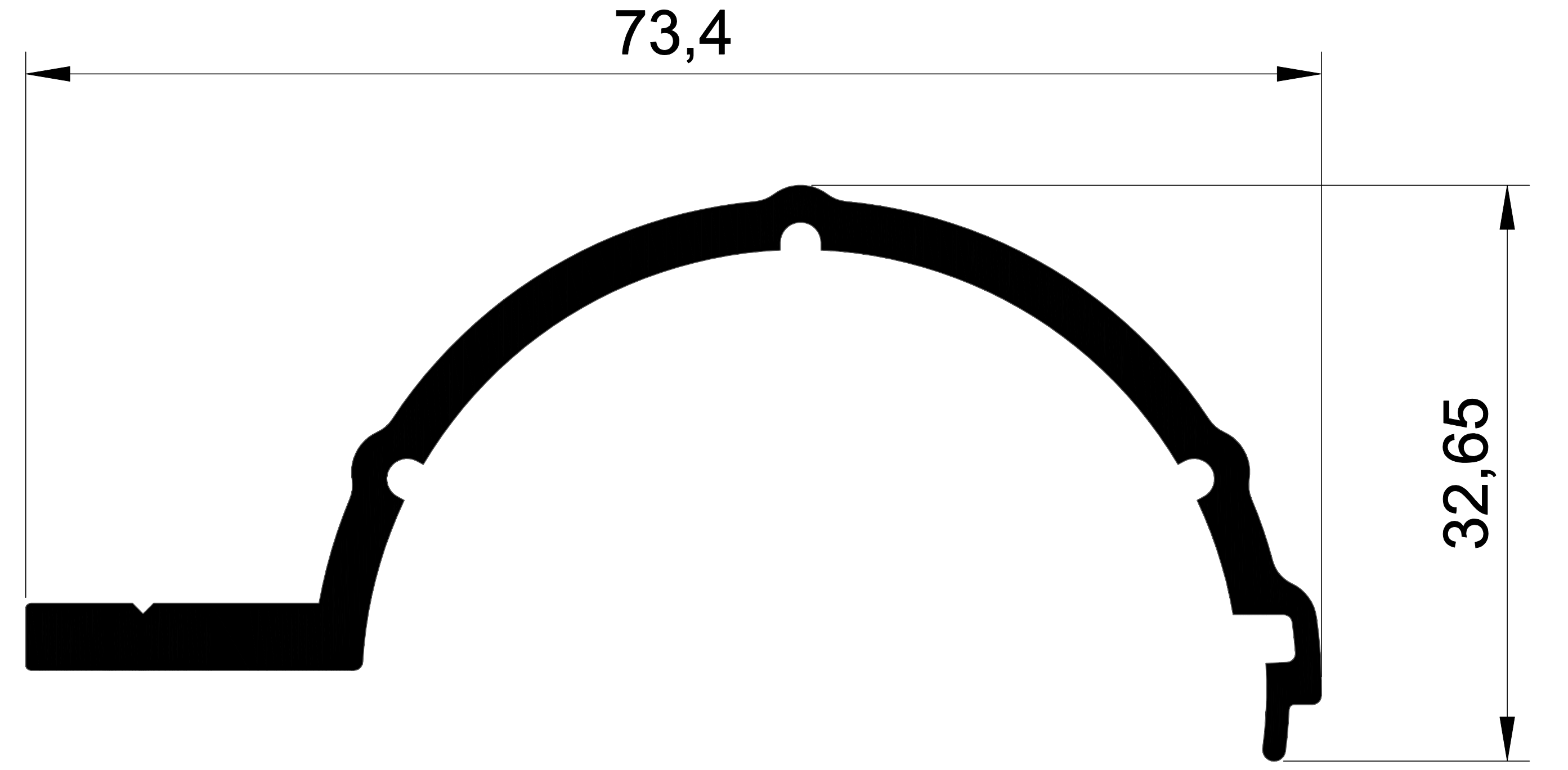
EKOL 1323 0,807 gr/m.
