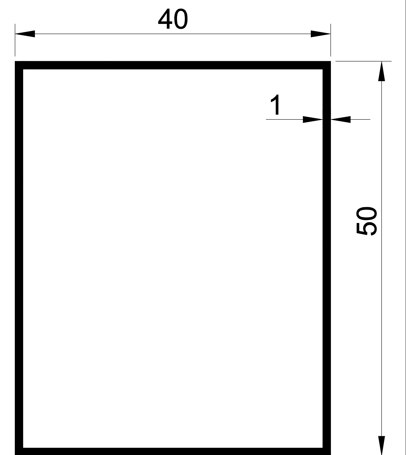
EKOL 1093 0,545 gr/m.
