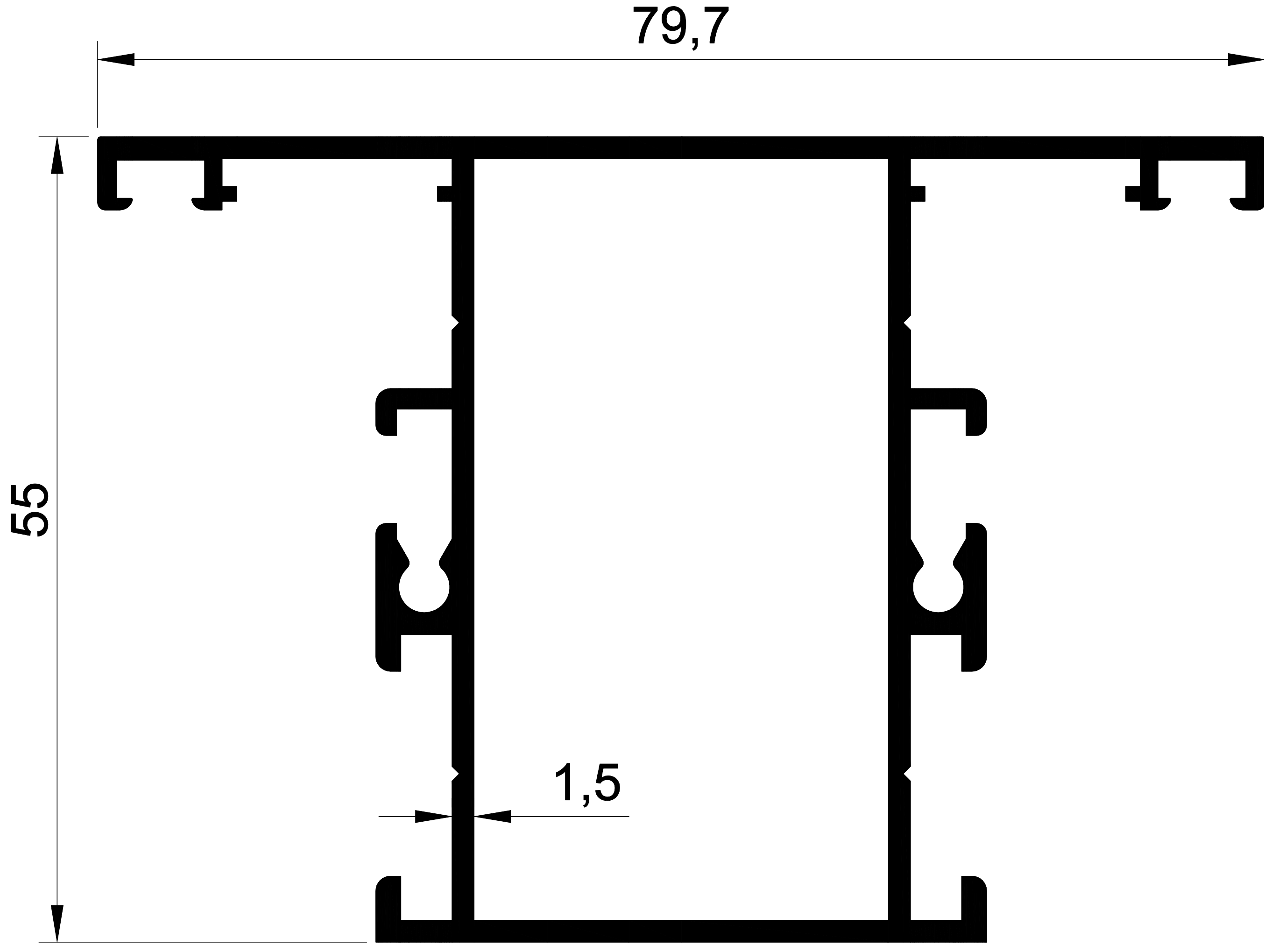
EKOL 1199 1,195 gr/m. SİSTEM ORTA
