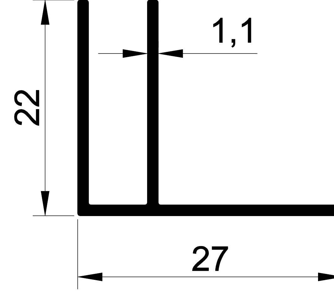
EKOL 1409 0,205 gr/m. MOBİLYA F PROFİLİ
