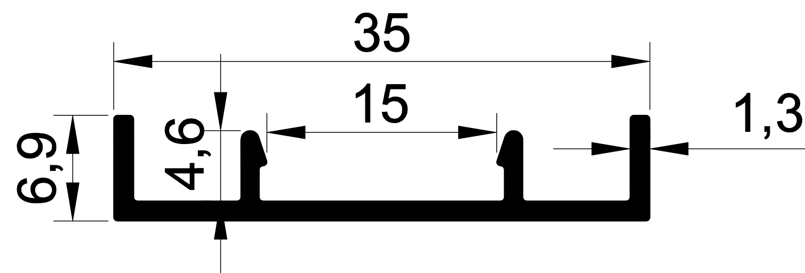
EKOL 1416 0,195 gr/m. JALUZİ OFİS BÖLME KAPAK
