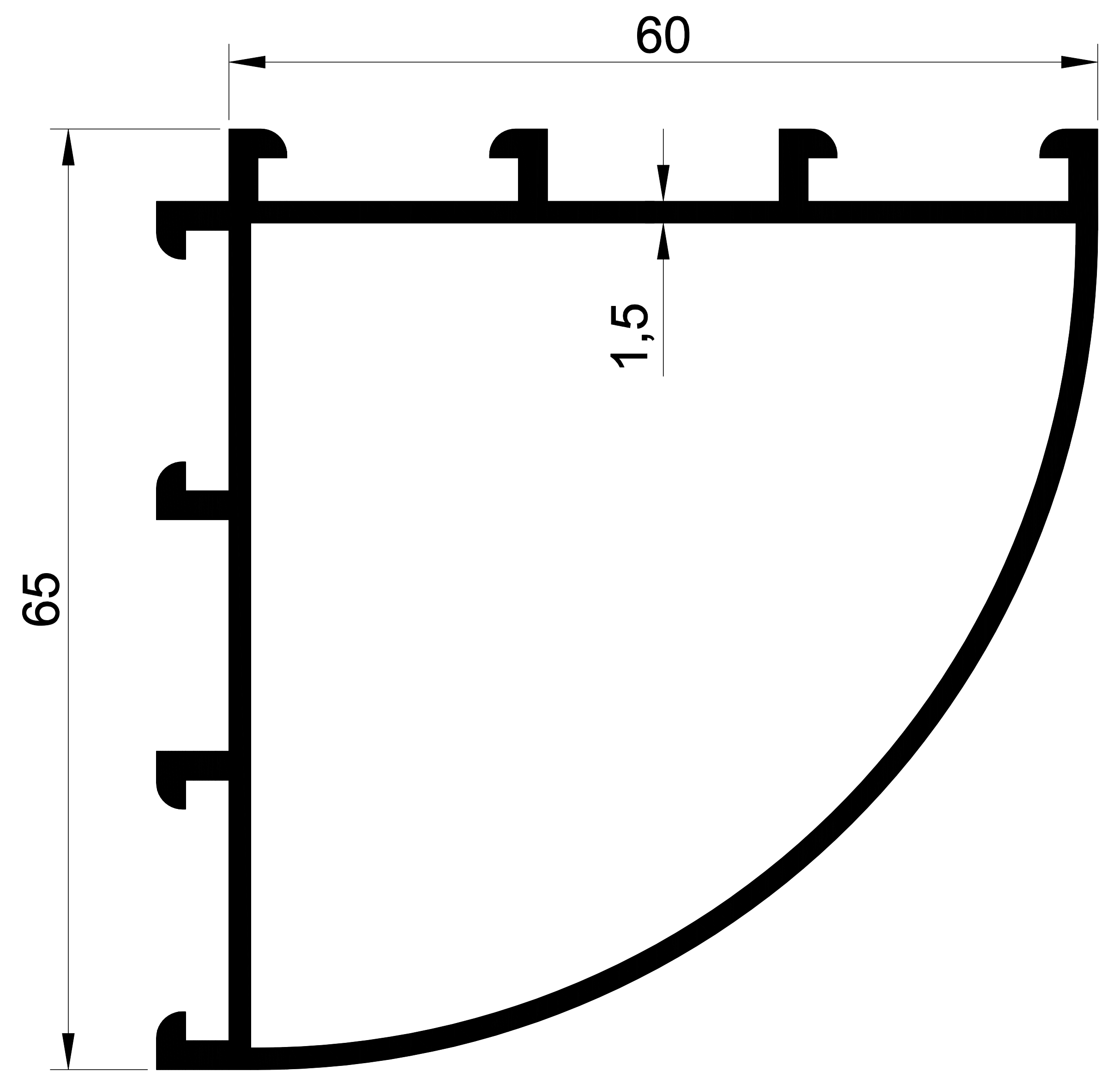
EKOL 1083 1,138 gr/m. C-60 OVAL KÖŞE DÖNÜŞ
