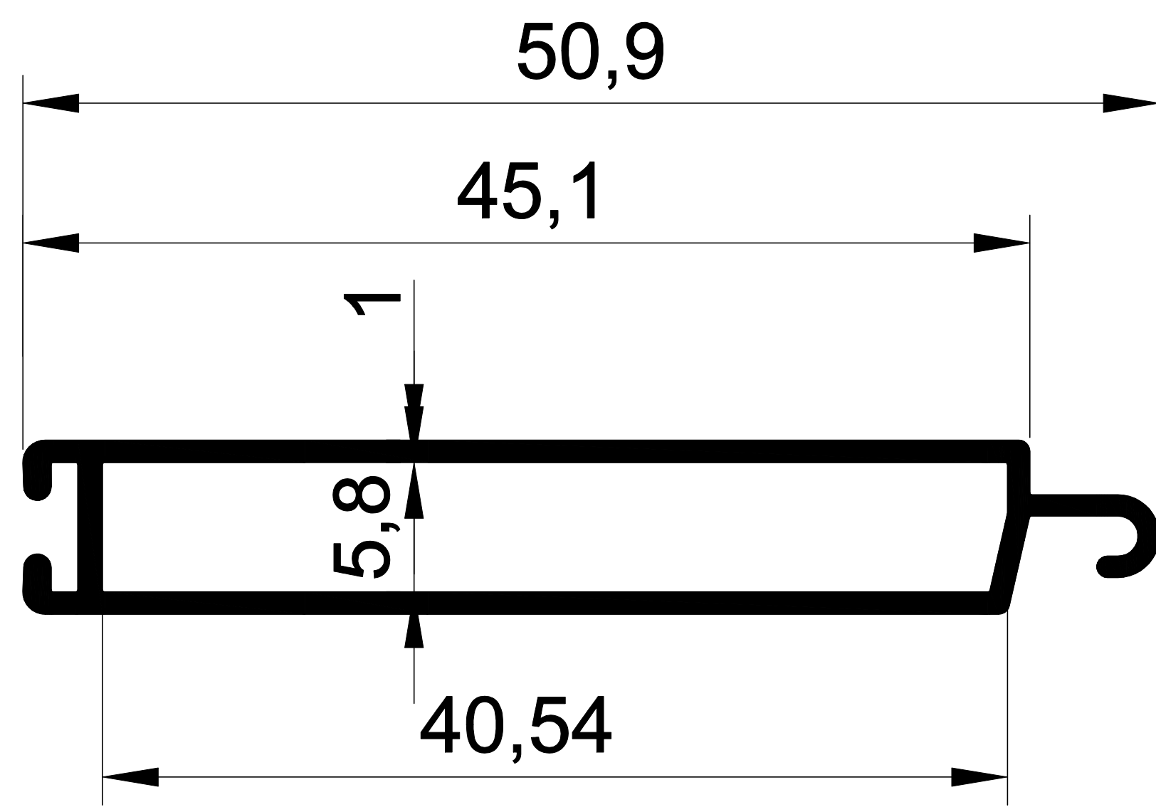
EKOL 1309 0,309 gr/m. ALT PARÇA
