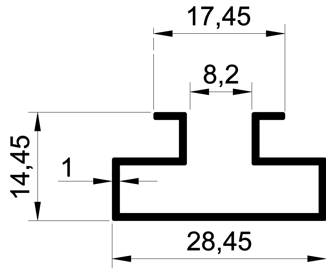
EKOL 1154 0,217 gr/m. RAF ASKILIK PROFİLİ
