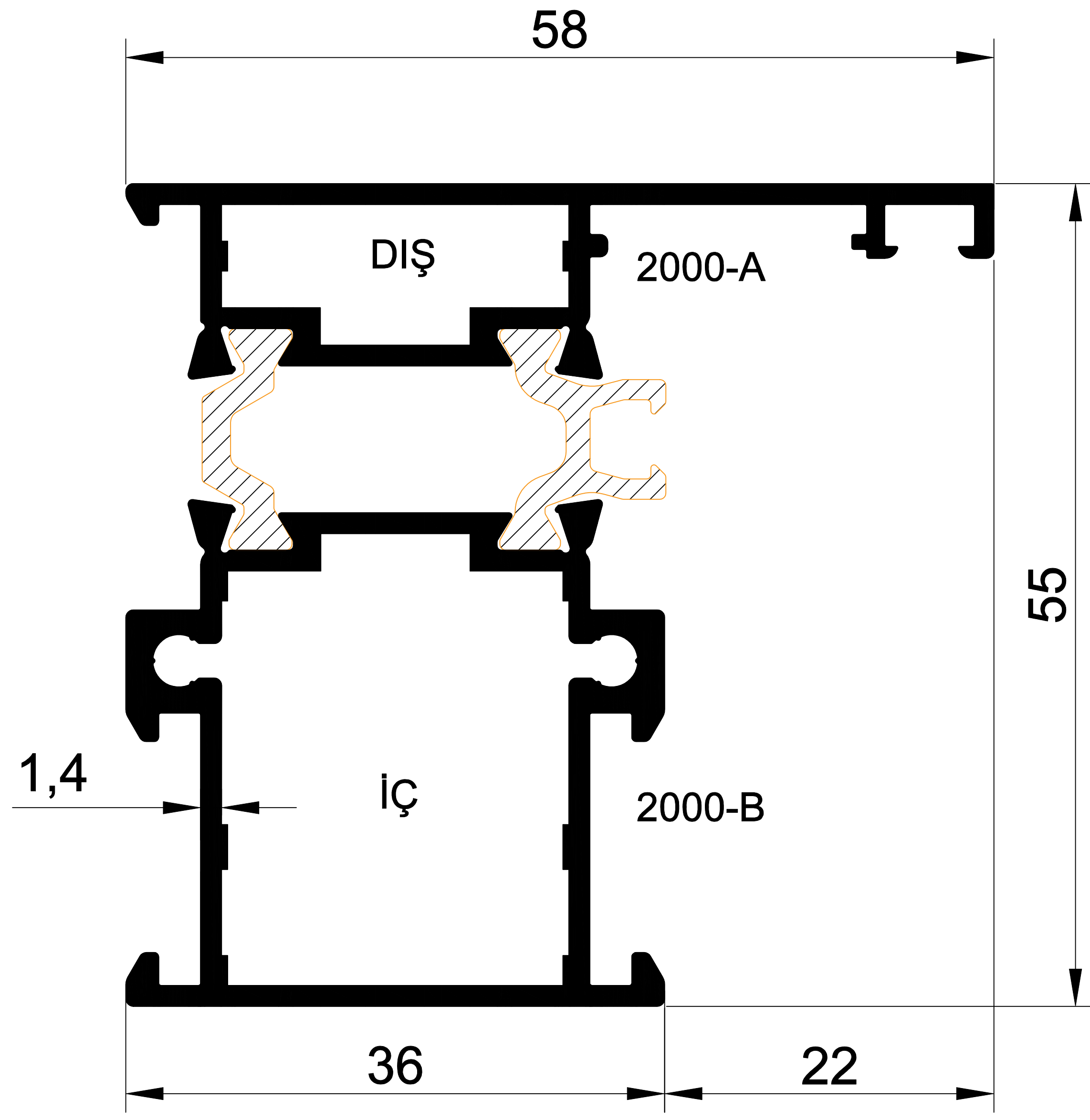
EKL-55- 2000 1,171 gr/m SİSTEM 55 ISI YALITIM KASA
