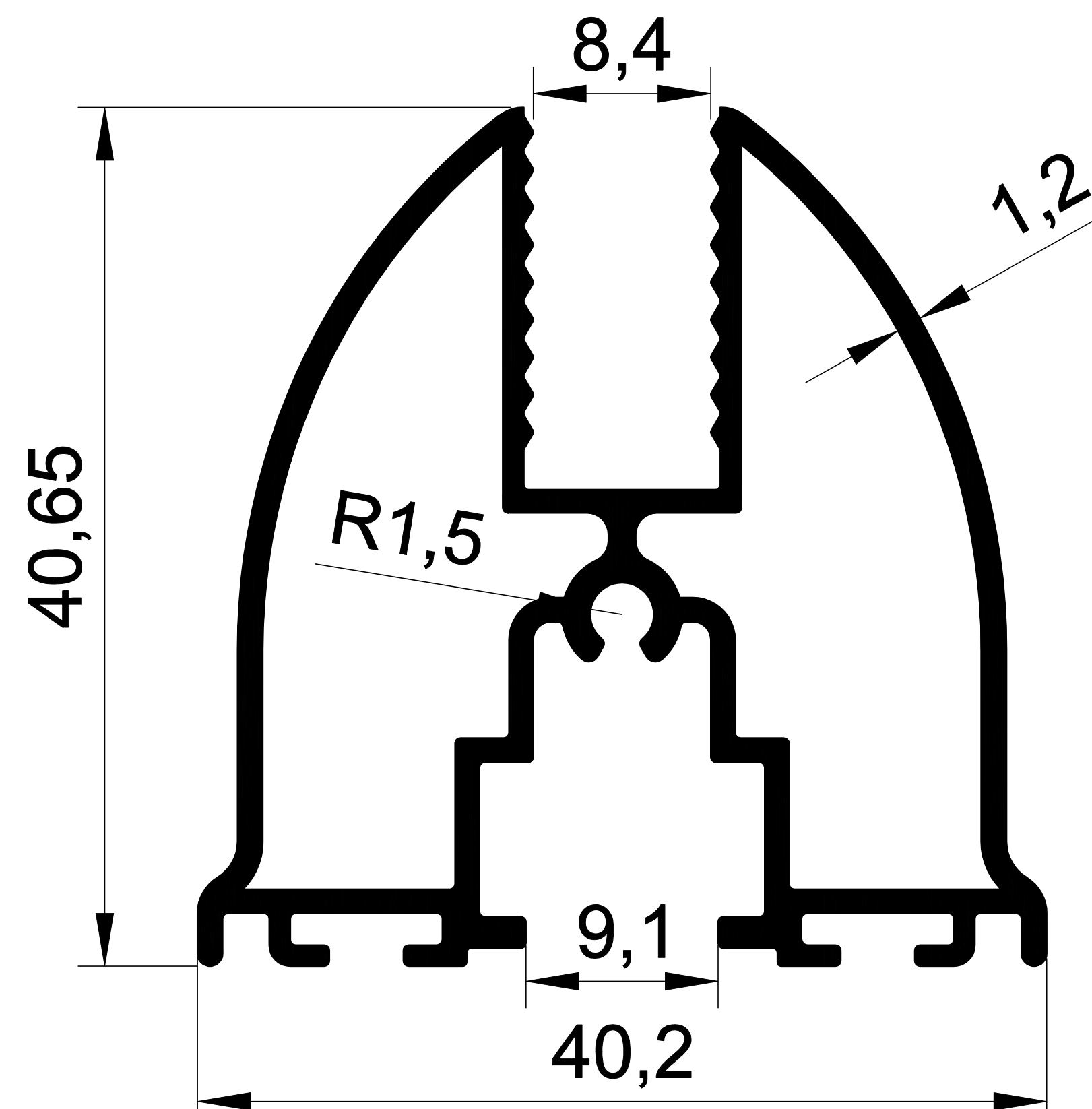
EKOL 1149 0,738 gr/m. GOLD KANAT
