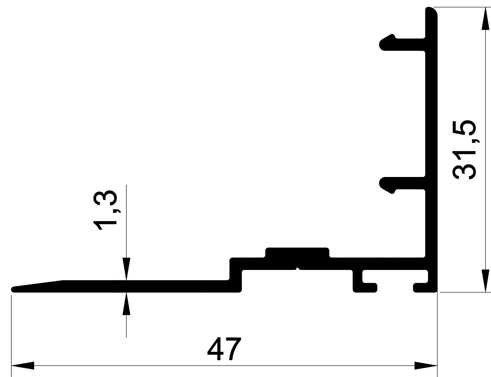
EKOL 1384 0,346 gr/m. 2000 SERİ SÜRME KENET
