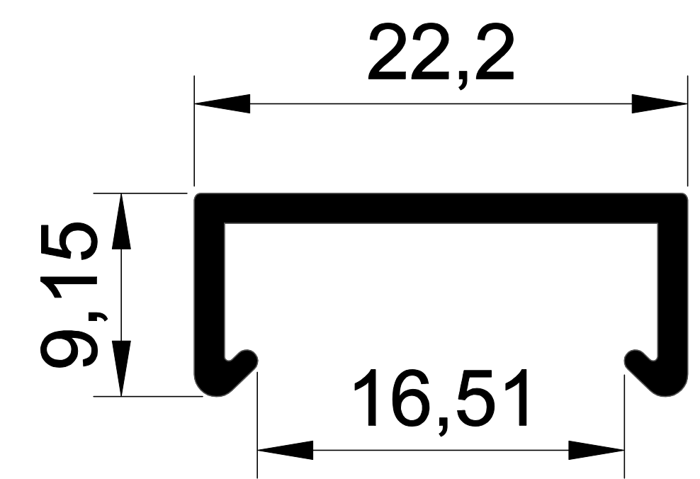
EKOL 1347 0,147 gr/m.
