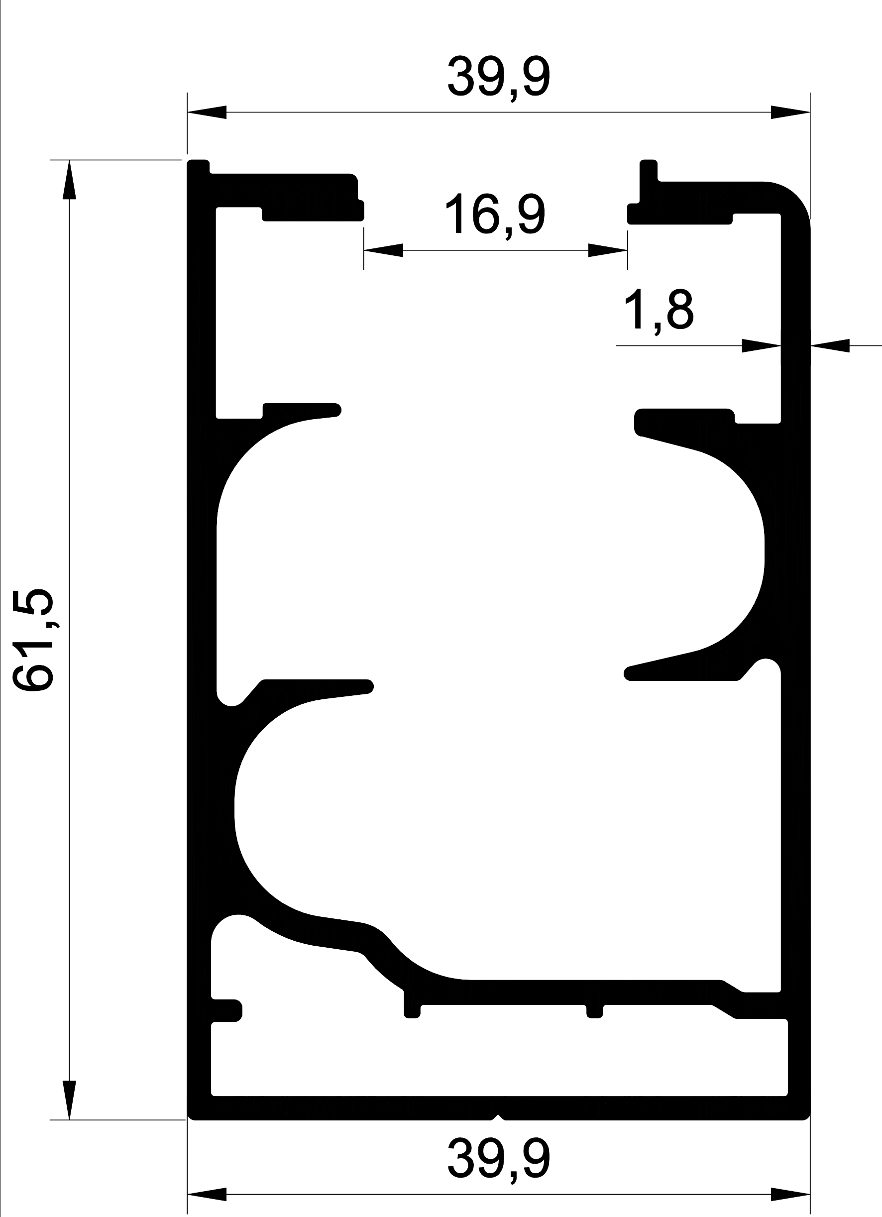
EKOL 1187 1,350 gr/m. BKS KASA
