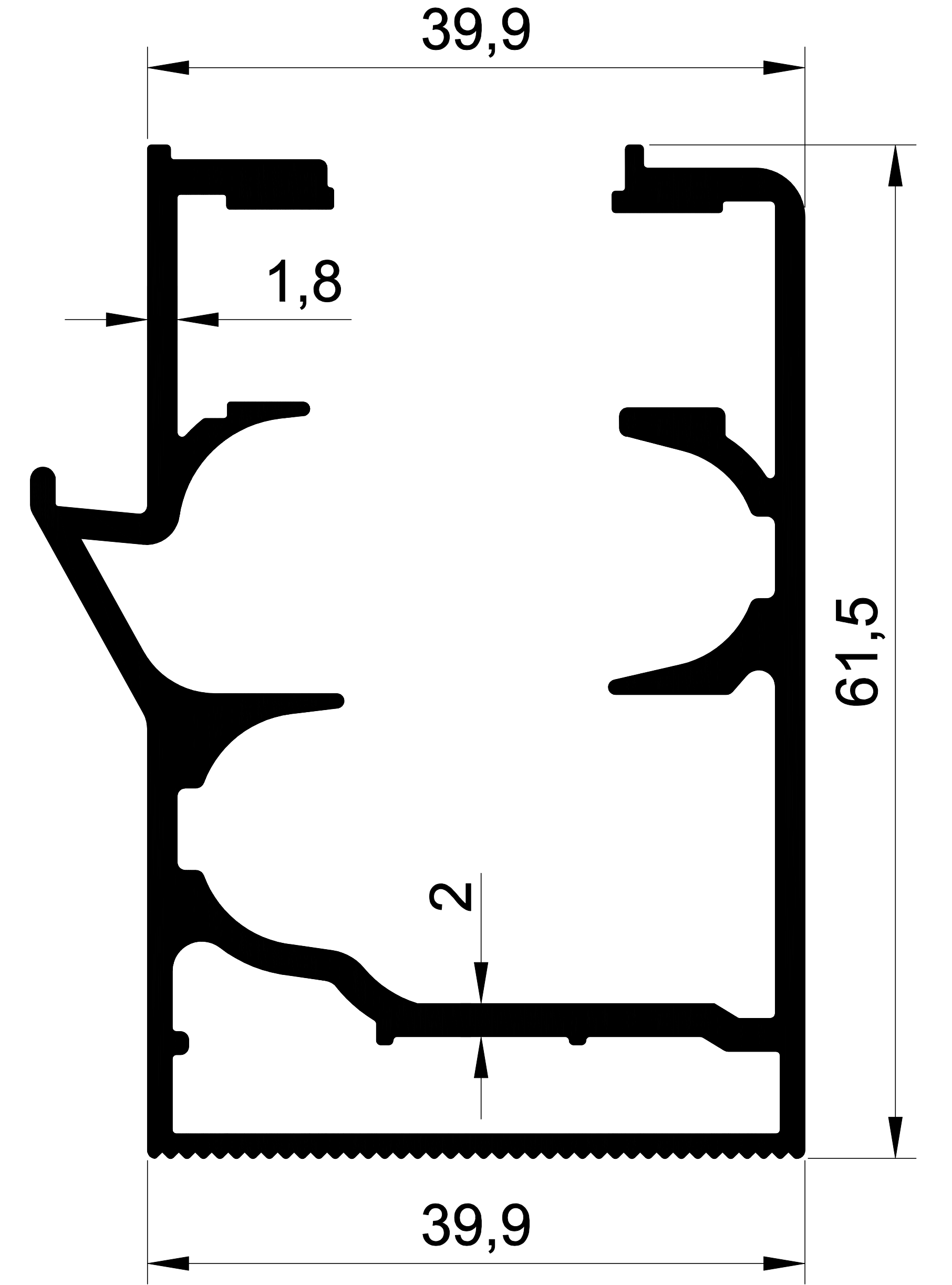
EKOL 1315 1,361 gr/m. ISI YALITIM ORTADAN DAMLALIKLI KASA
