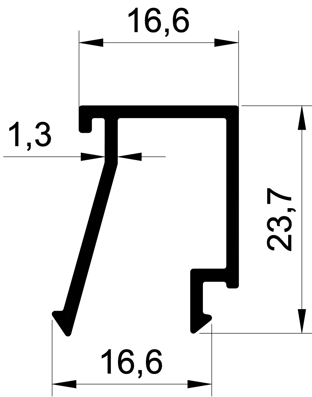
EKOL 1383 0,241 gr/m. 2000 SERİ SÜRME ÇITA
