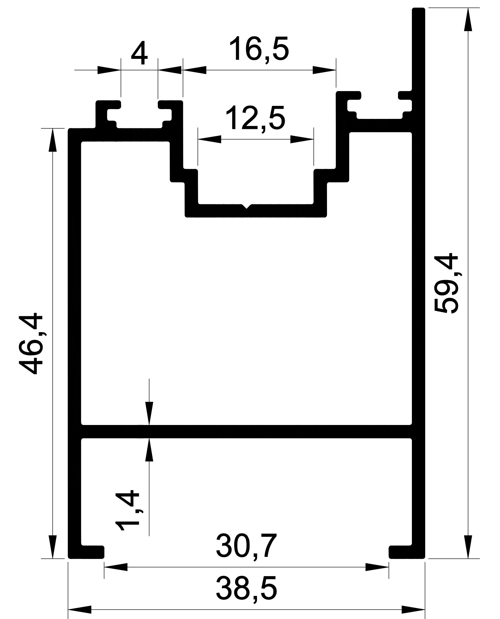
EKOL 1362 0,809 gr/m. ISI YALITIM KANAT KİLİTLEME
