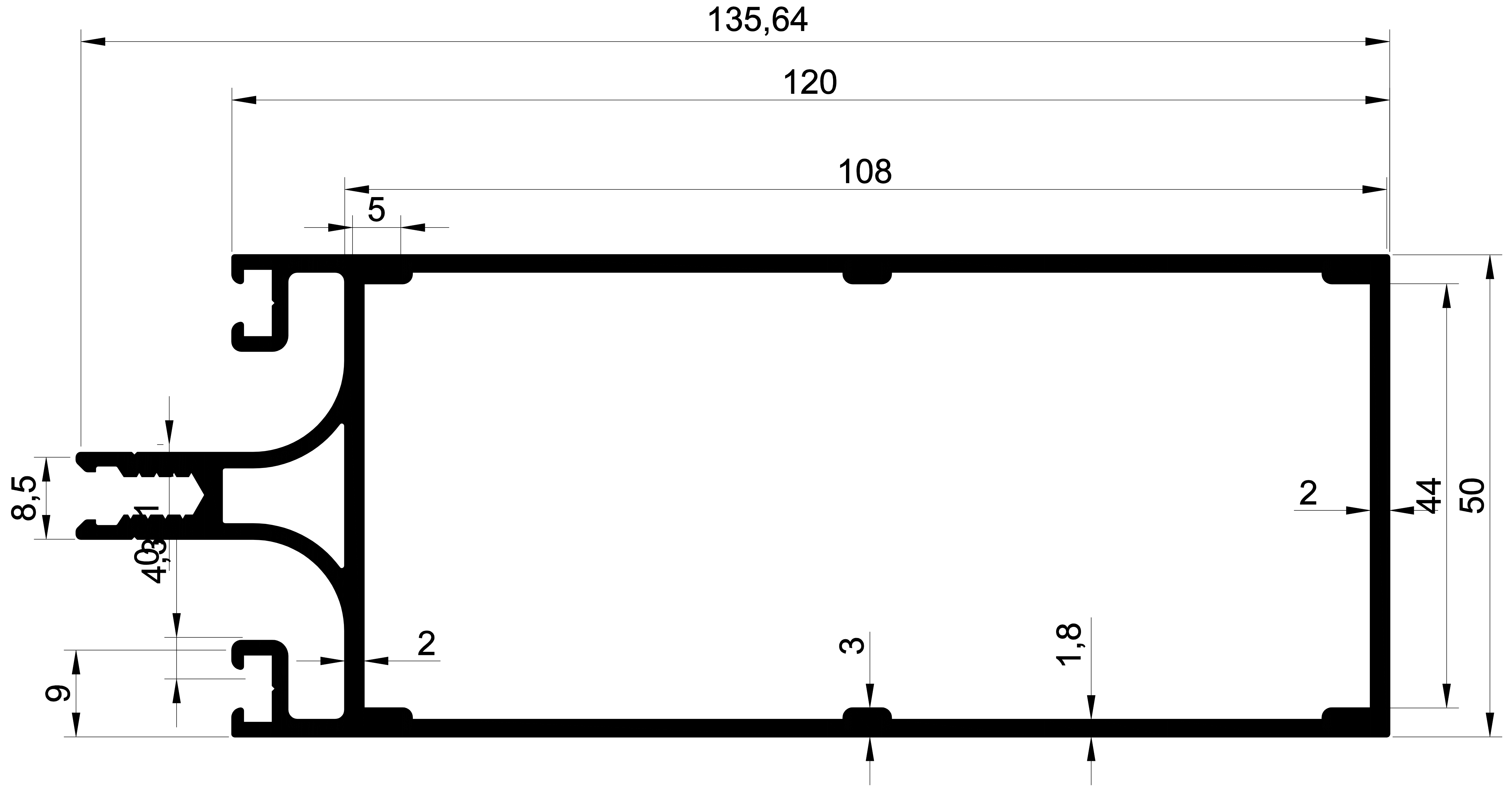
EKOL 1438 2,219 gr/m. 120'LİK CEPHE PROFİLİ UZUN GAGA
