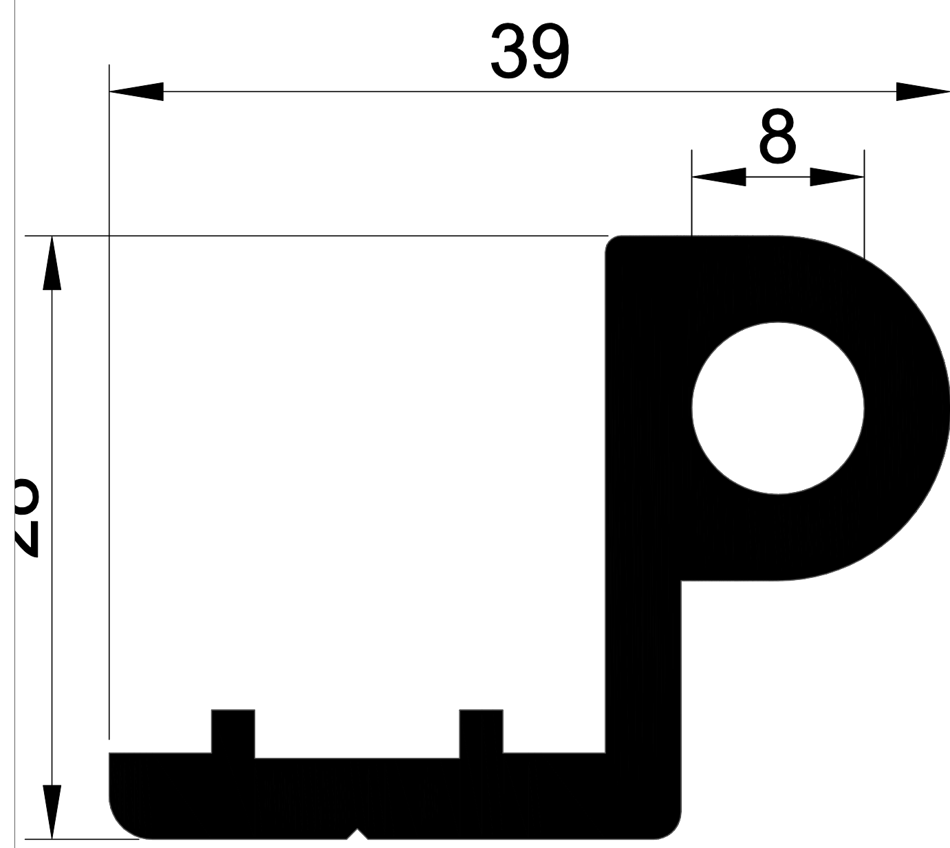
EKOL 1228 0,856 gr/m.
