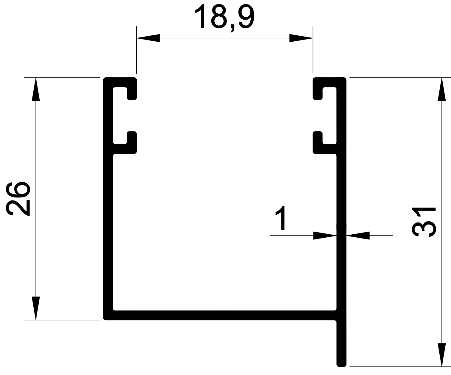
EKOL 1180 0,263 gr/m. PANJUR FİTİLLİ U
