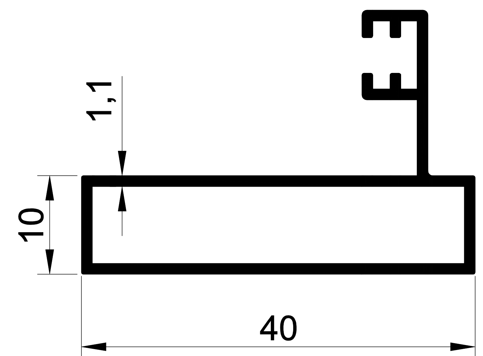
EKOL 1341 0,388 gr/m. 10 mm GOLD DİKME
