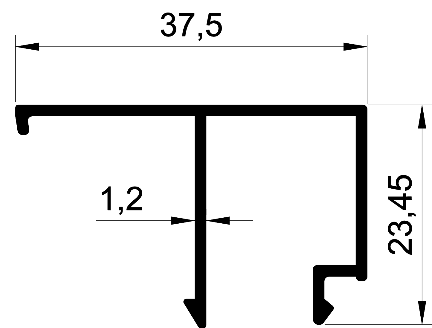
EKOL 1203 0,298 gr/m. SİSTEM TEK CAM ÇİTASI
