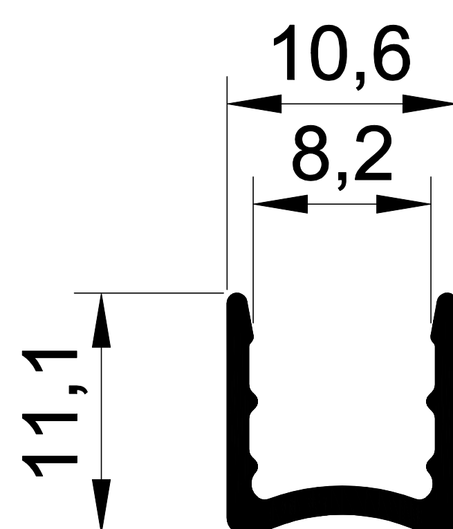
EKOL 1251 0,095 gr/m. CAM H
