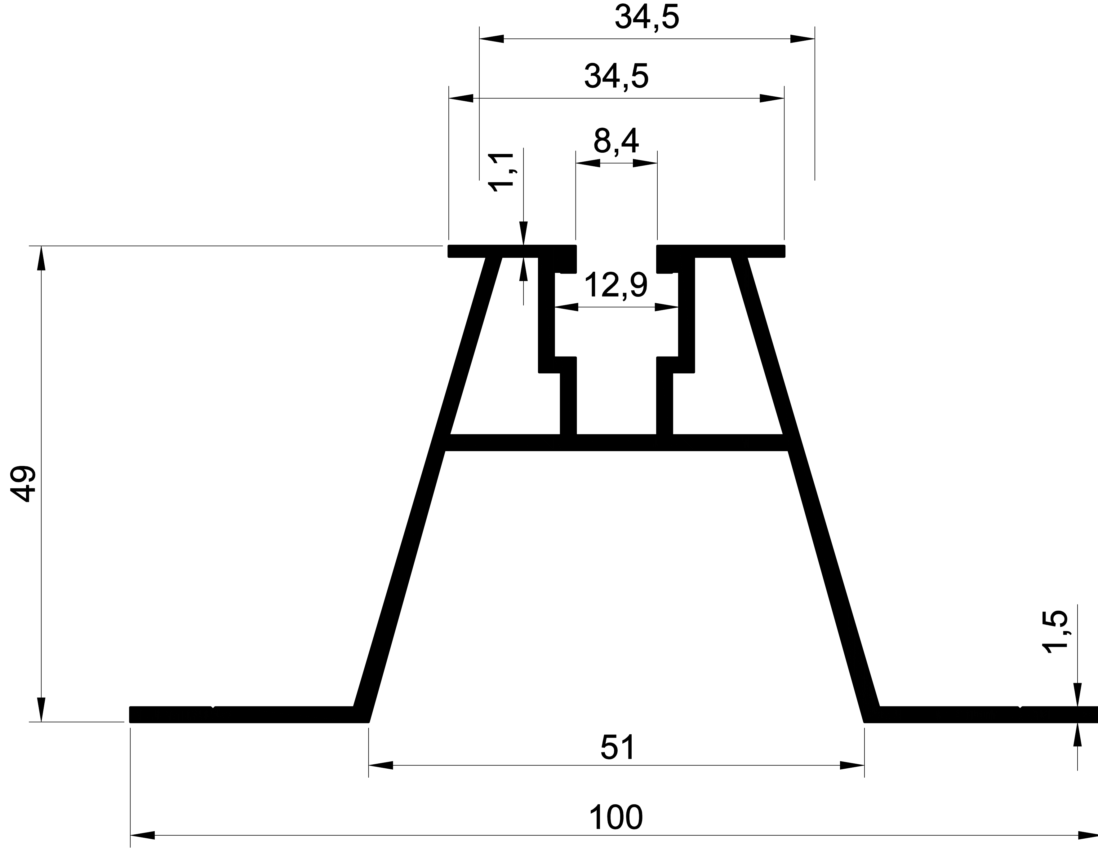
EKOL 1429 1,009 gr/m GES ALT KONTRÜKSİYON
