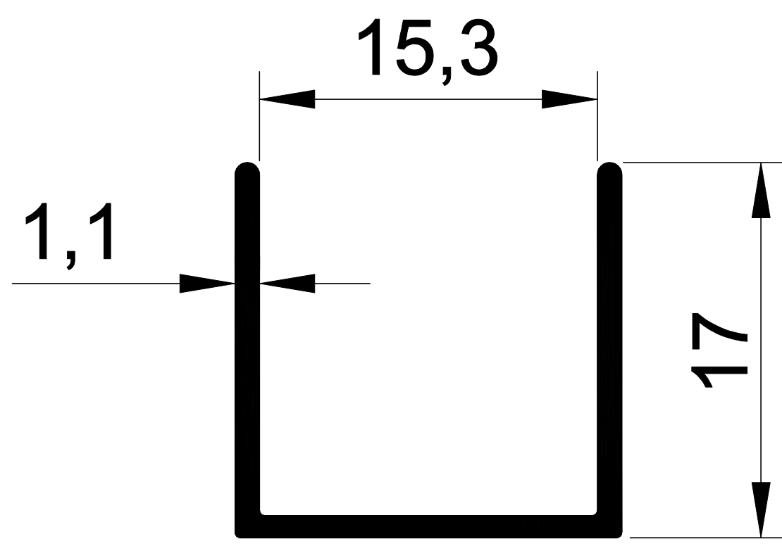
EKOL 1179 0,141 gr/m. PANJUR DAR U
