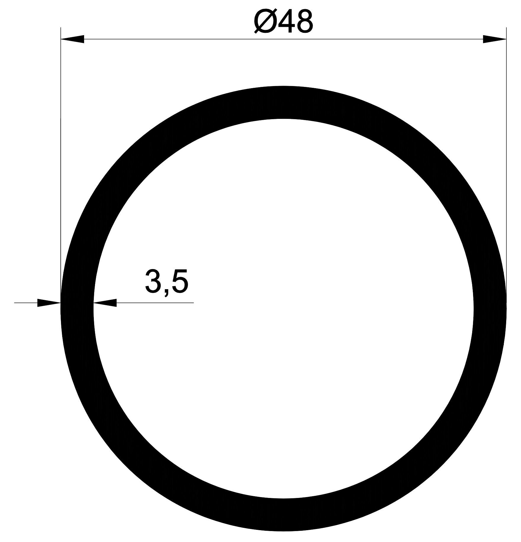
EKOL 1215 1,325 gr/m.
