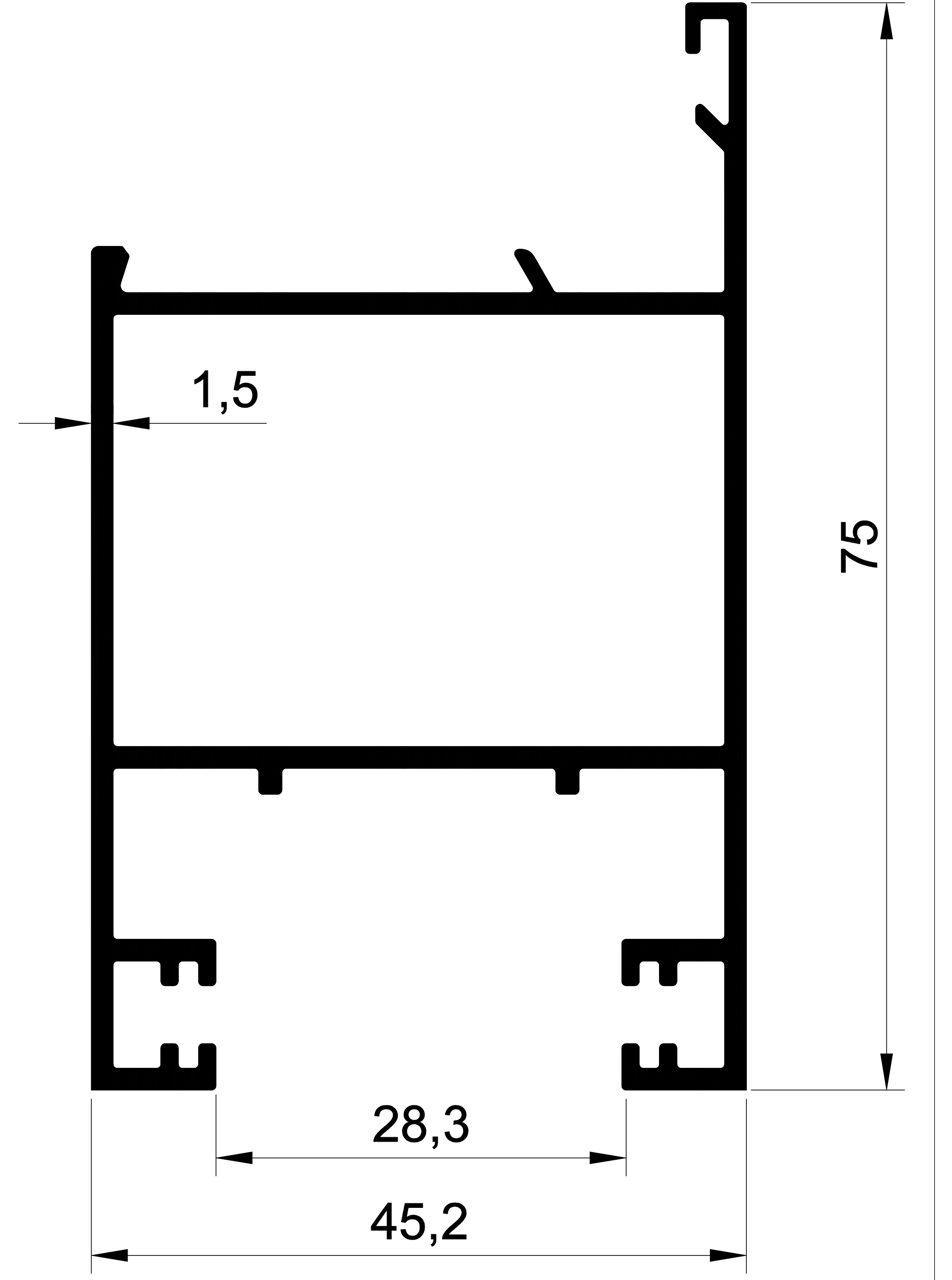
EKOL 1386 1,114 gr/m. 100'LÜK TUBA KANAT
