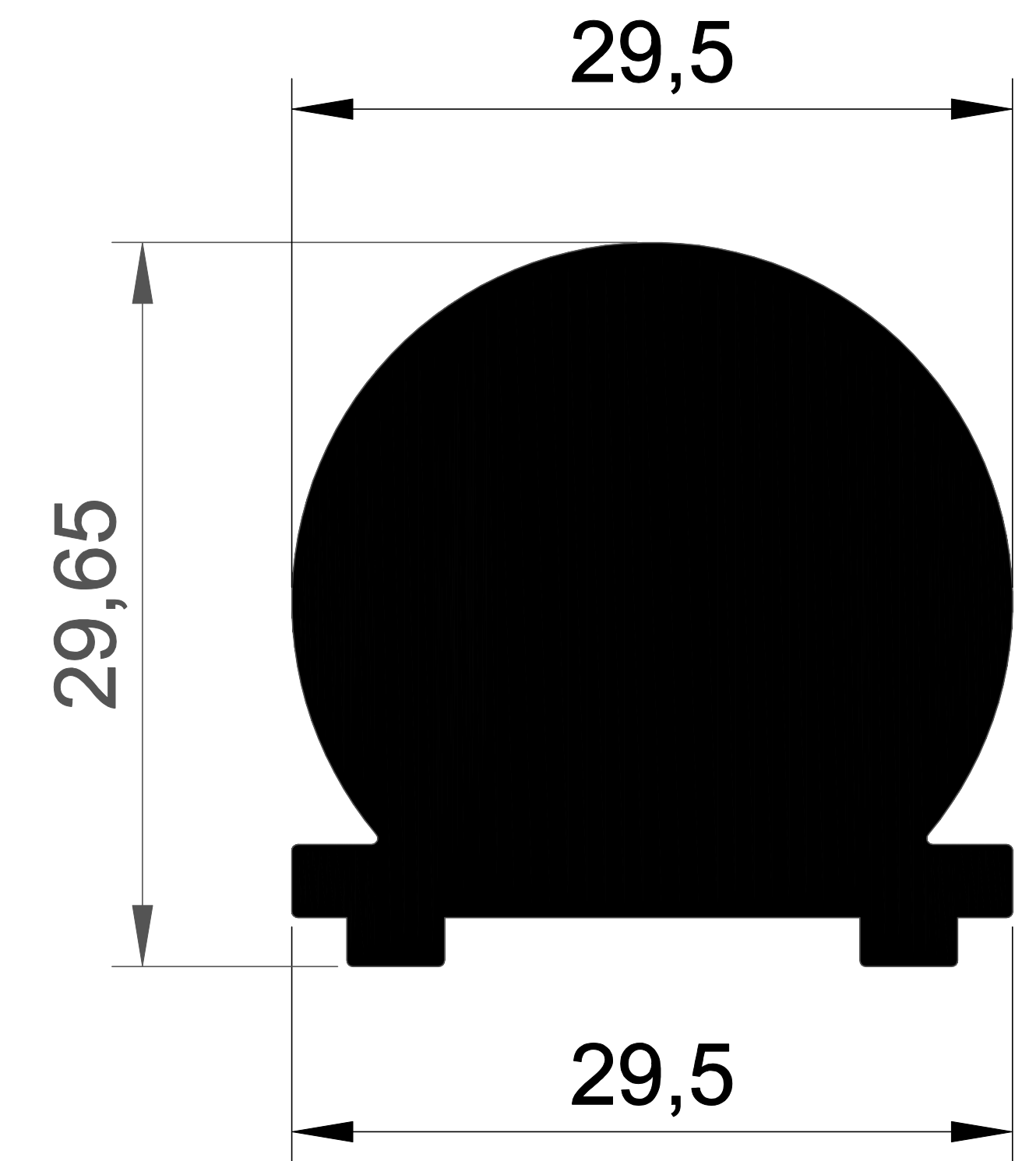
EKOL 1298 1,938 gr/m.
