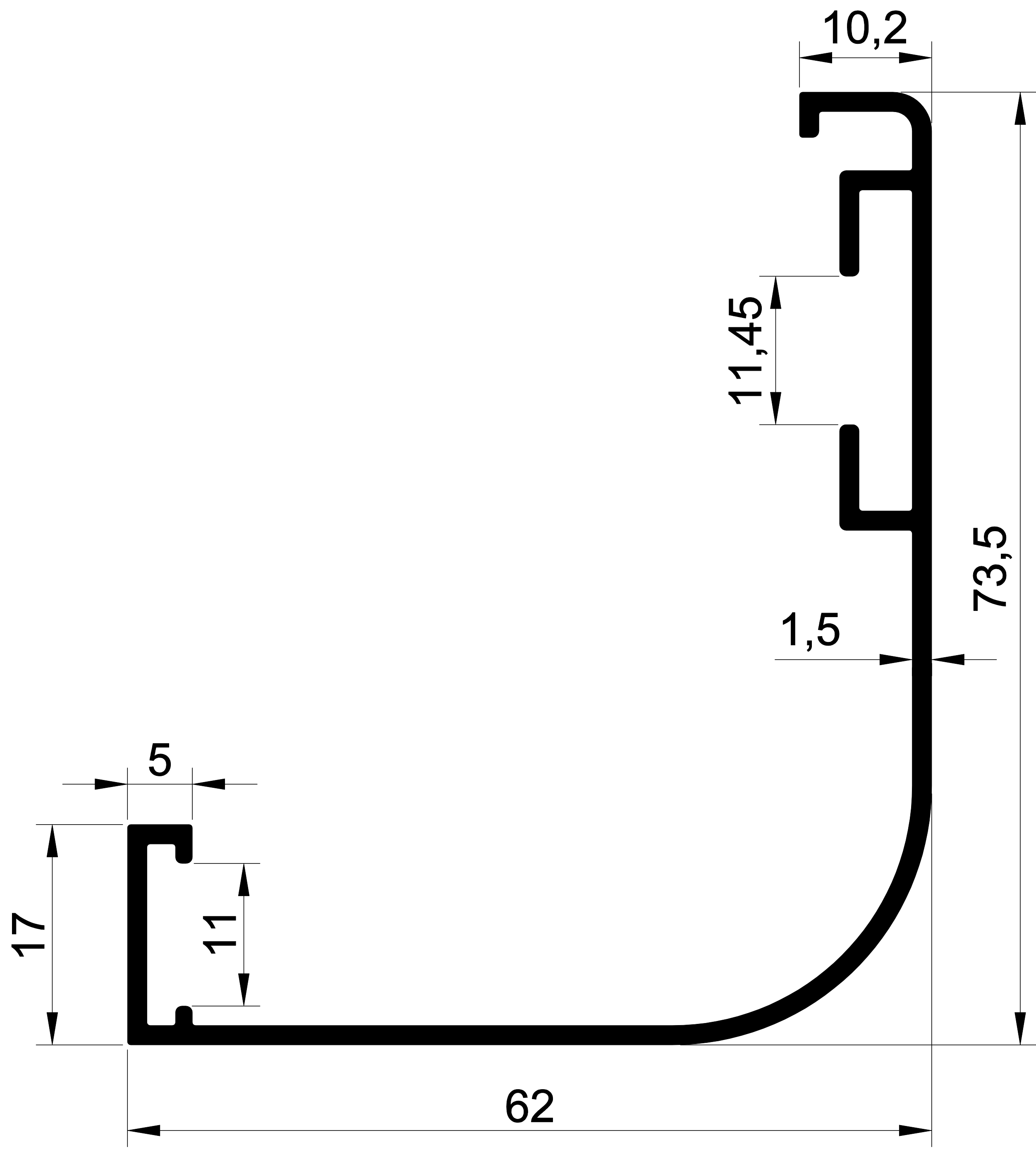
EKOL 1422 0,737 gr/m. MS-62'LİK PEERVAZ
