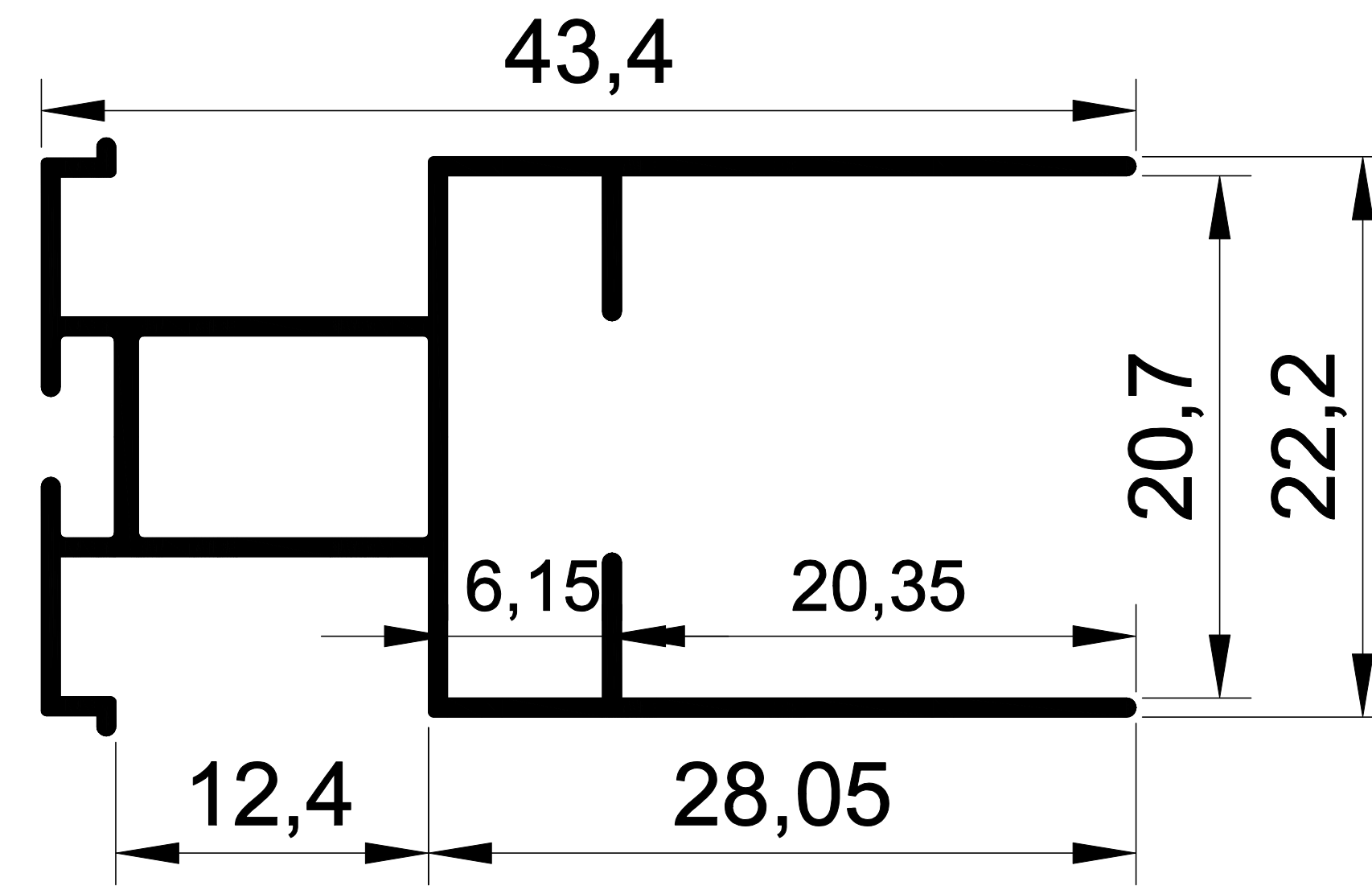
EKOL 1336 0,308 gr/m. MAVİ AY SİNEKLİK KANAT
