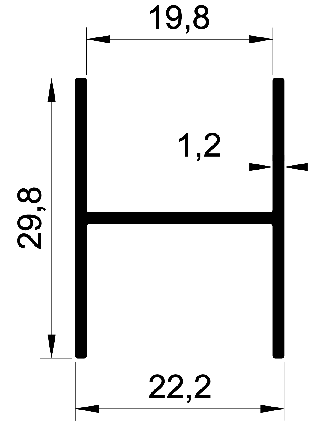
EKOL 1411 0,257 gr/m. MOBİLYA H PROFİLİ
