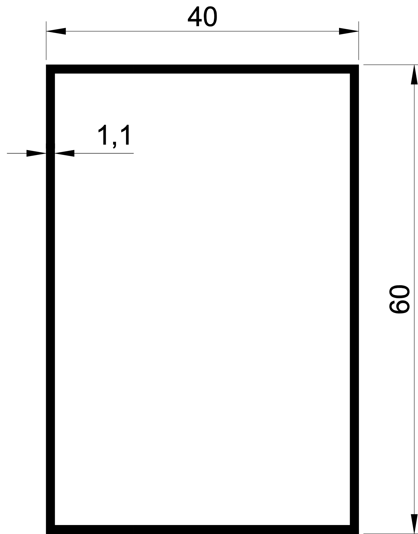
EKOL1312 0,583 gr/m.
