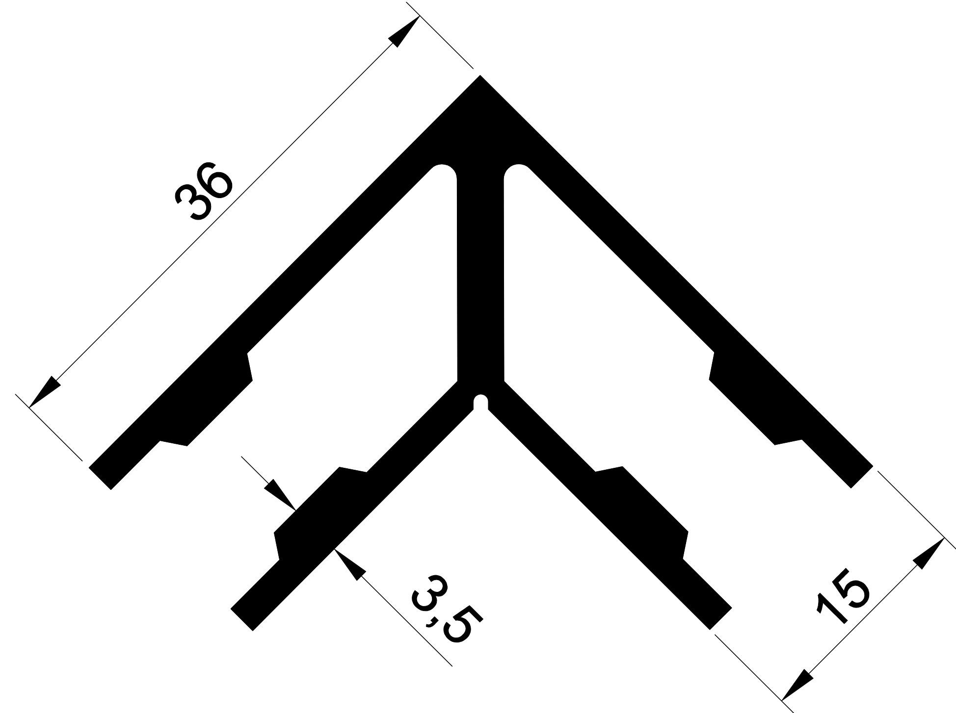
EKOL 1096 0,863 gr/m. DAR ÇAVUŞ (KÖŞE BAĞLANTI)
