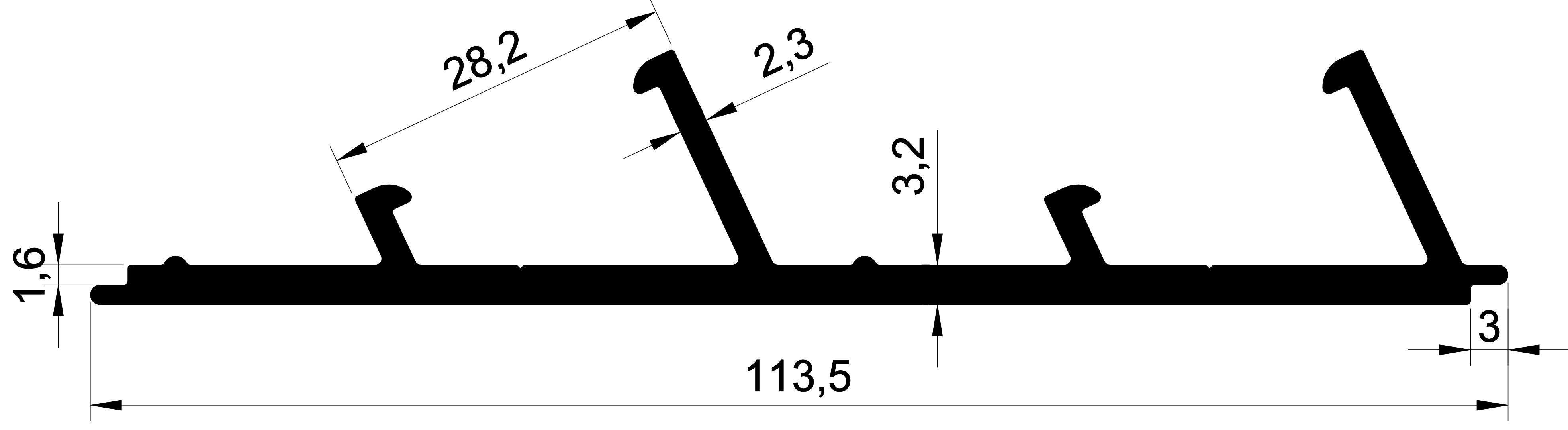
EKOL 1432 1,311 gr/m. MENFEZ KASA
