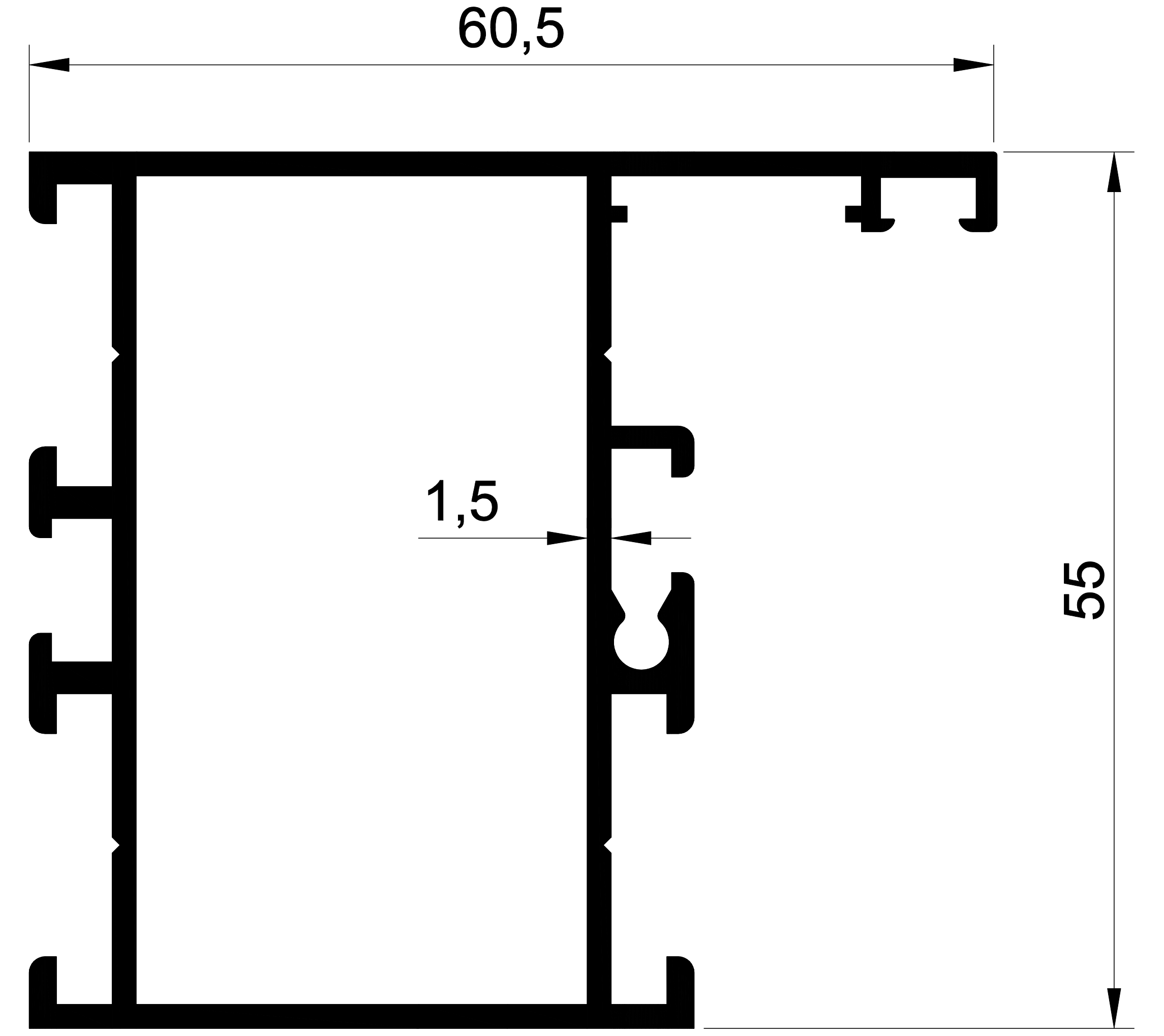
EKOL 1200 1,098 gr/m. SİSTEM KASA
