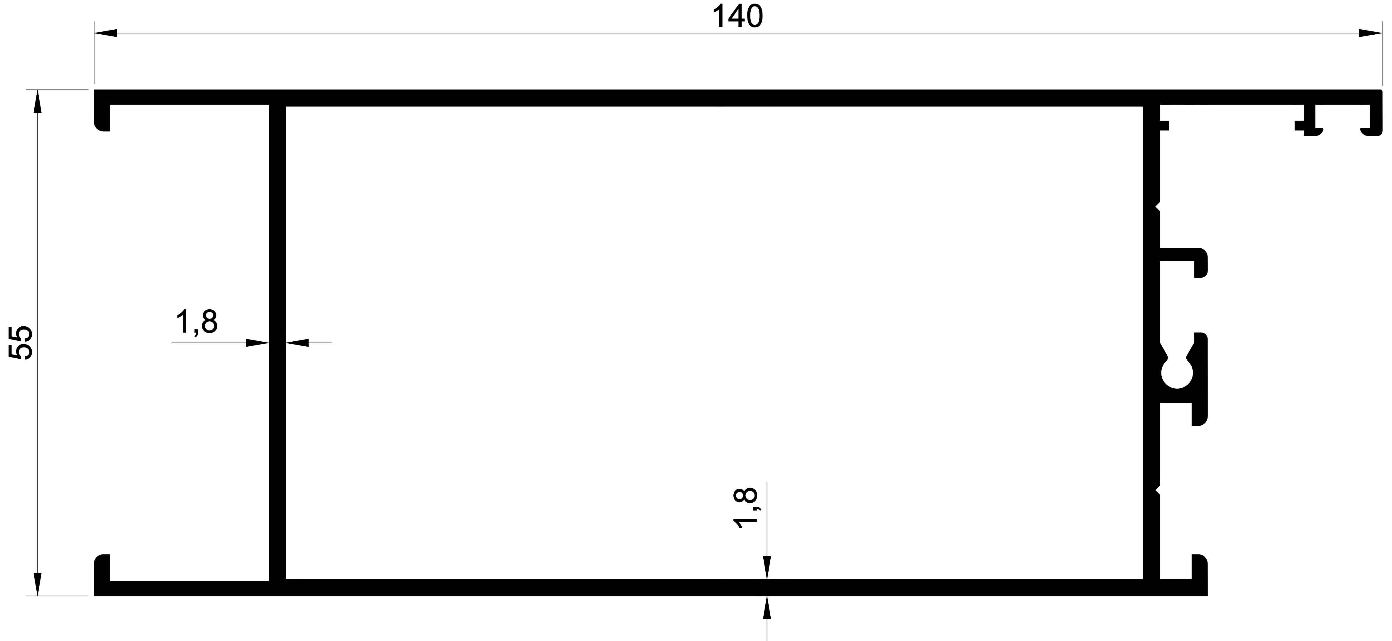
EKOL 1205 1,902 gr/m. SİSTEM ETEK
