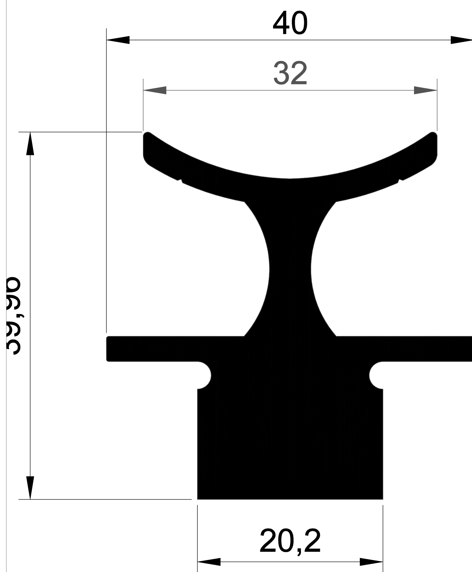
EKOL 1172 1,615 gr/m.
