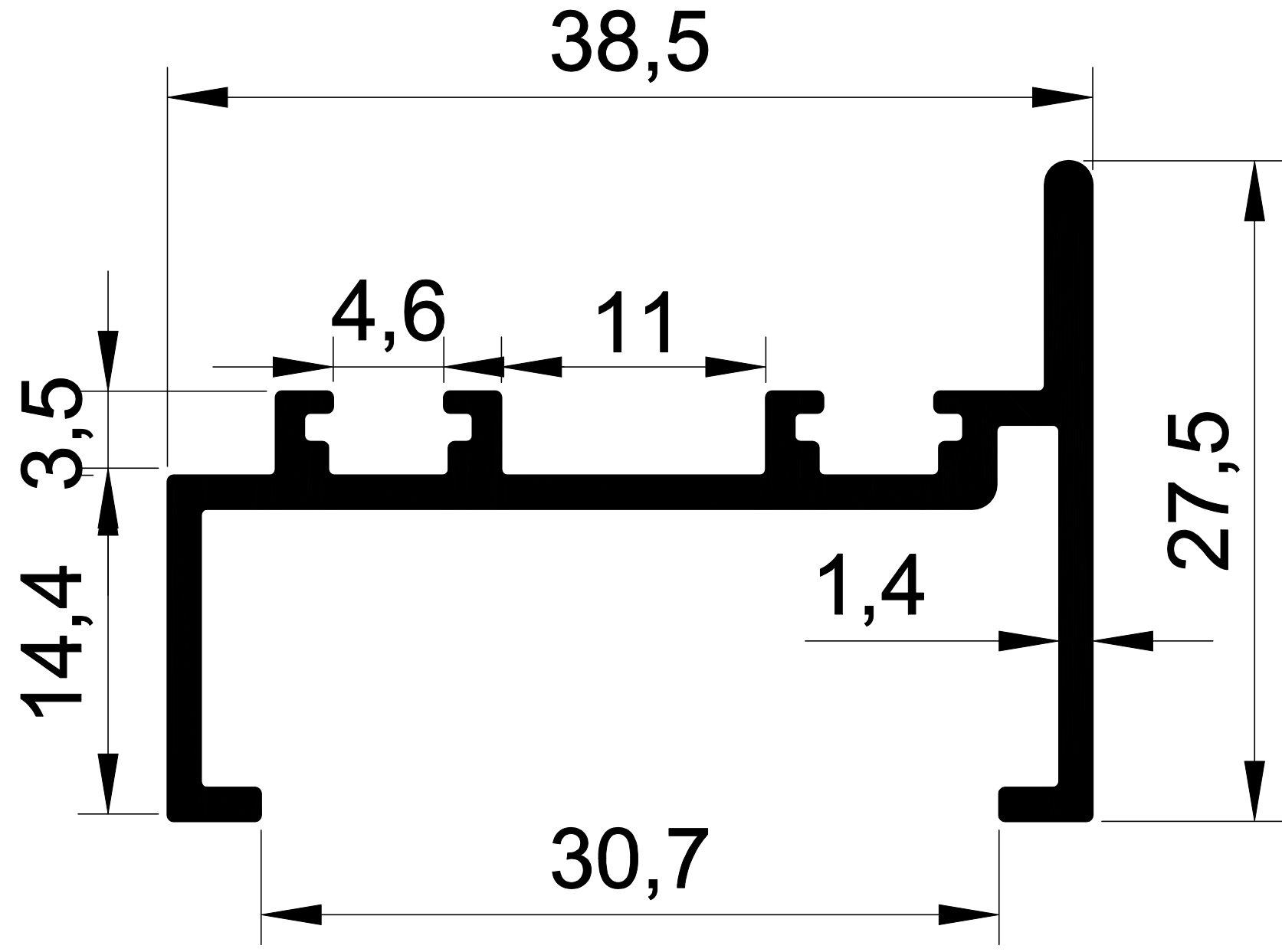
EKOL 1361 0,402 gr/m. ISI YALITIM KANAT
