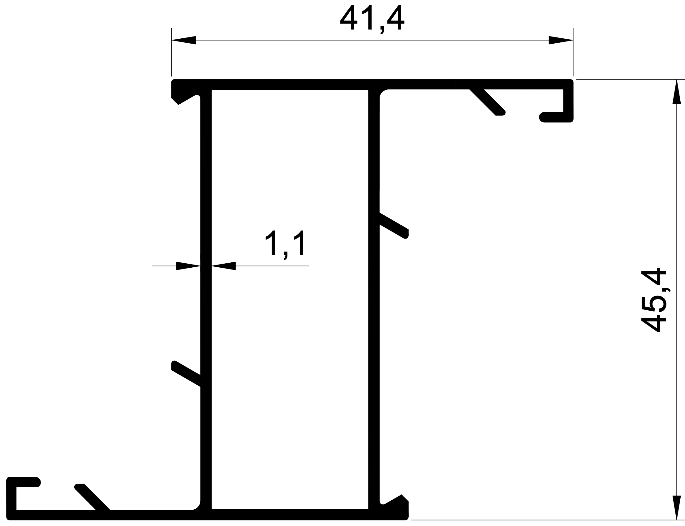
EKOL 1101 0,547 gr/m. ALDOKS DAR KANAT
