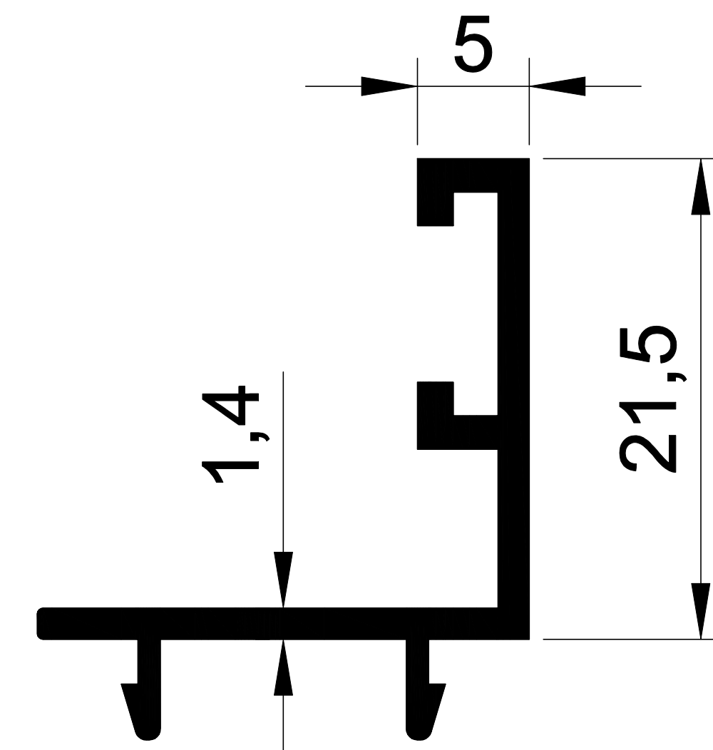
EKOL 1352 0,231 gr/m. C-60 TIRNAK
