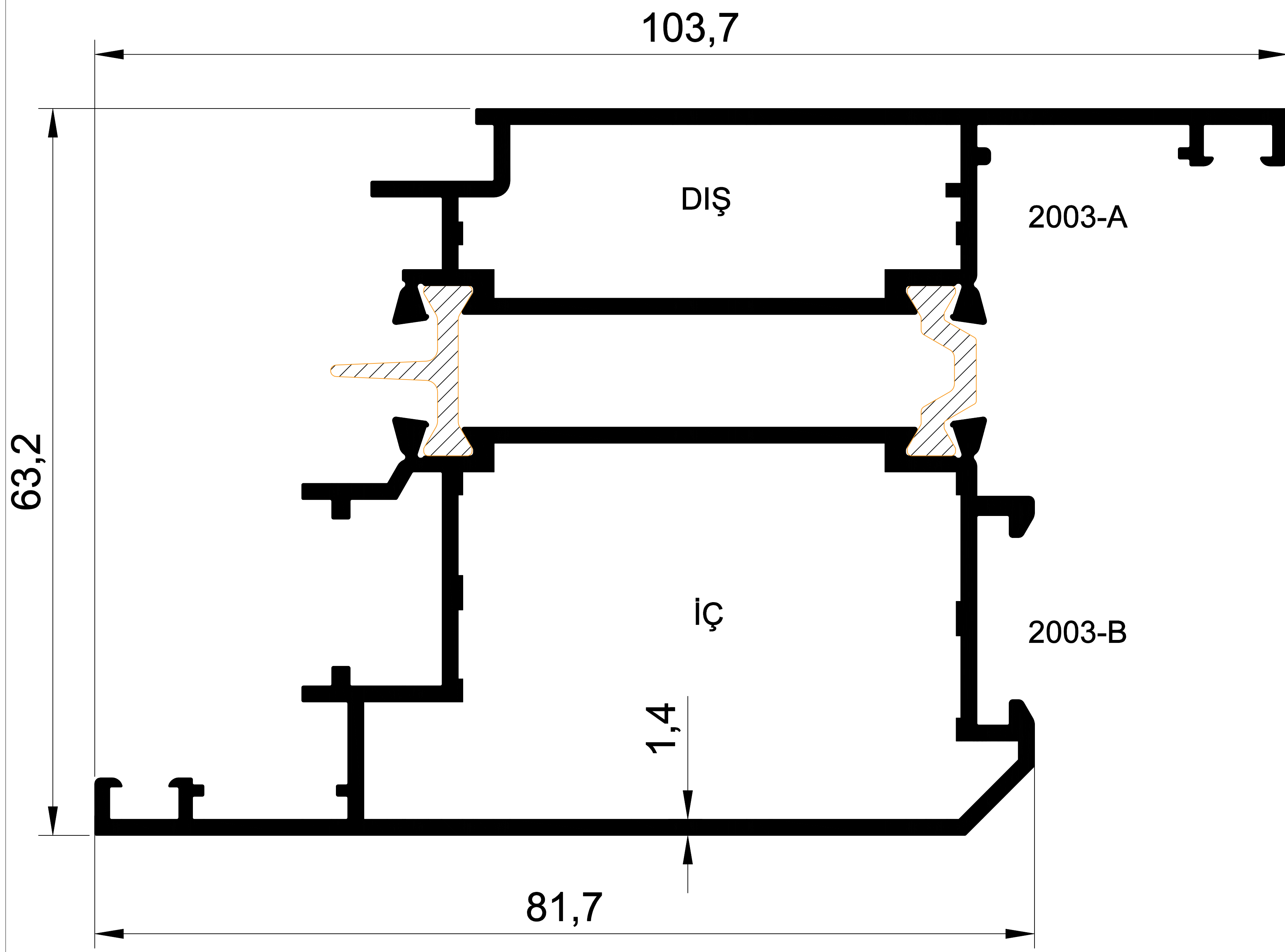
EKL-55- 2003 1,697 gr/m SİSTEM 55 ISI YALITIM İÇE AÇILIR KAPI
