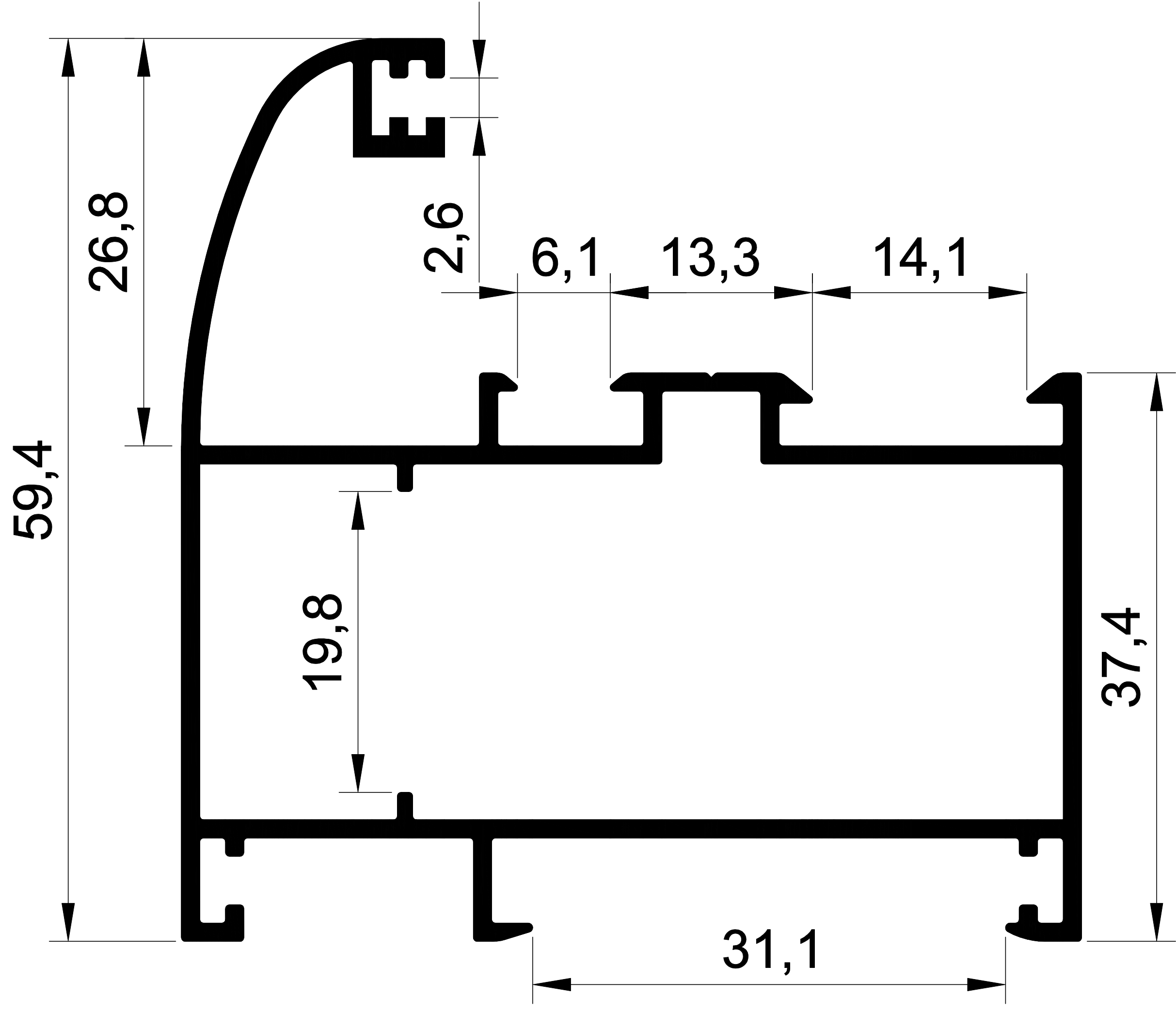
EKOL 1369 0,917 gr/m. OVAL KASA
