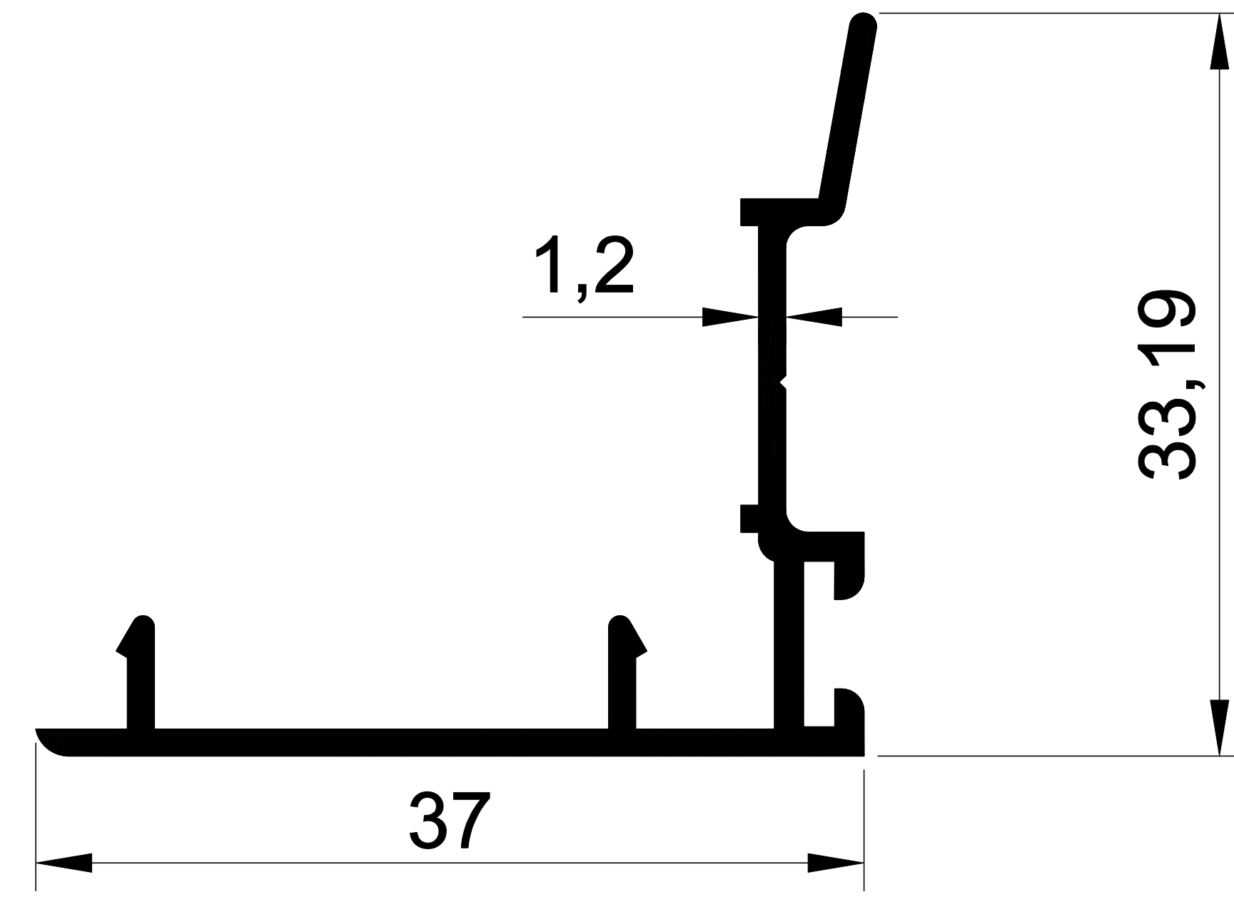
EKOL 1195 0,295 gr/m DAR TUBA KAPAK
