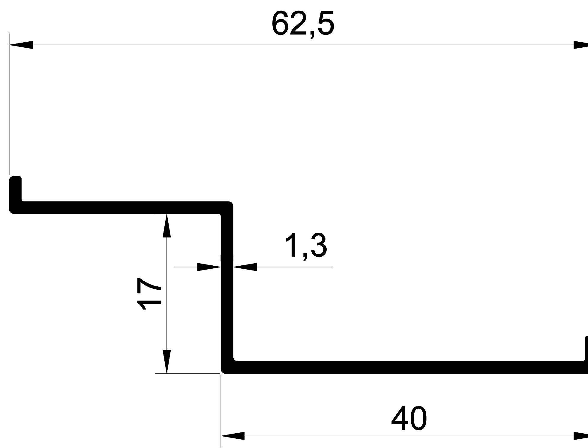
EKOL 1427 0,298 gr/m. MS-AHŞAP GİZLİ KAPI KANAT ÇERÇEVESİ
