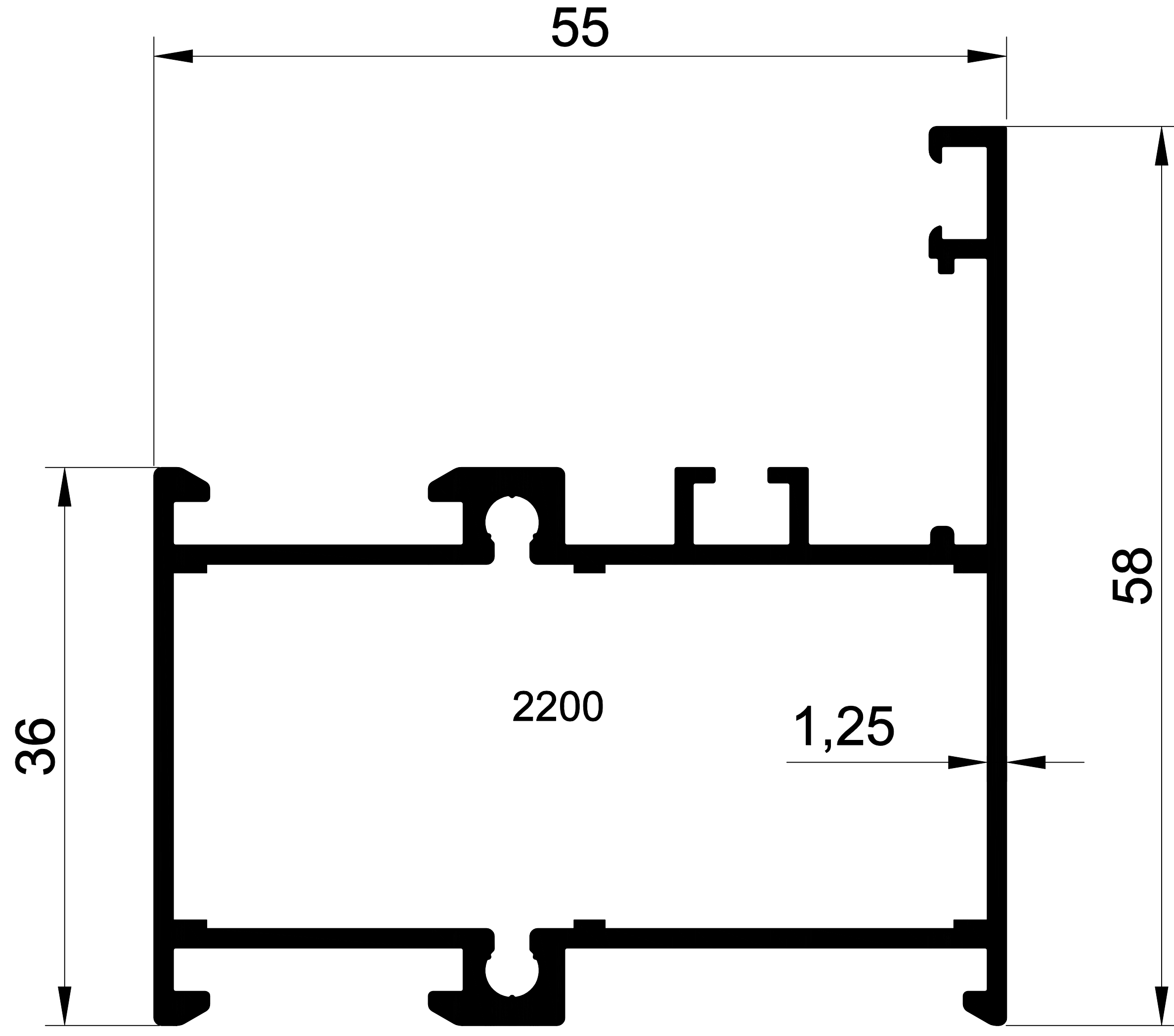
EK-55- 2200 0,929 gr/m SİSTEM 55 YALITIMSIZ KASA
