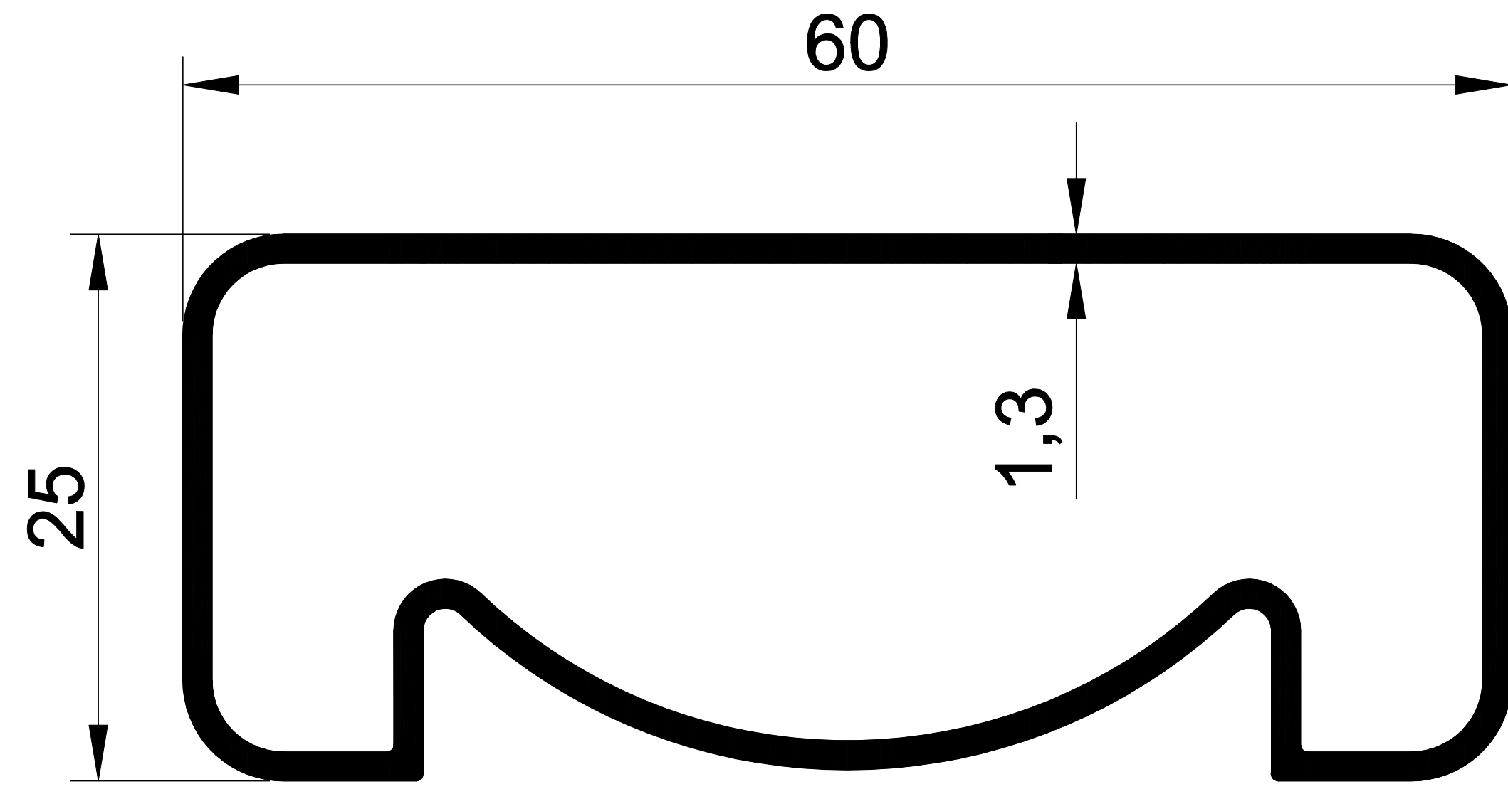
EKOL 1335 0,613 gr/m. 25X60 CAMSIZ
