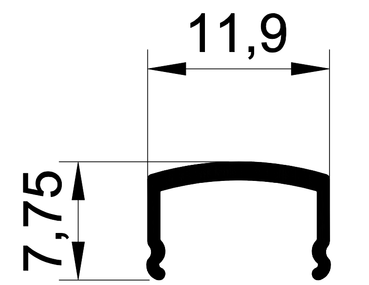
EKOL 1123 0,065 gr/m.
