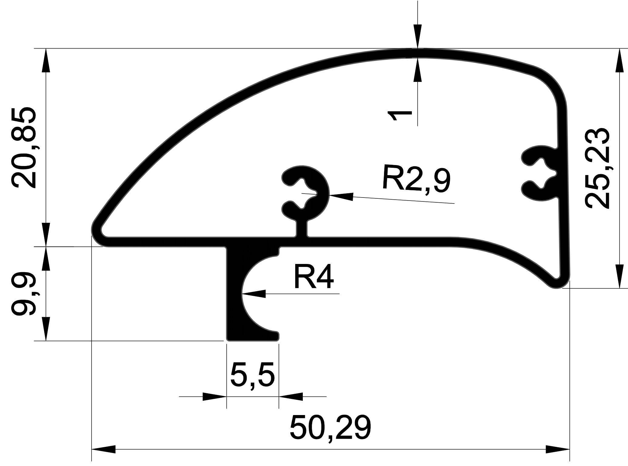
EKOL 1451 0.515 gr/m. RAY PROFİLİ
