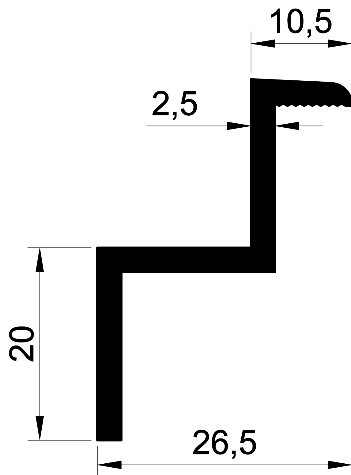
EKOL 1431 0,410 gr/m GES PANEL TUTUCU APARATI KÖŞE
