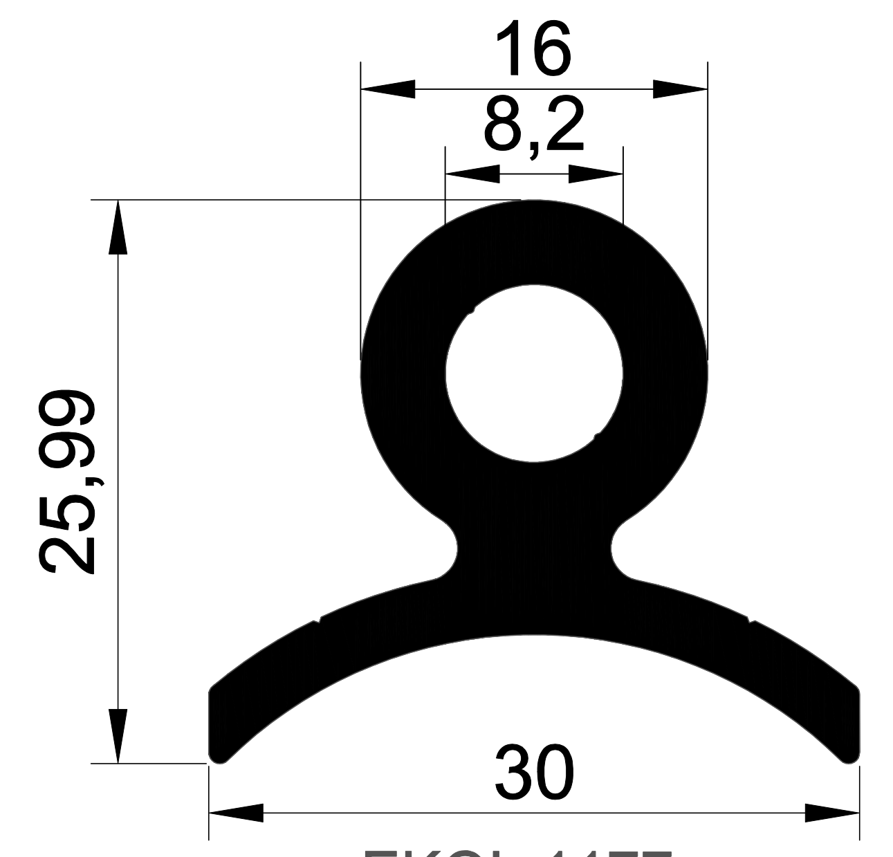
EKOL 1177 0,699 gr/m.
