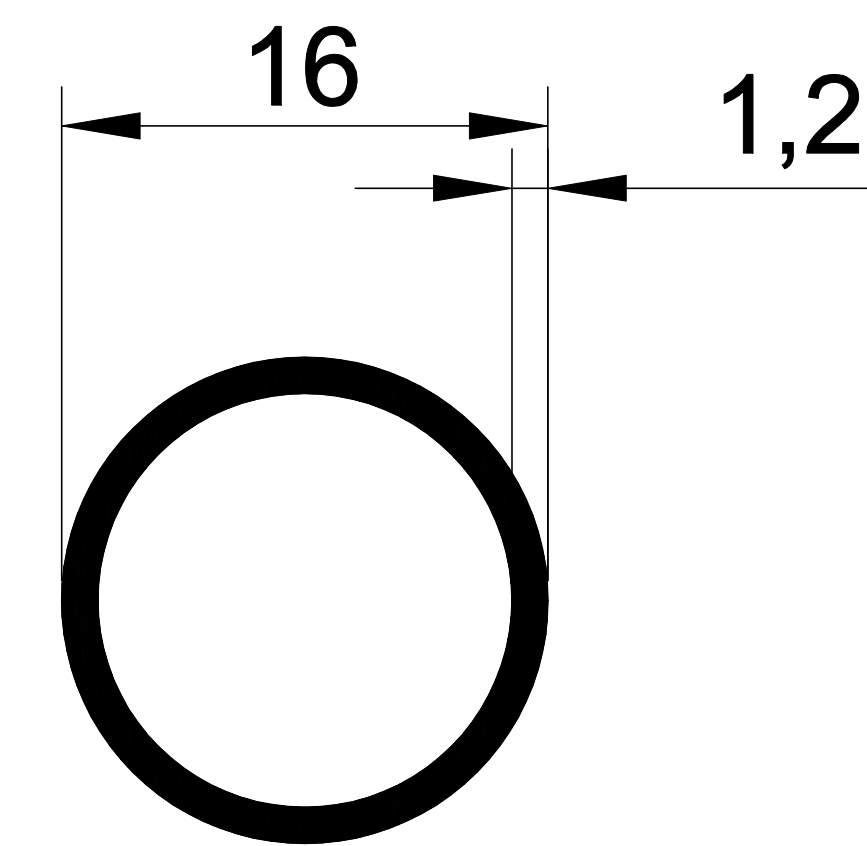
EKOL 1343 0,140 gr/m.
