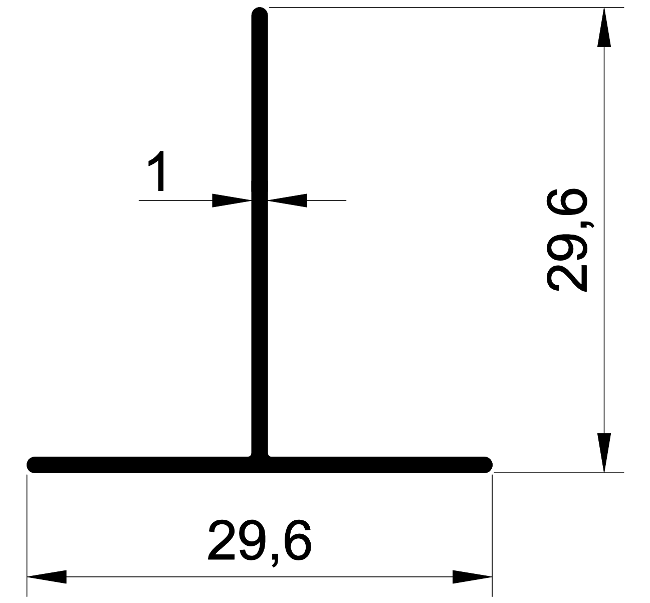
EKOL 1188 0,157 gr/m. 30X30 T BİNİ
