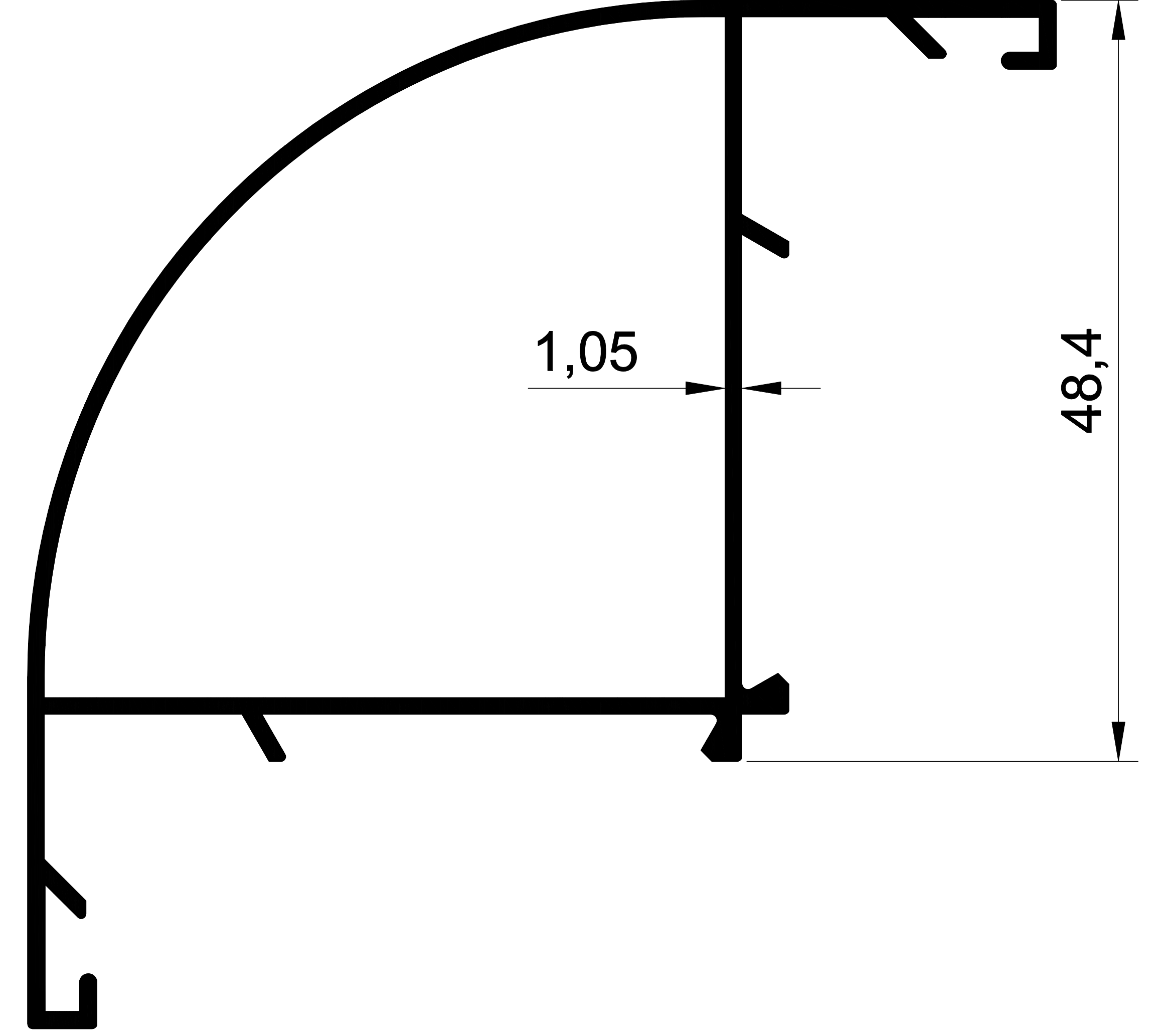
EKOL 1100 0,677 gr/m. ALDOKS OVAL KÖŞE DÖNÜŞ
