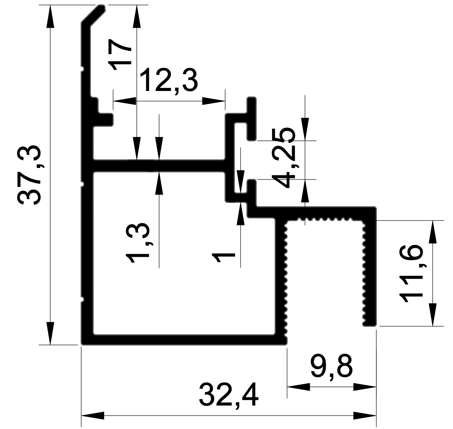
EKOL 1449 0.440 gr/m. C.B KOL PROFİLİ-2
