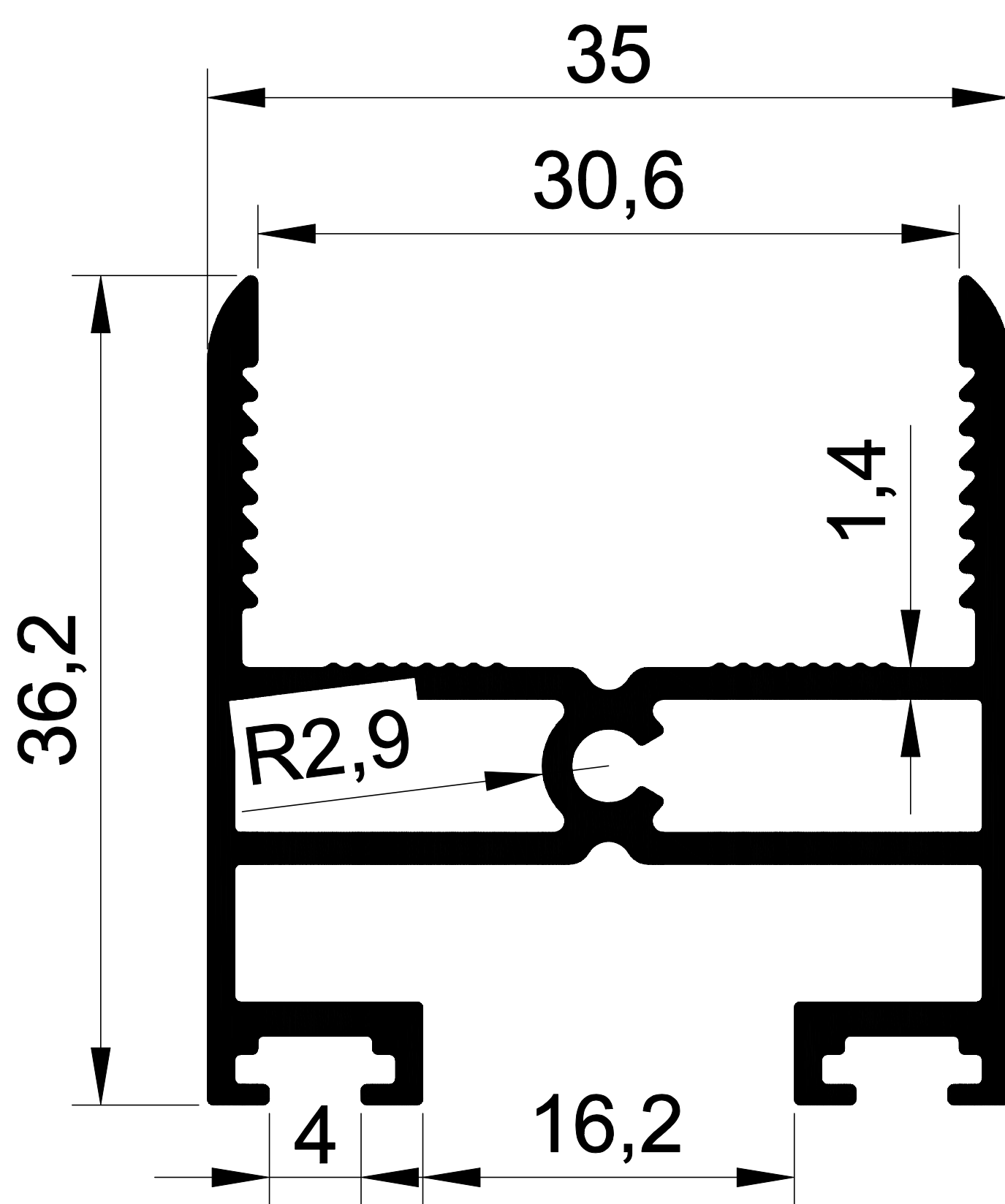
EKOL 1360 0,686 gr/m. ISI YALITIM BAZA
