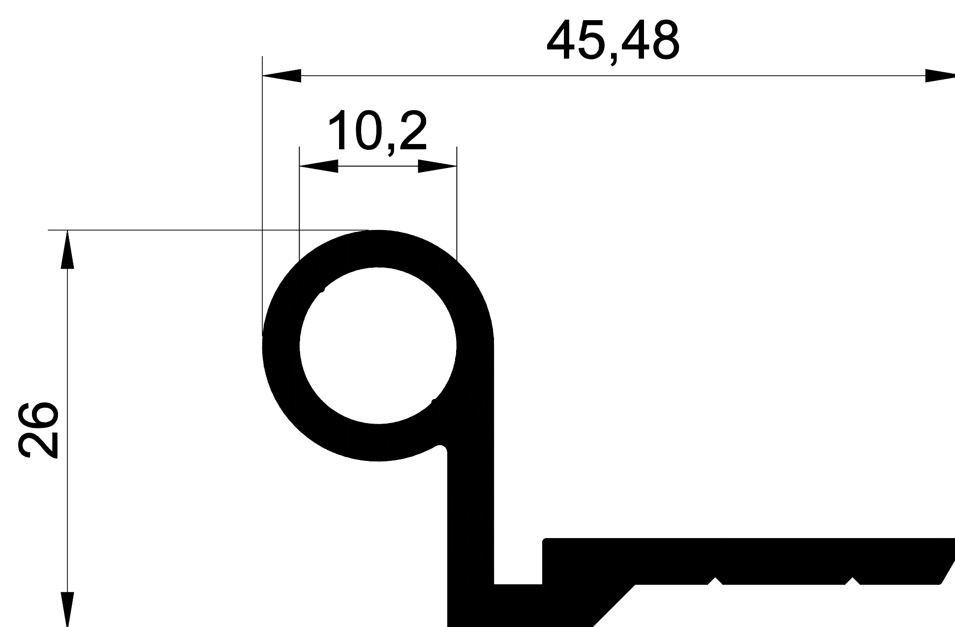
EKOL 1023 0,650 gr/m.
