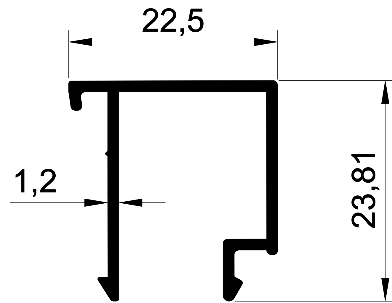
EKOL 1204 0,249 gr/m. SİSTEM ISI CAM ÇİTASI
