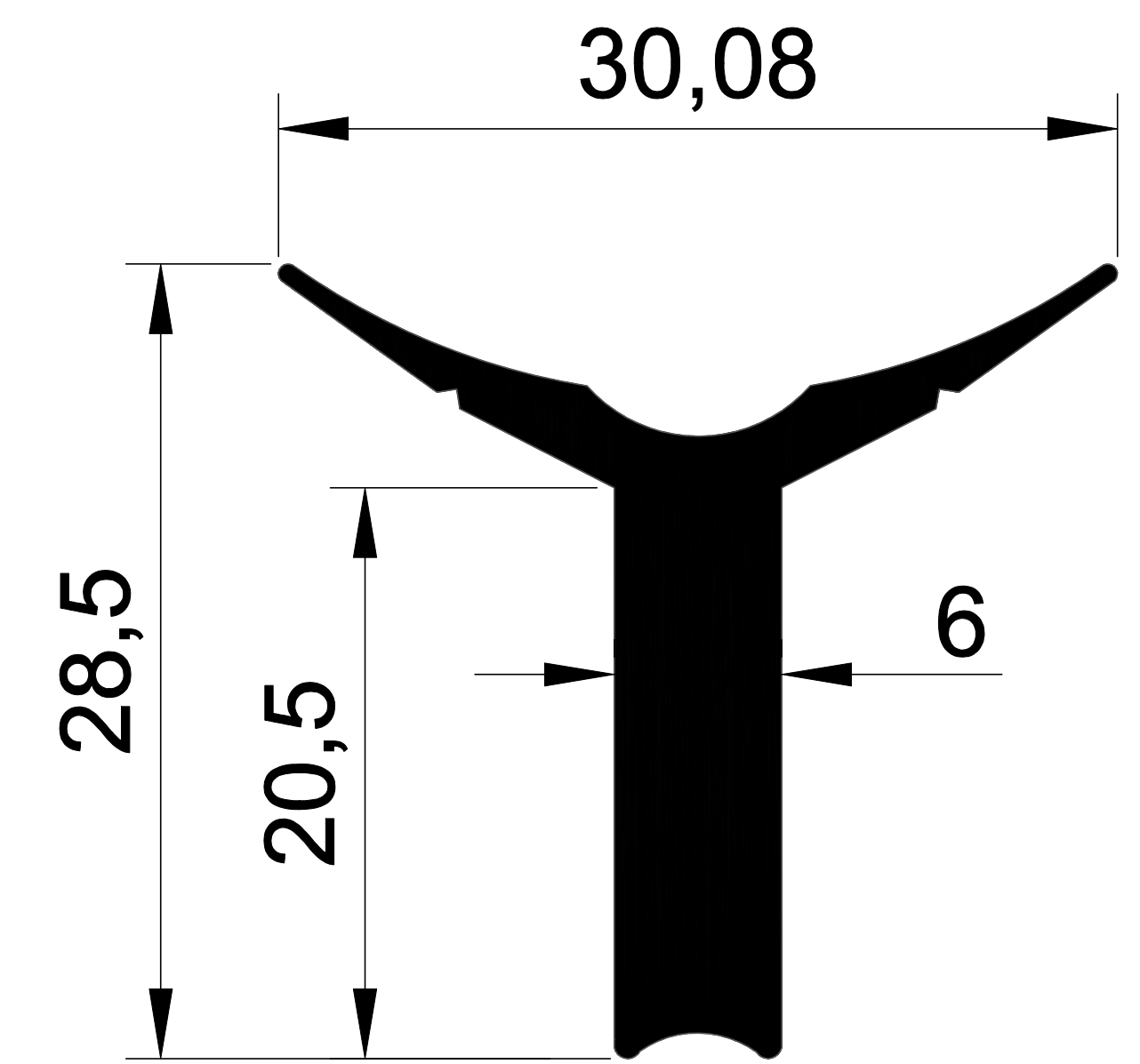
EKOL 1339 0,478 gr/m.
