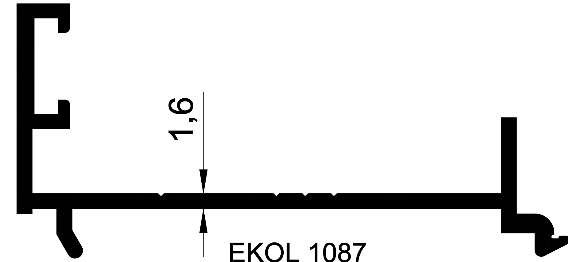
EKOL 1087 0,462 gr/m. C-60 ADAPTÖR
