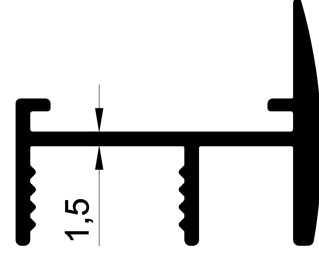
EKOL 1157 0,457 gr/m. MEBO KASA
