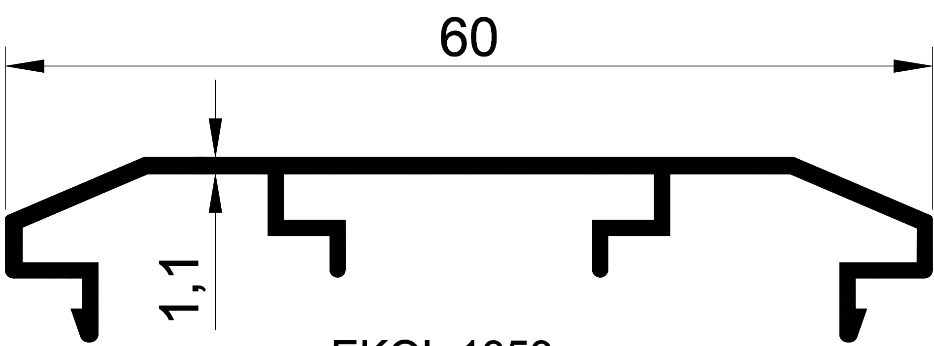
EKOL 1353 0,310 gr/m. C-60 ÇARPMA KAPI ADAPTÖRÜ
