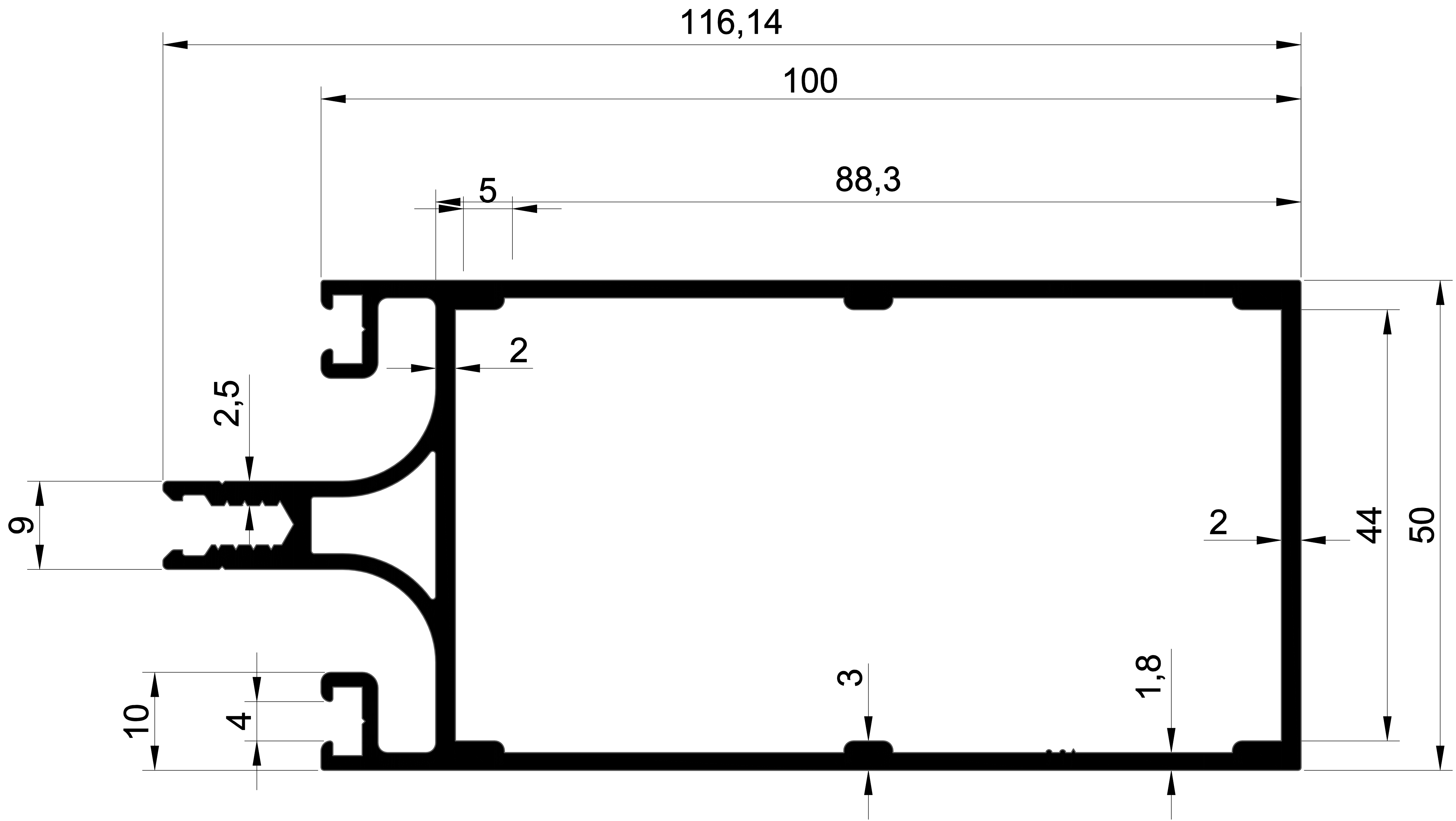
EKOL 1439 2,024 gr/m. 110'LİK CEPHE PROFİLİ UZUN GAGA
