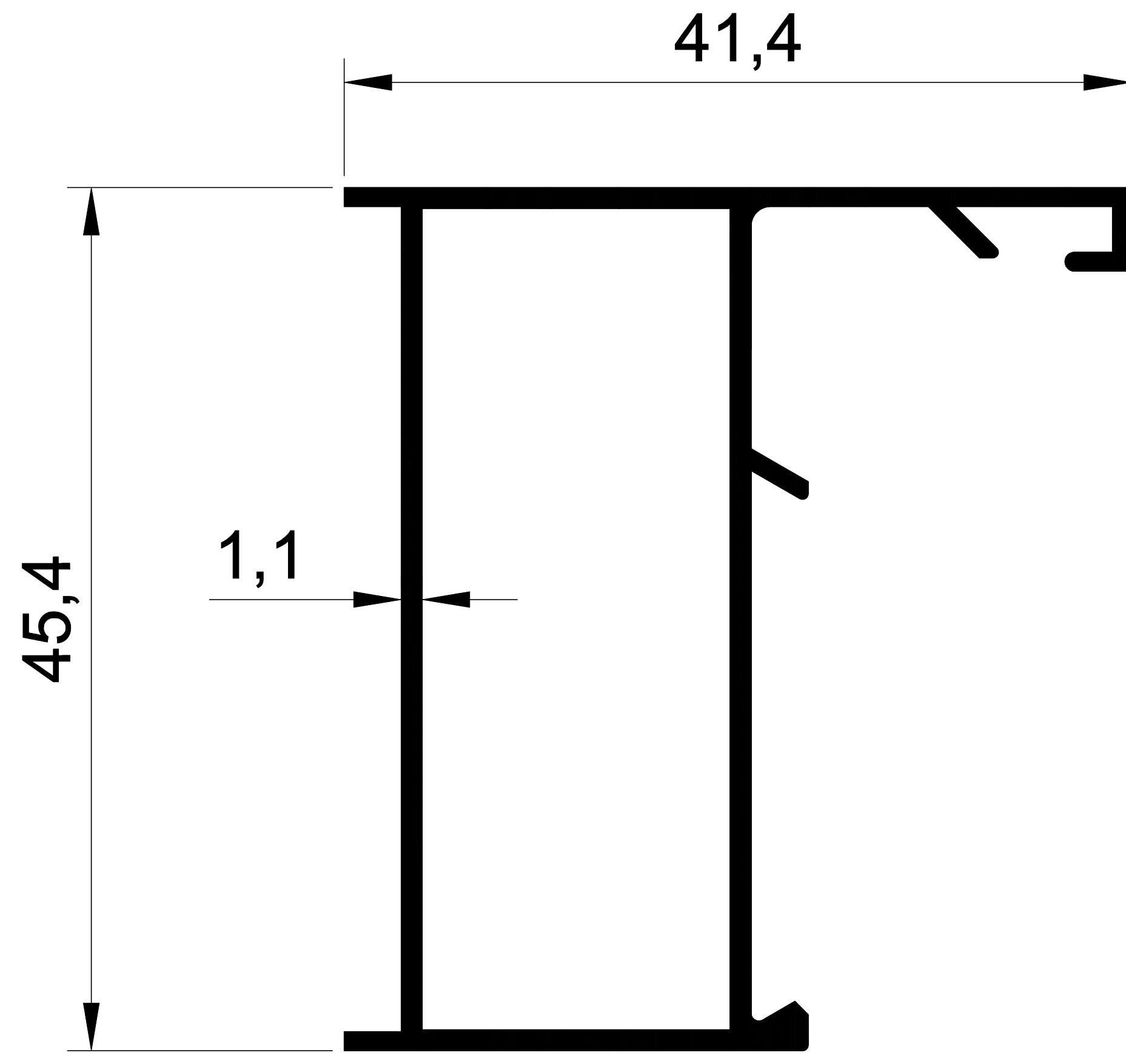
EKOL 1103 0,458 gr/m. ALDOKS DAR KASA
