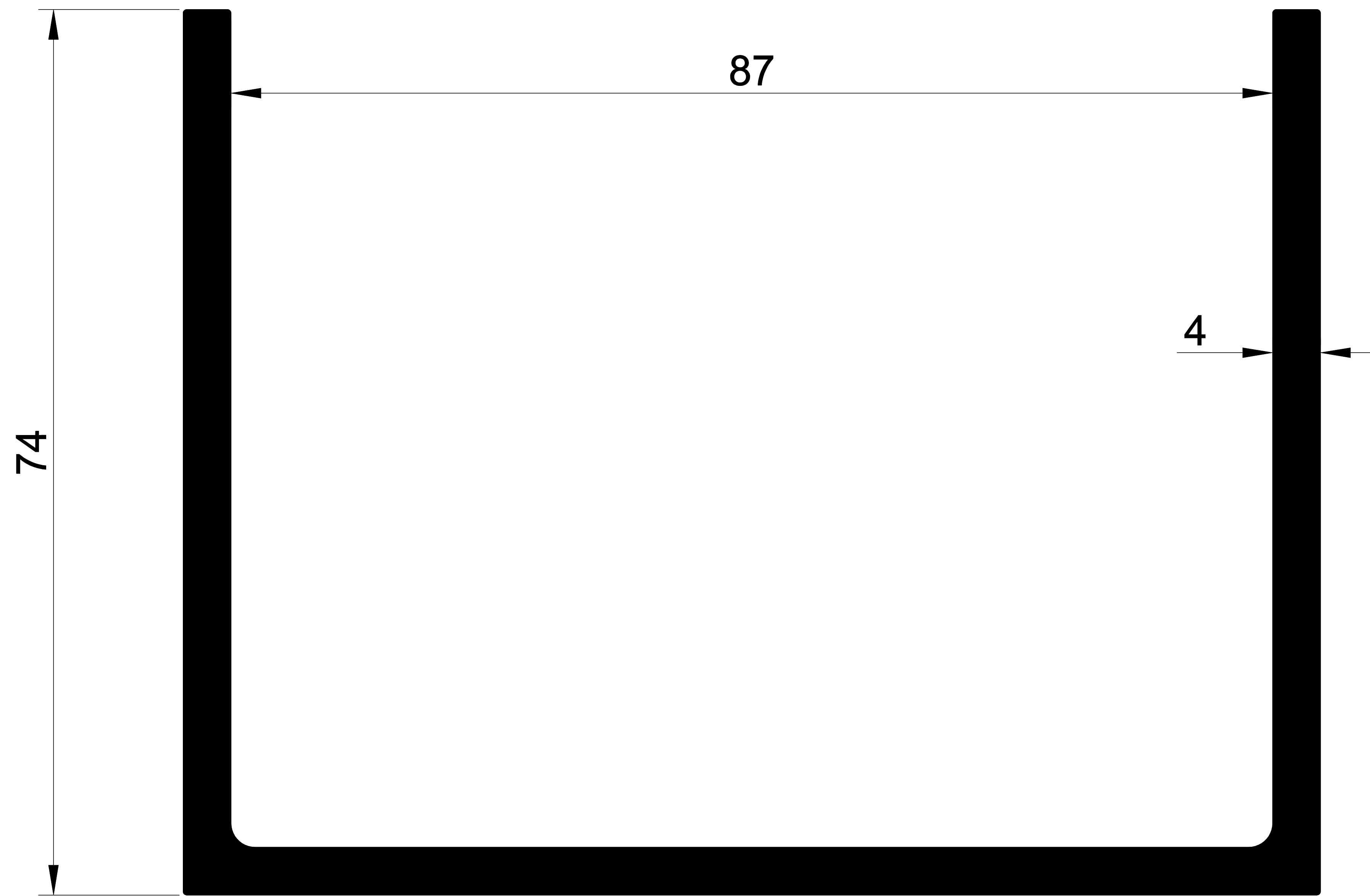
EKOL 1013-B 2,552 gr/m.
