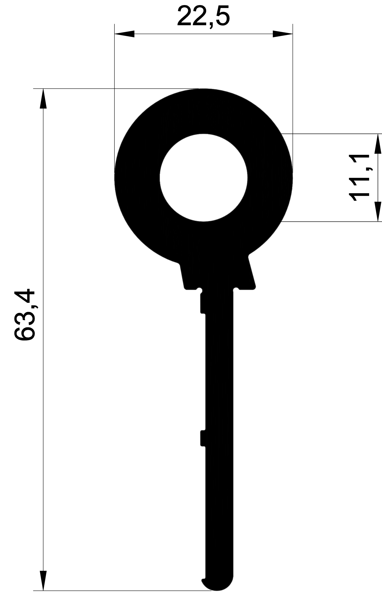
EKOL 1010-B 1,261 gr/m.
