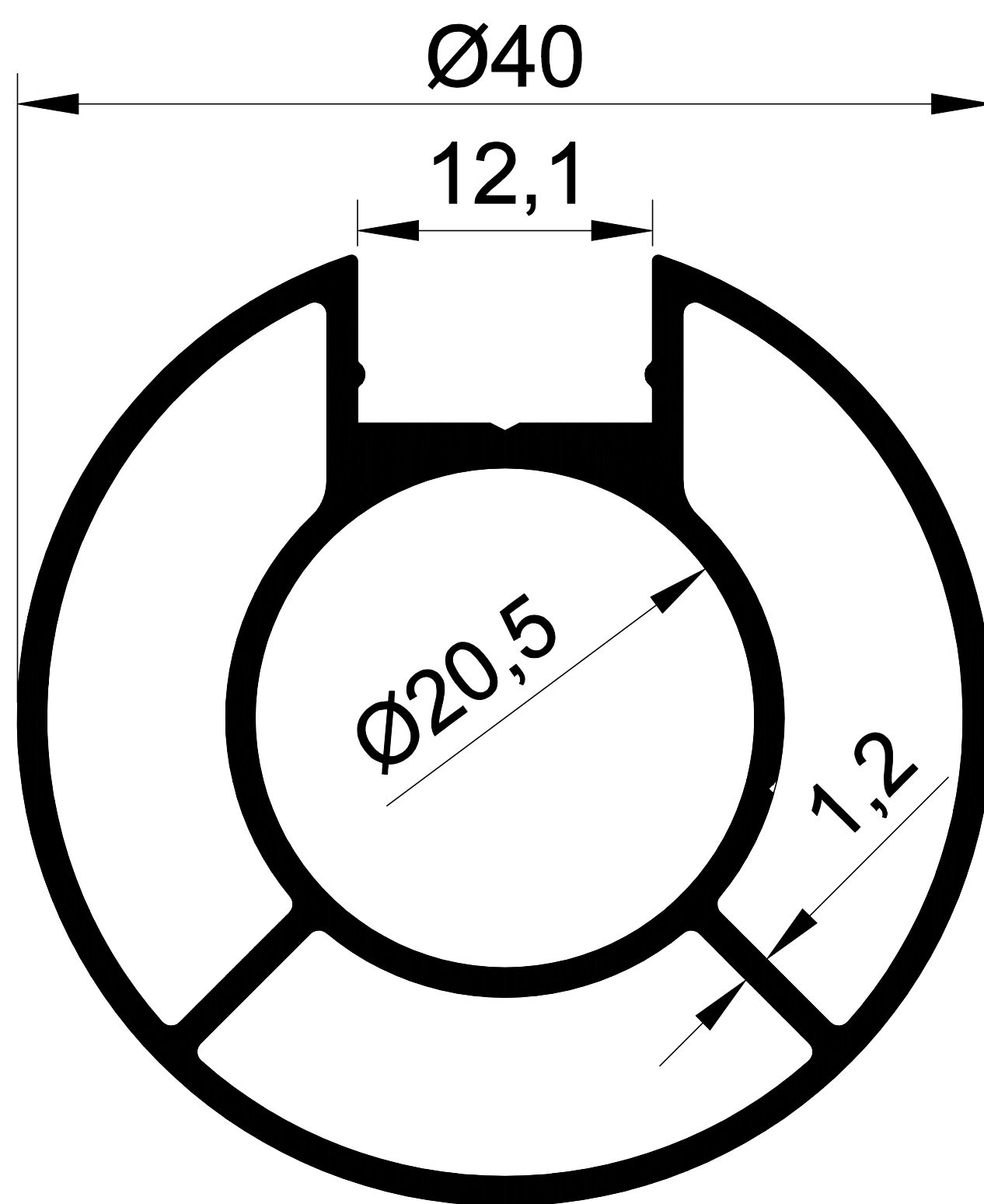
EKOL 1064 0,723 gr/m.
