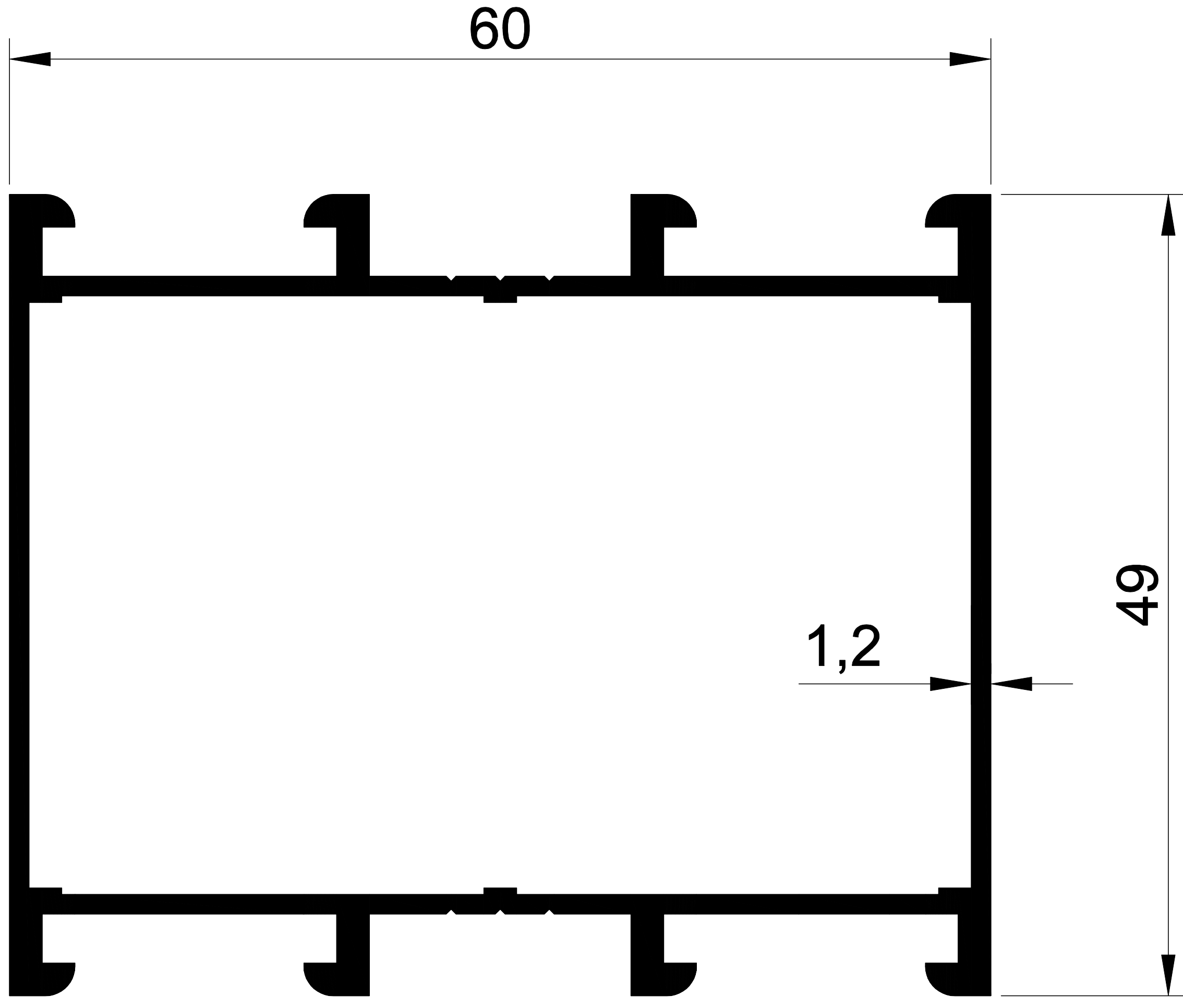
EKOL 1089 0,928 gr/m. 1.2 MM C-60 KASA
