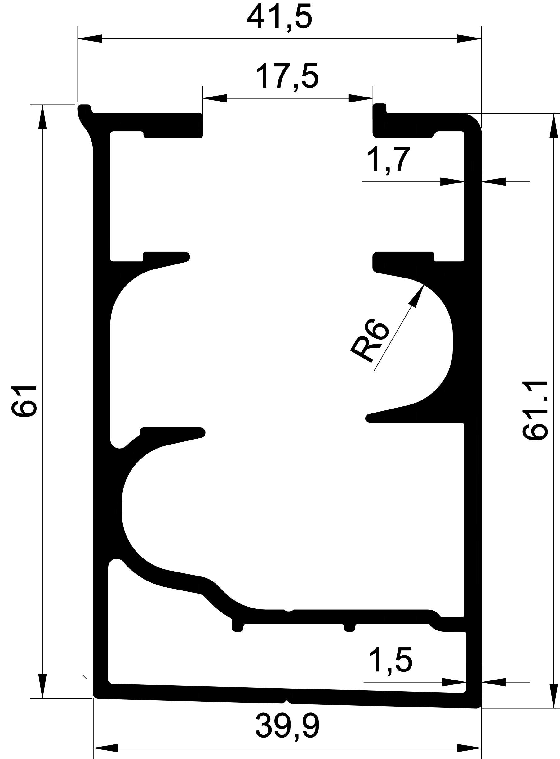
EKOL 1187-E 1,292 gr/m. BKS EĞİMLİ KASA
