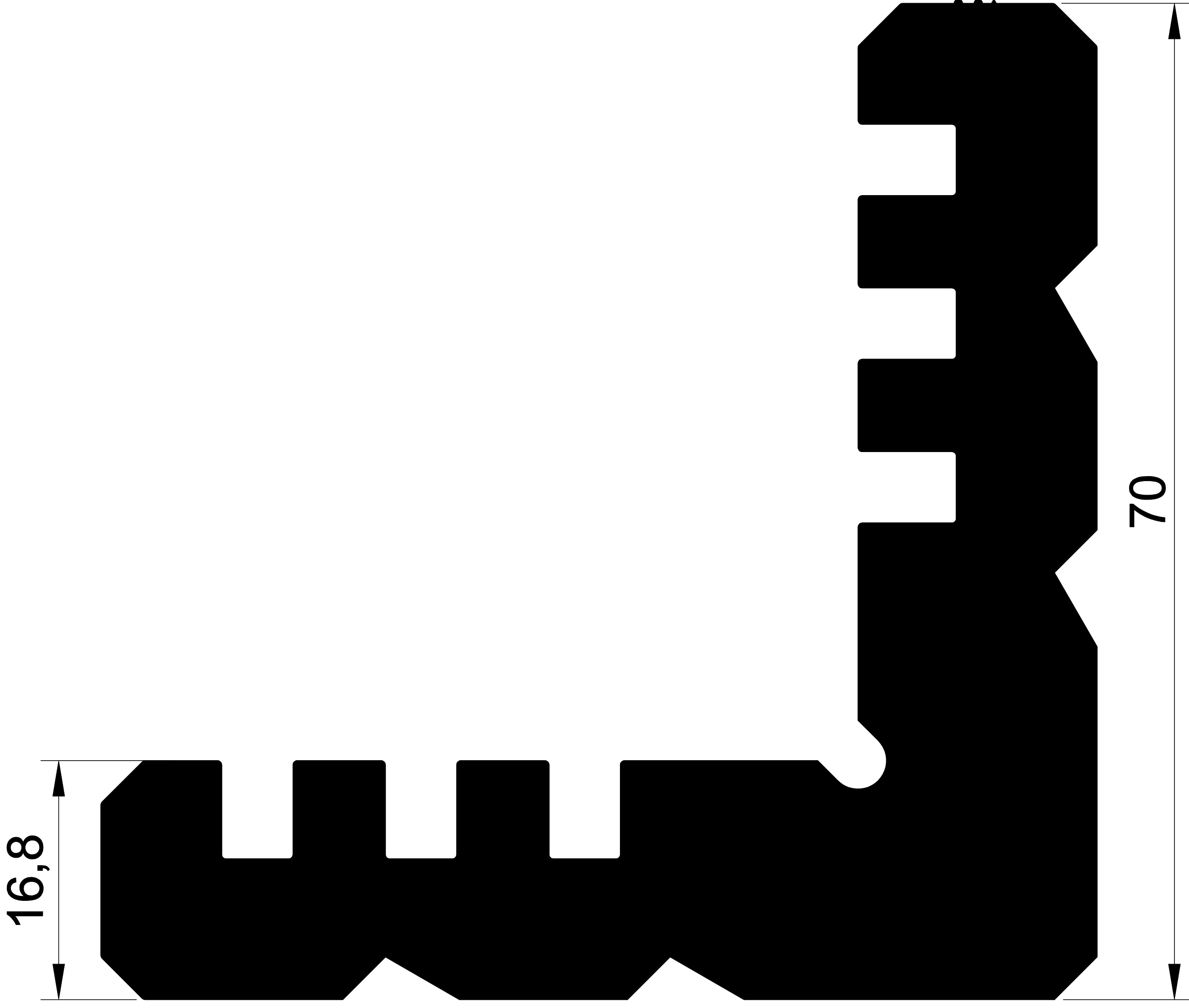
EKOL 1399 4,827 gr/m. 17 MM CEPHE KÖŞE
