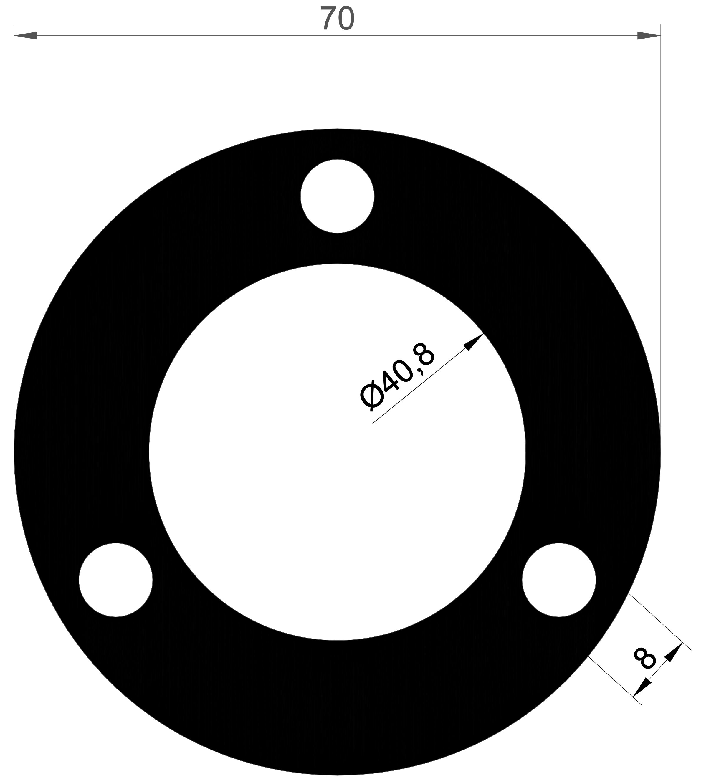
EKOL 1021 6,477 gr/m.
