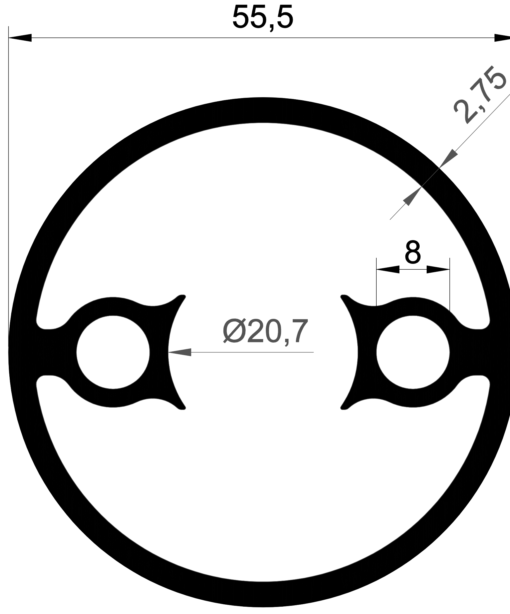
EKOL 1017-B 1,743 gr/m.
