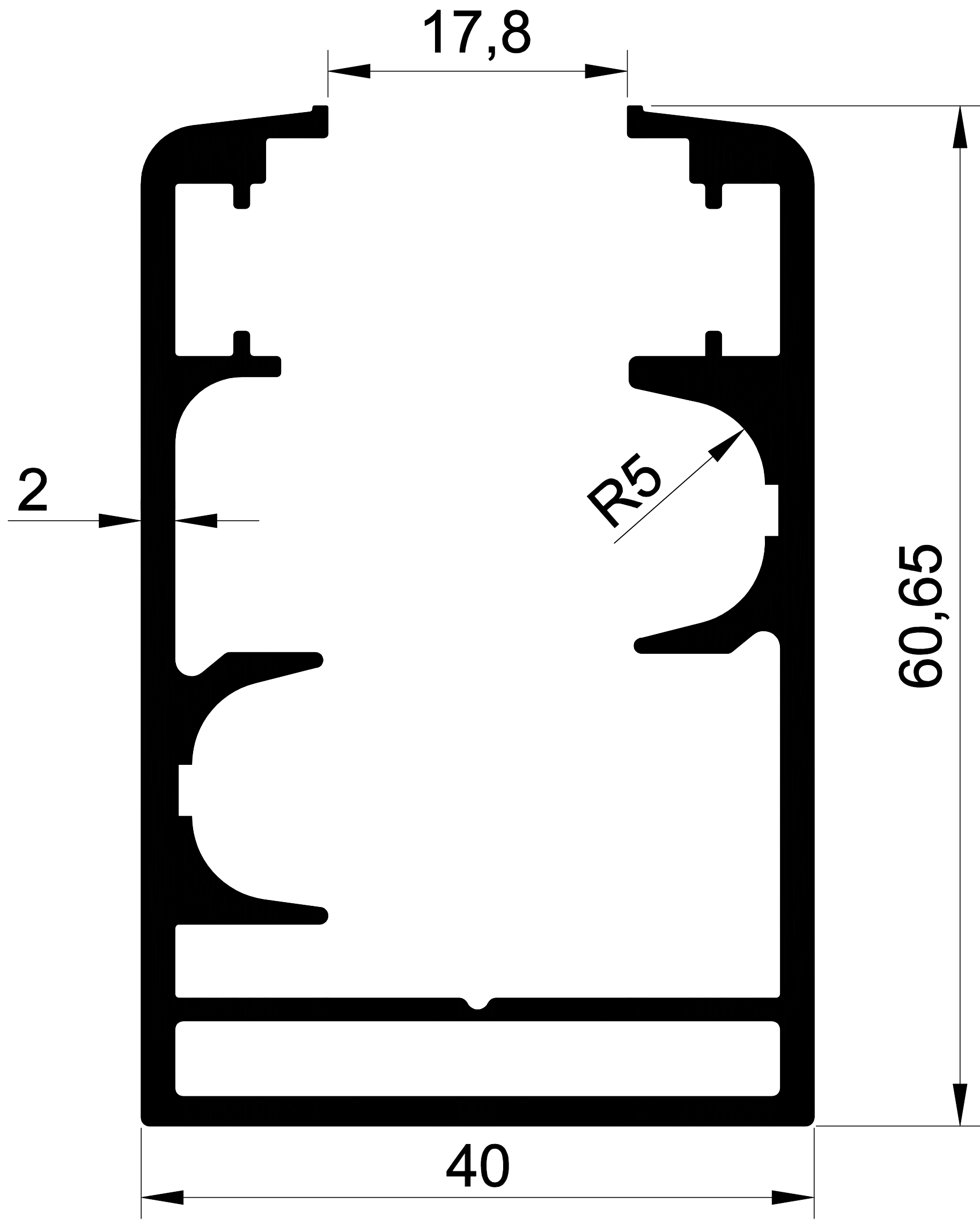
EKOL 1212 1,371 gr/m. FIRTINA KASA
