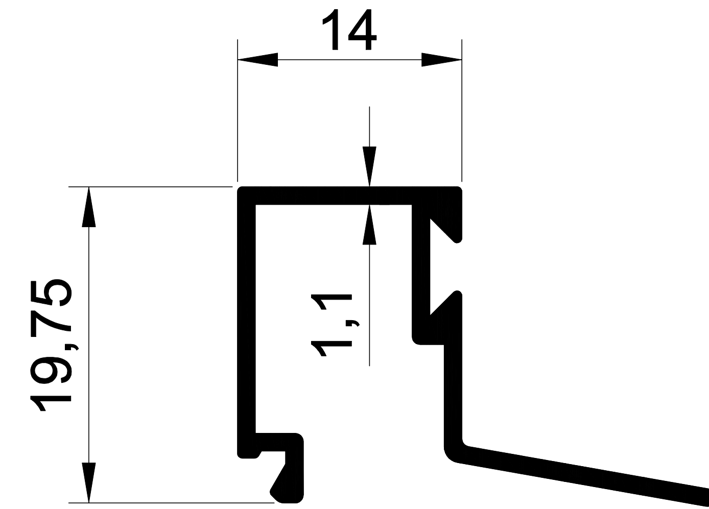
EKOL 1091 0,232 gr/m. ALDOKS ISI CAM ÇİTASI
