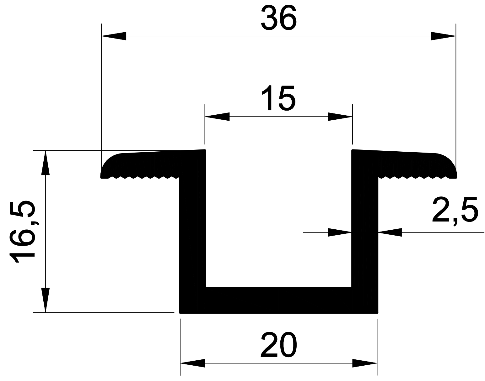
EKOL 1430 0,420 gr/m GES PANEL TUTUCU APARATI ORTA
