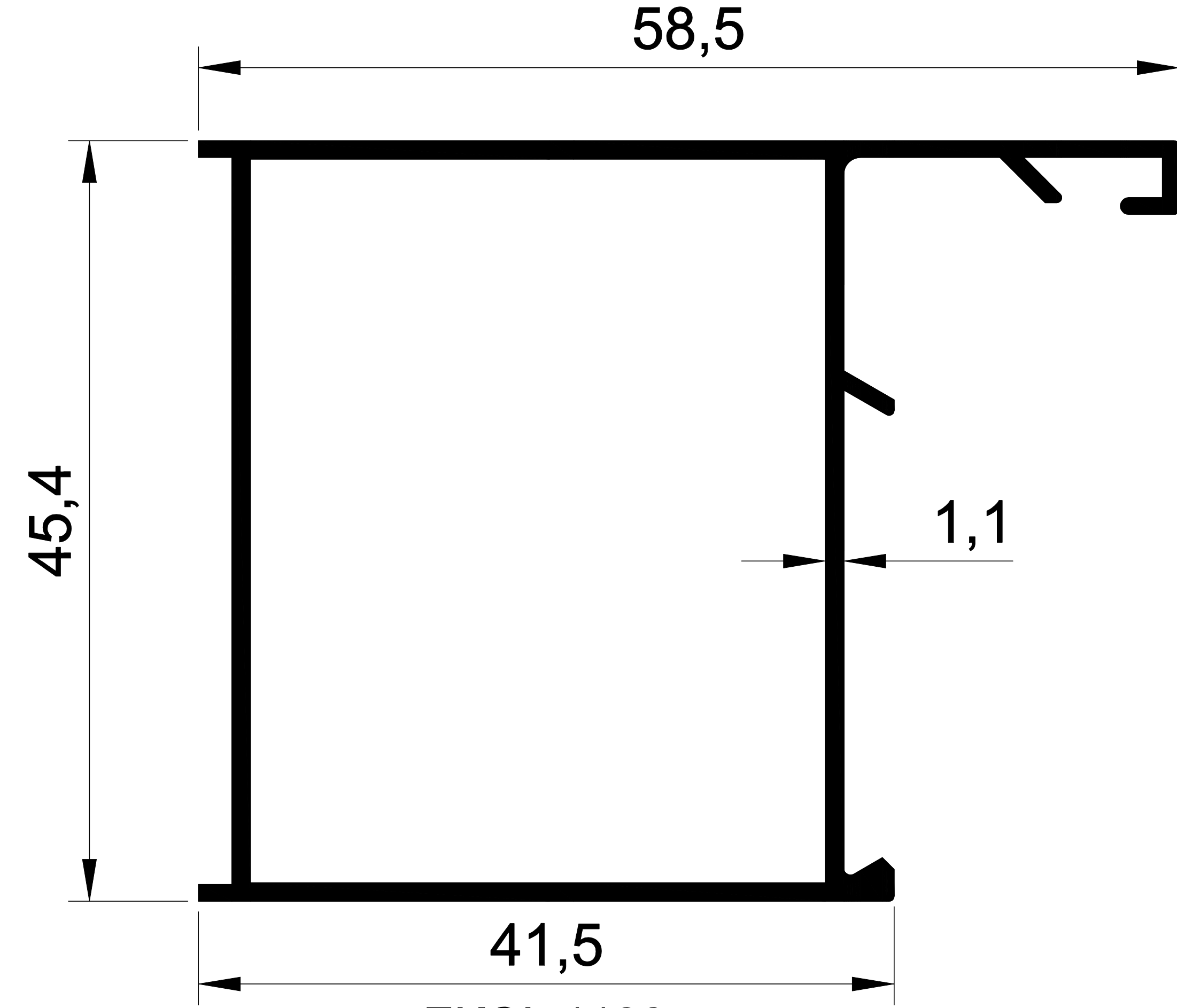
EKOL 1106 0,550 gr/m. ALDOKS GENİŞ KASA
