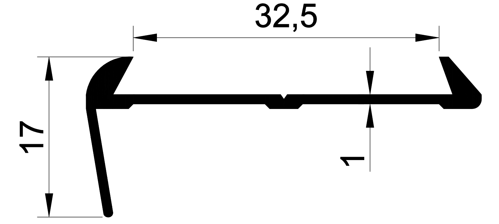
EKOL 1366 0,213 gr/m. MERDİVEN PROFİLİ
