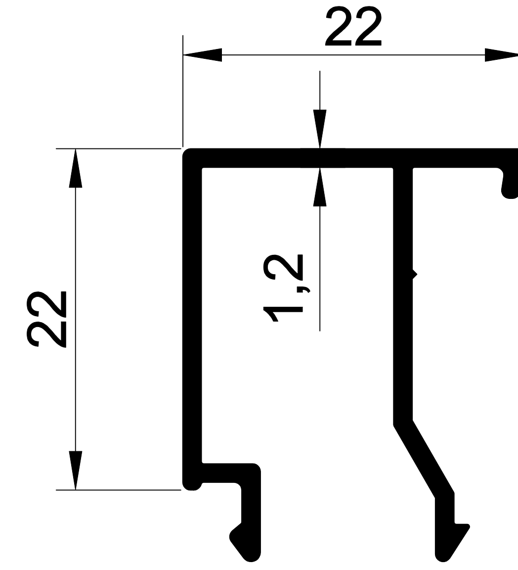
EKL-55- 2008 0,264 gr/m SİSTEM 55 ÇİFT CAM ÇITASI
