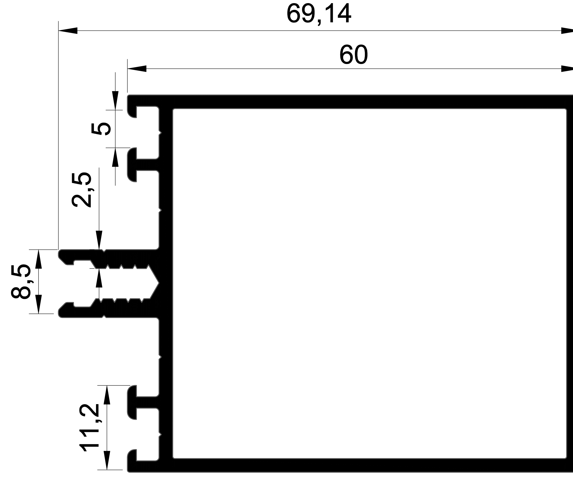
EKOL 1442 1,251 gr/m. 60'LIK CEPHE PROFİLİ
