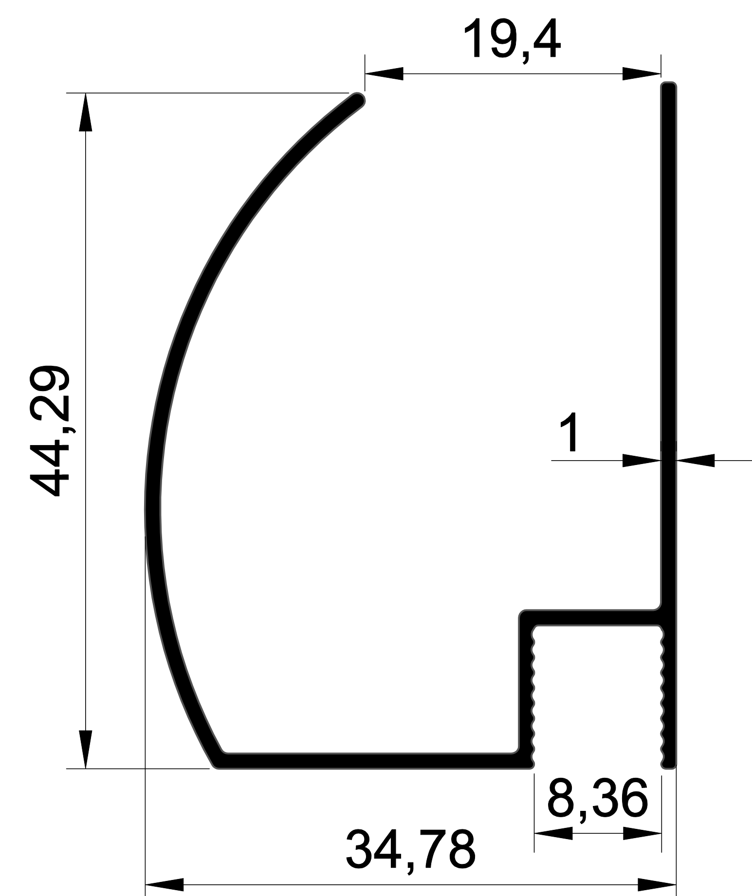
EKOL 1454 0.353 gr/m. KENAR PROFİLİ
