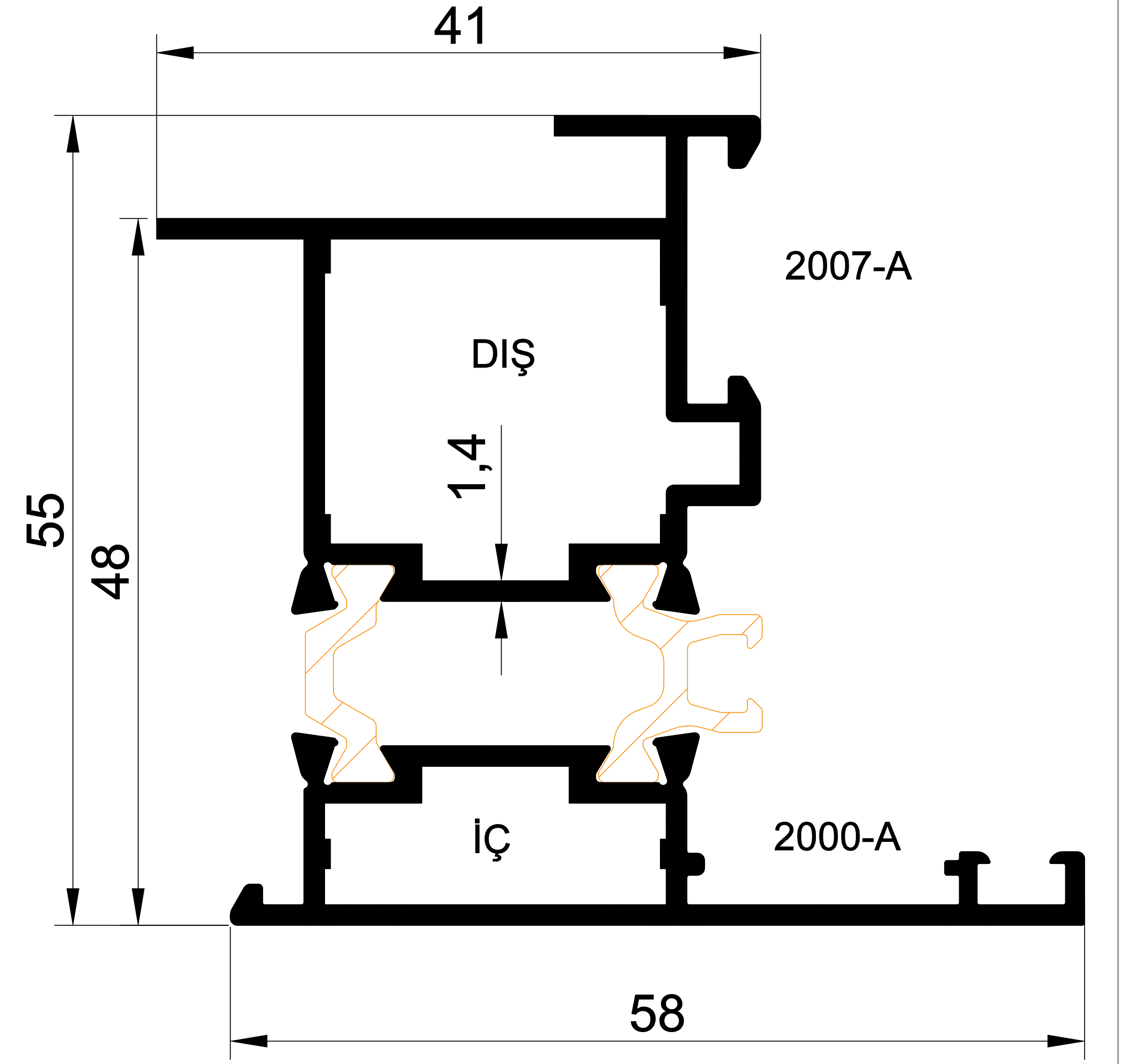
EKL-55- 2007 1,084 gr/m SİSTEM 55 ISI YALITIM TERS KAPI ADAPTÖRÜ
