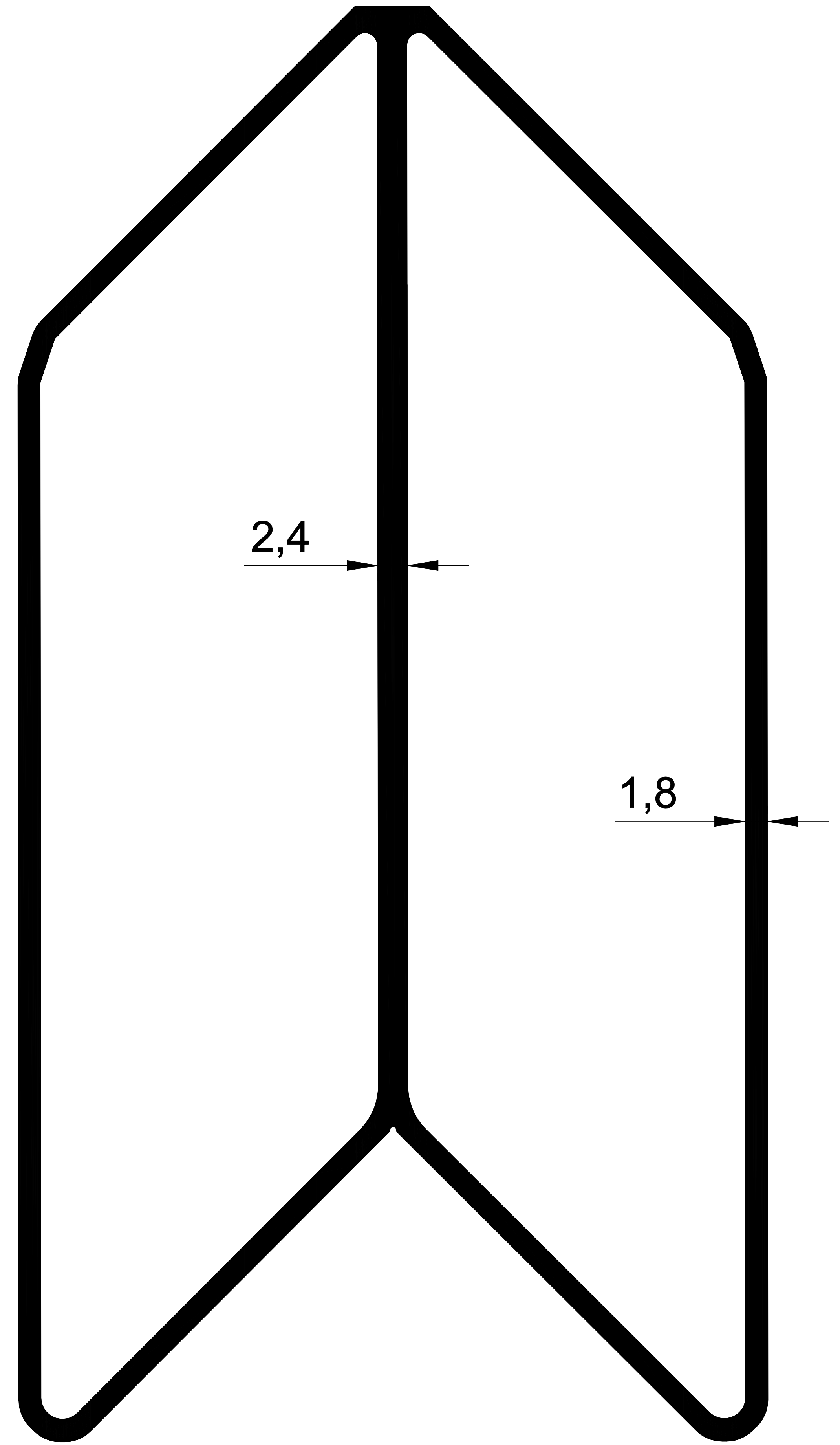
EKOL 1092 2,205 gr/m. BAZA ÇAVUŞ (GENİŞ BAĞLANTI)
