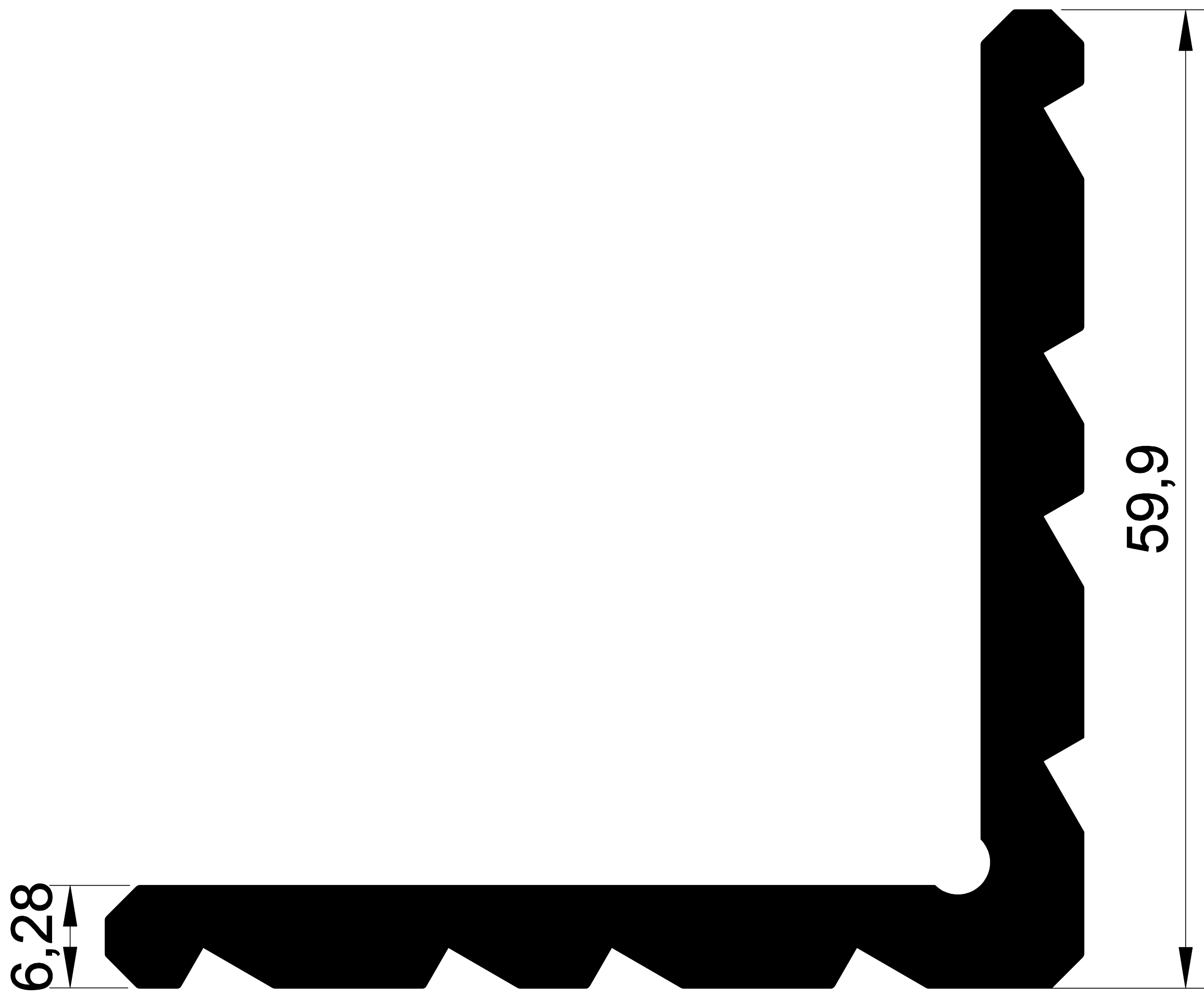
EKOL 1401 1,748 gr/m. 6 MM CEPHE KÖŞE
