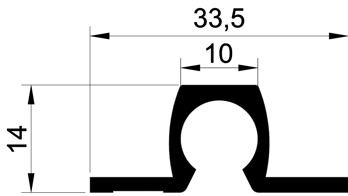
EKOL 1232 0,314 gr/m.
