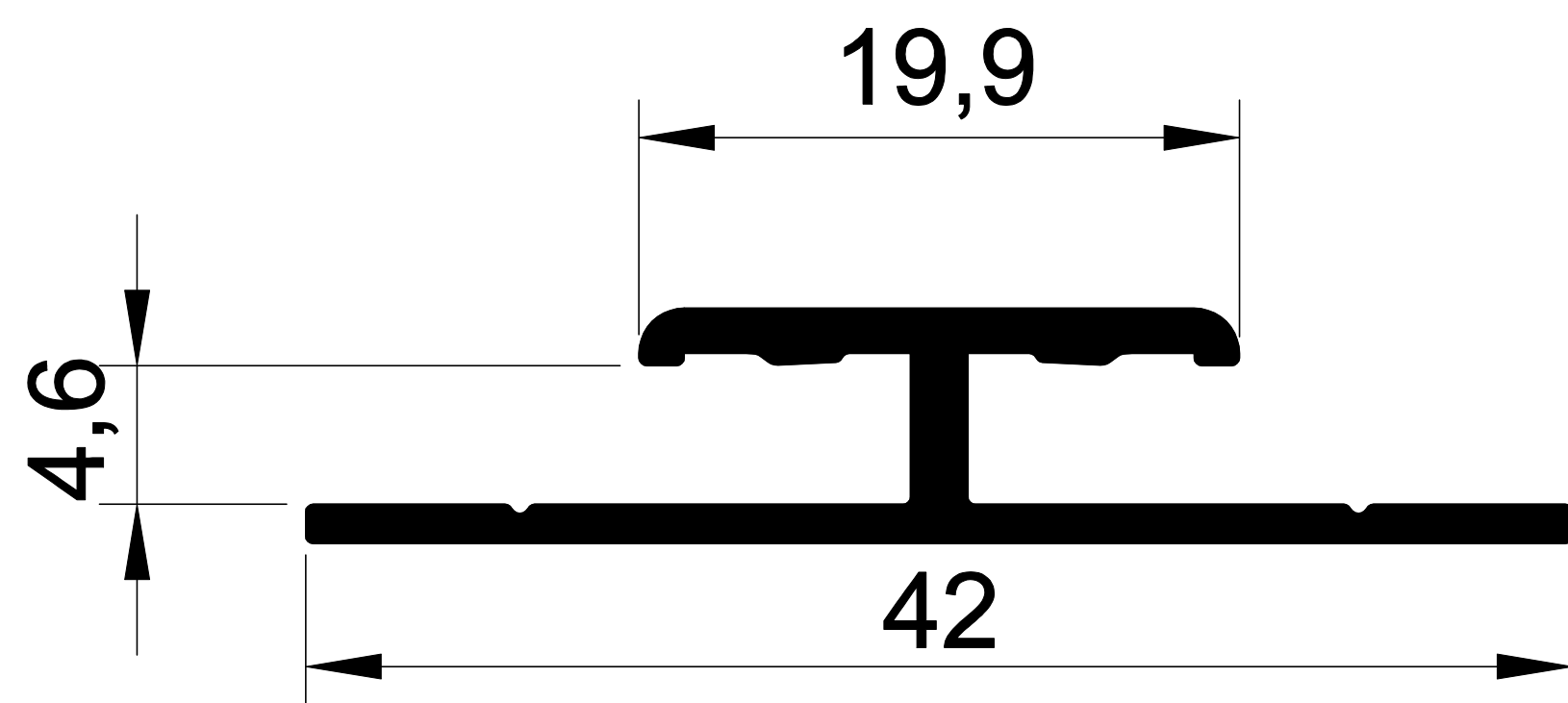
EKOL 1207 0,260 gr/m. KOMPAZİT - H
