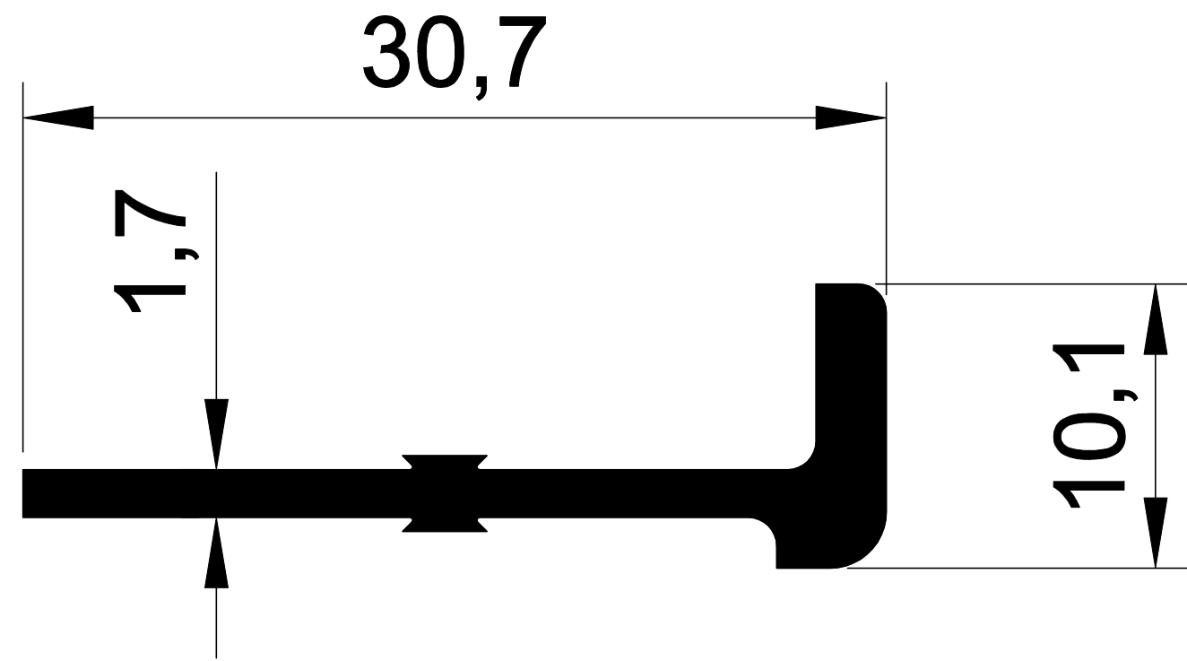
EKOL 1394 0,203 gr/m. CEPHE AYAR TAKOZU
