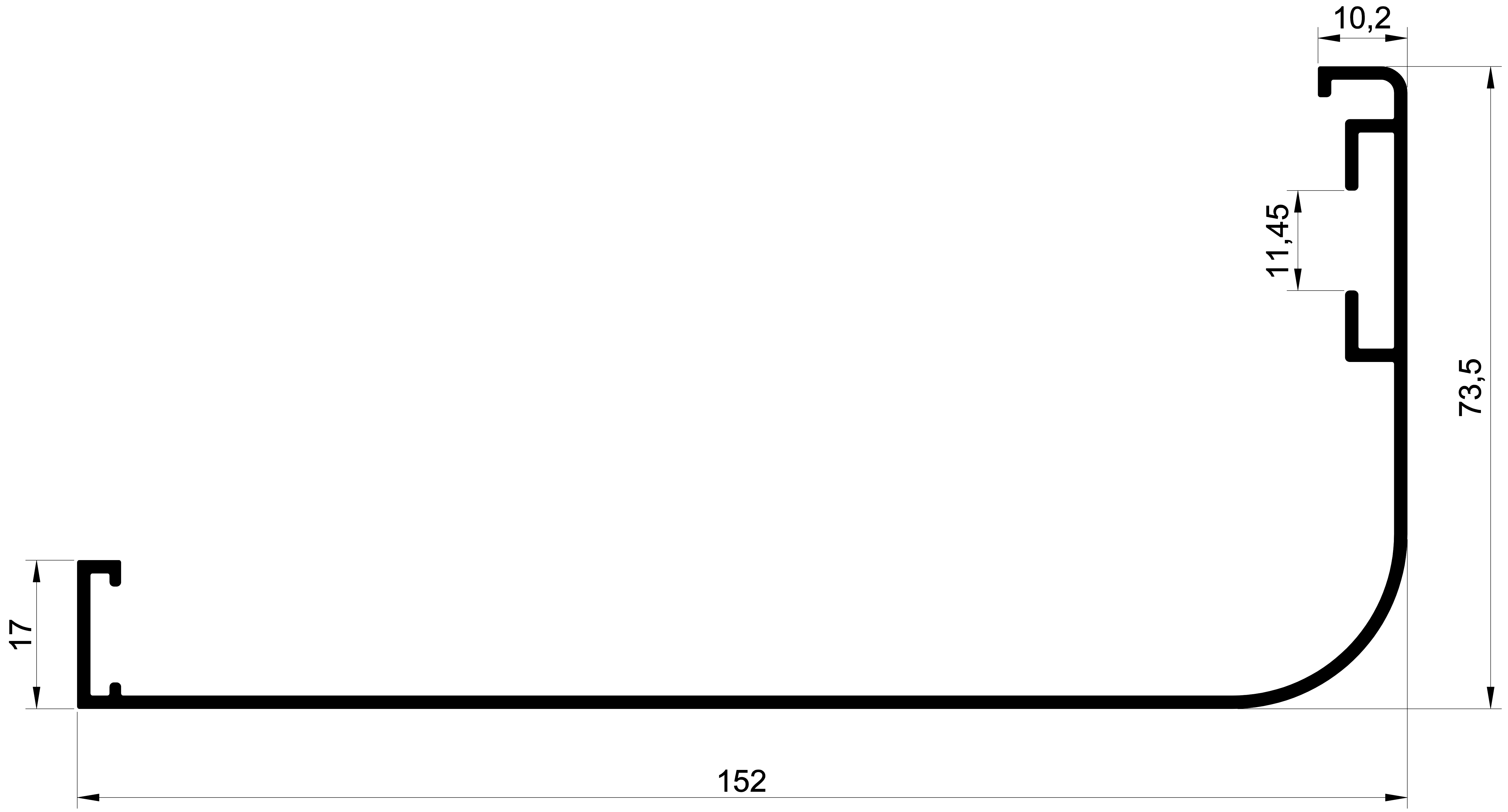
EKOL 1425 1,102 gr/m. MS-152'LİK PEERVAZ
