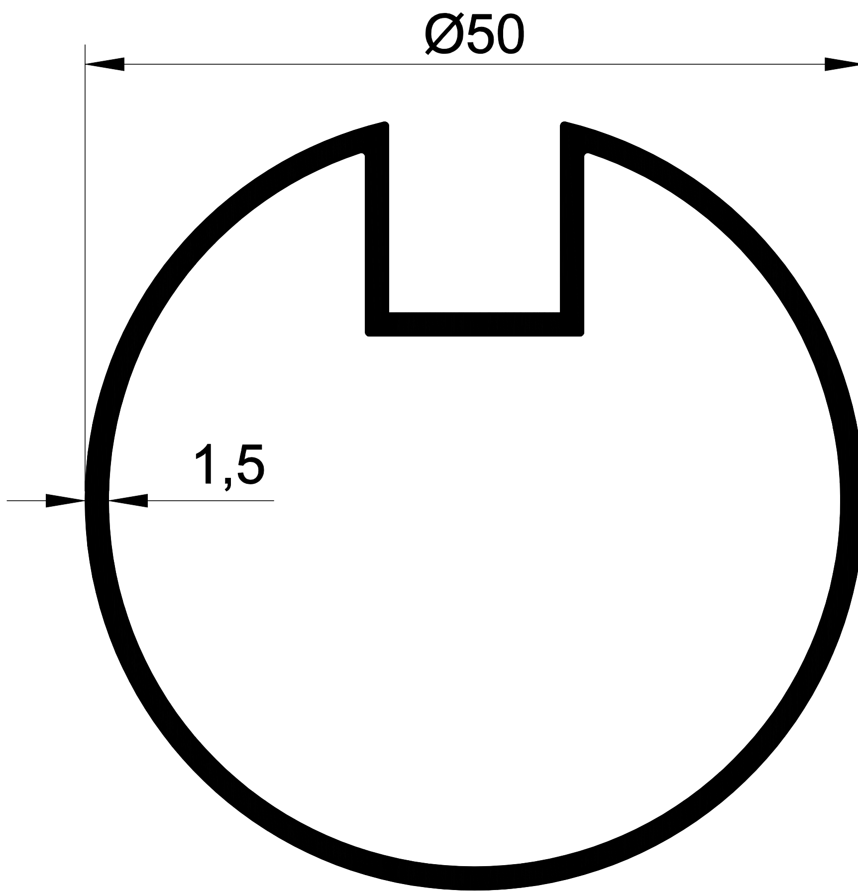
EKOL 1069 0,715gr/m.
