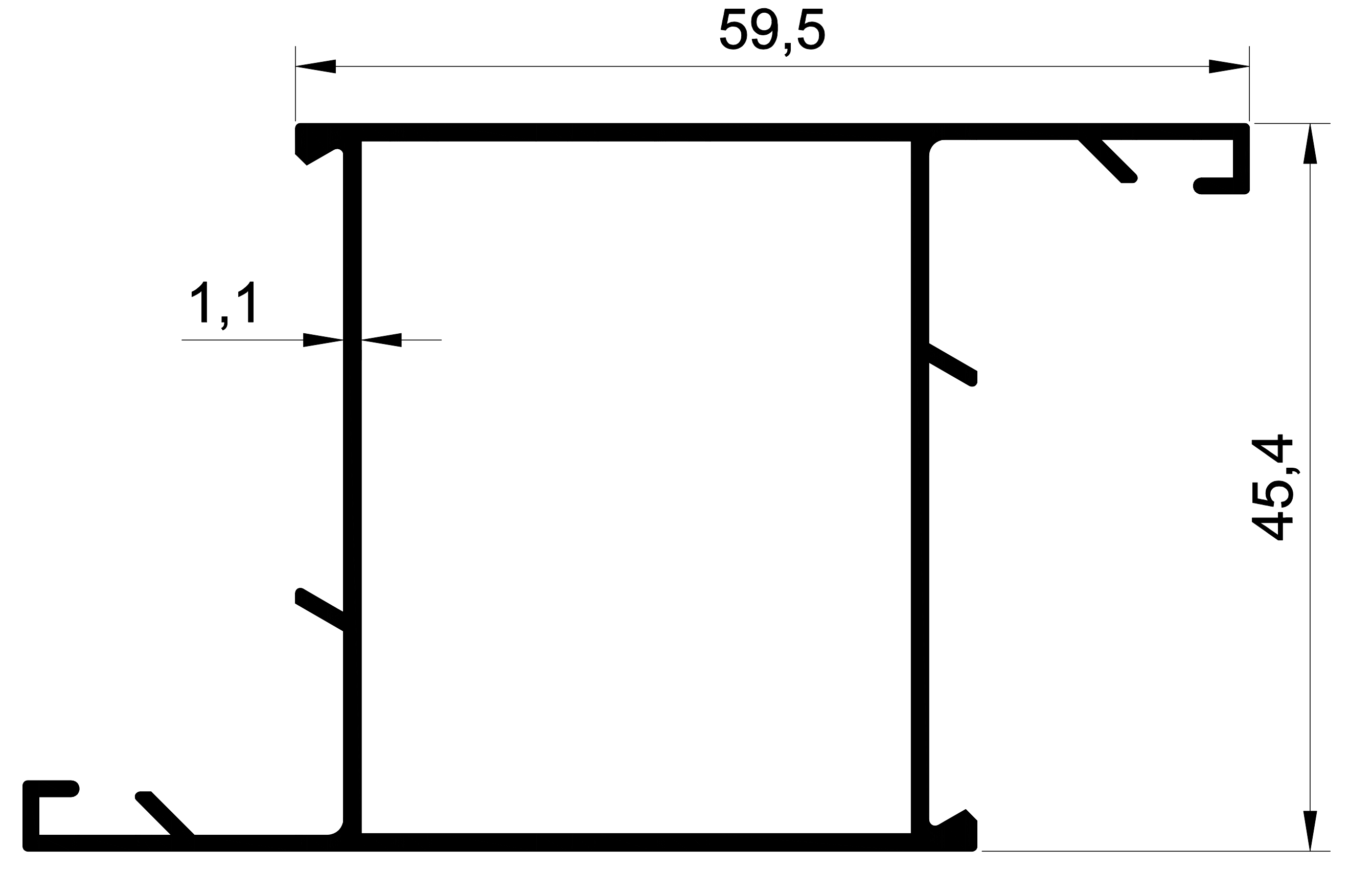
EKOL 1104 0,645gr/m. ALDOKS GENİŞ KANAT
