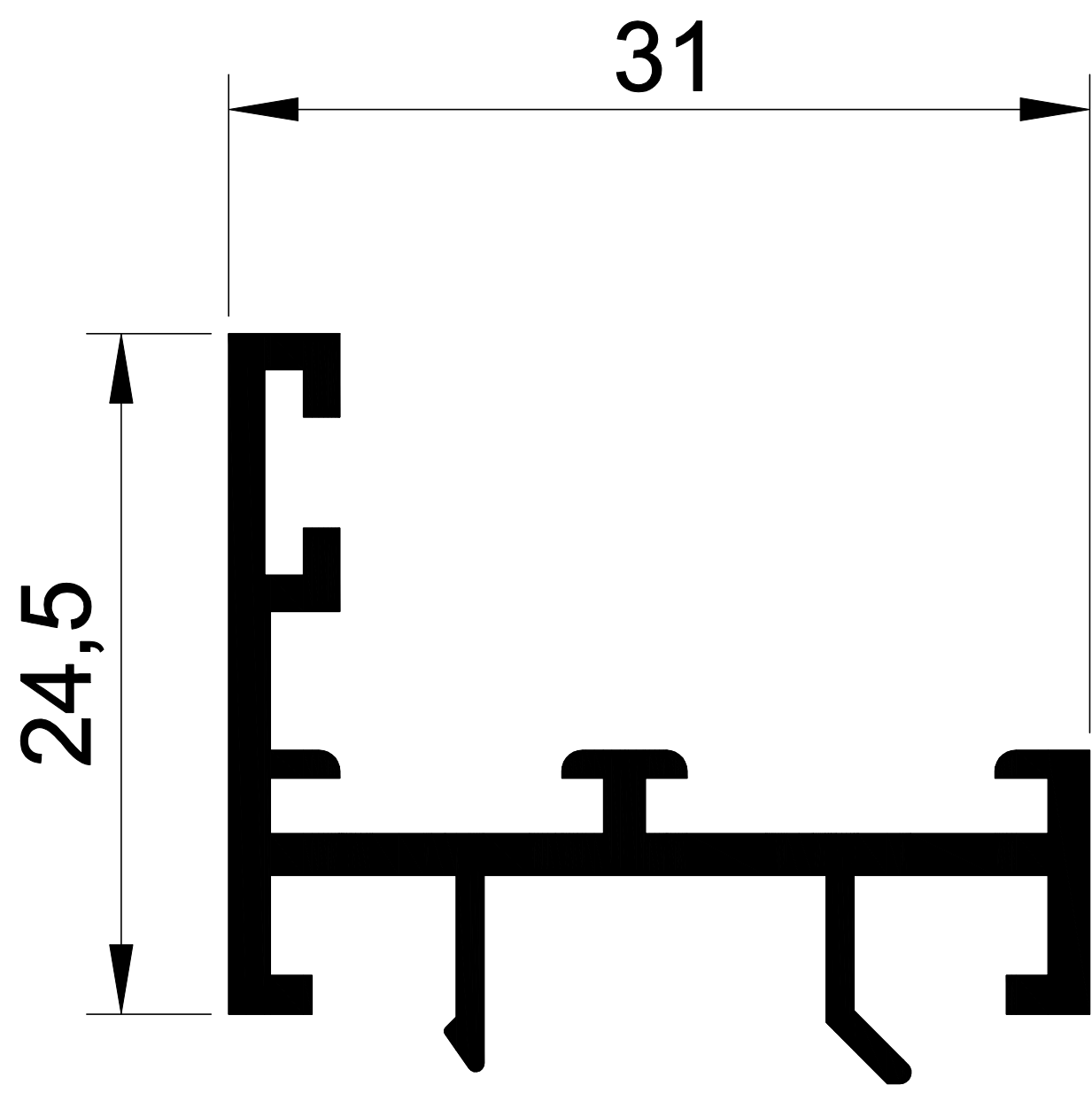
EKOL 1194 0,360 gr/m DAR TUBA TIRNAK
