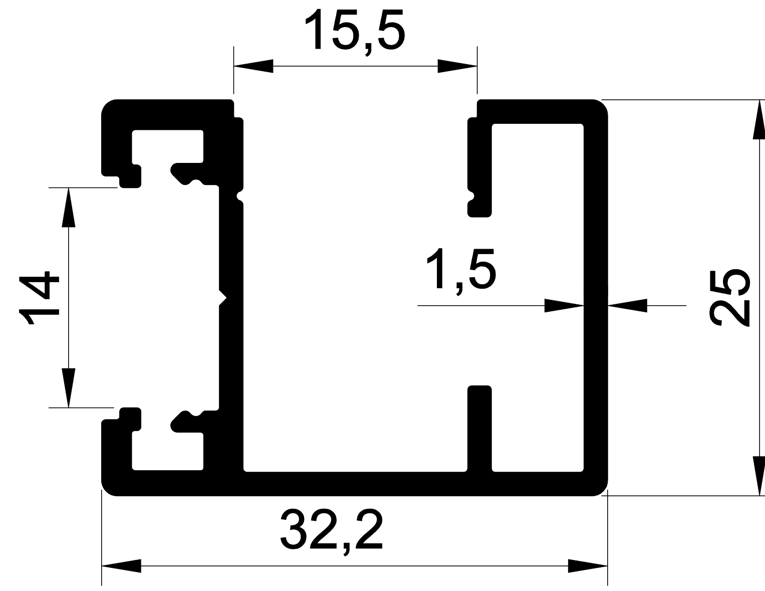
EKOL 1269 0,504 gr/m 32*25 GEMİCİ
