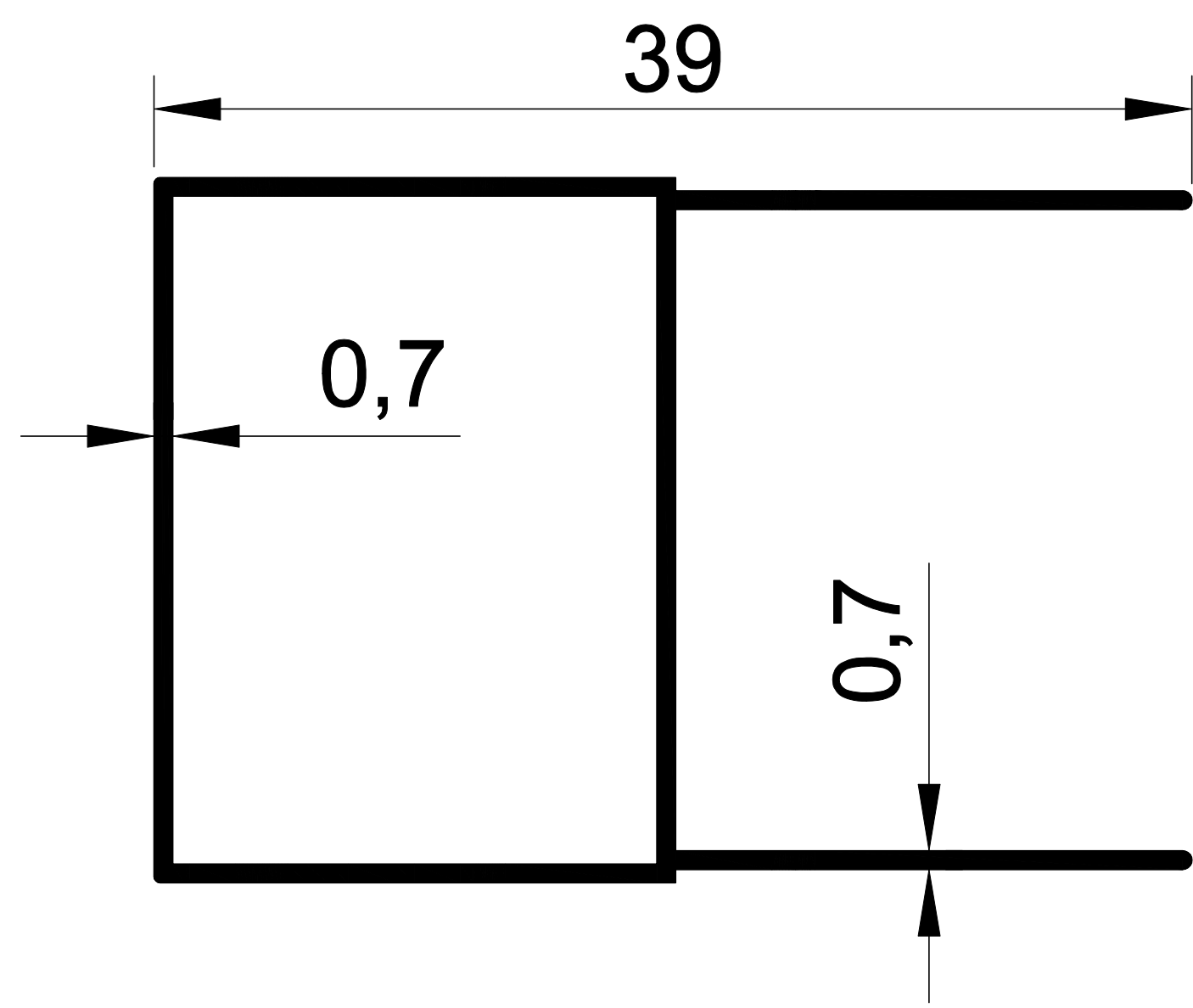
EKOL 1325 0,243 gr/m. MAVİ AY SİNEKLİK KASA
