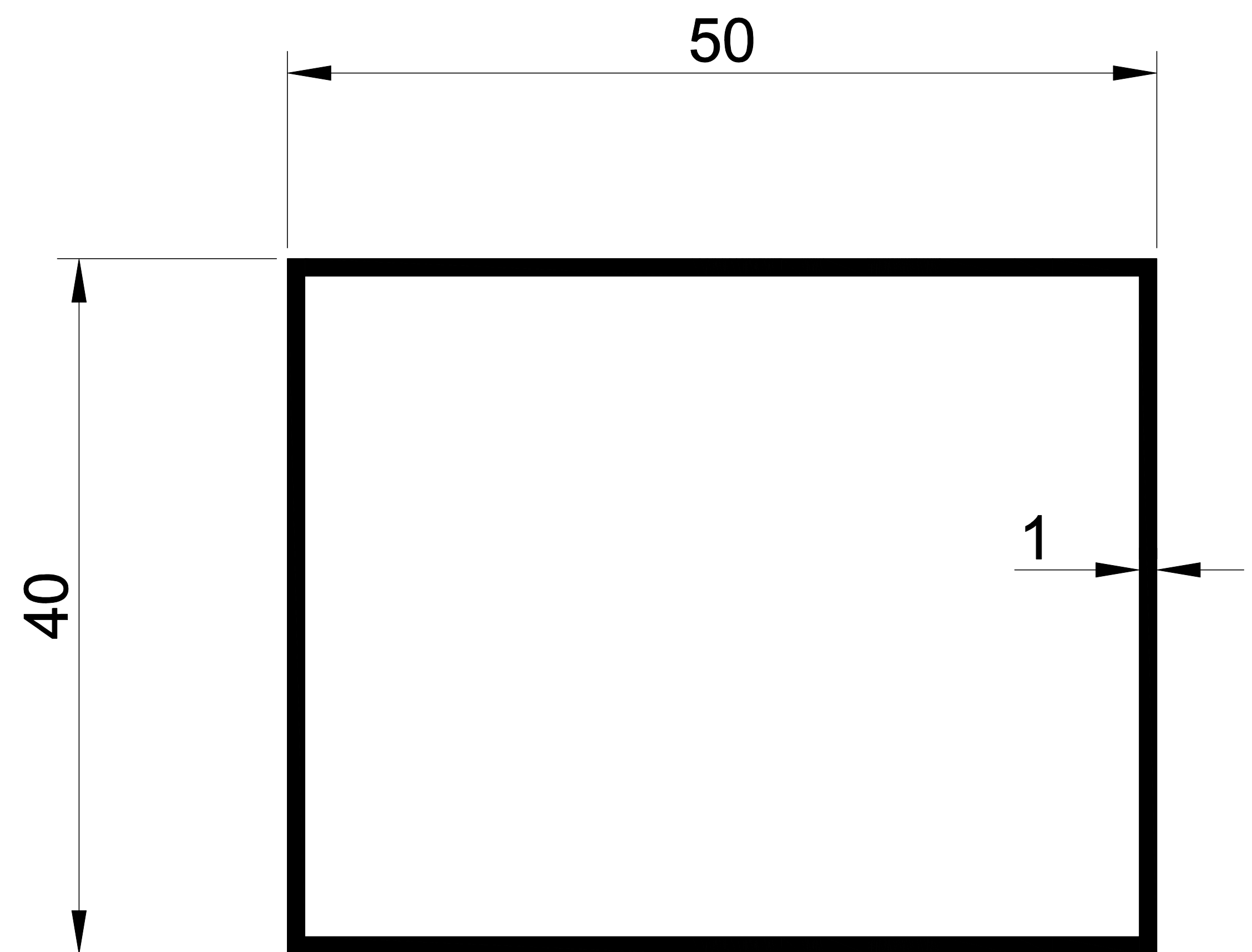
EKOL 1093 0,454 gr/m. 40*50 KUTU
