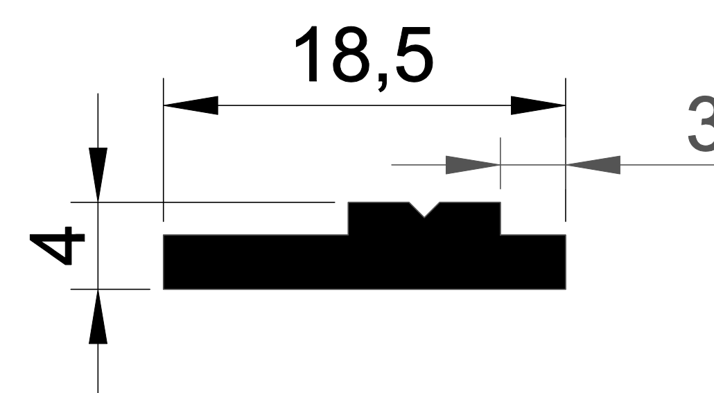
EKOL 1229 0,152 gr/m.
