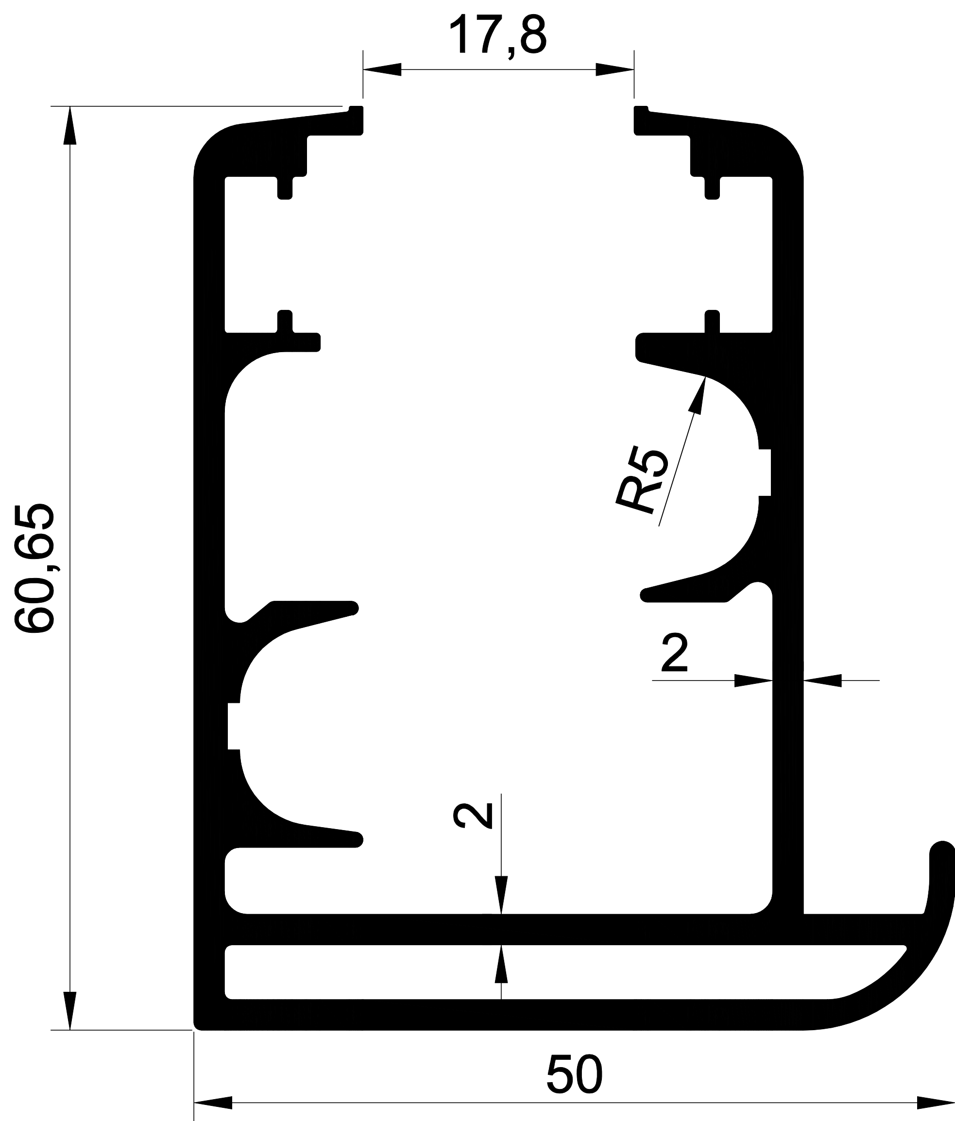
EKOL 1271 1,561 gr/m. FIRTINA DAMLALIKLI KASA
