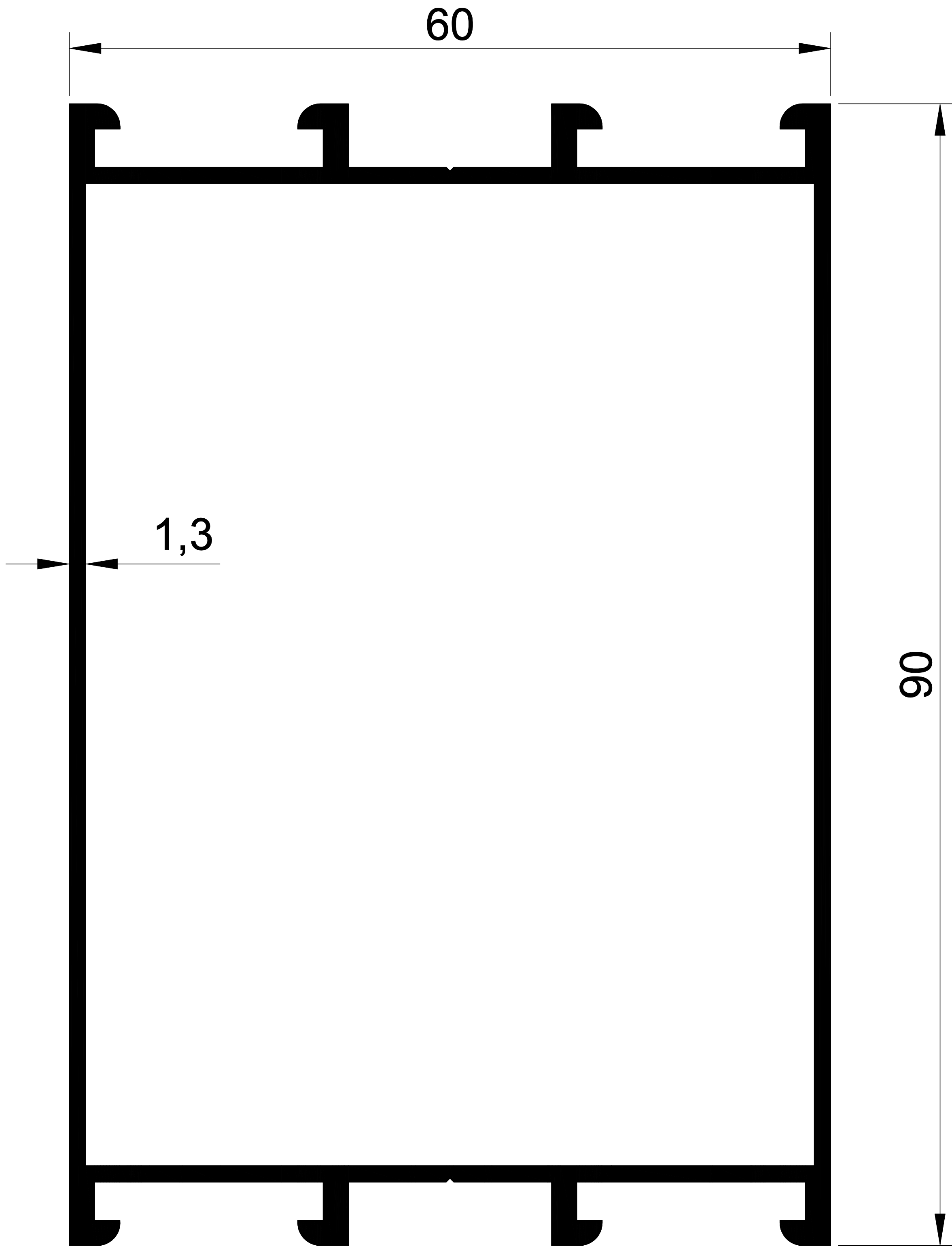
EKOL 1084 1,255 gr/m. C-90 KASA
