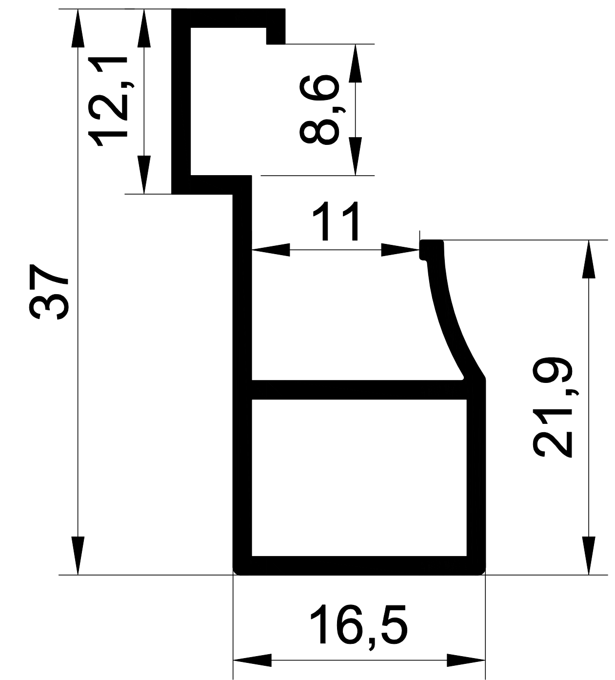
GİZLİ VİDALI MİNİ GEMİCİ EKOL 1458 0,320 gr/m
