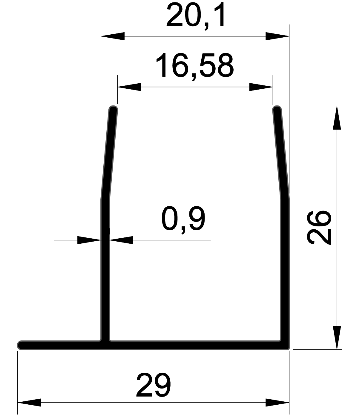
EKOL 1452 0.193 gr/m. DUVAR DİKMESİ
