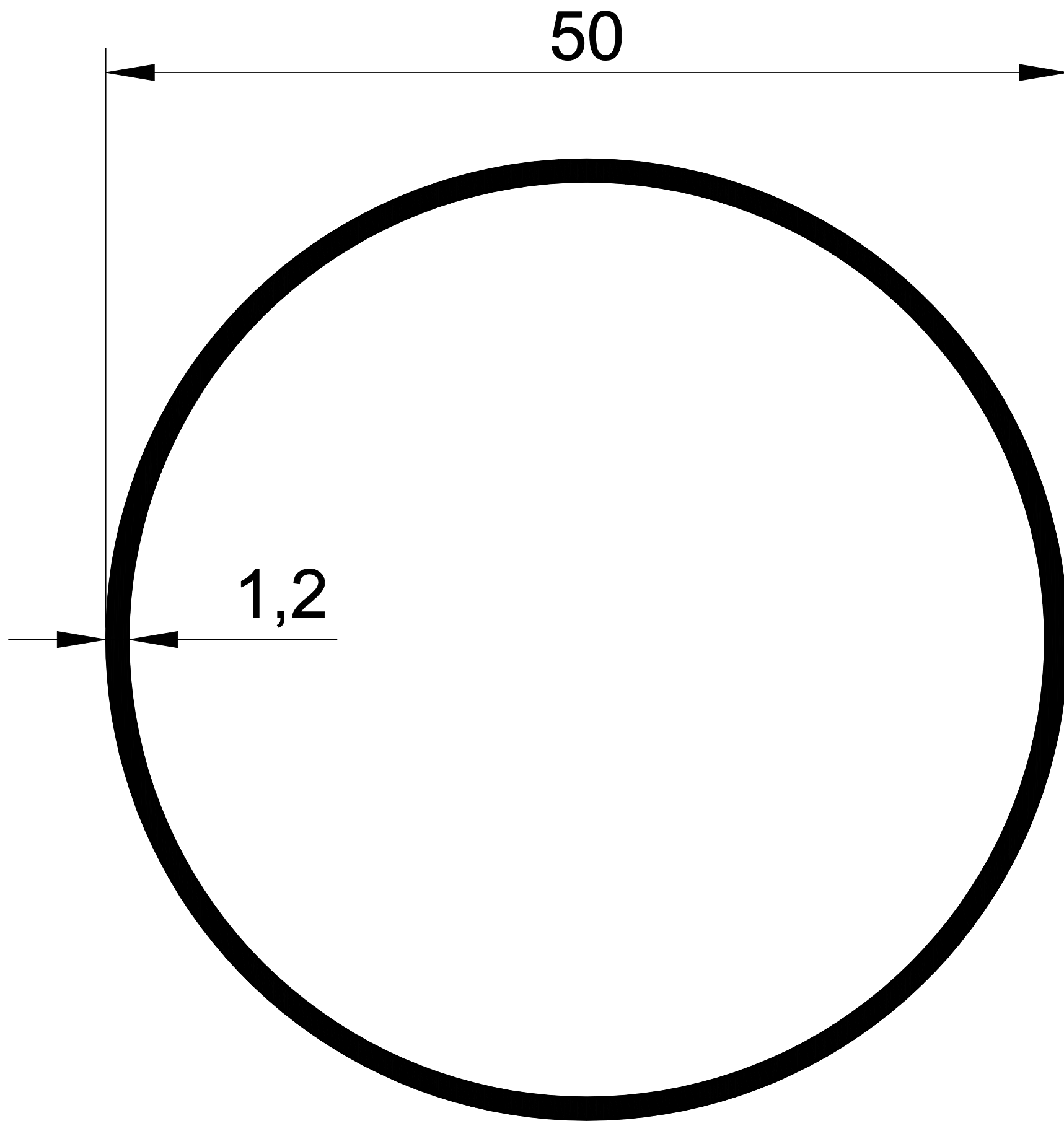
EKOL 1344 0,493 gr/m.
