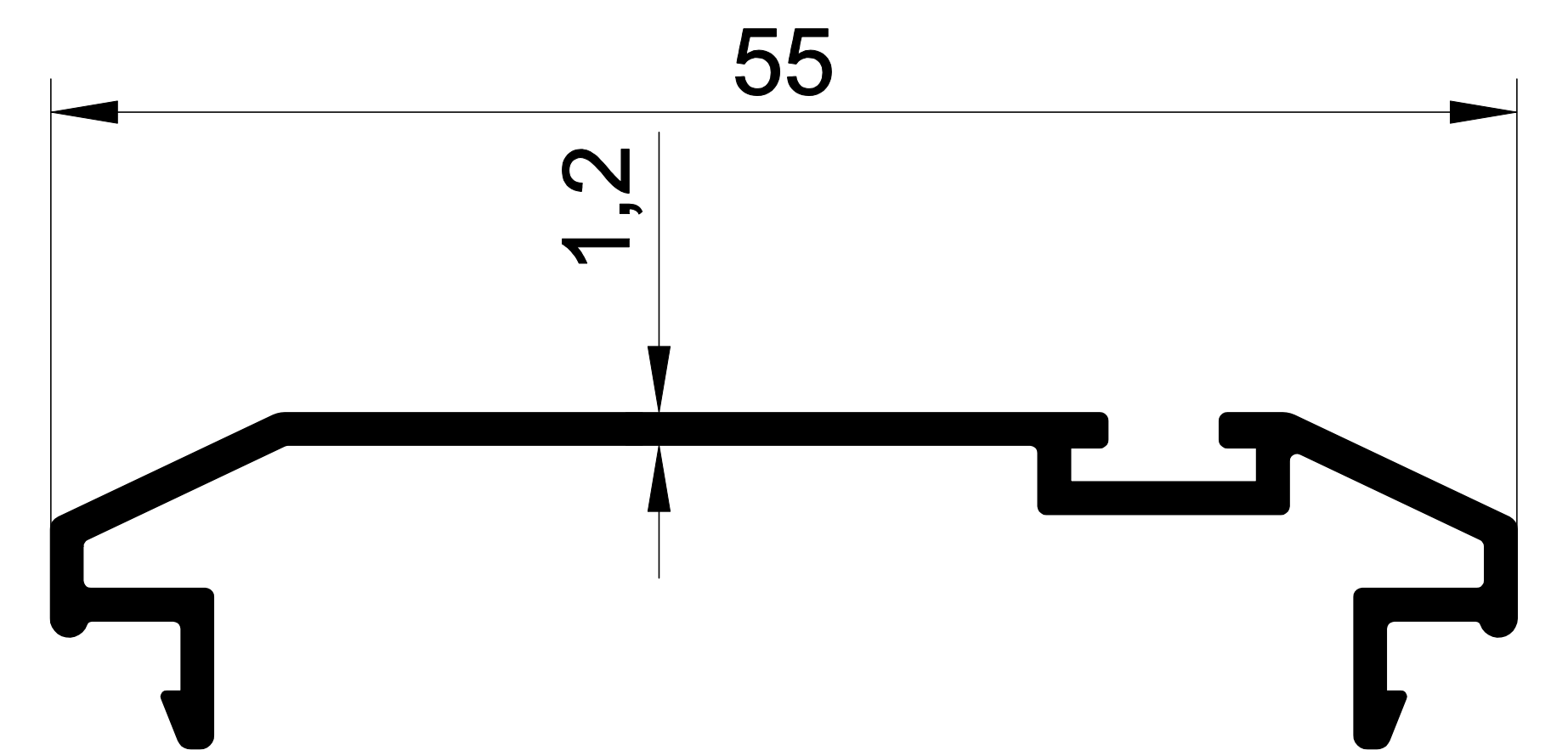
EKOL 1461 0,300 gr/m. SİSTEM ÇARPMA KAPI ADAPTÖRÜ
