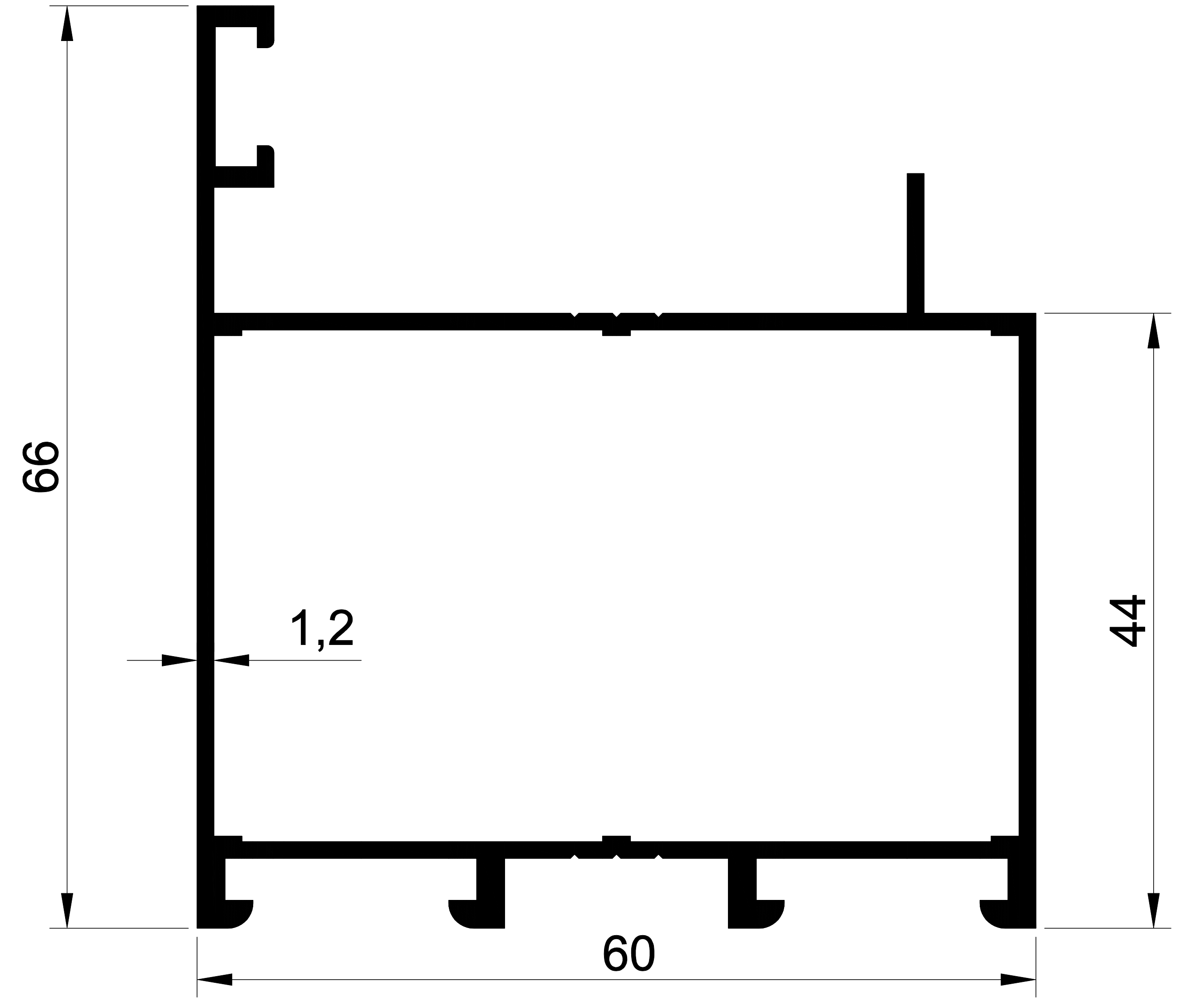
EKOL 1088 0,935 gr/m. 1.2 MM C-60 KANAT
