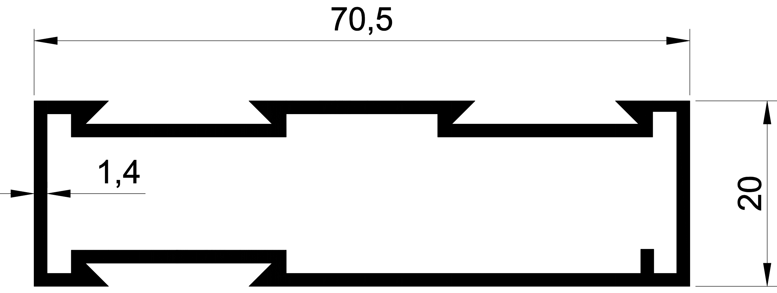
EKOL 1197 0,786 gr/m. DAR TUBA KASA
