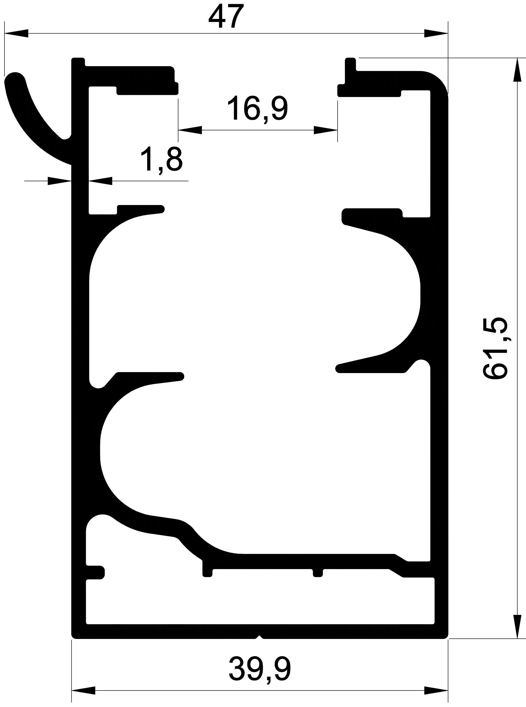
EKOL 1359 1,416 gr/m. ISI YALITIM DAMLALIKLI KASA
