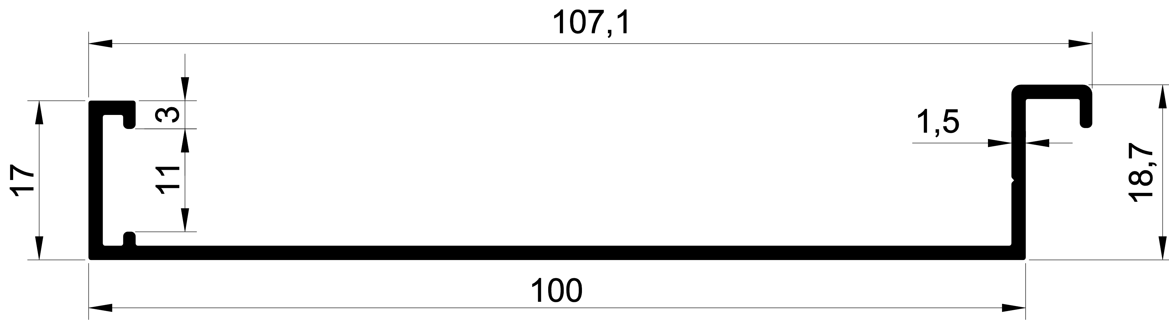
EKOL 1426 0,602 gr/m. MS-PEERVAZ UZATMA PROFİLİ
