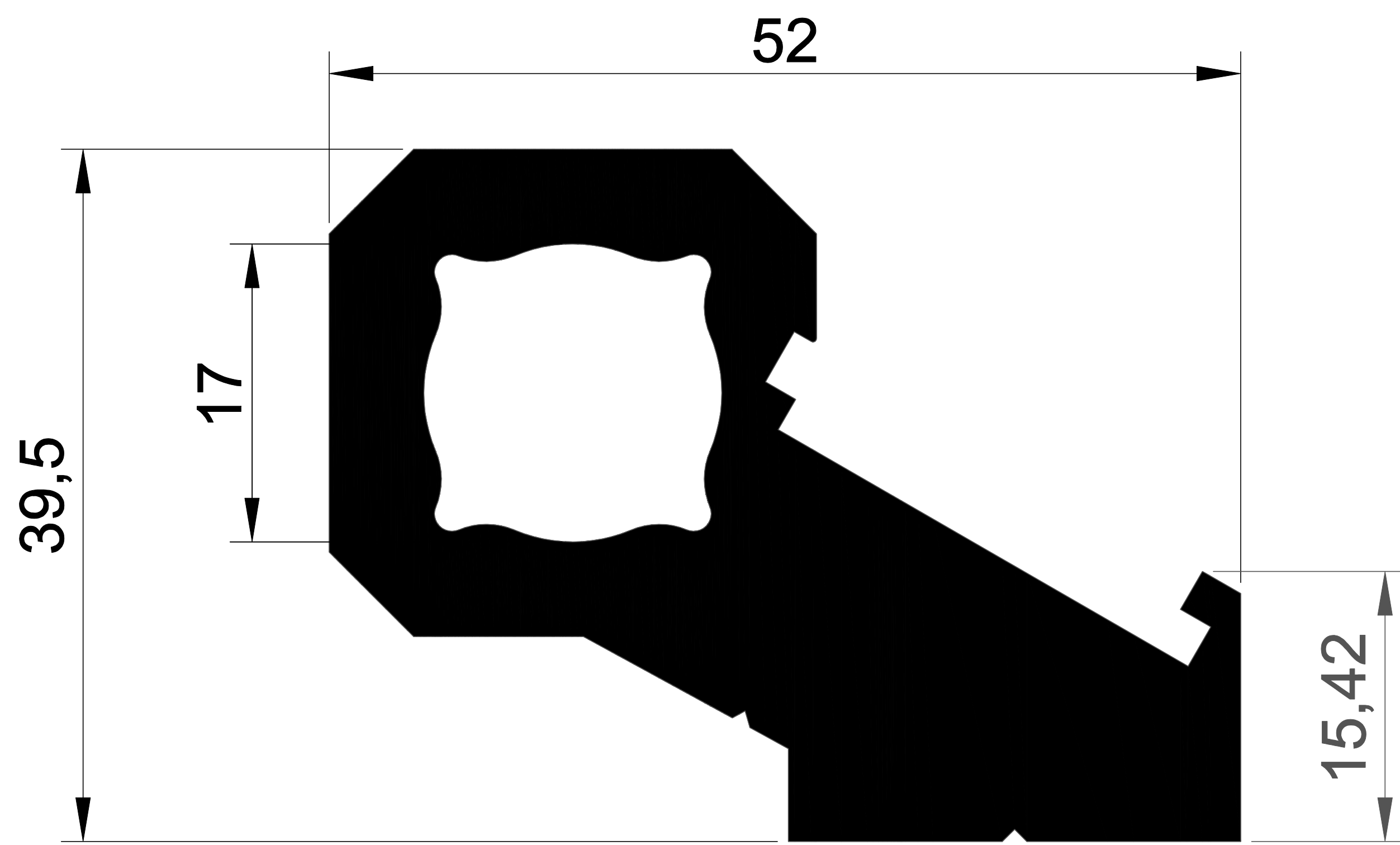
EKOL 1236 2,480 gr/m.
