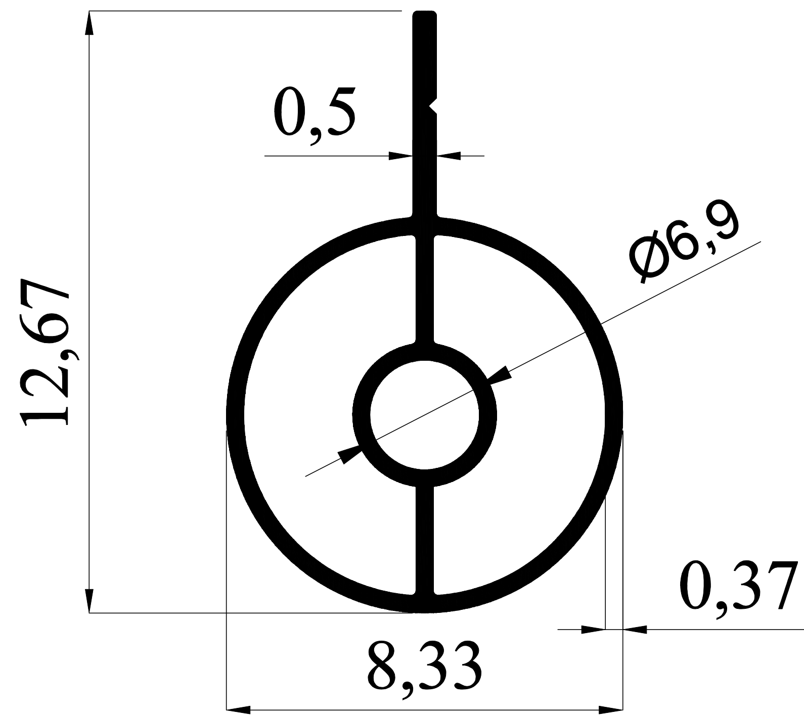
EKOL 1417 0,392 gr/m.
