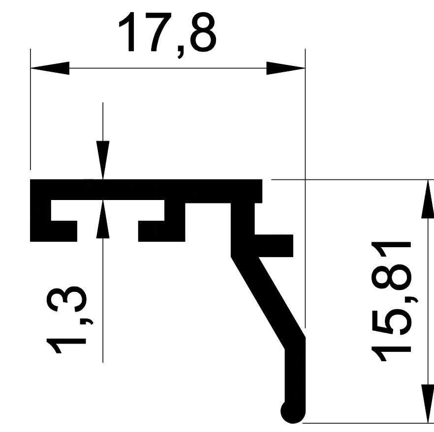
EKOL 1192 0,154 gr/m ISI CAM ÇITASI
