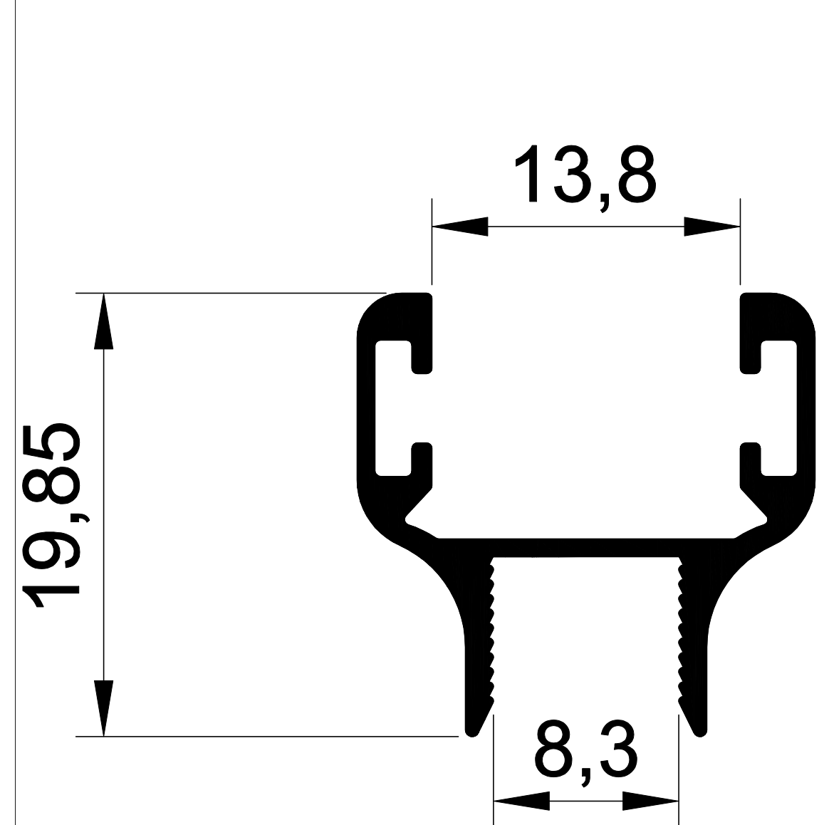
EKOL 1150 1,008 gr/m. CAM BALKON ETEK
