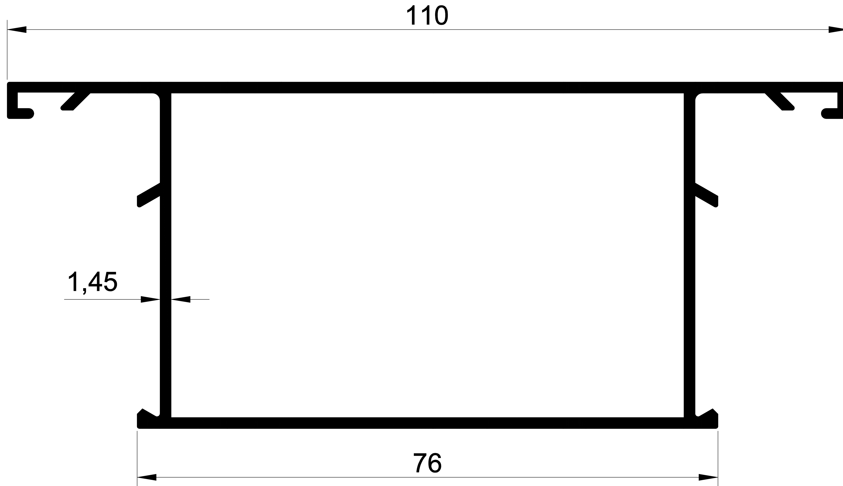
EKOL 1111 1,162 gr/m. ALDOKS BAZA ORTA
