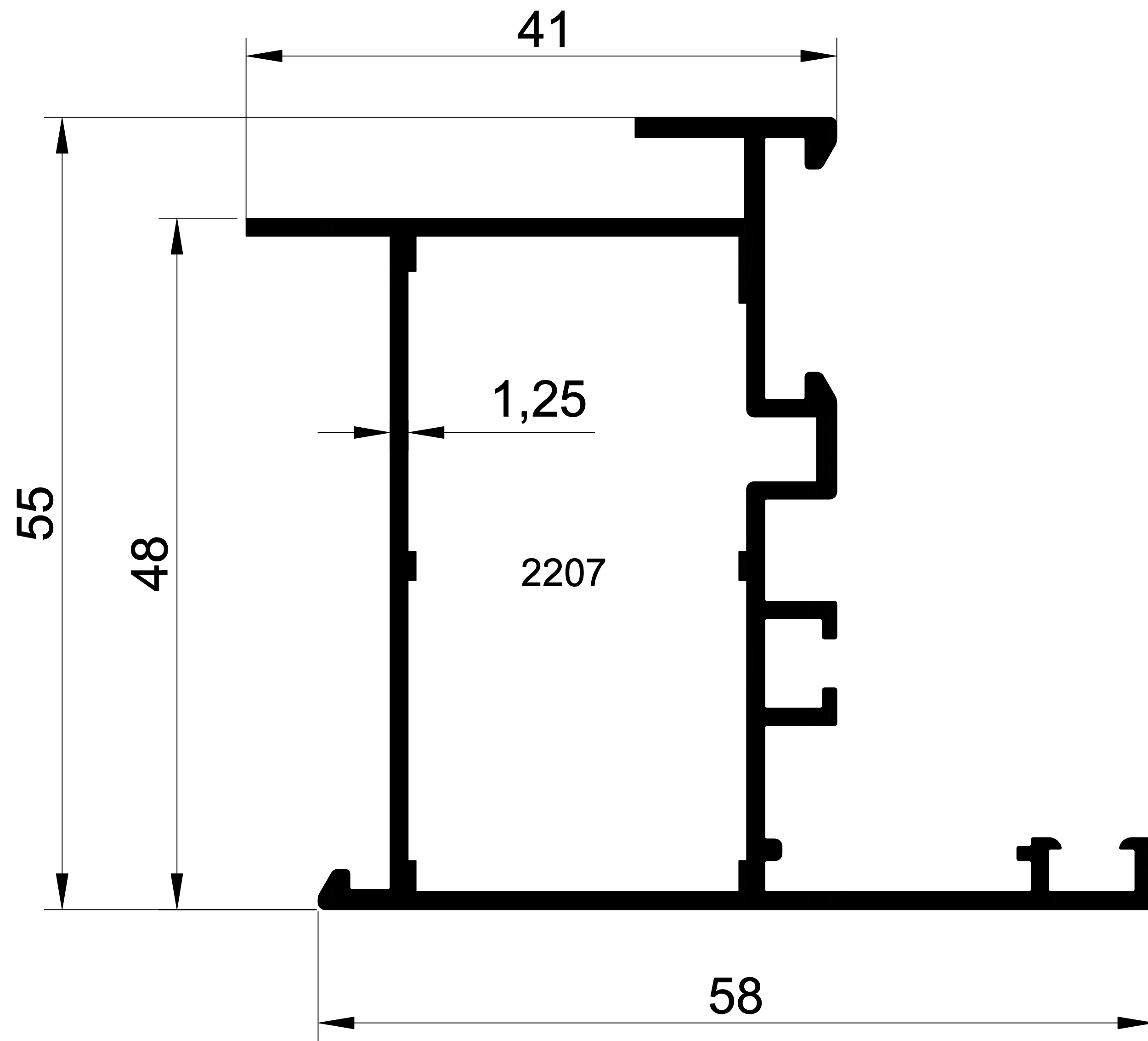
EK-55- 2207 0,860 gr/m SİSTEM 55 TERS KAPI ADAPTÖRÜ
