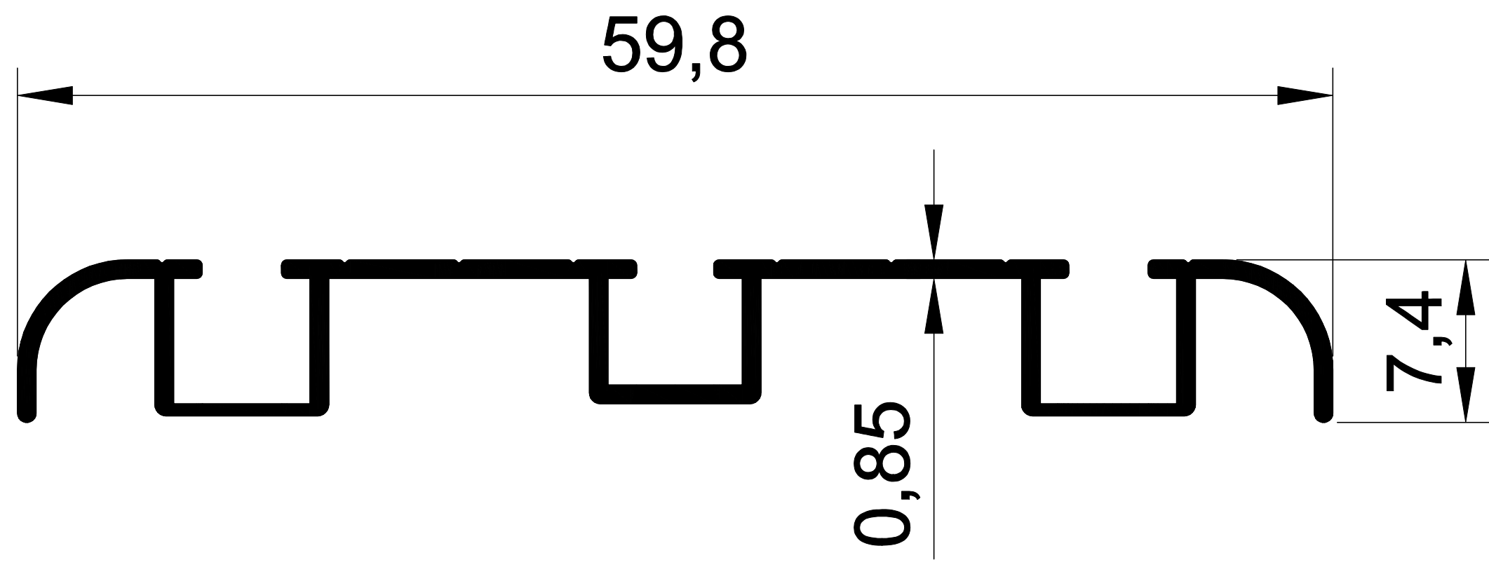
EKOL 1311 0,249 gr/m. 3'LÜ SÜRME EŞİKSİZ RAY
