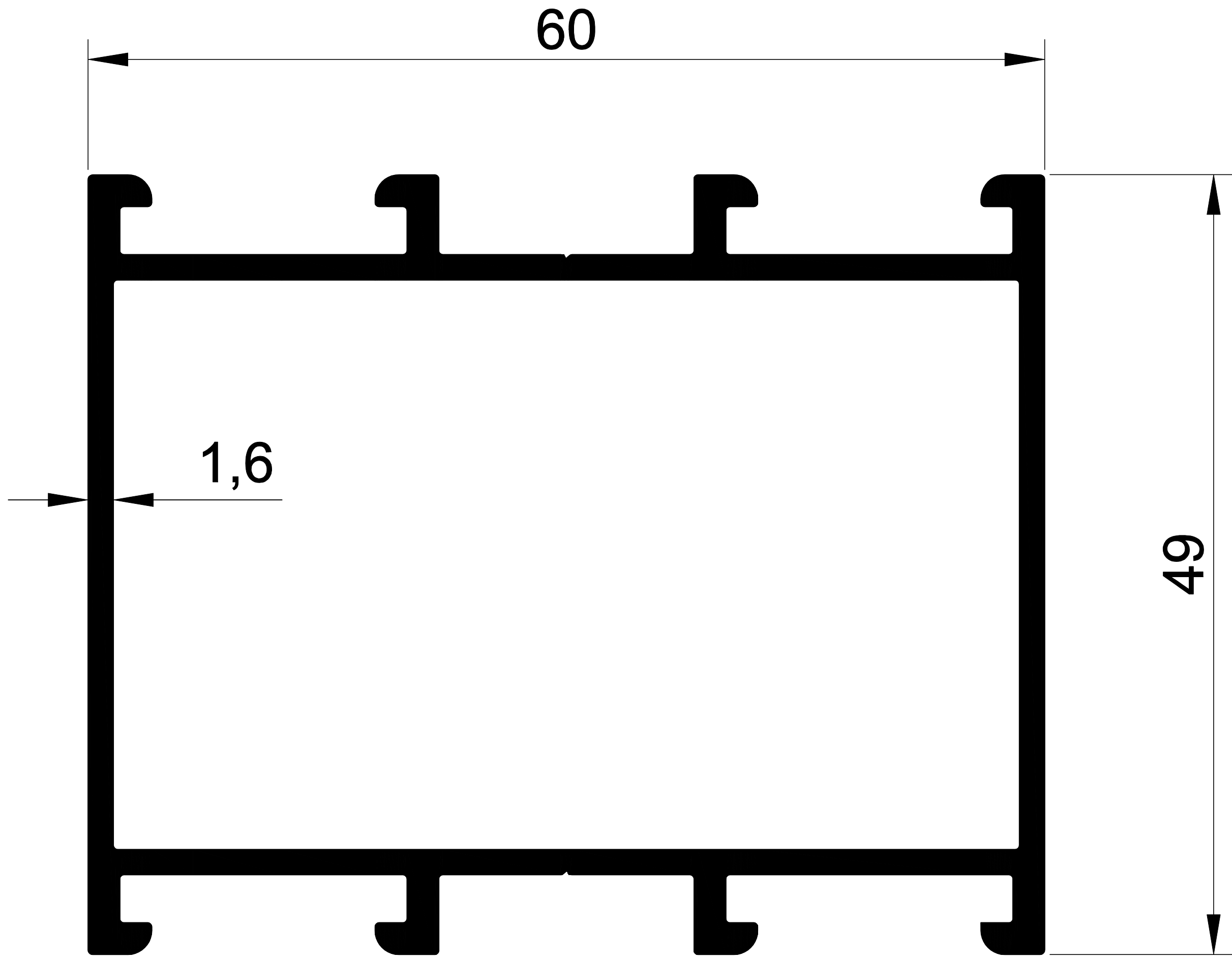
EKOL 1407 1,123 gr/m. 1.6 MM C-60 KASA
