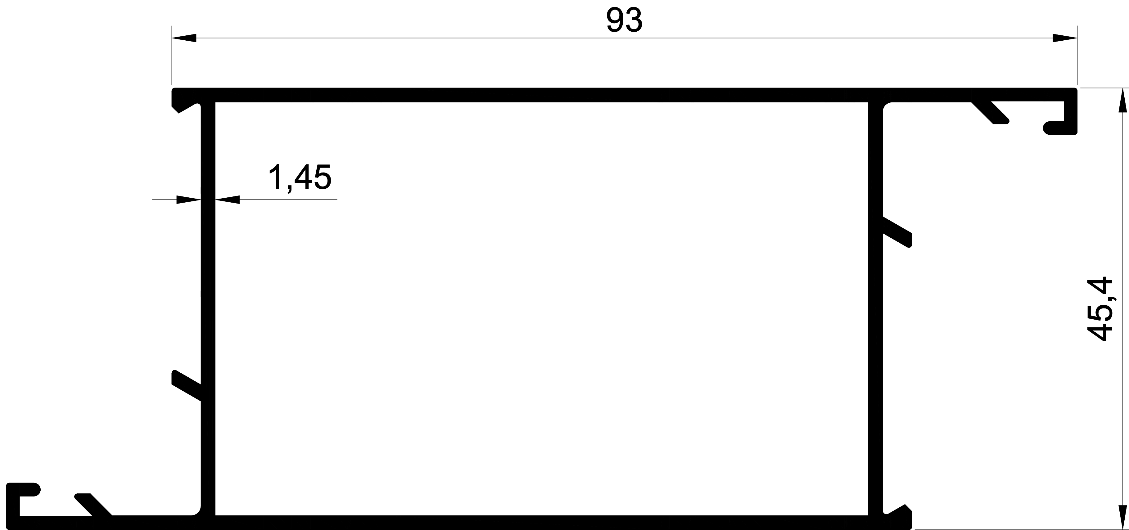
EKOL 1109 1,162 gr/m. ALDOKS BAZA KAPI
