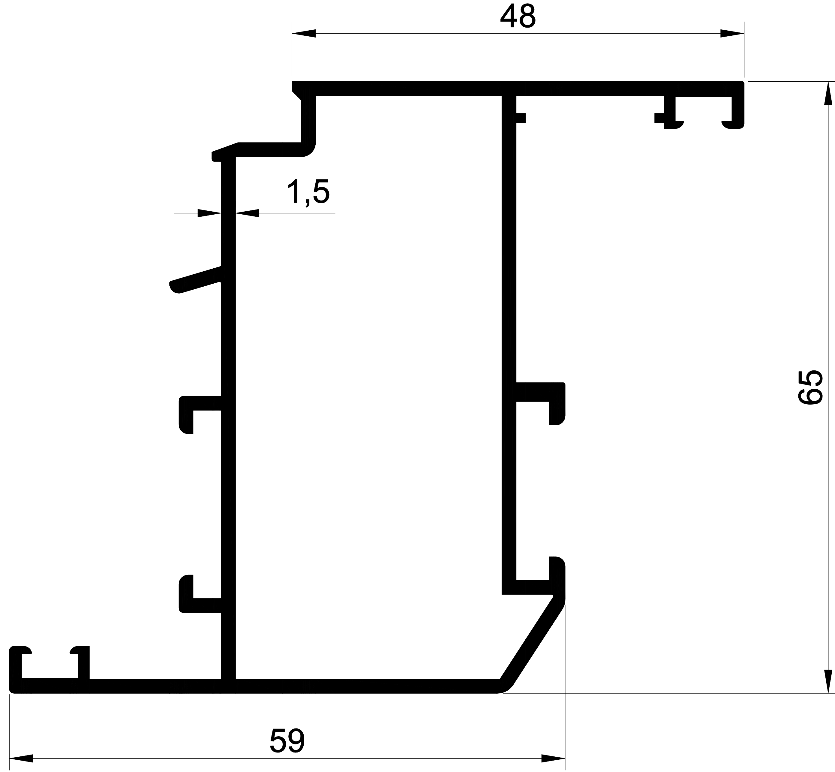
EKOL 1201 1,168 gr/m. SİSTEM KANAT
