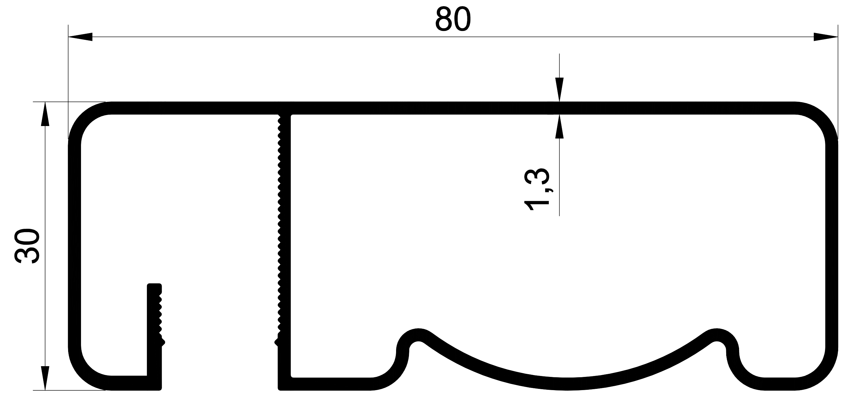
EKOL 1133 0,852 gr/m. 30X80 YANDAN CAMLI
