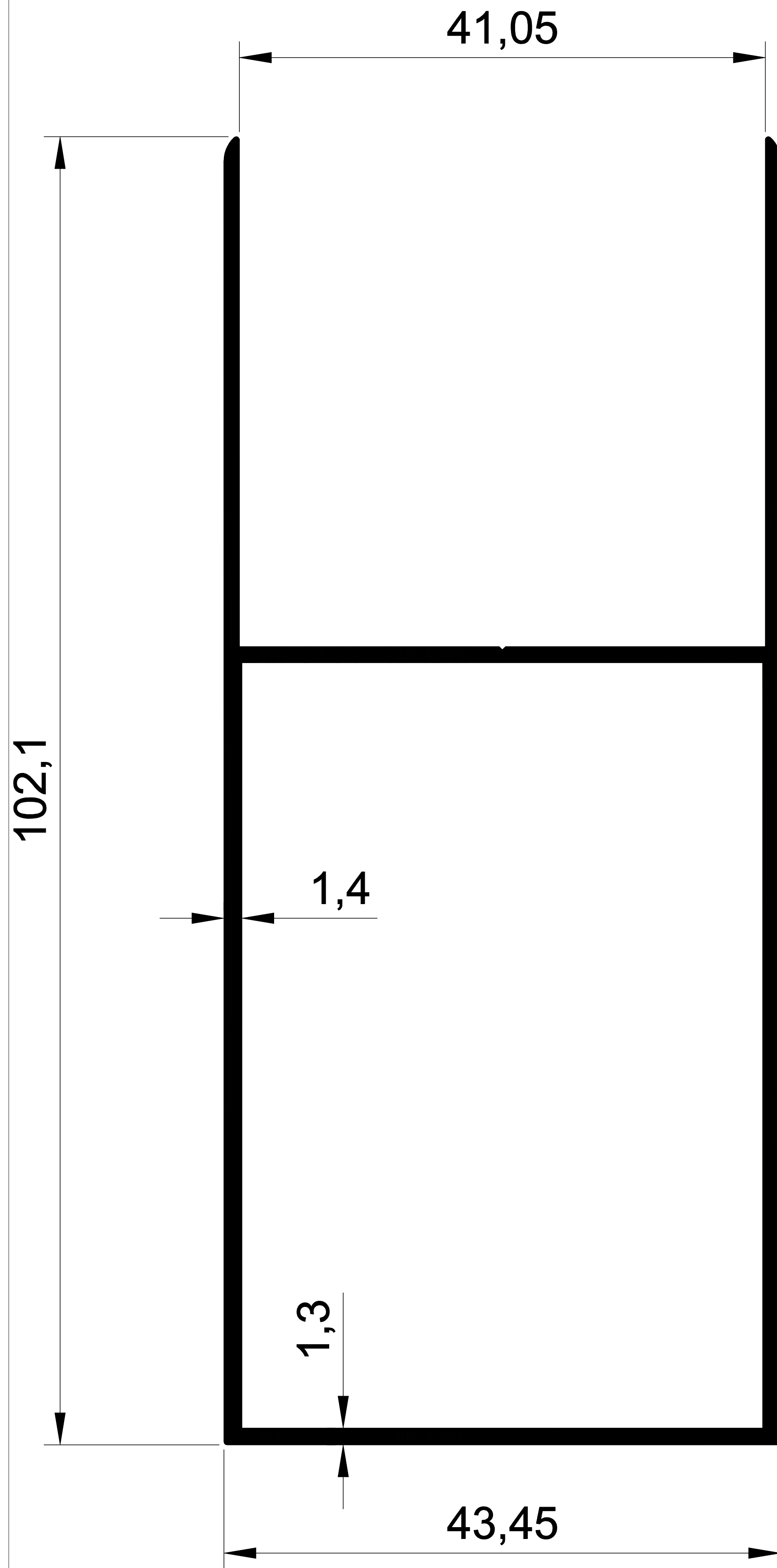
EKOL 1150 1,008 gr/m. CAM BALKON ETEK
