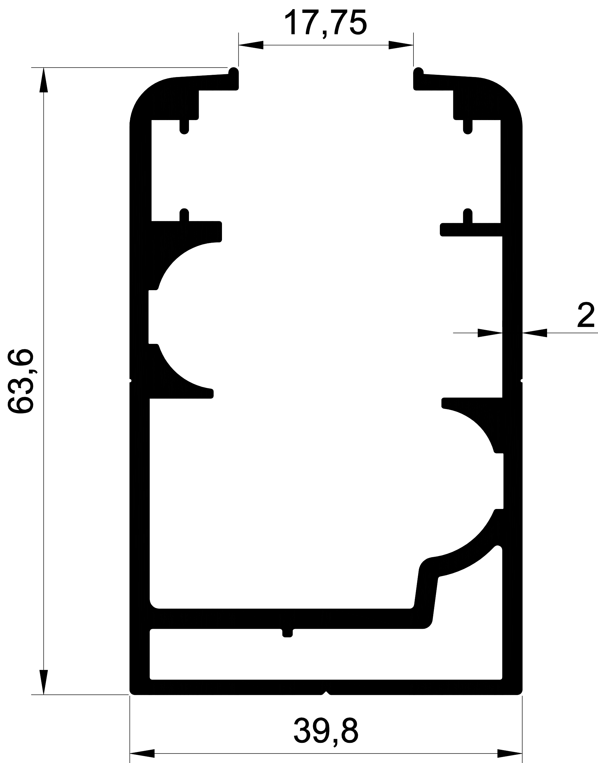
EKOL 1250 1,387 gr/m. GOLD KASA
