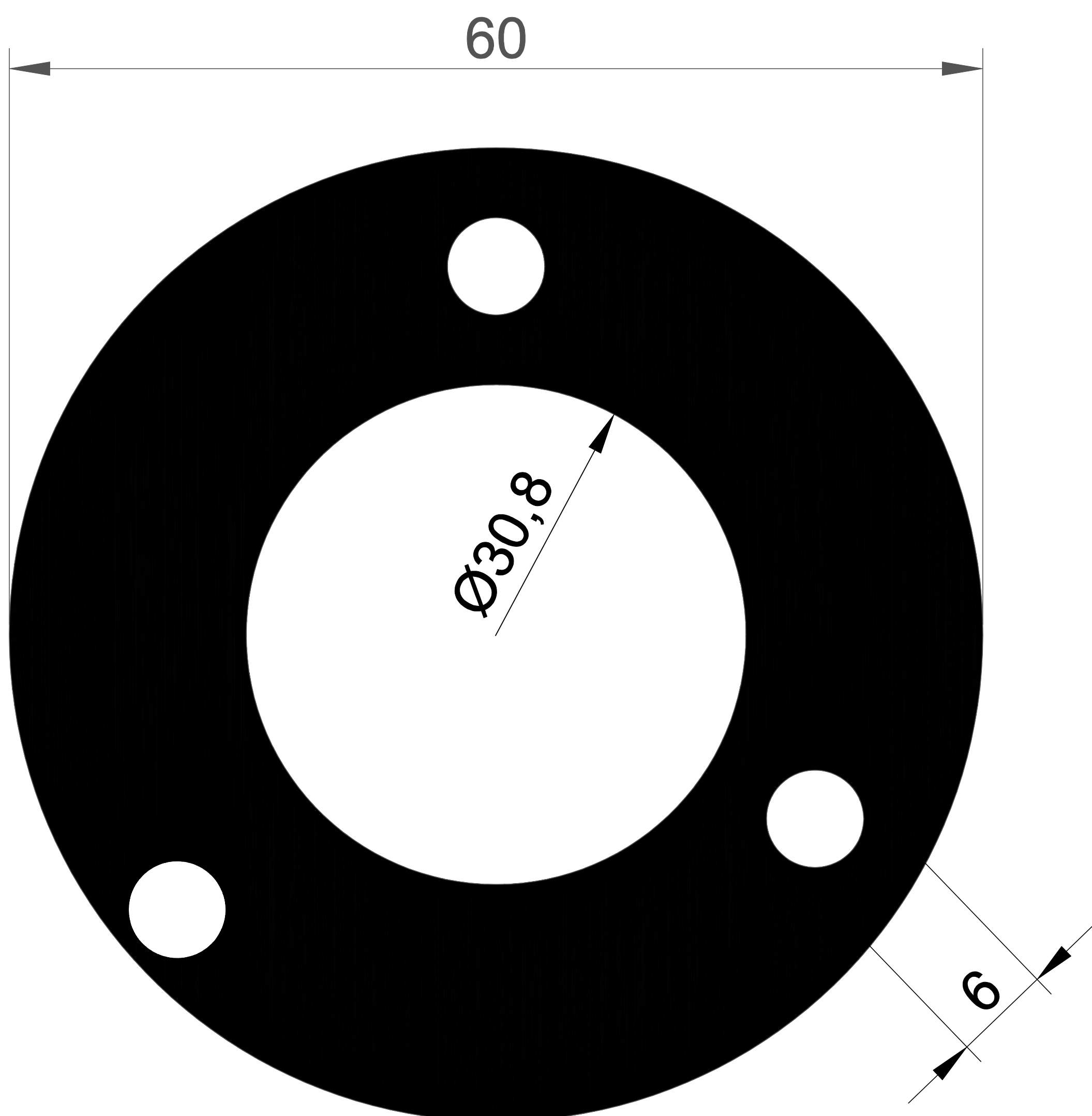
EKOL 1175 5,414 gr/m.
