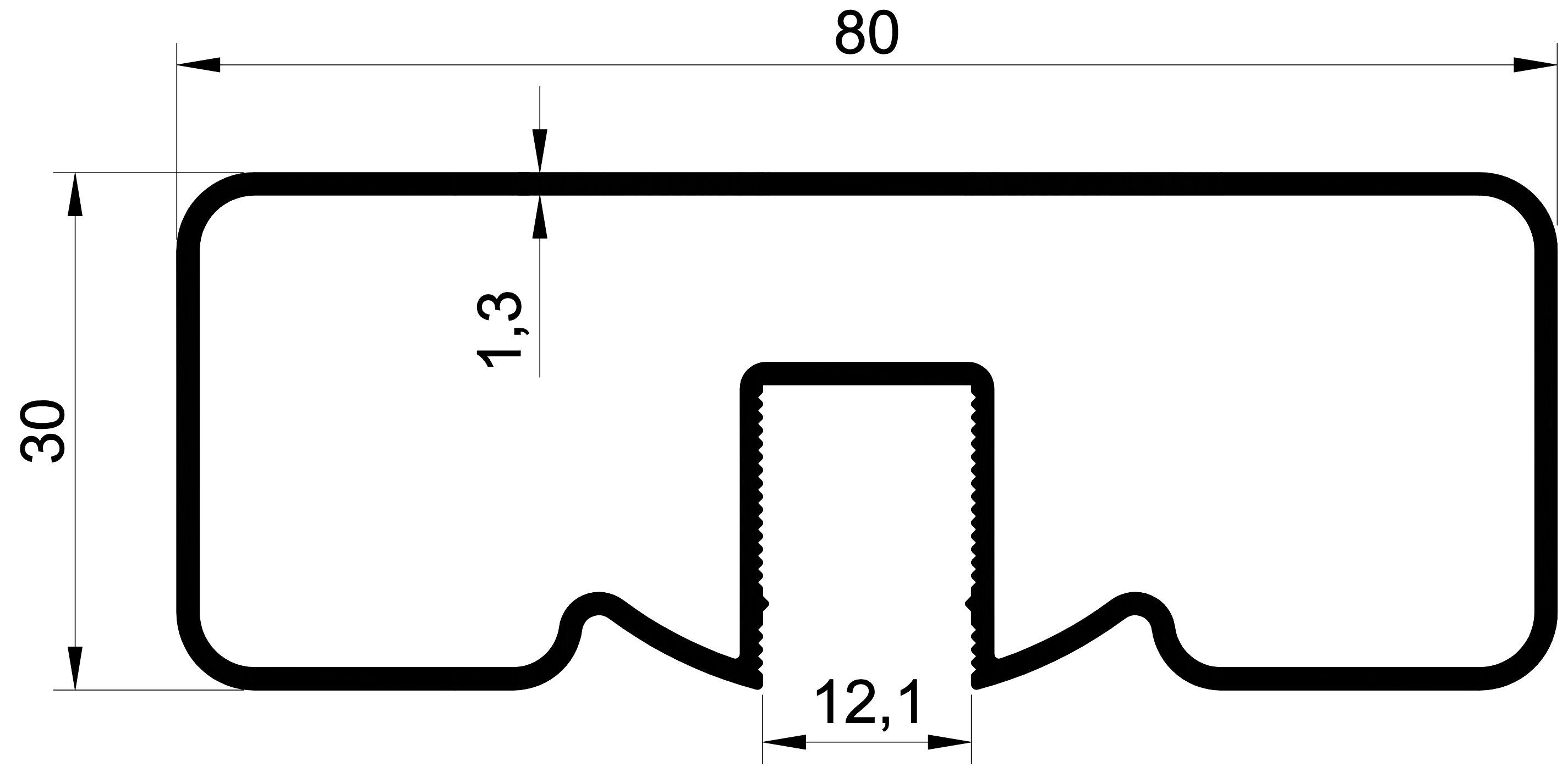
EKOL 1130 0,870 gr/m. 30X80 ORTADAN CAMLI
