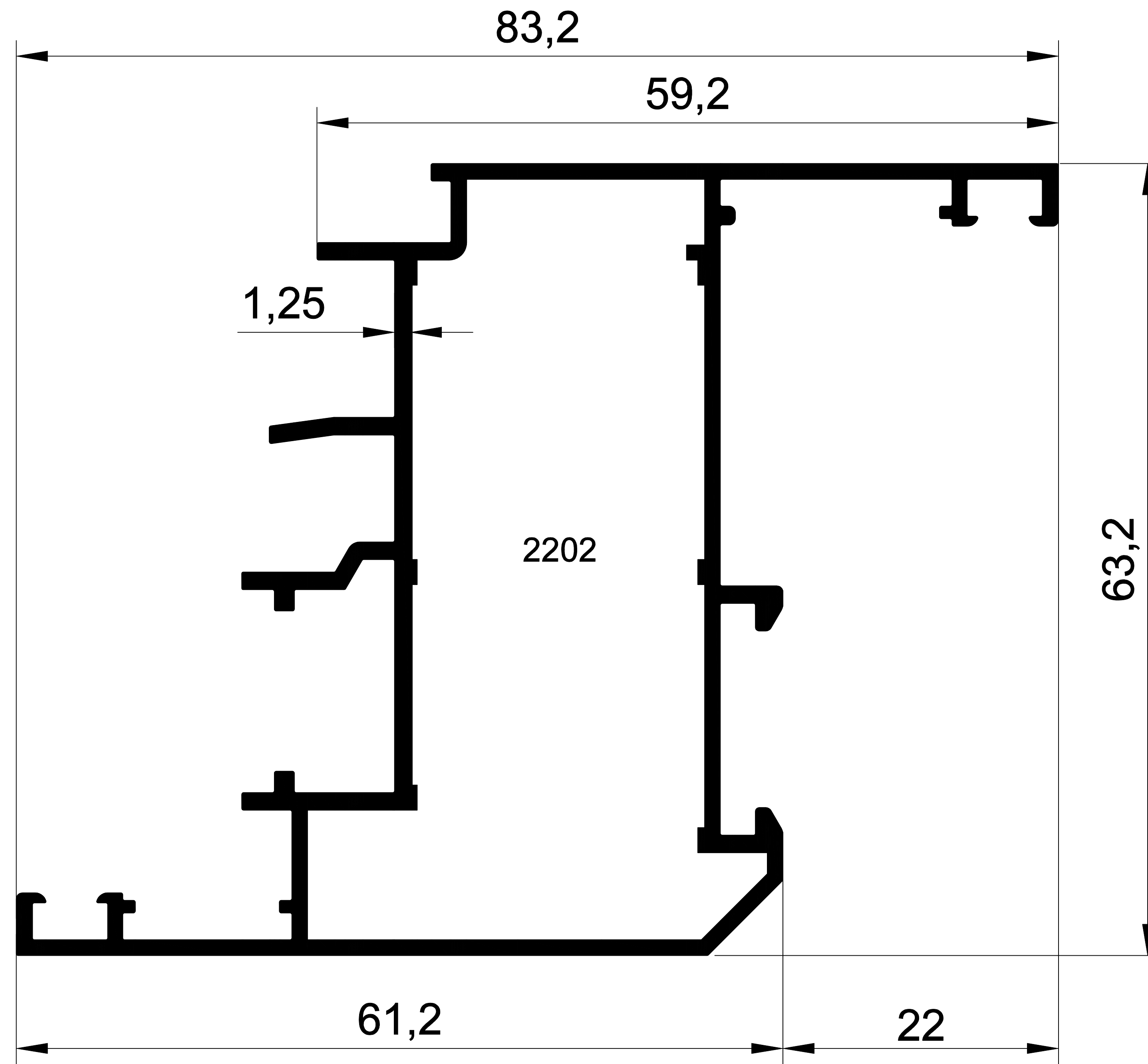
EK-55- 2202 1,135 gr/m SİSTEM 55 YALITIMSIZ KANAT
