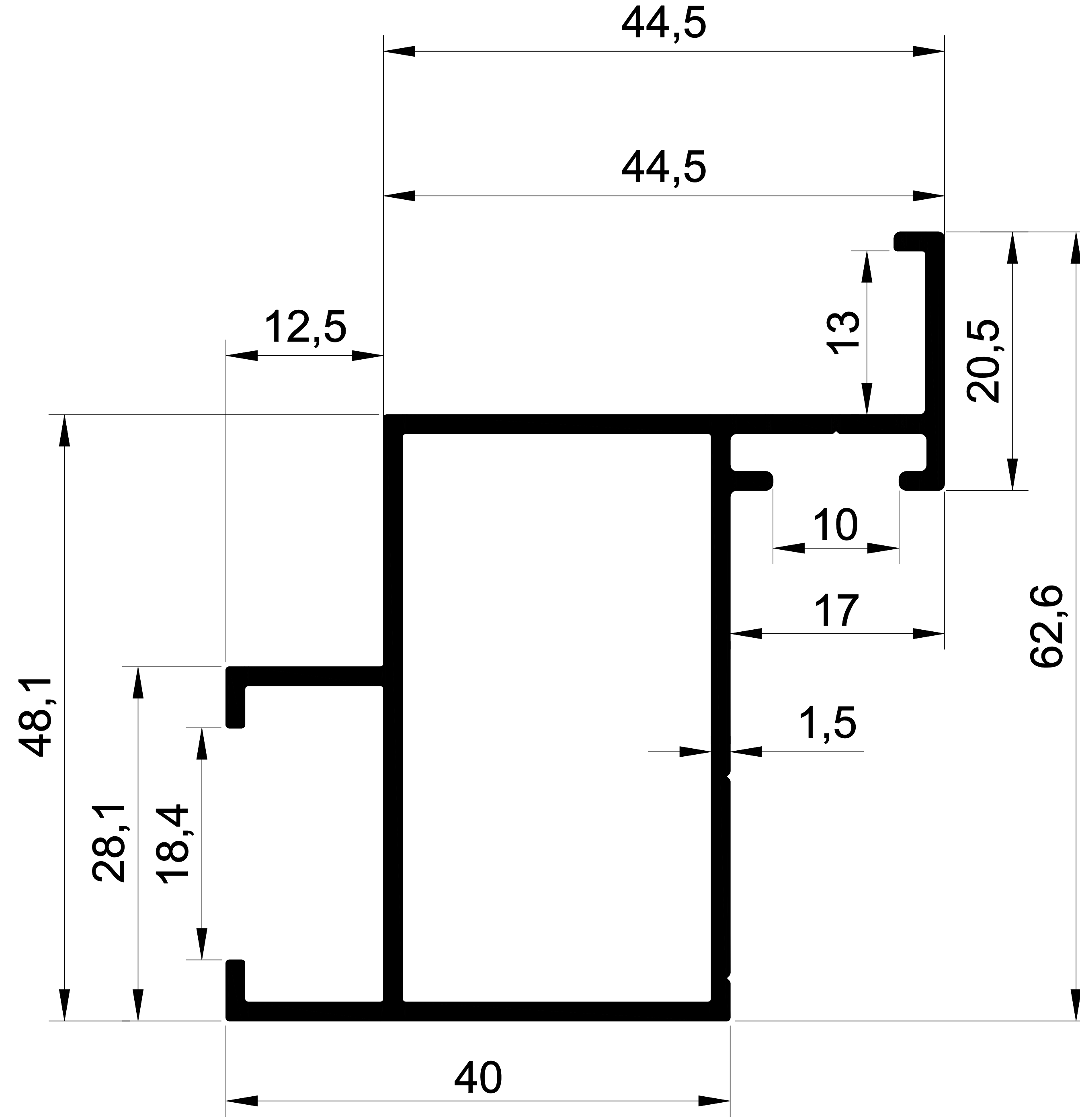
EKOL 1418 0,897 gr/m. MS-AHŞAP GİZLİ KAPI KASASI
