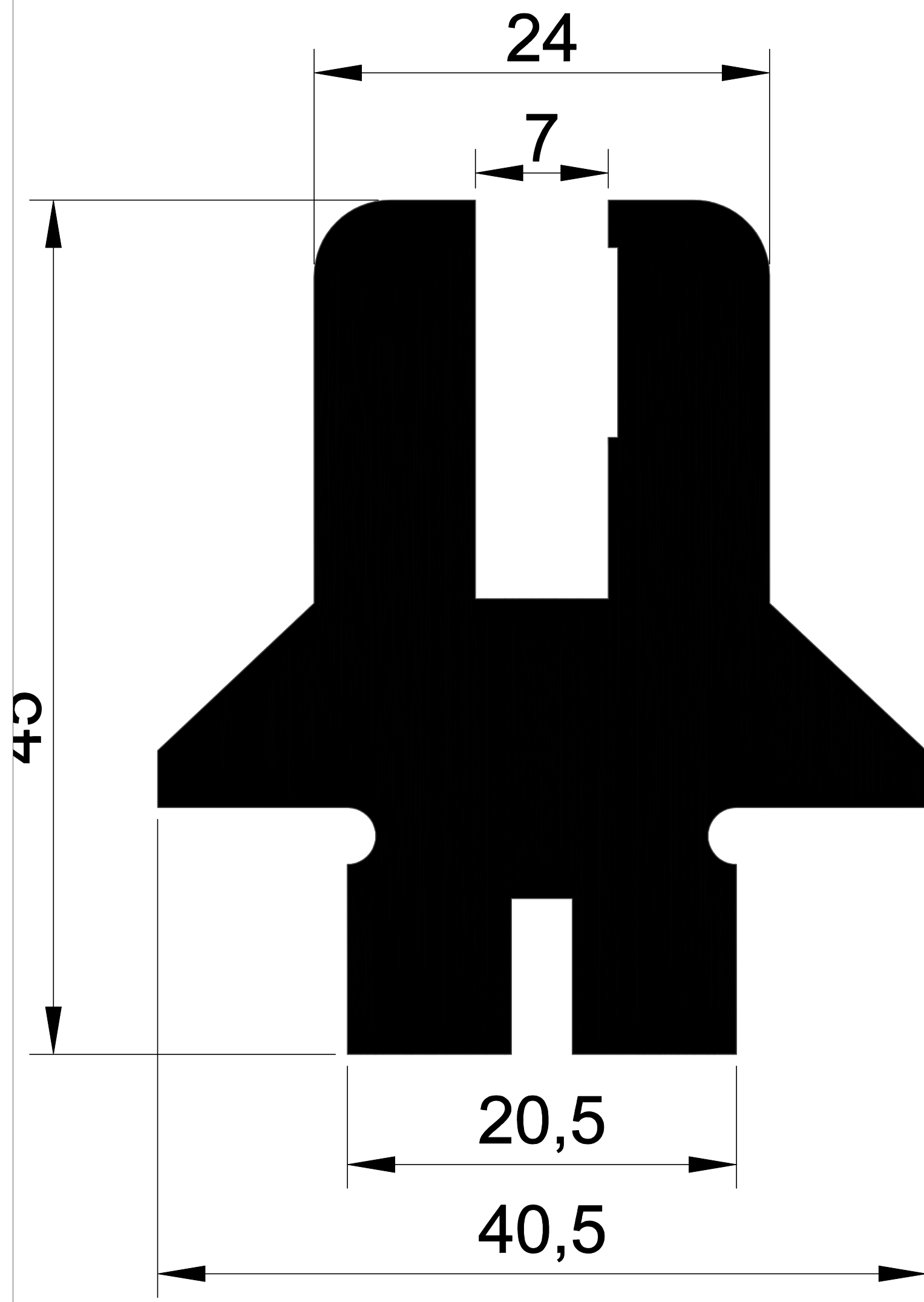
EKOL 1015 2,588 gr/m.
