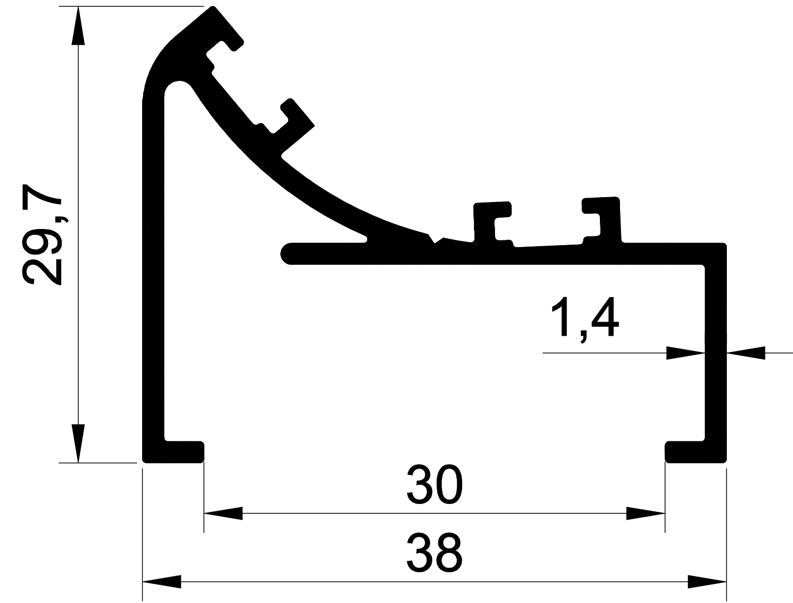
EKOL 1364 0,430 gr/m. ISI YALITIM EKSENAL KÖŞE DÖNÜŞ
