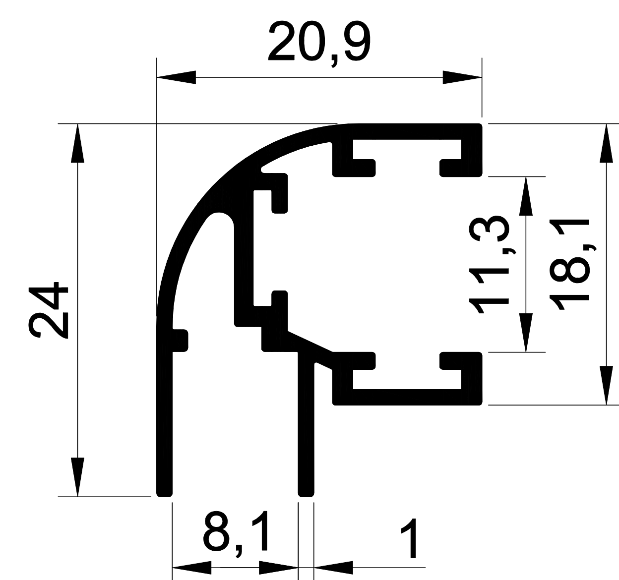
EKOL 1300 0,282 gr/m. CAM H
