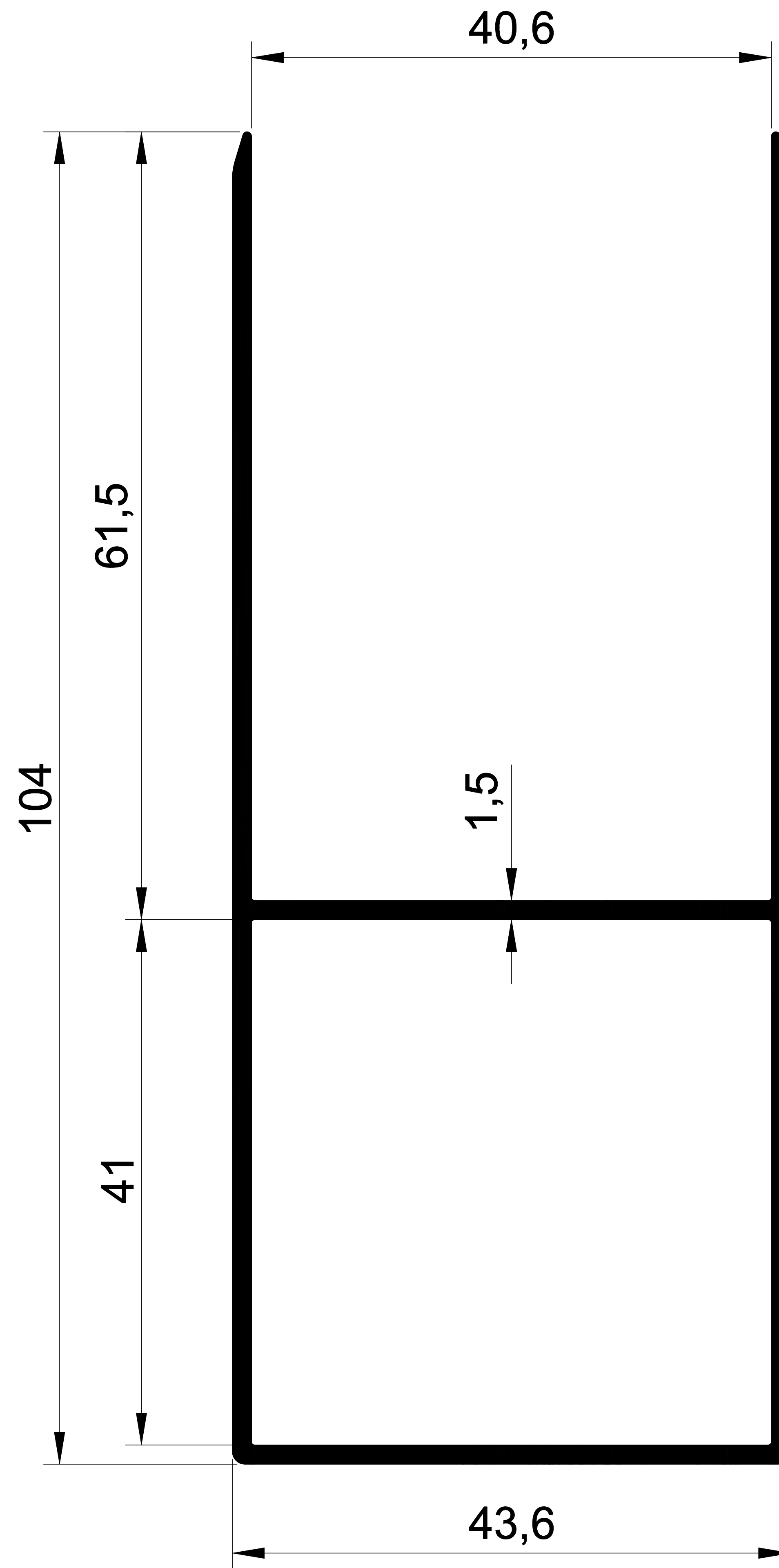
EKOL 1252 1,168 gr/m. CAM BALKON ETEK
