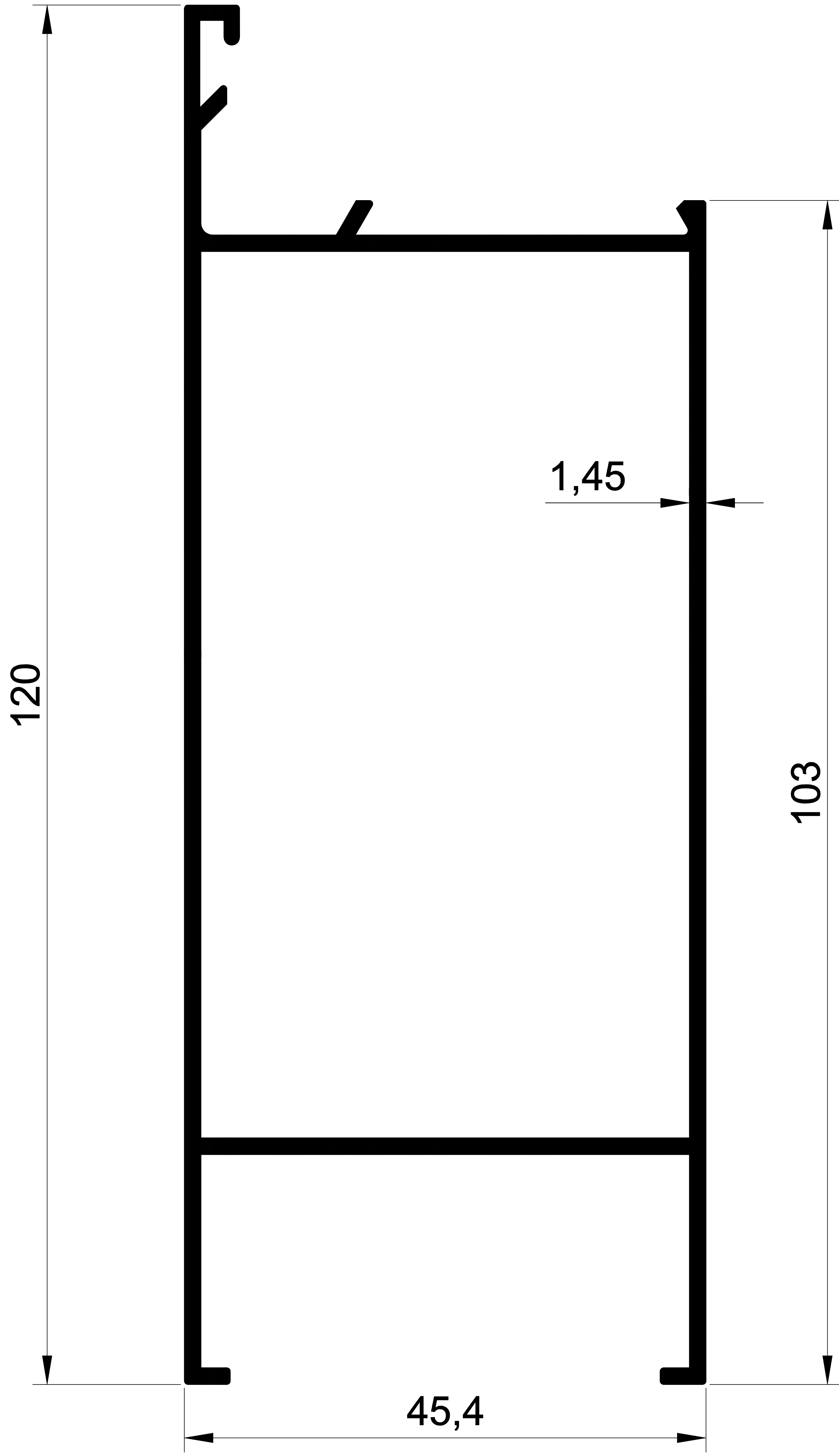
EKOL 1107 1,279 gr/m. ALDOKS ETEK
