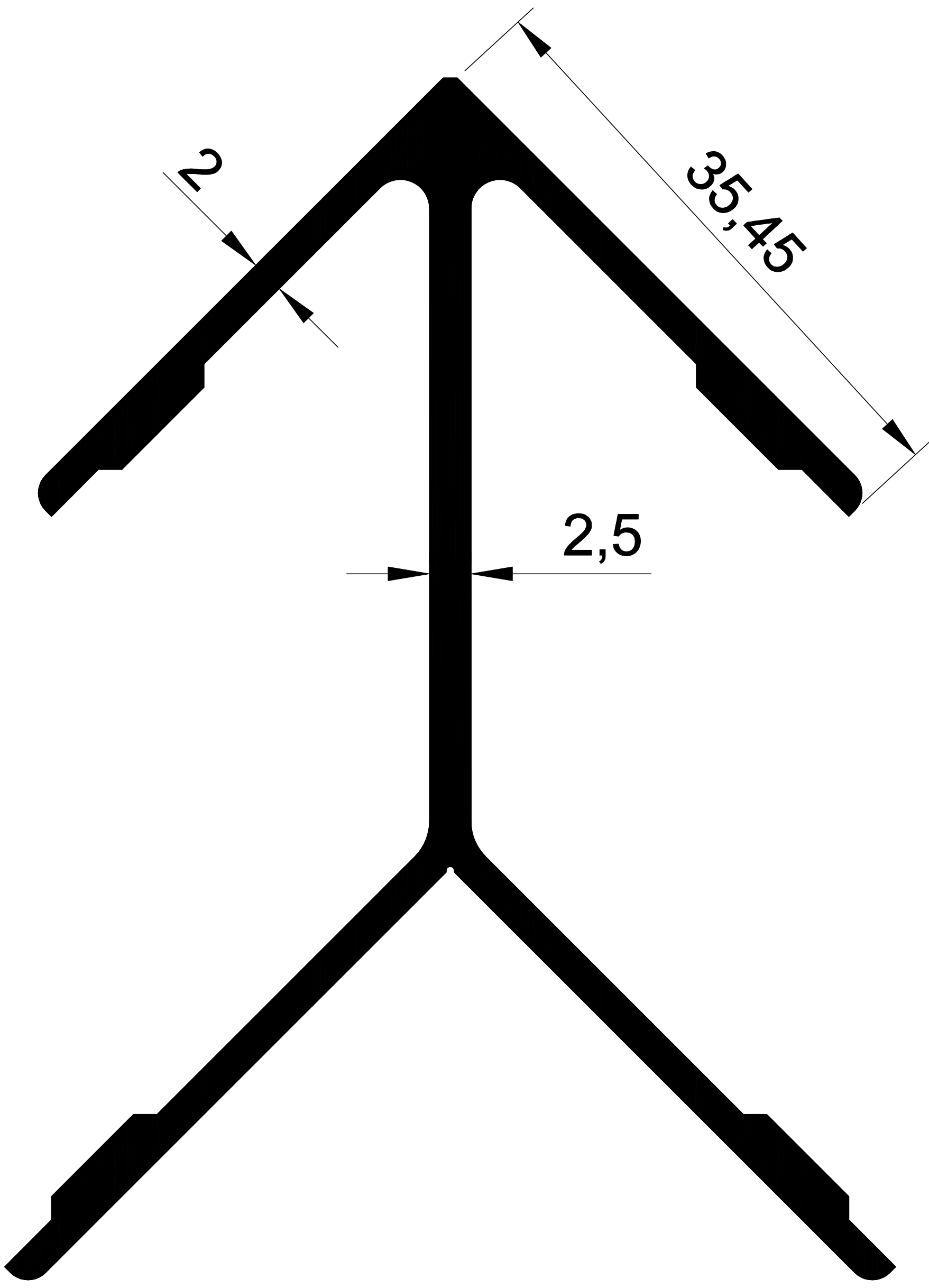
EKOL1094 1,170 gr/m. GENİŞ ÇAVUŞ (KÖŞE BAĞLANTI)
