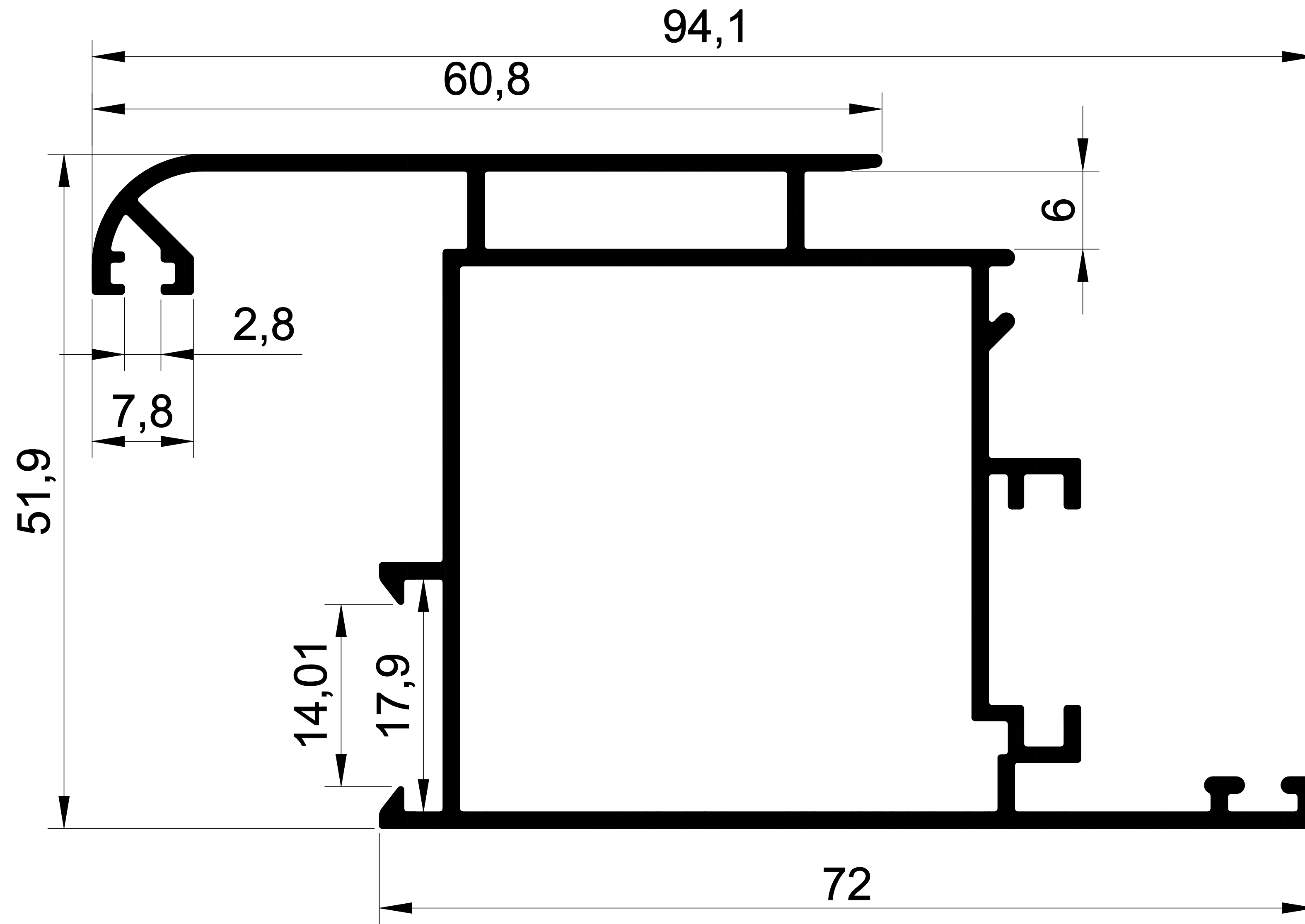
EKOL 1371 1,164 gr/m. OVAL KANAT
