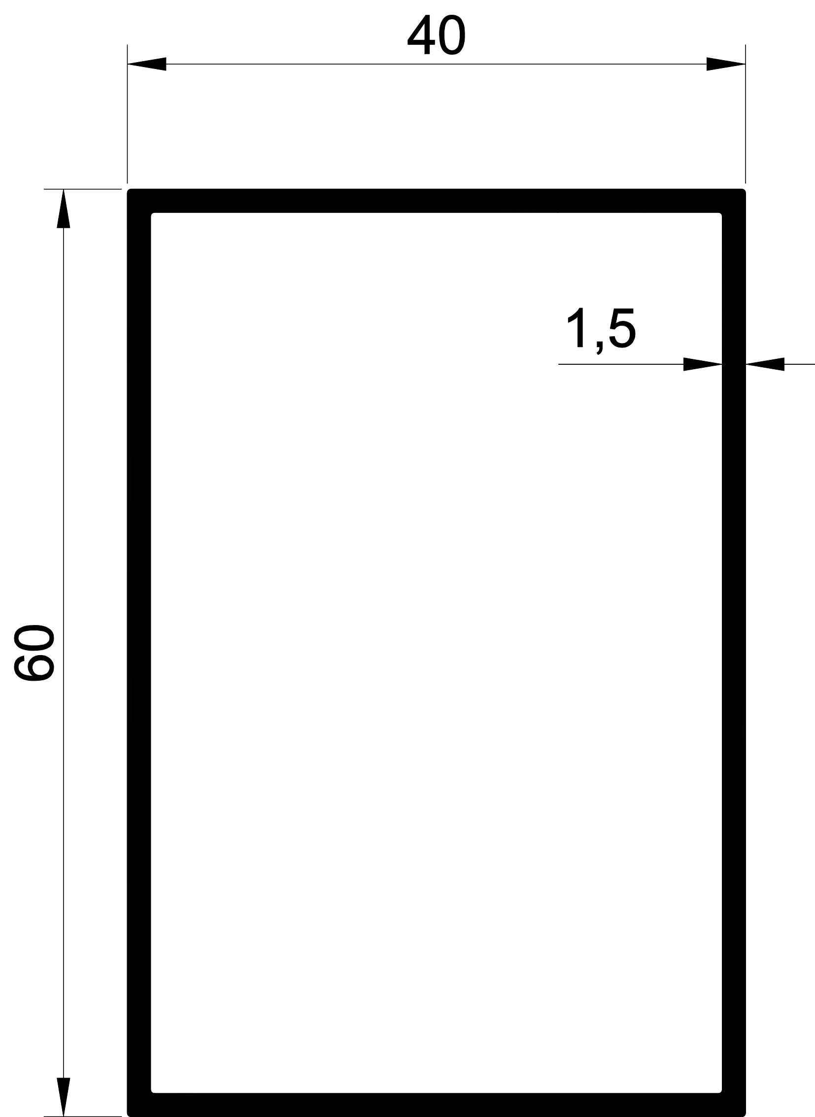
EKOL 1413 0,789 gr/m.
