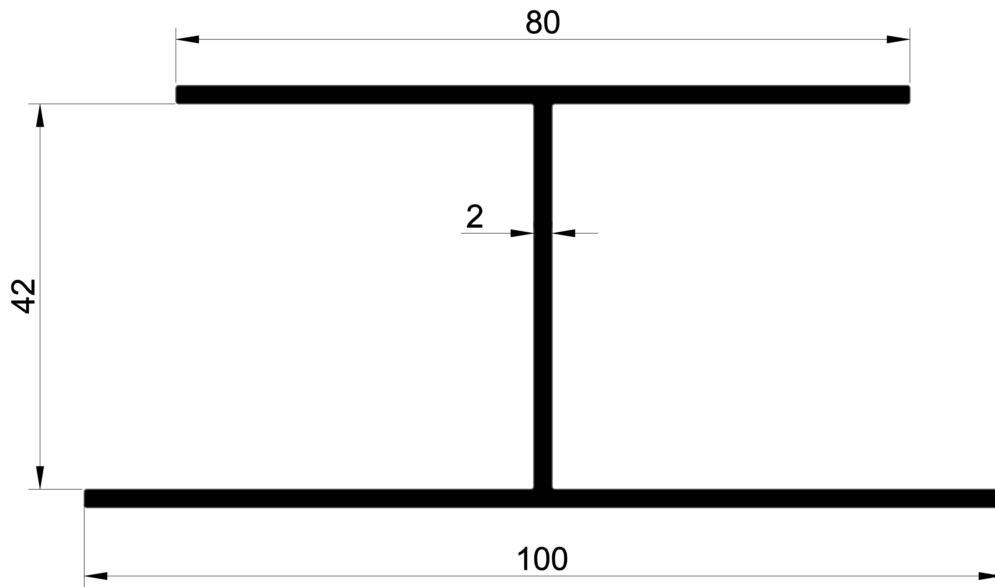
EKOL 1447 1.203 gr/m. PANEL H PROFİLİ
