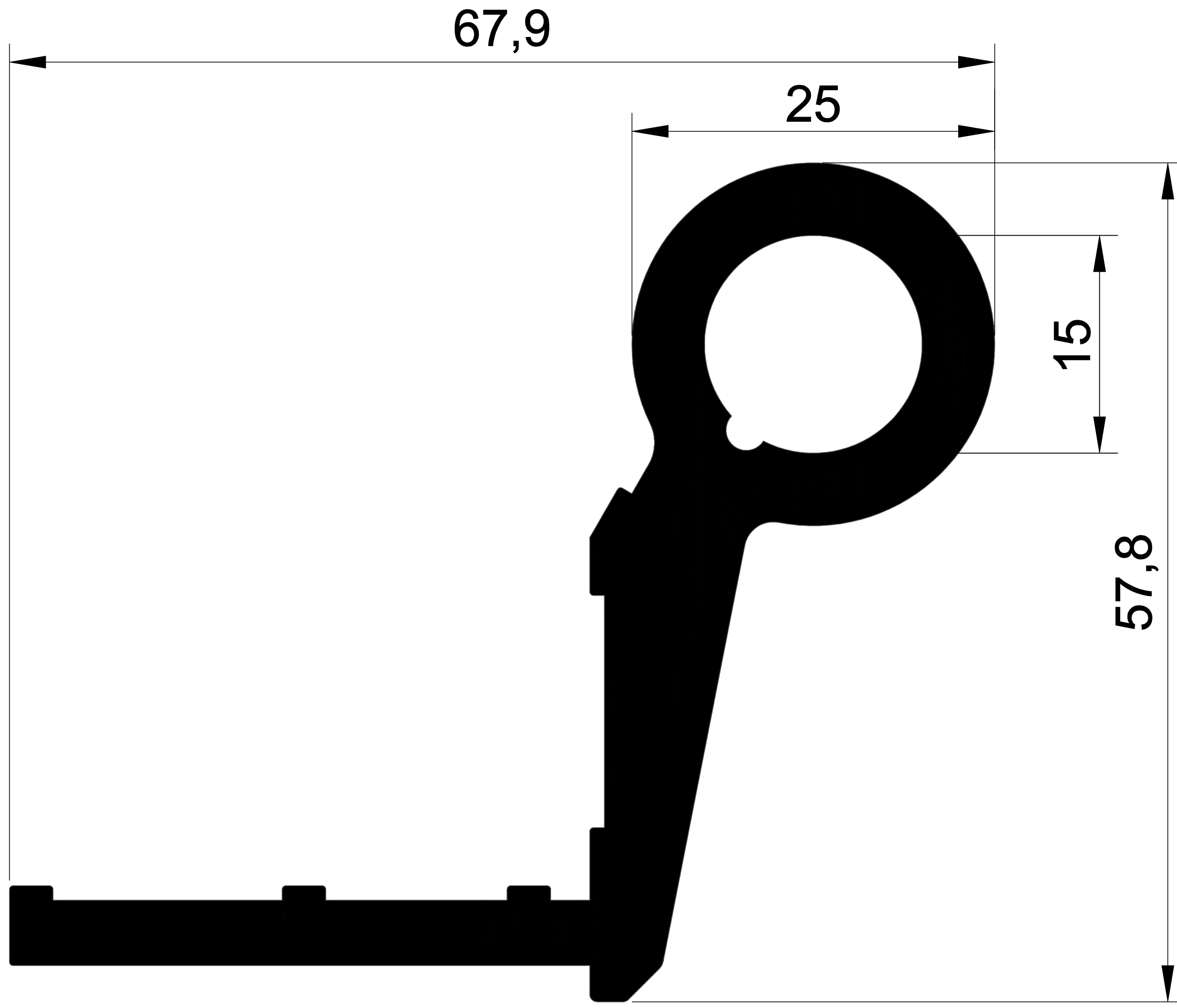
EKOL 1011 2,073 gr/m.
