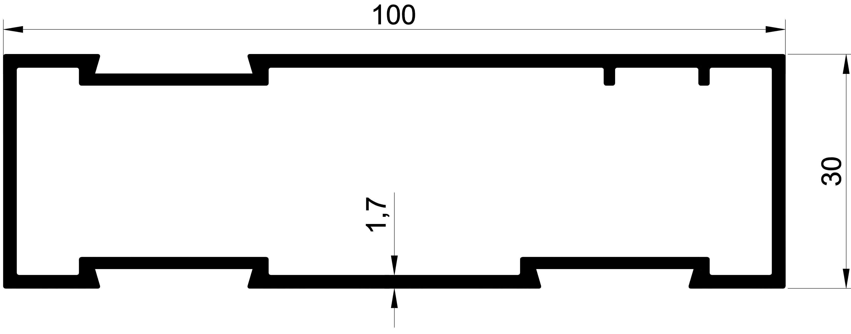
EKOL 1385 1,240 gr/m. 100'LÜK TUBA KASA
