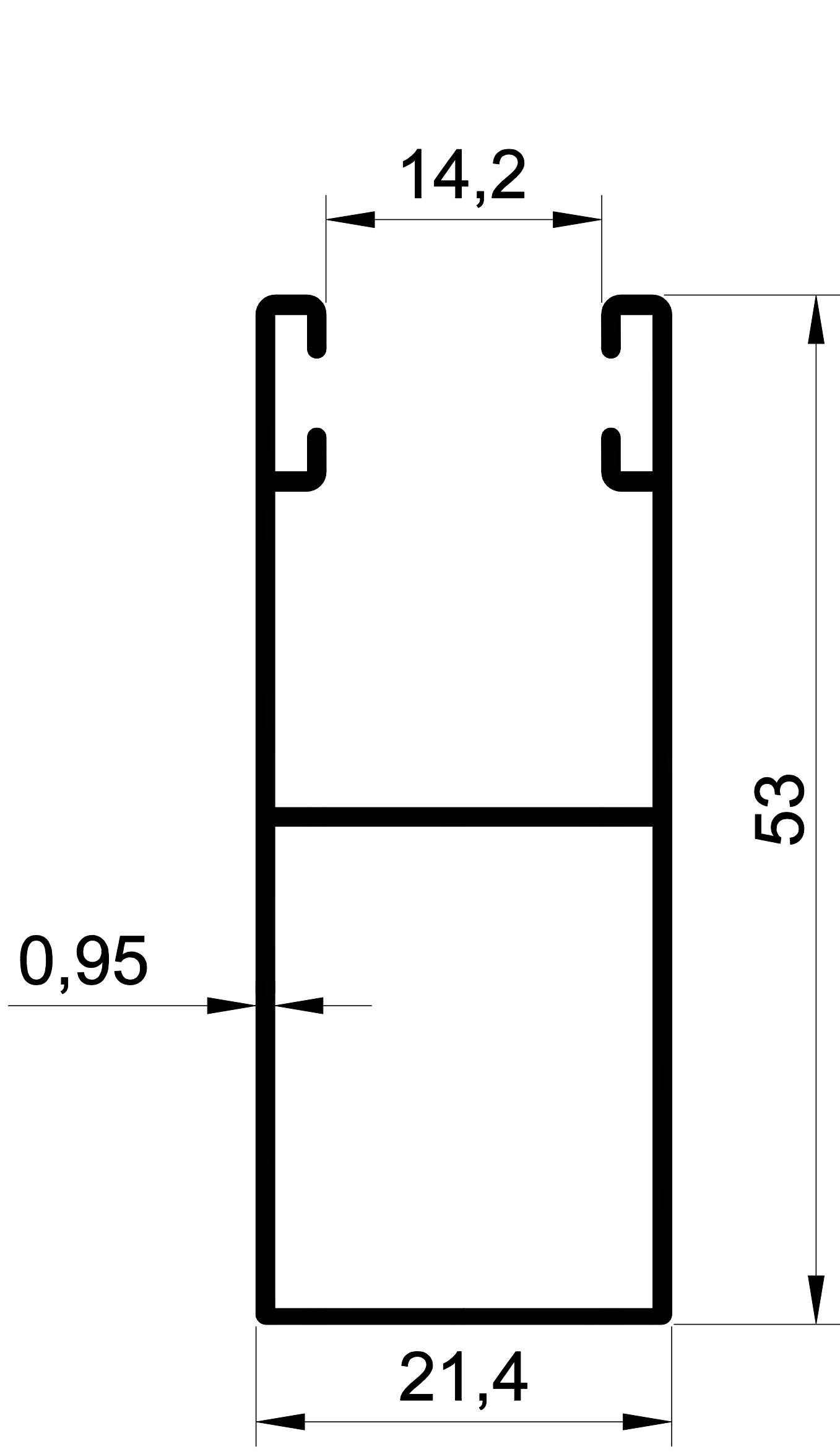
EKOL 1307 0,412 gr/m. 53'LÜK DİKME
