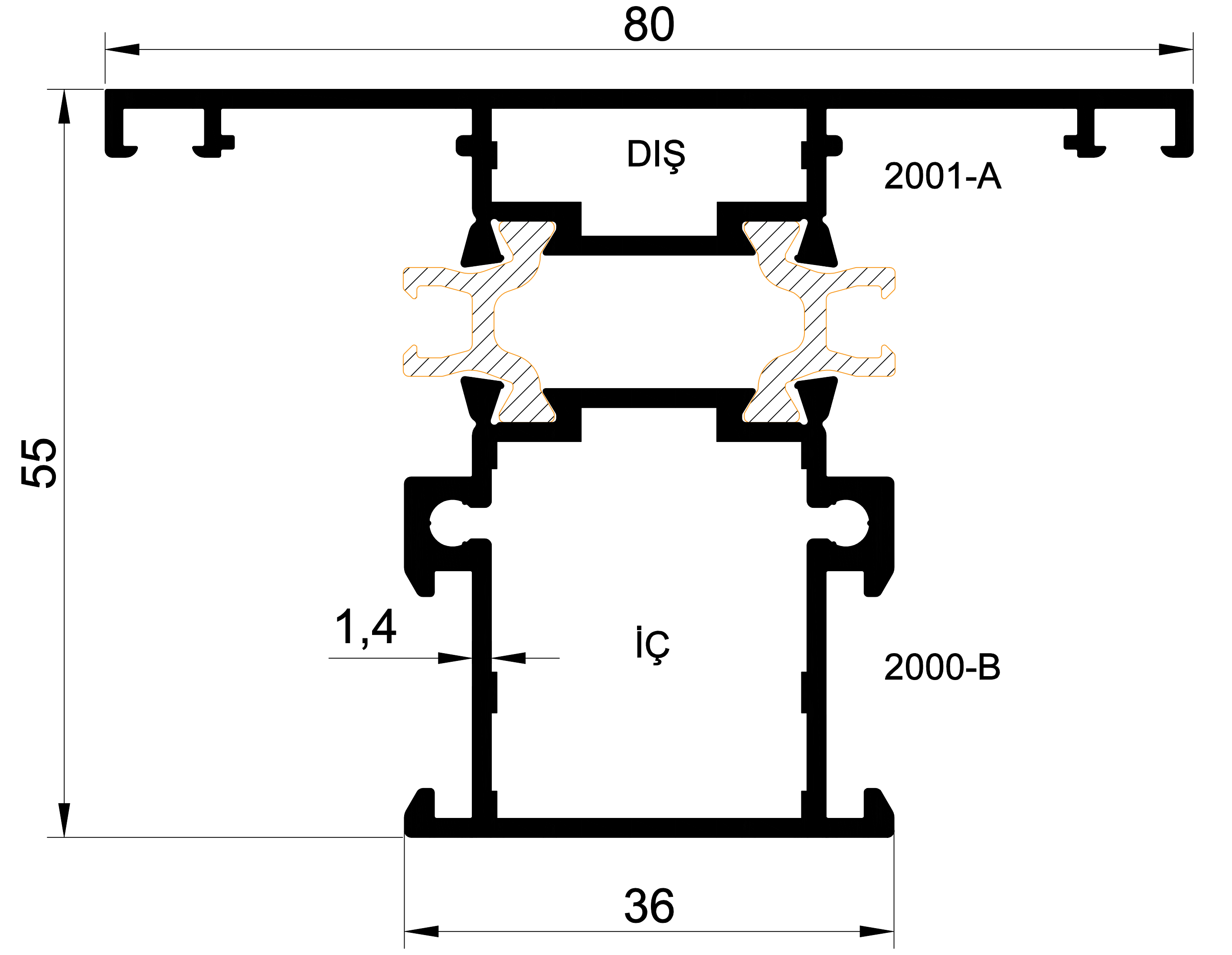
EKL-55- 2001 1,283 gr/m SİSTEM 55 ISI YALITIM ORTA
