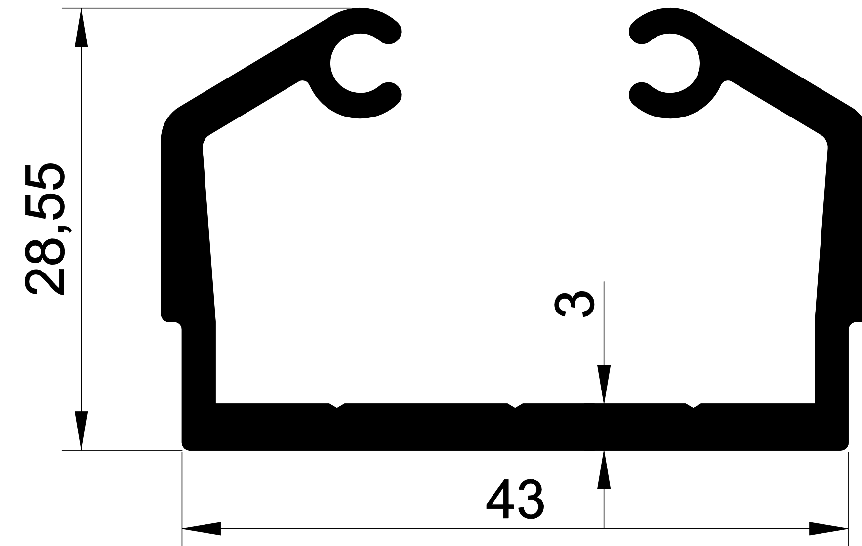
EKOL 1398 0,864 gr/m. CEPHE U BAĞLANTI
