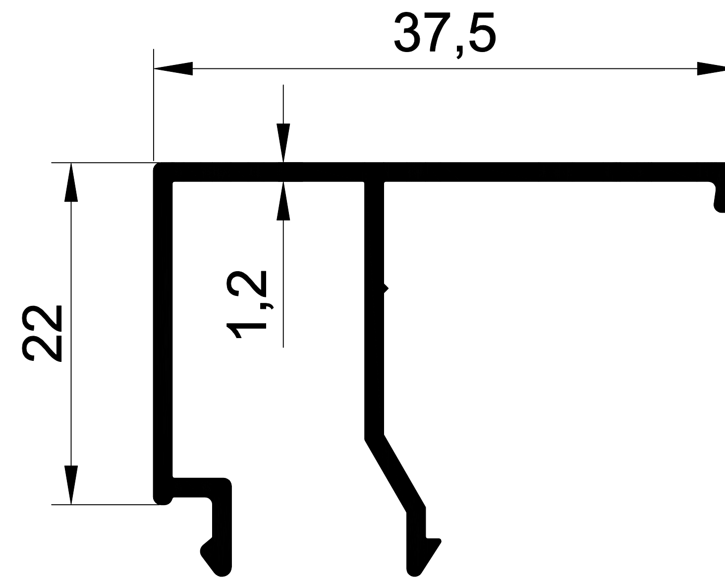
EKL-55- 2009 0,314 gr/m SİSTEM 55 TEK CAM ÇITASI
