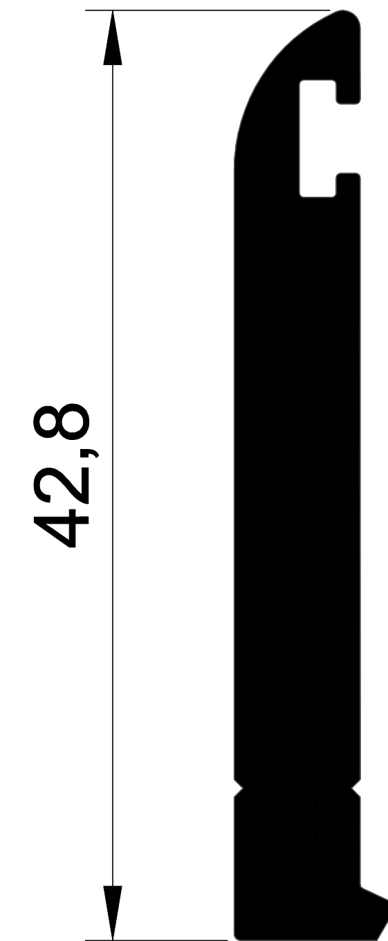
EKOL 1147 0,618 gr/m.
