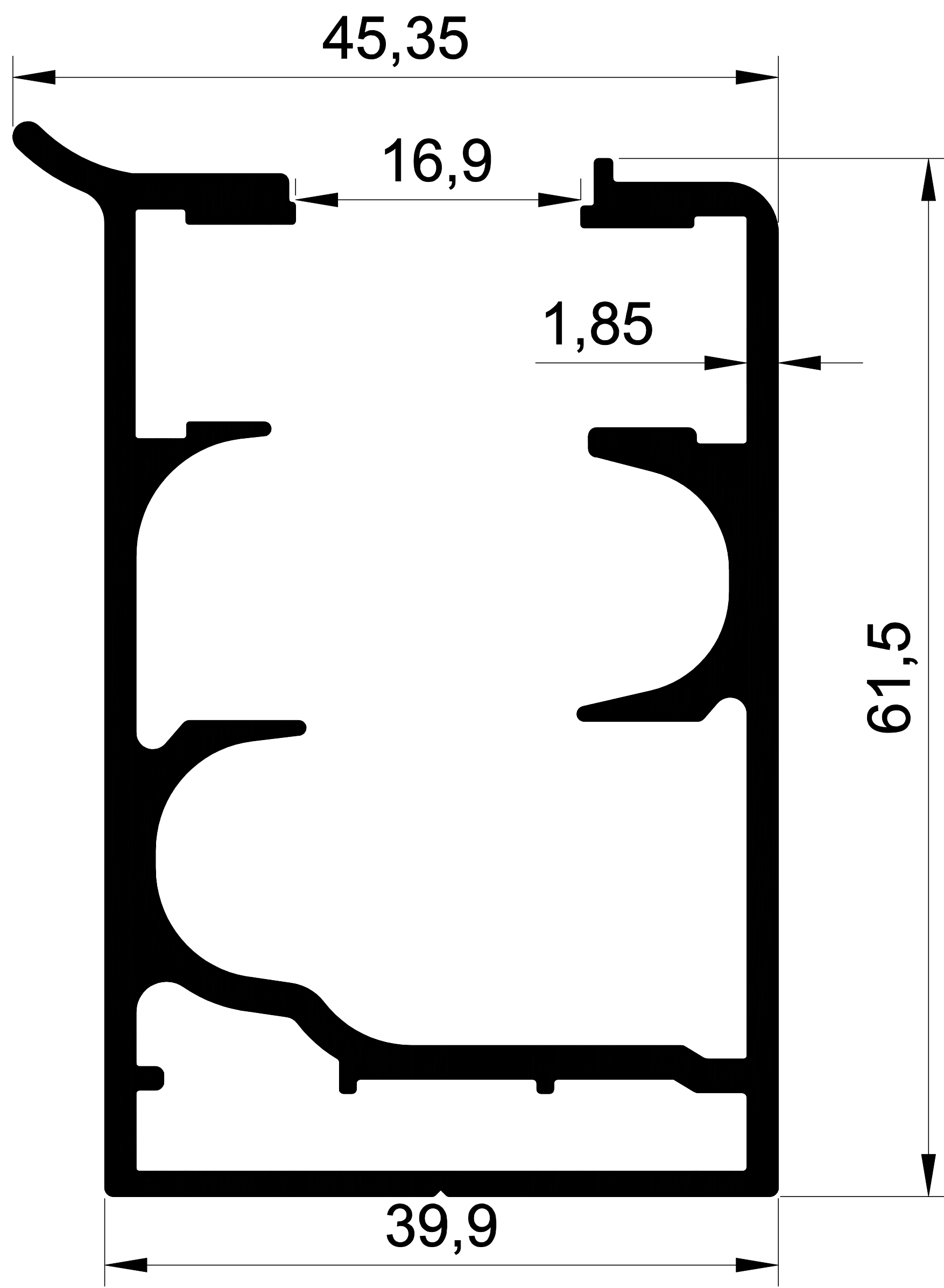
EKOL 1290 1,428 gr/m. BKS ÜSTTEN DAMLALIKLI KASA
