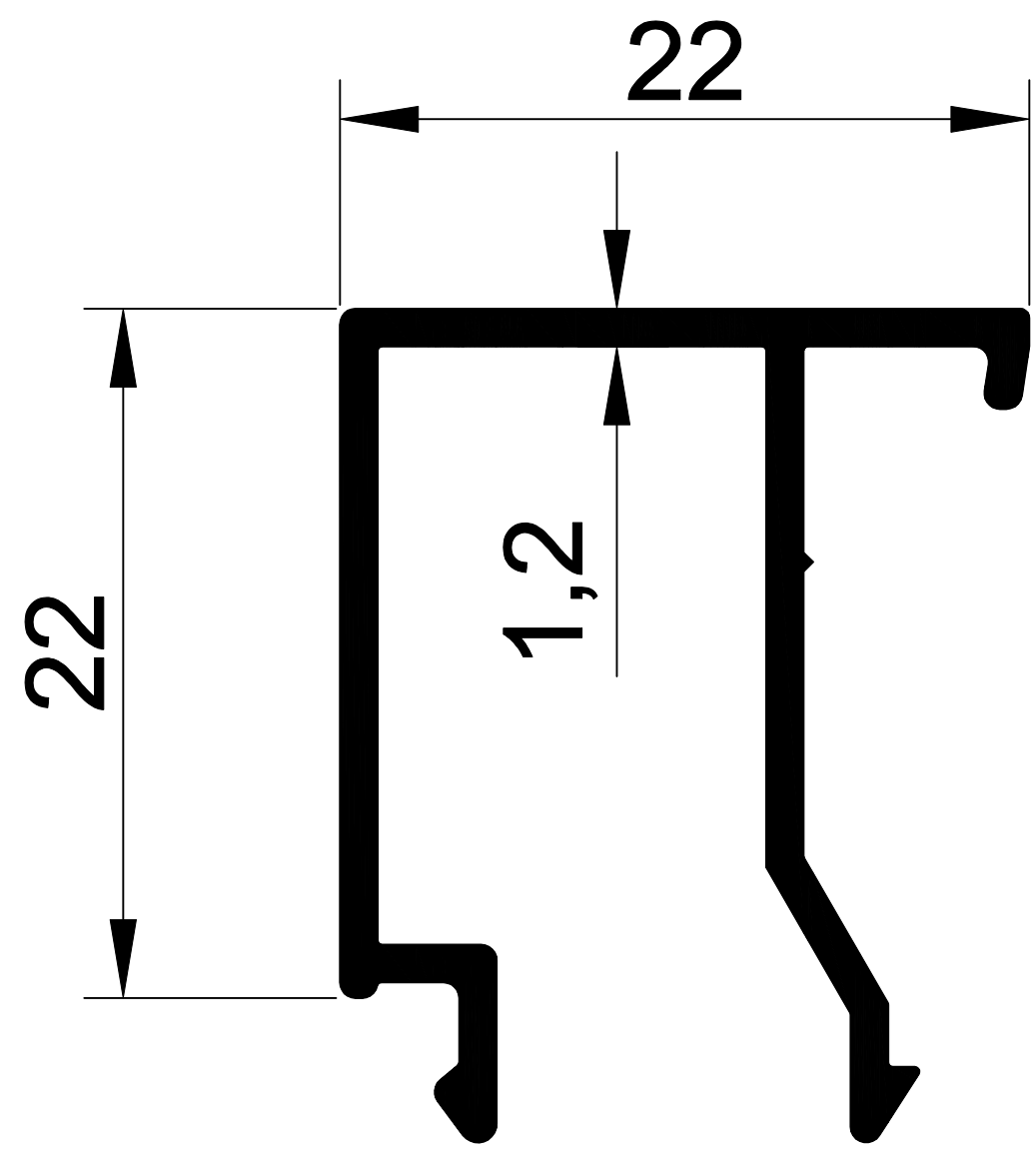
EKL-55- 2008 0,264 gr/m SİSTEM 55 ÇİFT CAM ÇITASI
