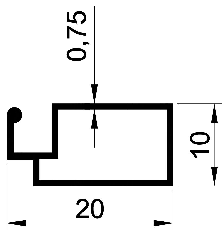
EKOL 1074 0,140 gr/m. 10*20 SİNEKLİK
