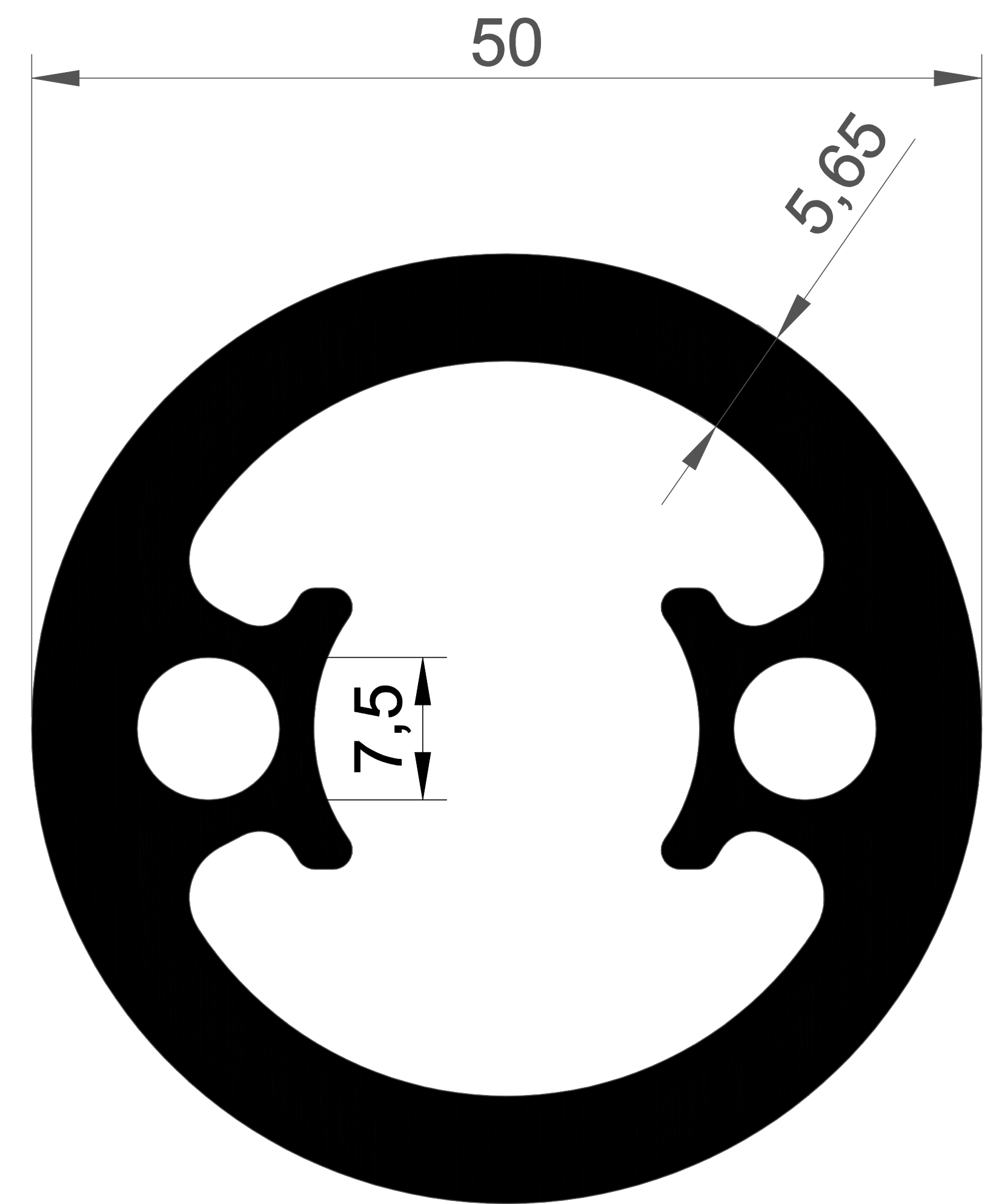
EKOL 1029-B 2,593 gr/m.
