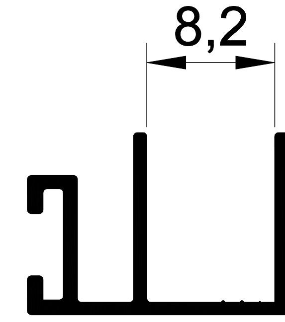
EKOL 1171 0,122 gr/m. SÜRME YAN ÇITA
