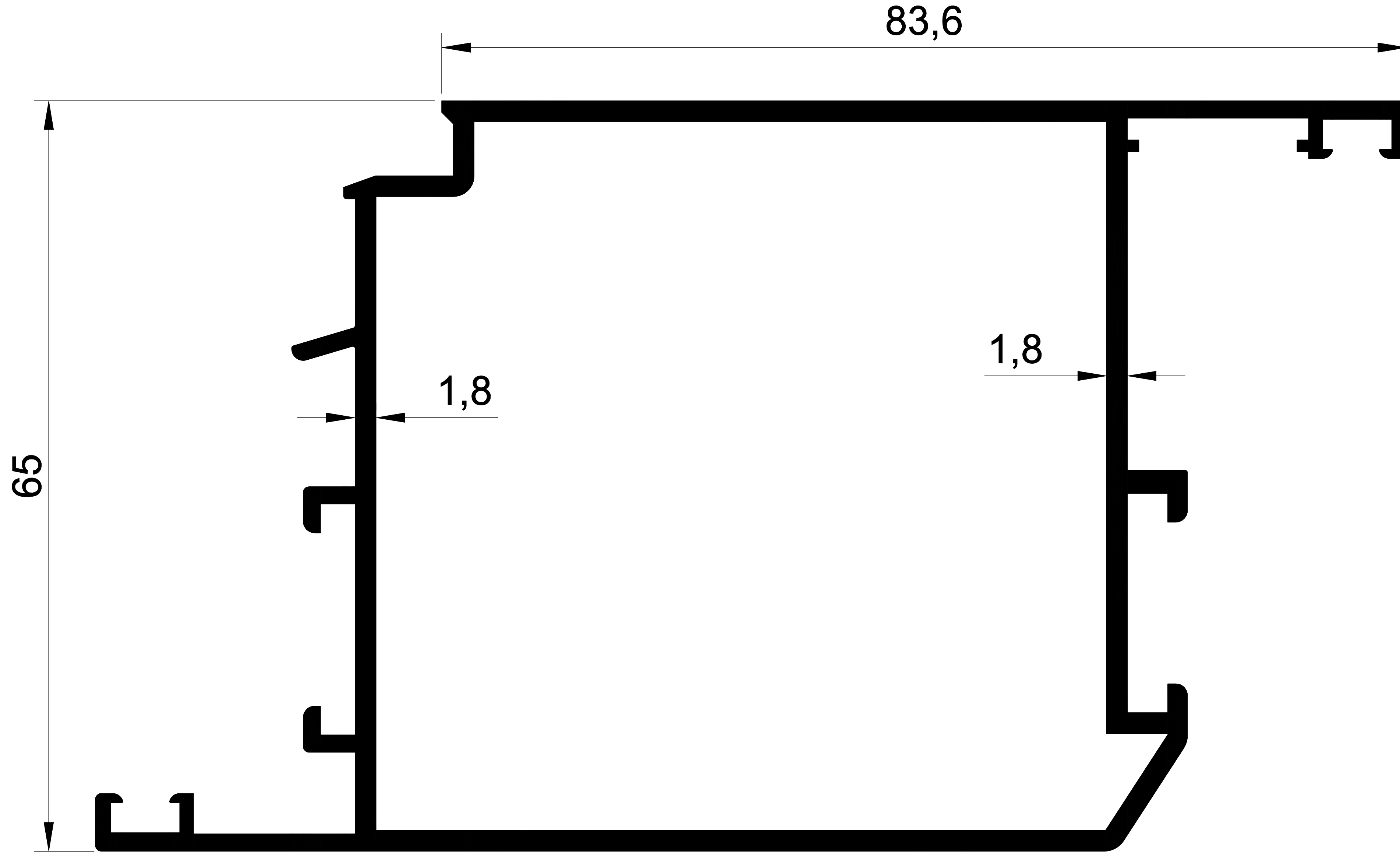
EKOL 1202 1,667 gr/m. SİSTEM BAZA KAPI
