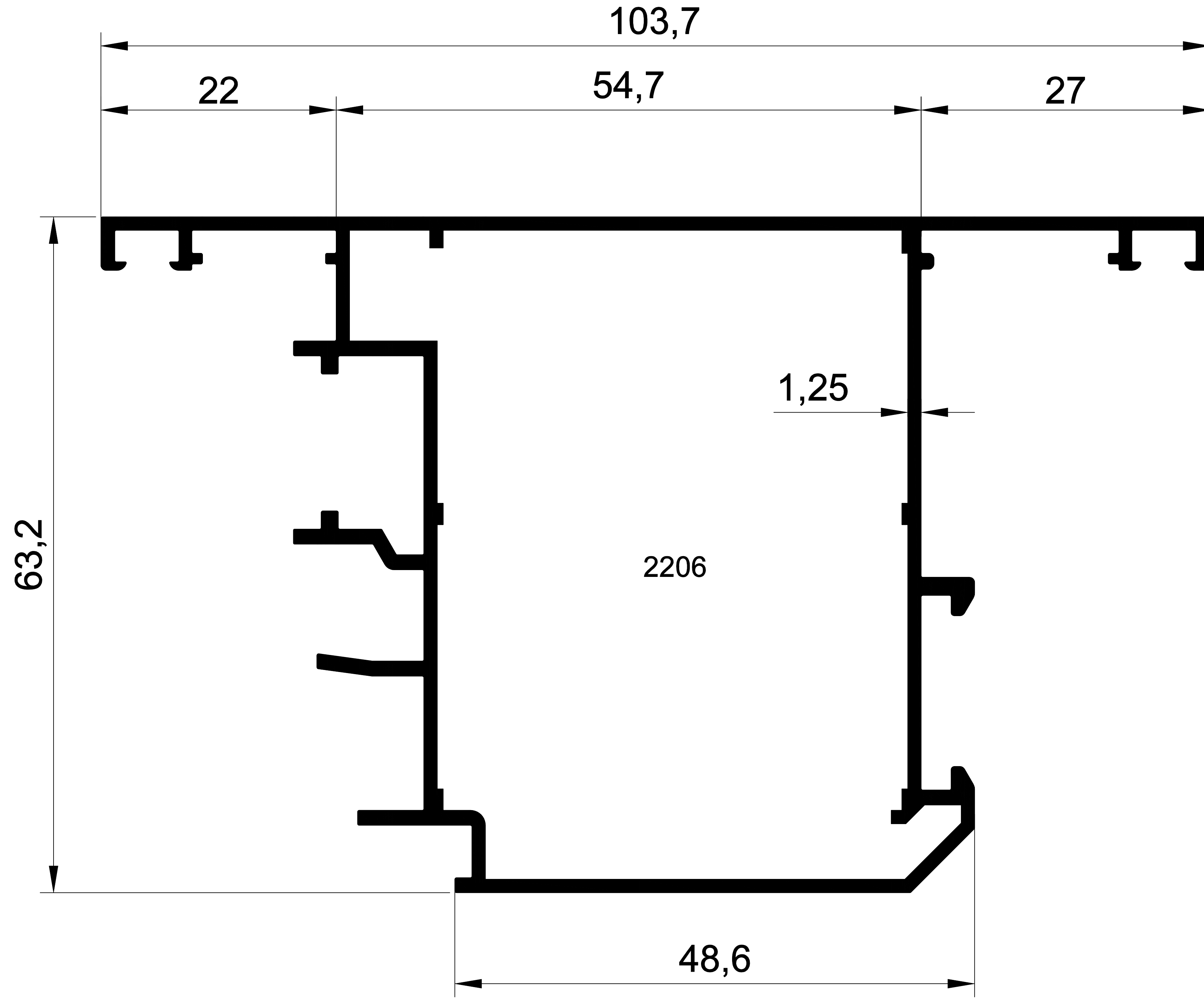
EK-55- 2206 1,267 gr/m SİSTEM 55 DIŞA AÇILIR KAPI
