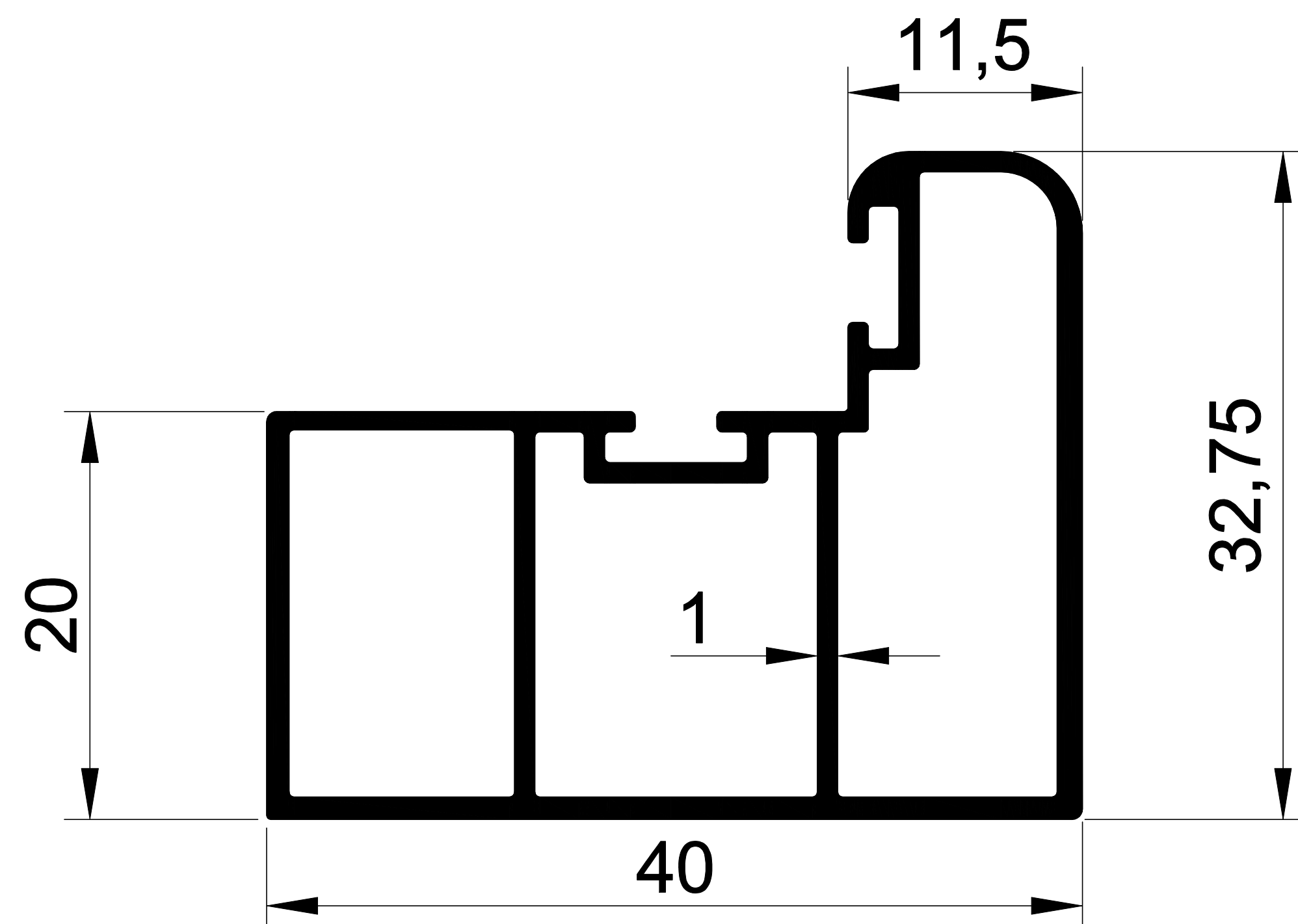
EKOL 1184 0,533 gr/m. BKS DİKME
