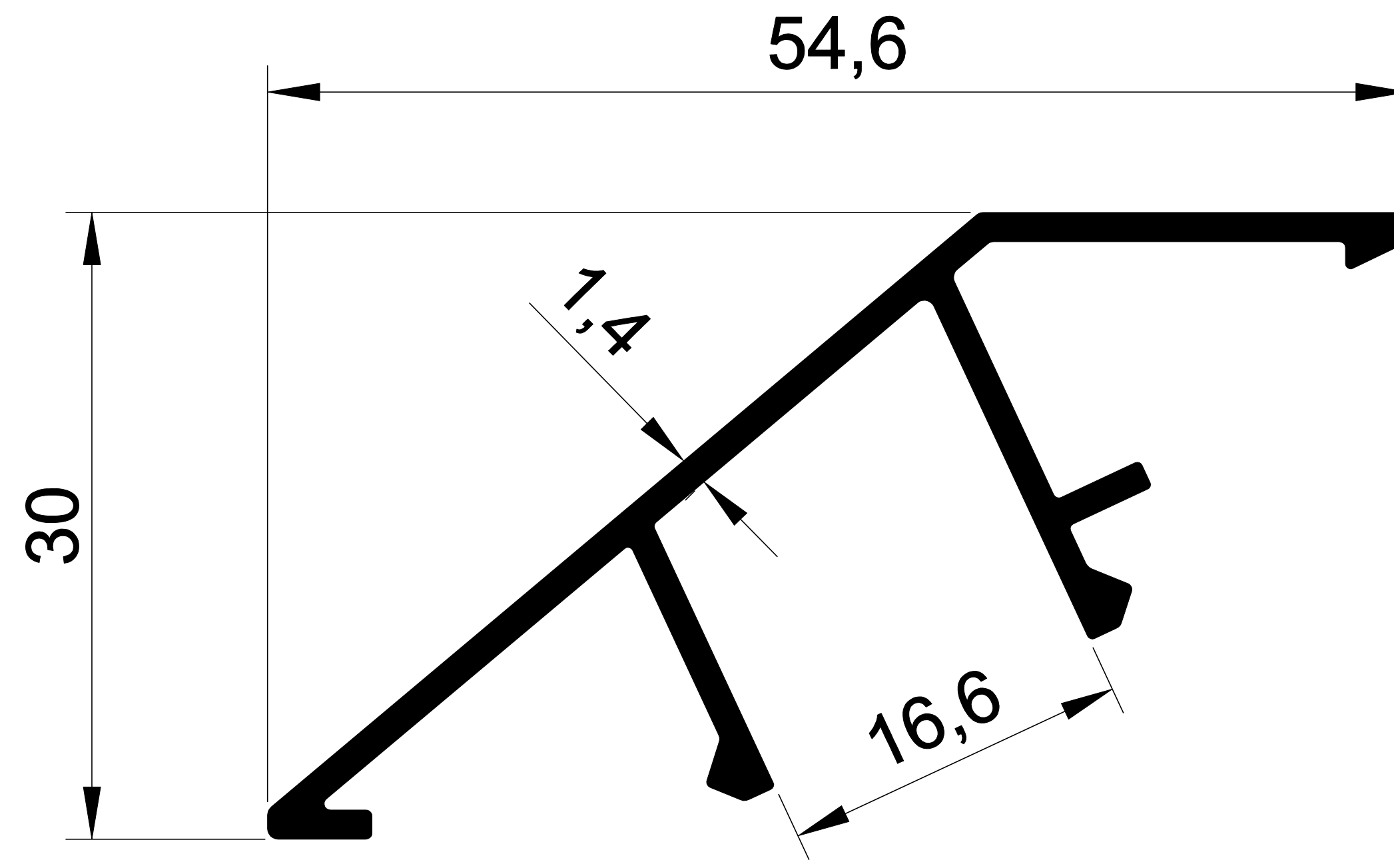
EKOL 1433 0,420 gr/m. MENFEZ YAPRAK
