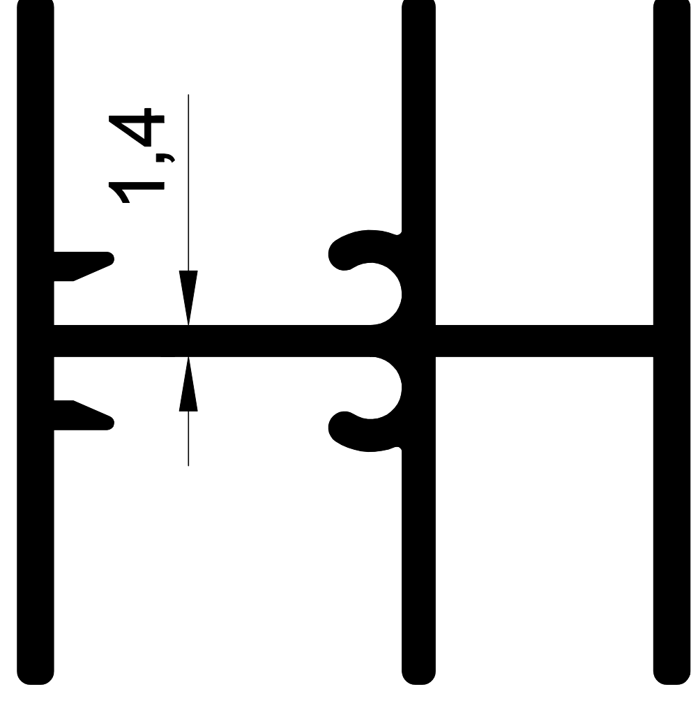
EKOL 1156 0,550 gr/m. MEBO ORTA
