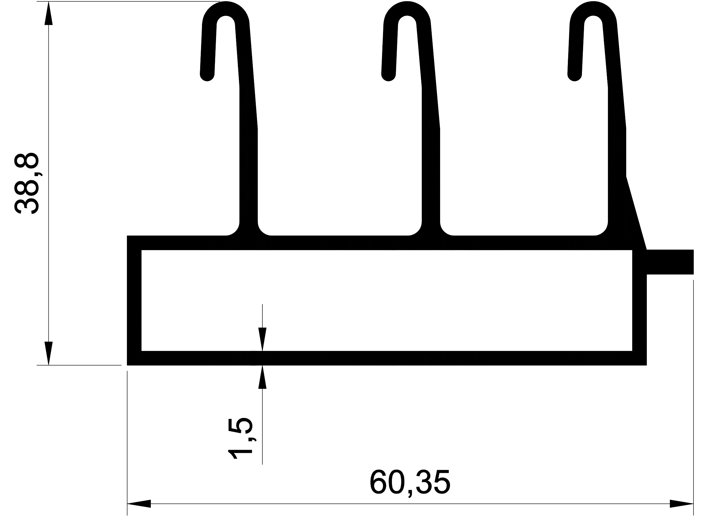
EKOL 1314 1,051 gr/m. 3'LÜ SÜRME EŞİKLİ RAY
