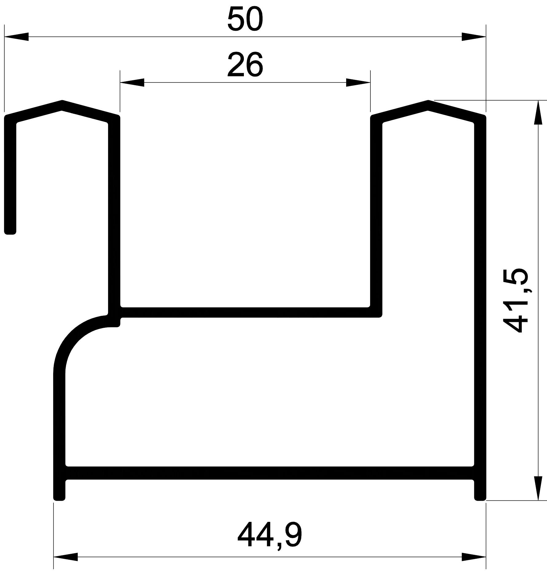
EKOL 1381 0,655 gr/m. 2000 SERİ SÜRME KASA
