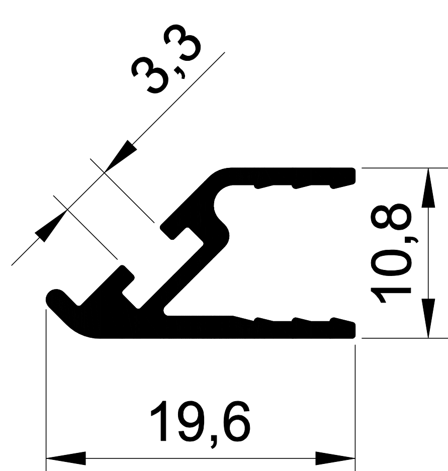
EKOL 1249 0,152 gr/m. CAM H
