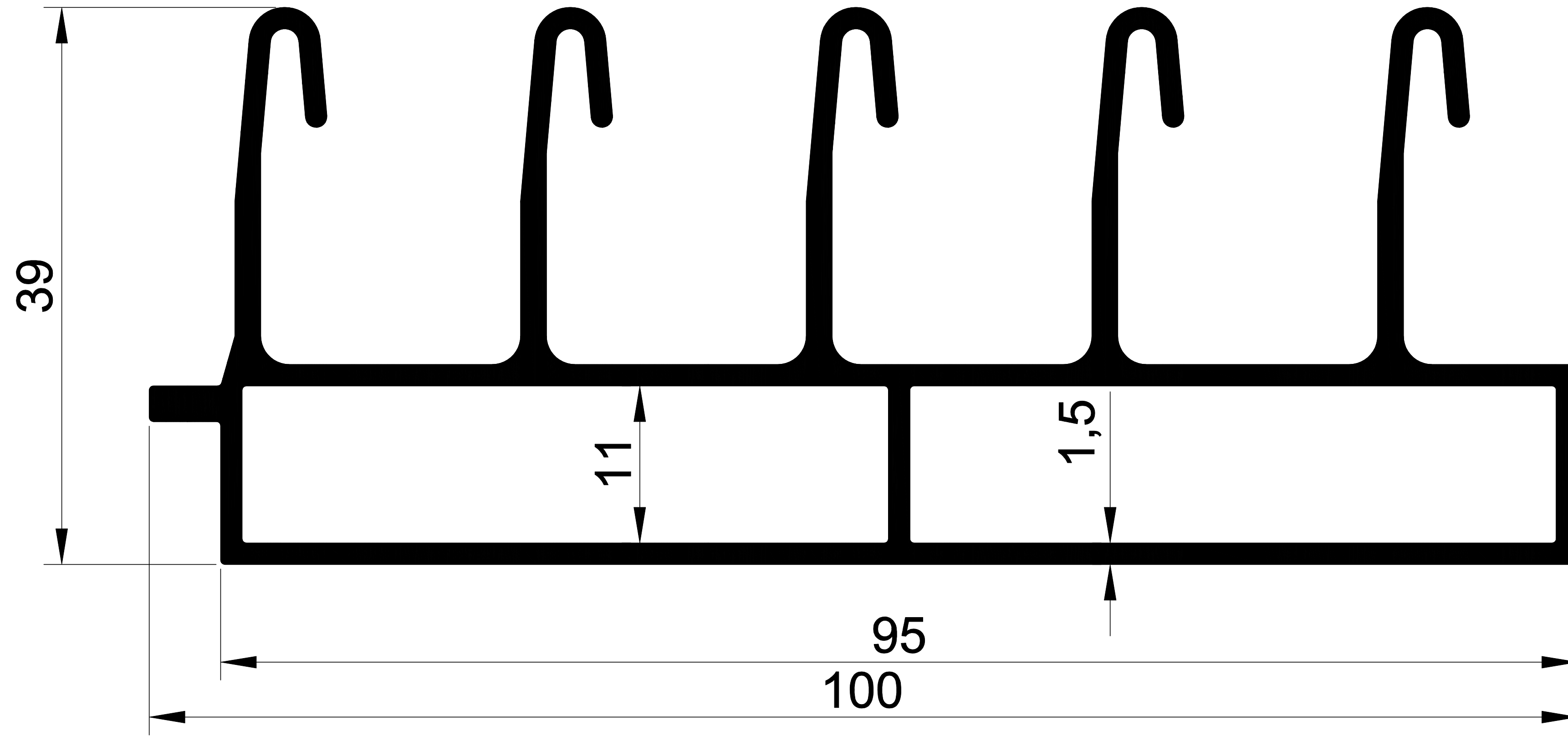
EKOL 1164 1,702 gr/m. SÜRME EŞİKLİ RAY
