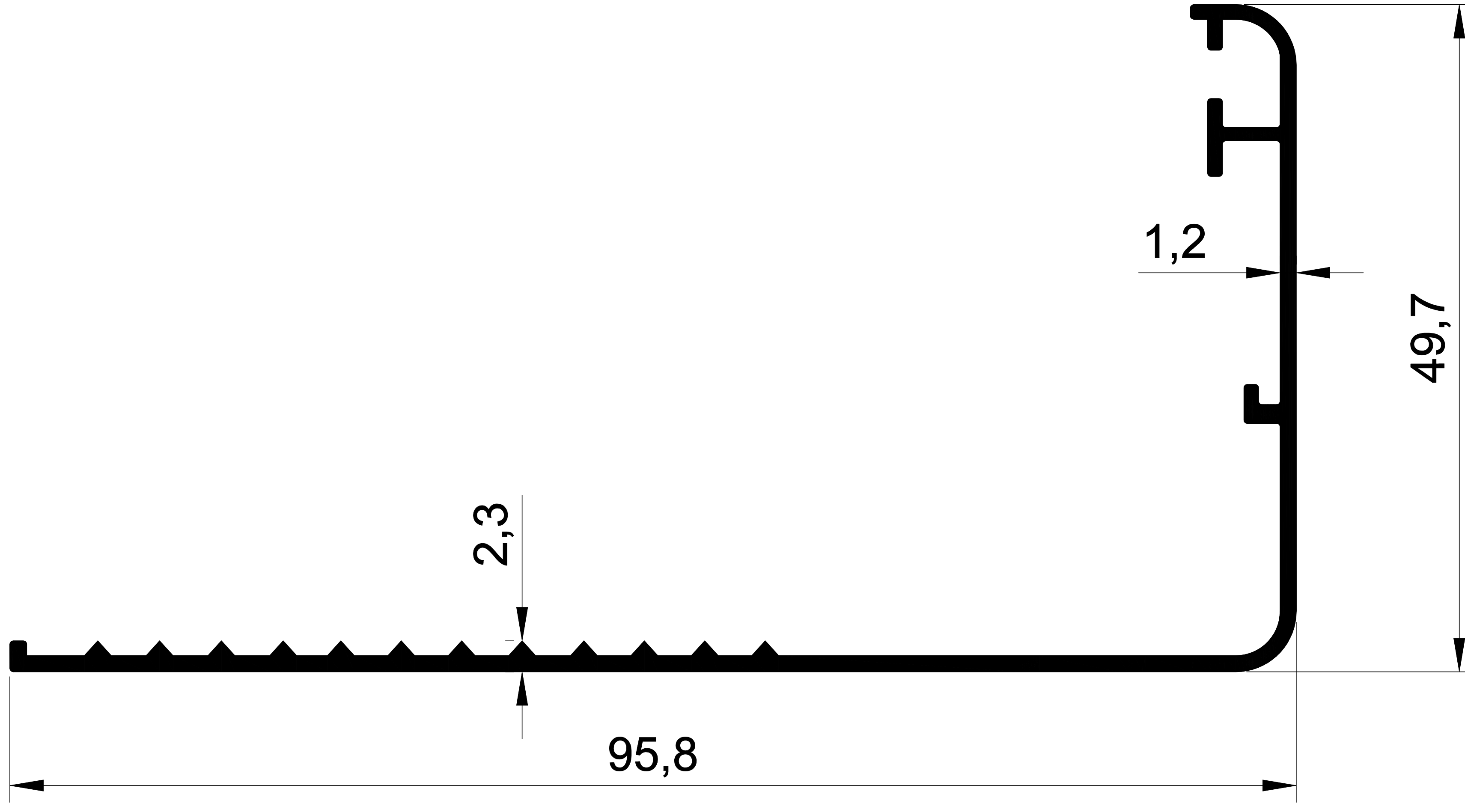
EKOL 1267 0,566 gr/m. ALÜMİNYUM PERVAZ
