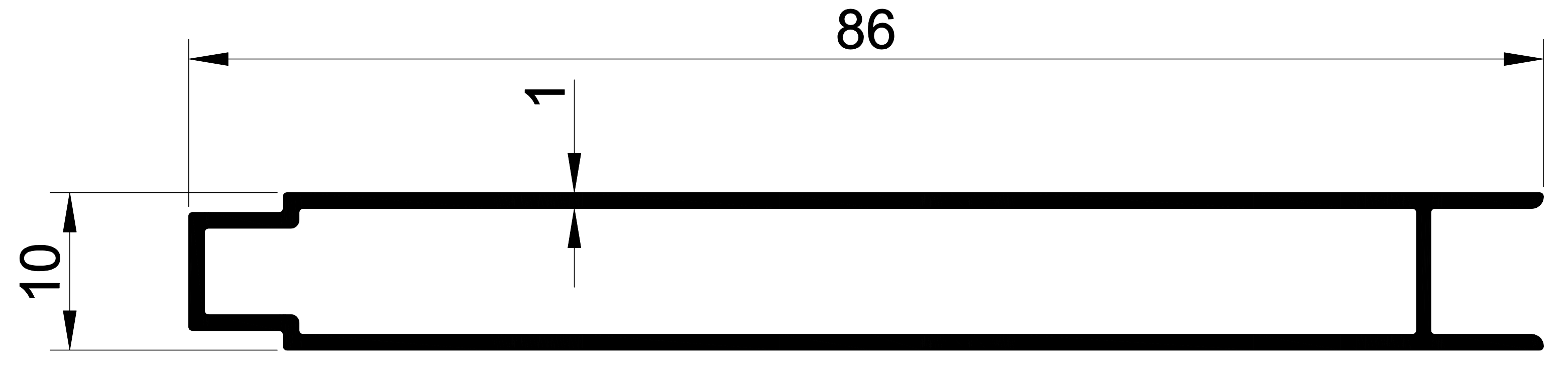
EKOL 1182 0,507 gr/m. ALÜMİNYUM TAHTA LAMBİRİ
