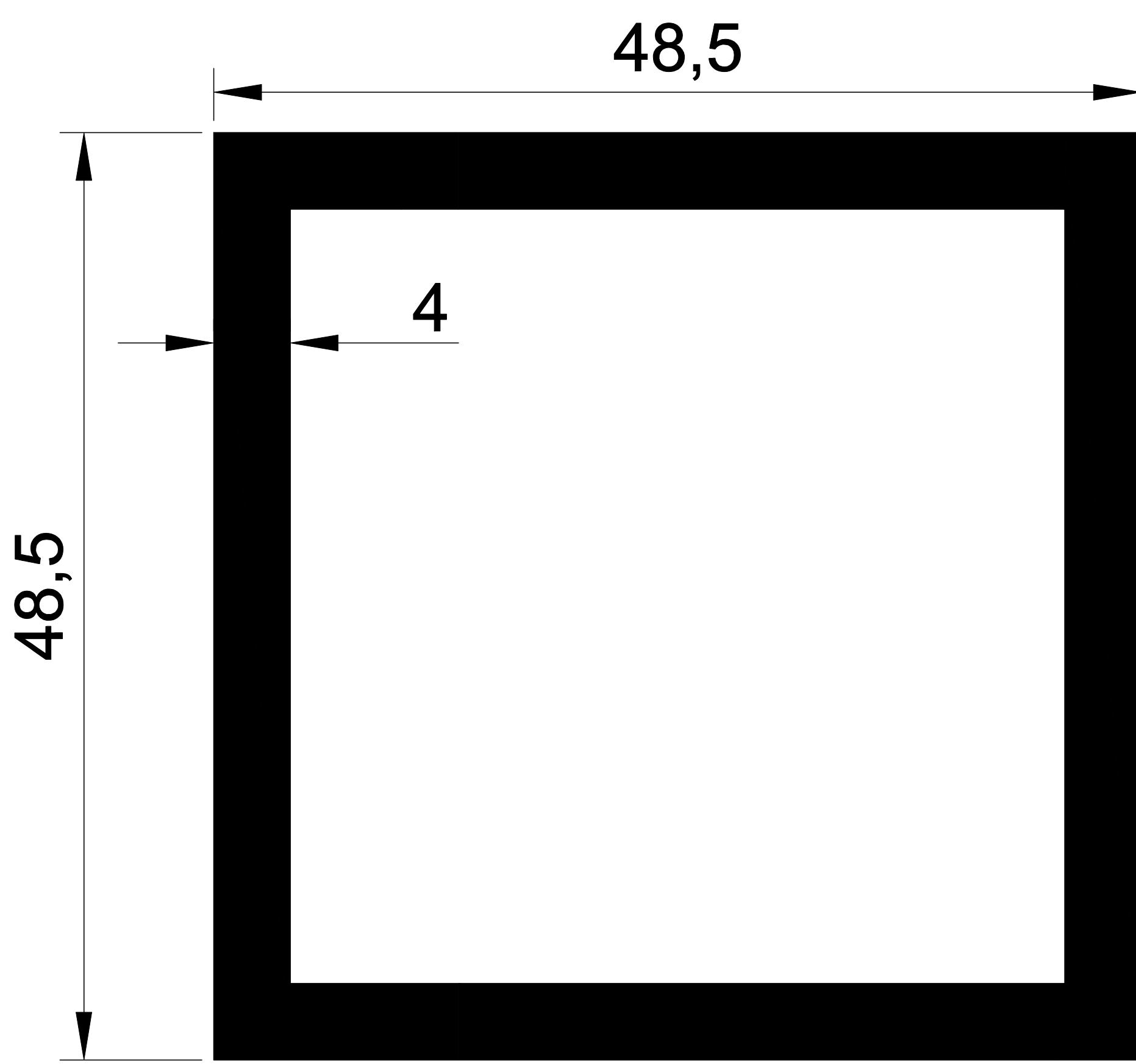
EKOL 1049 1,929 gr/m.
