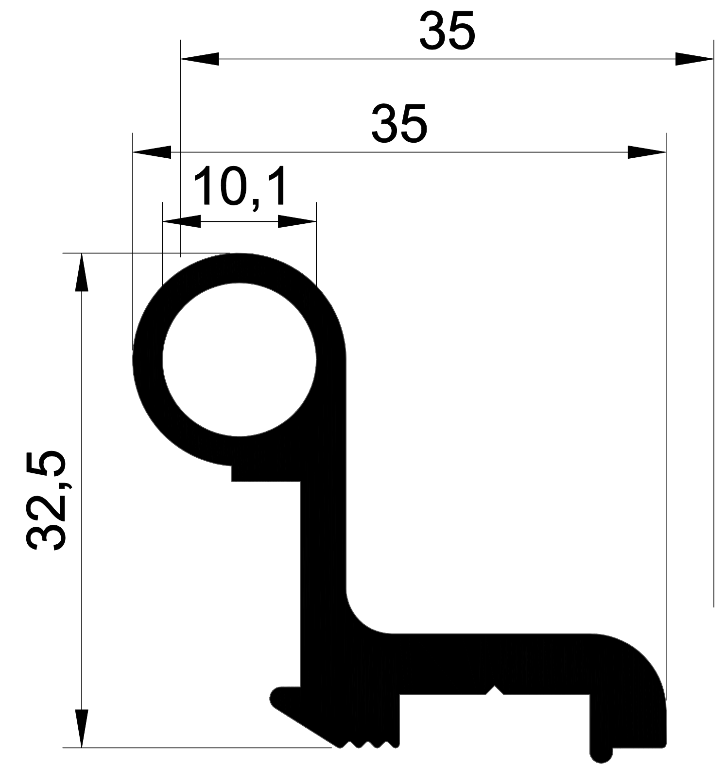
EKOL 1241 0,694 gr/m.
