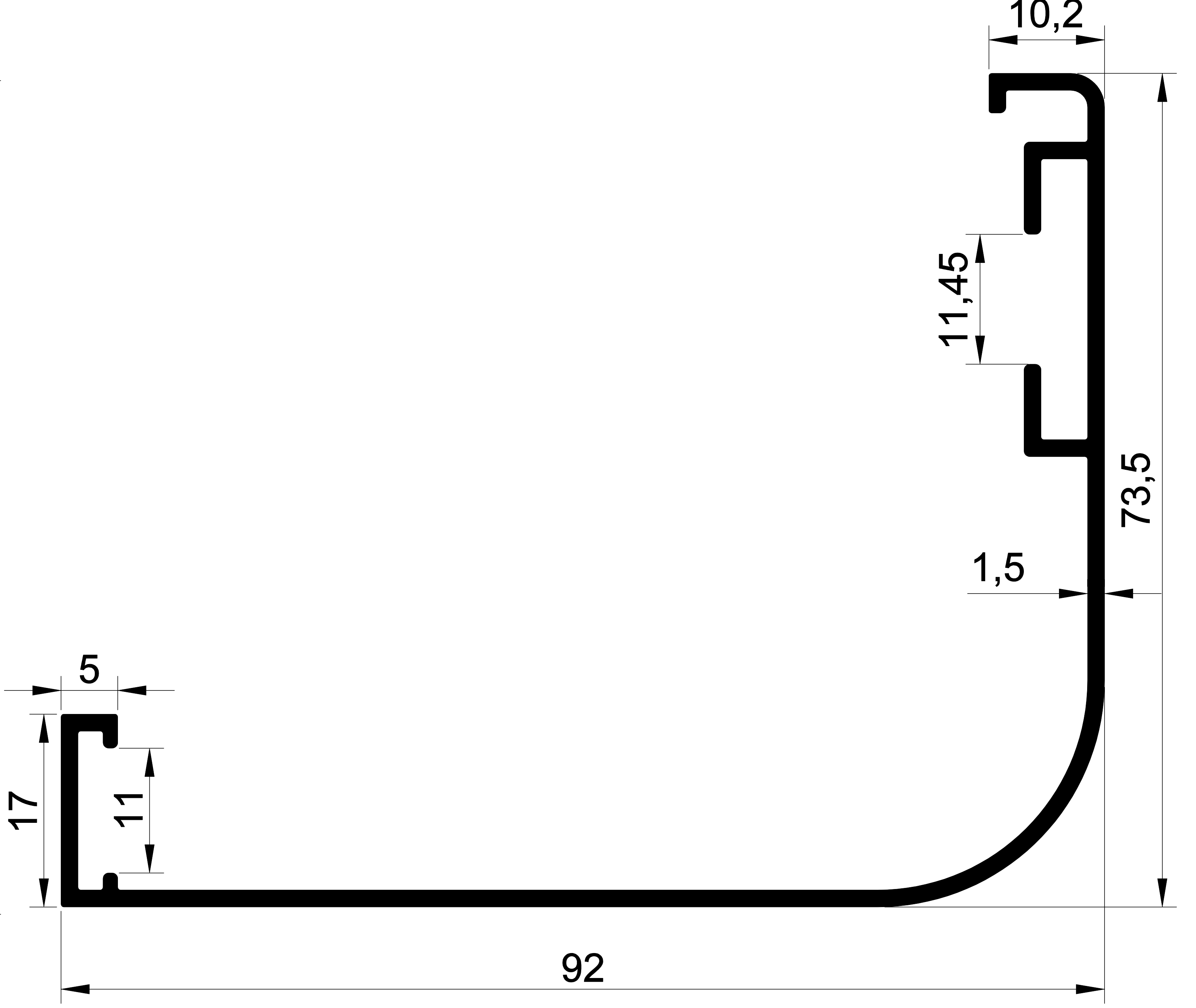
EKOL 1423 0,859 gr/m. MS-92'LİK PEERVAZ
