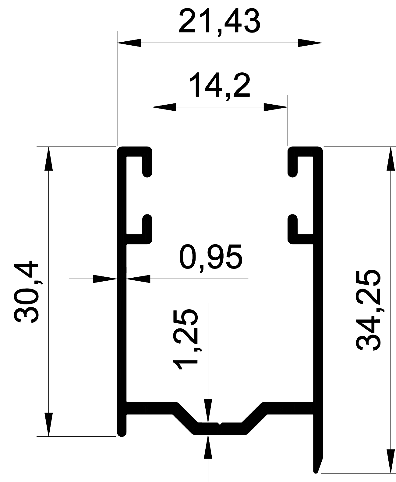
EKOL 1310 0,287 gr/m. MAKAS FİTİLLİ U
