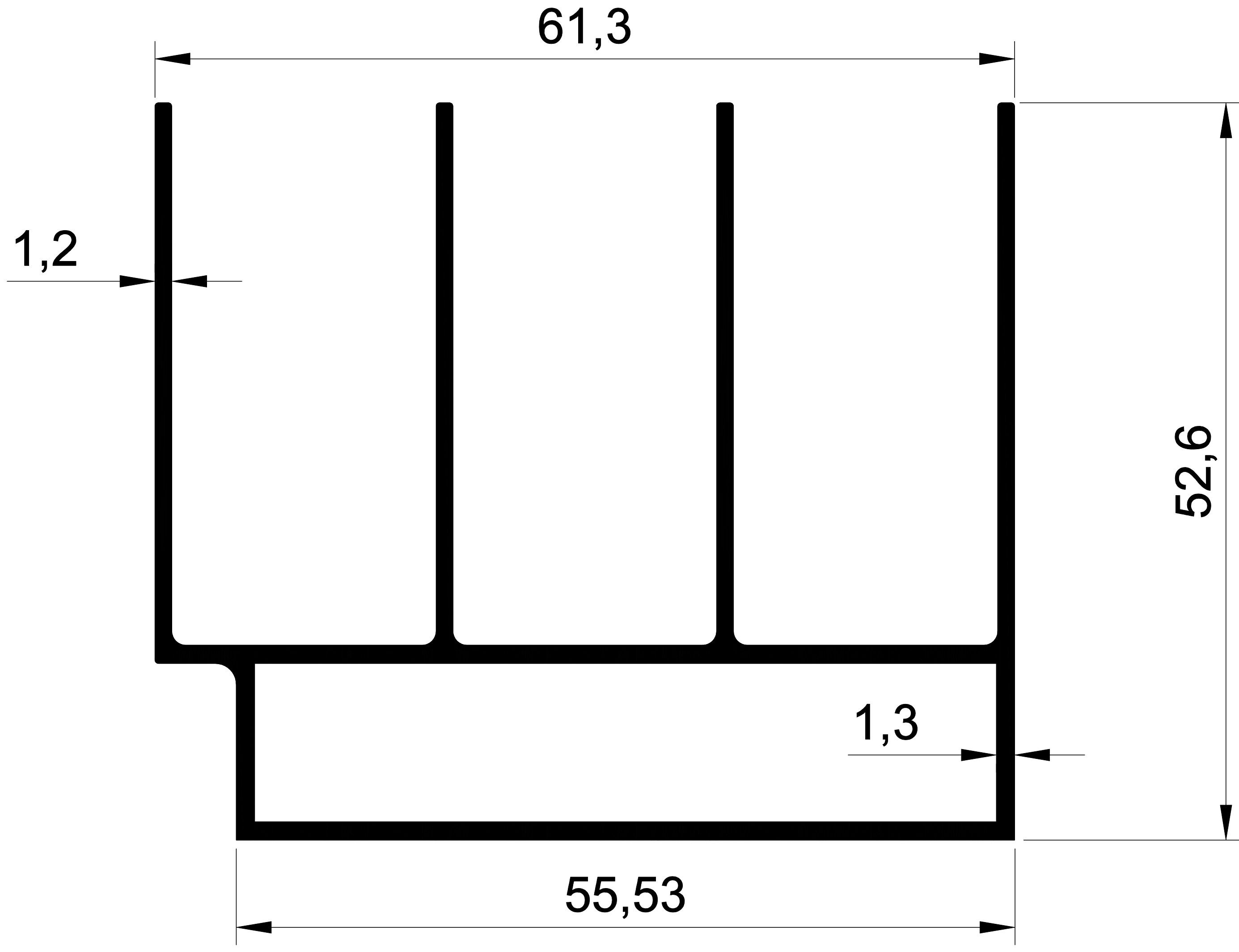
EKOL 1313 1,000 gr/m. 3'LÜ SÜRME KASA
