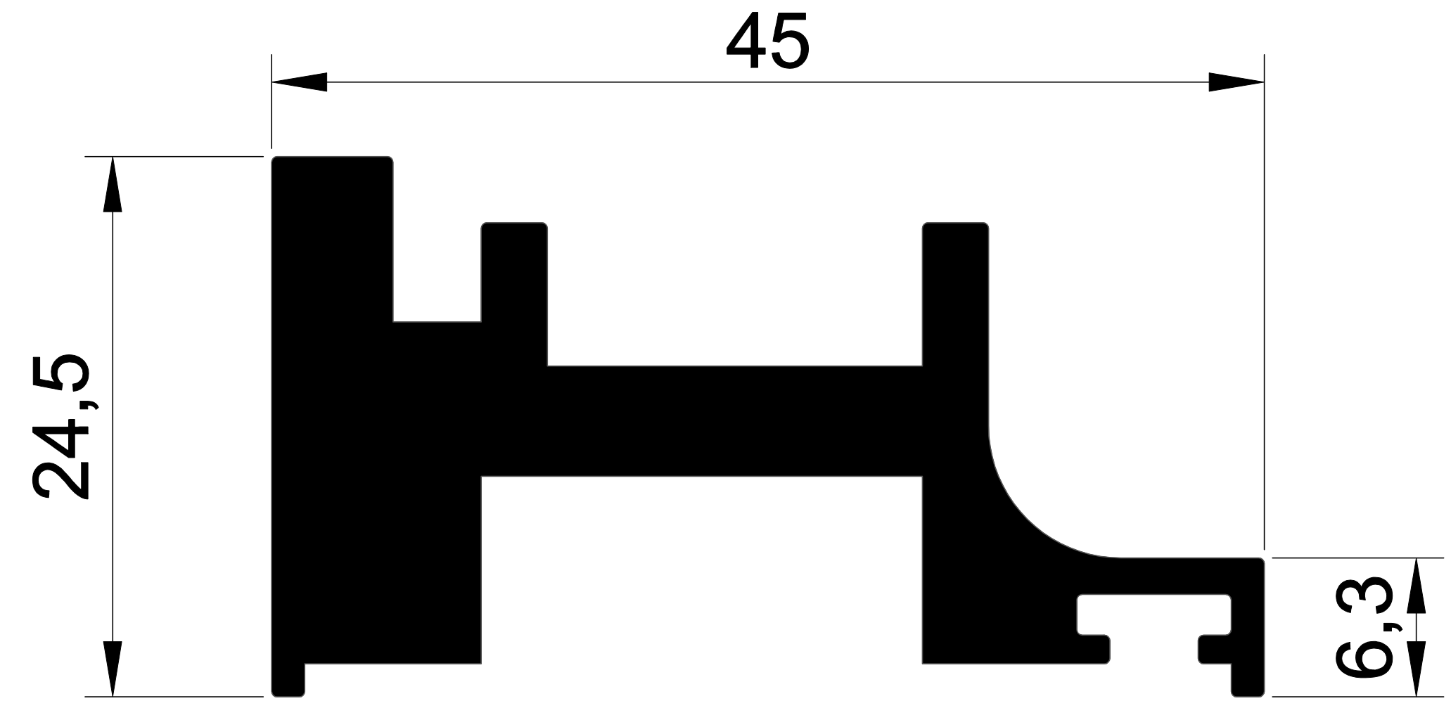
EKOL 1223 1,140 gr/m.
