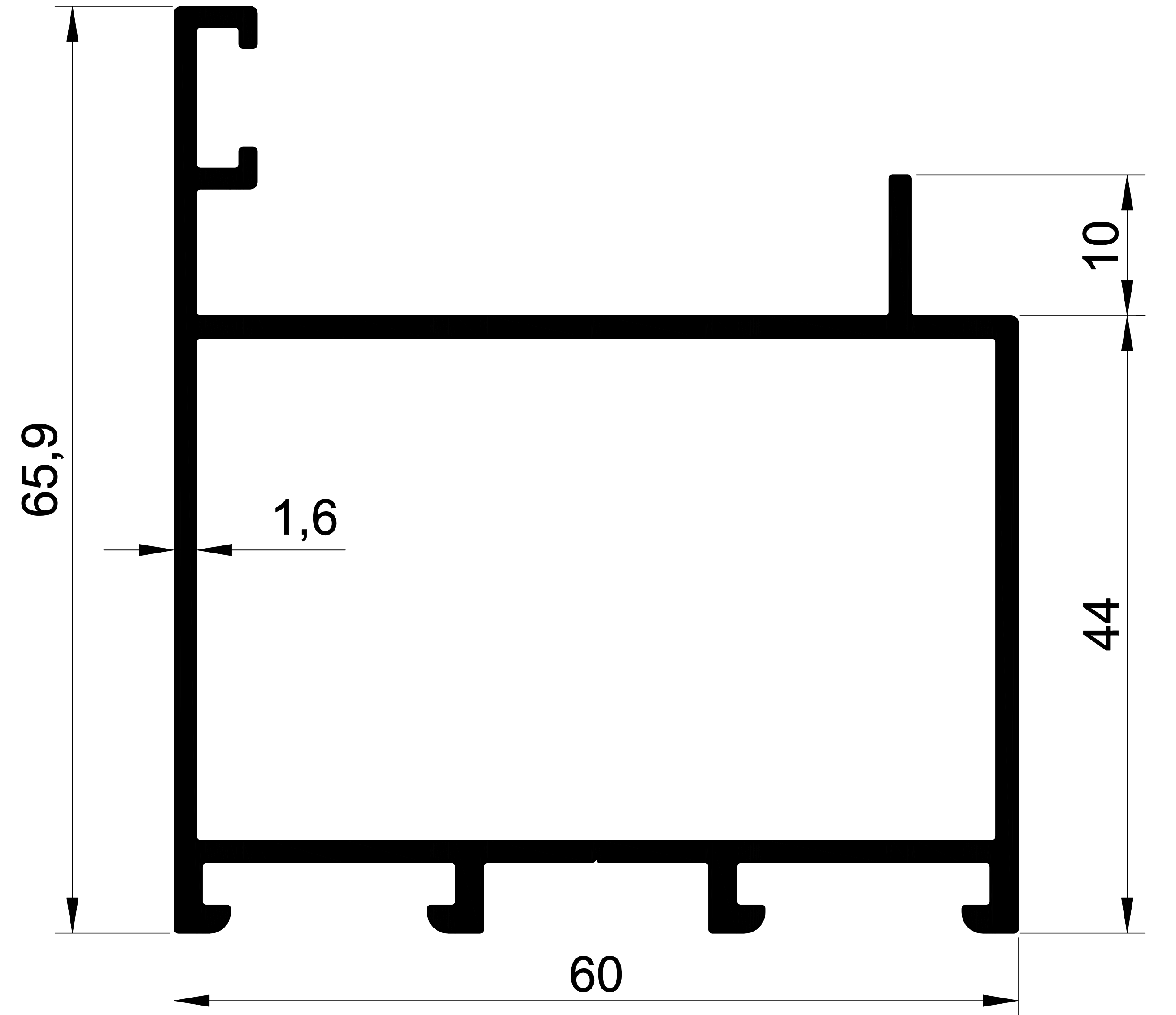
EKOL 1088 0,935 gr/m. 1.2 MM C-60 KANAT
