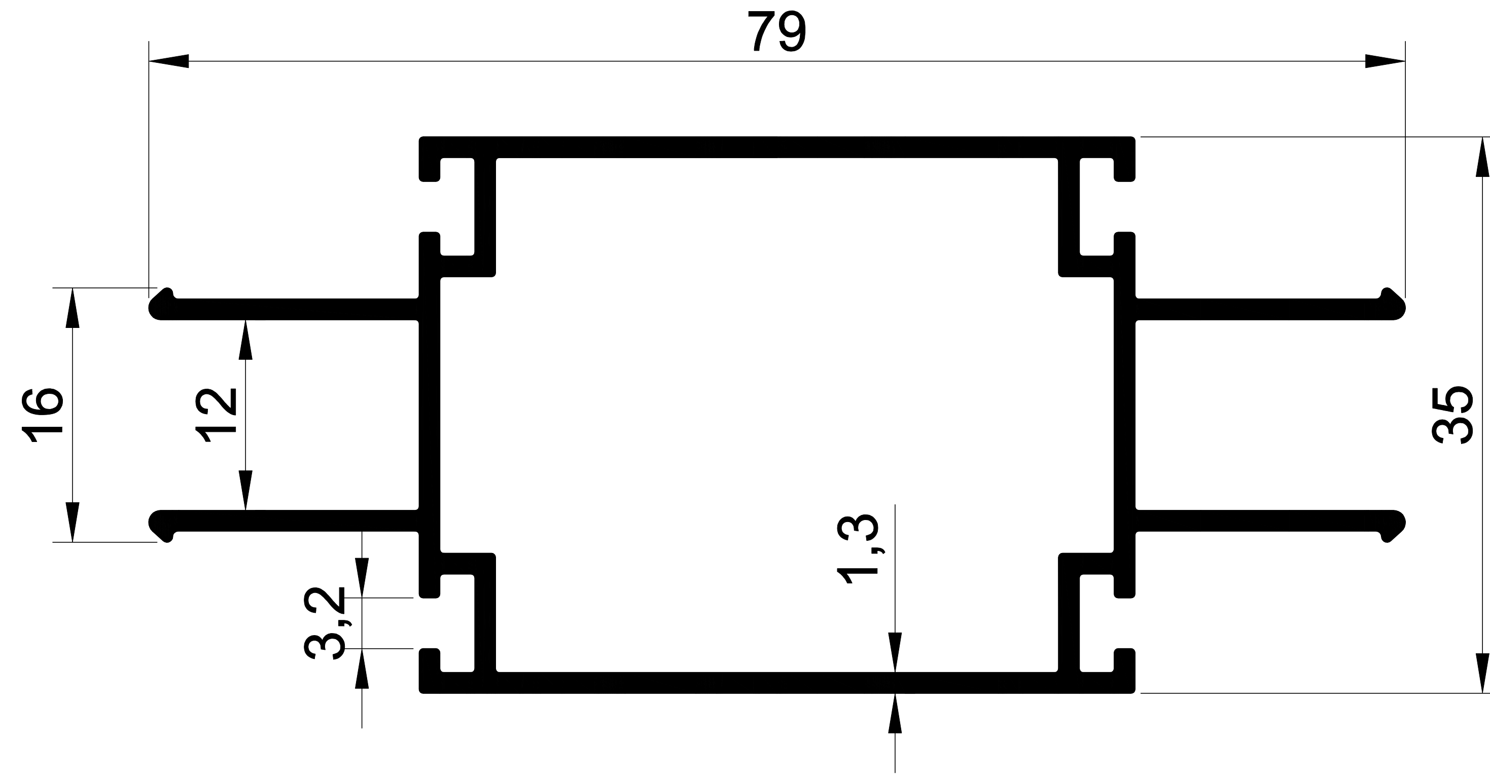
EKOL 1414 0,882 gr/m. JALUZİ OFİS BÖLME KASA
