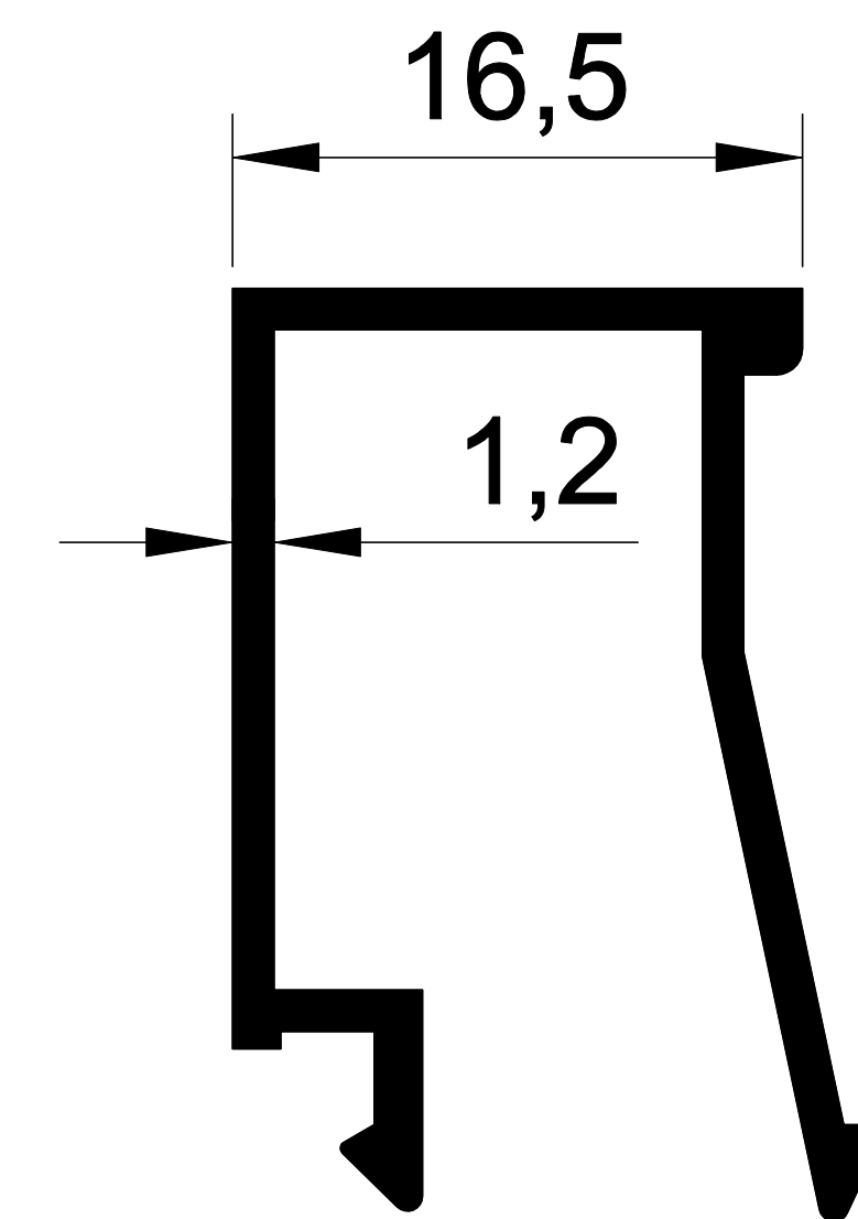
EKOL 1085 0,249 gr/m. C-60 ISI CAM ÇİTASI
