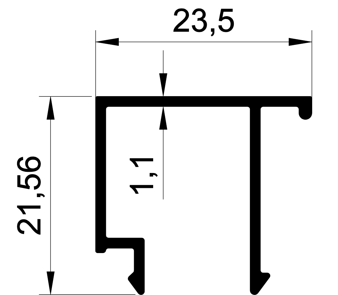
EKOL 1086 0,215 GR/M C-60 TEK CAM ÇİTASI
