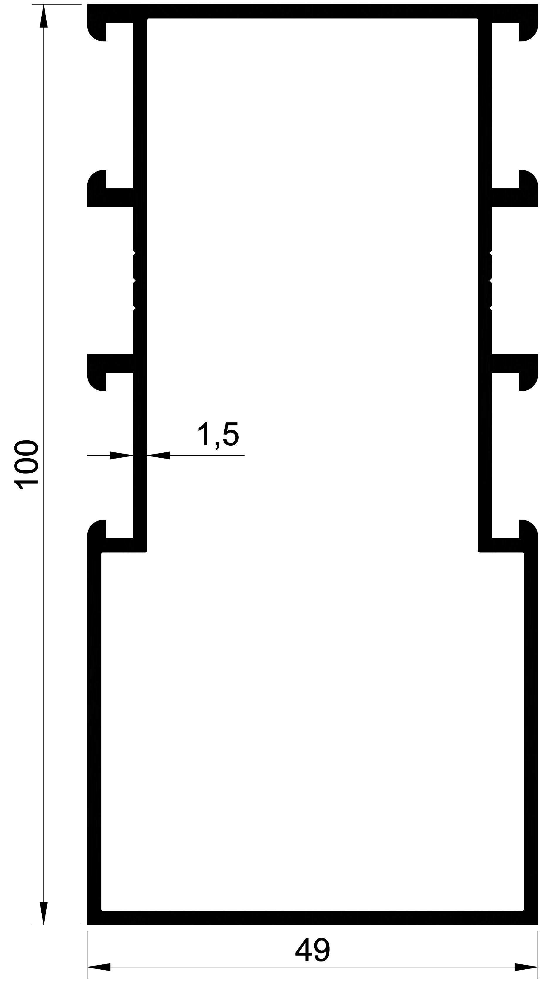
EKOL 1306 1,420 gr/m. C-60 TAKVİYELİ KASA
