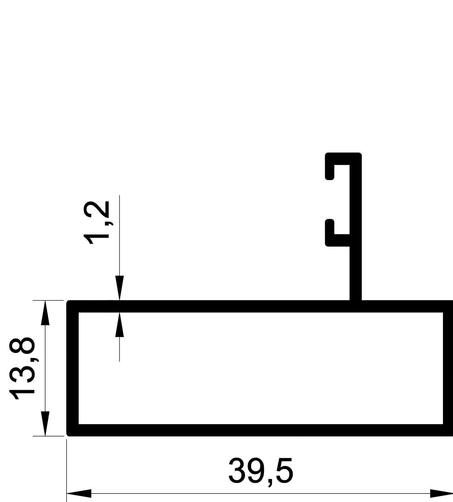
EKOL 1145 0,404 gr/m. GOLD DİKME
