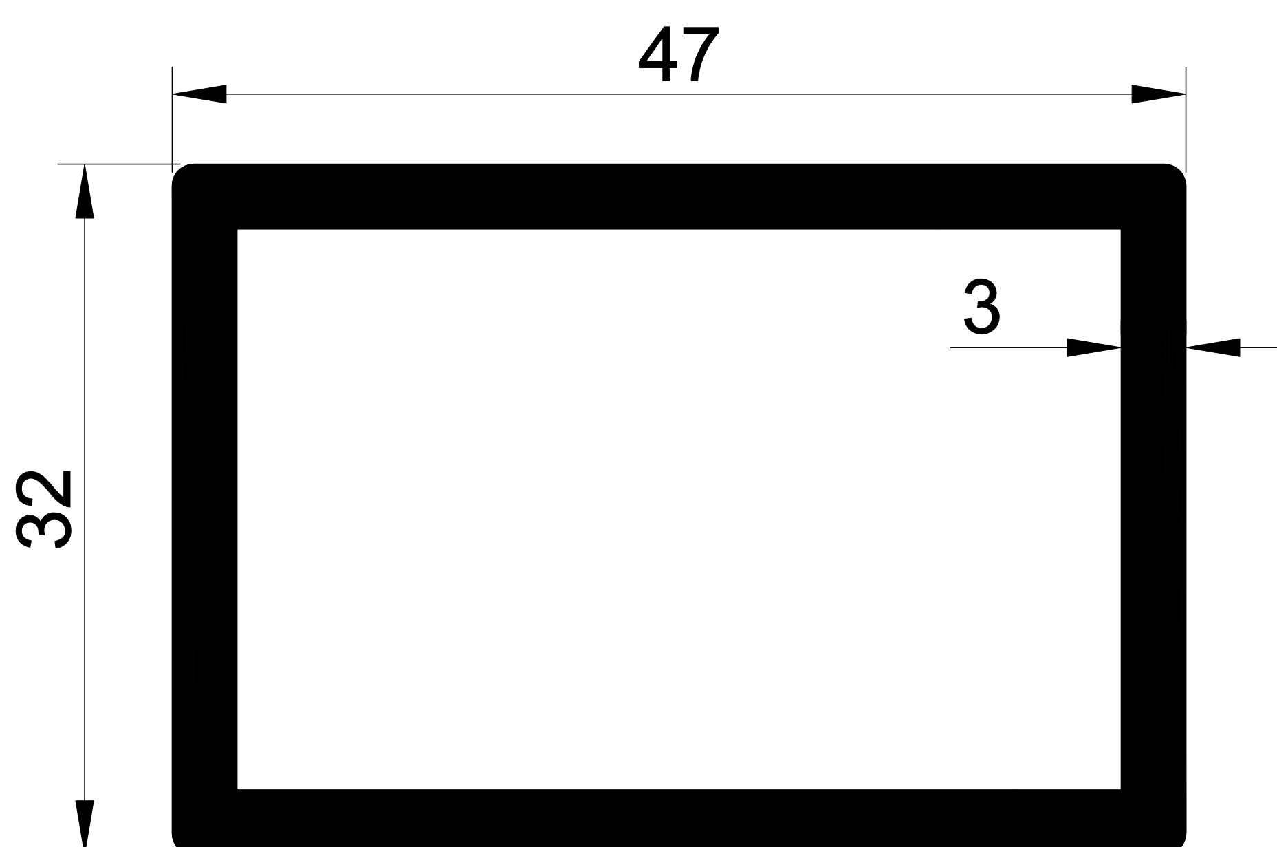
EKOL 1277 1,184 gr/m.
