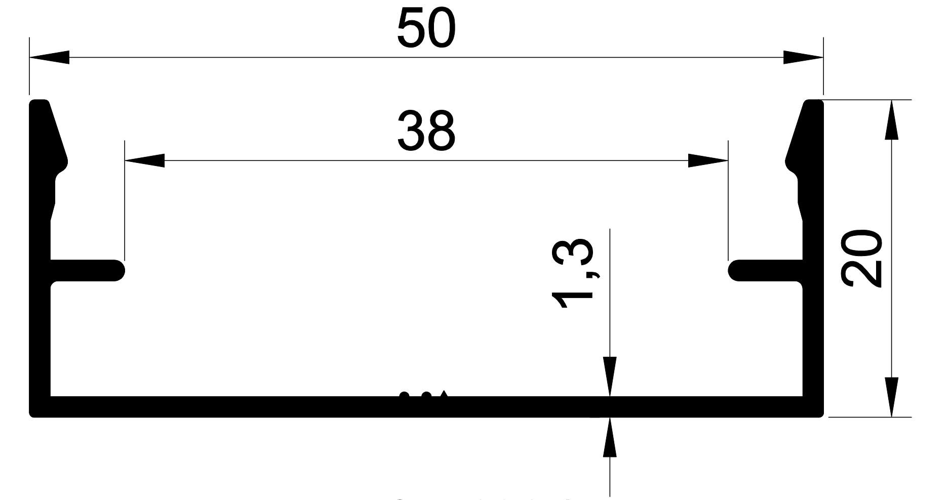
EKOL 1396 0,522 gr/m. 20 MM CEPHE KAPAK
