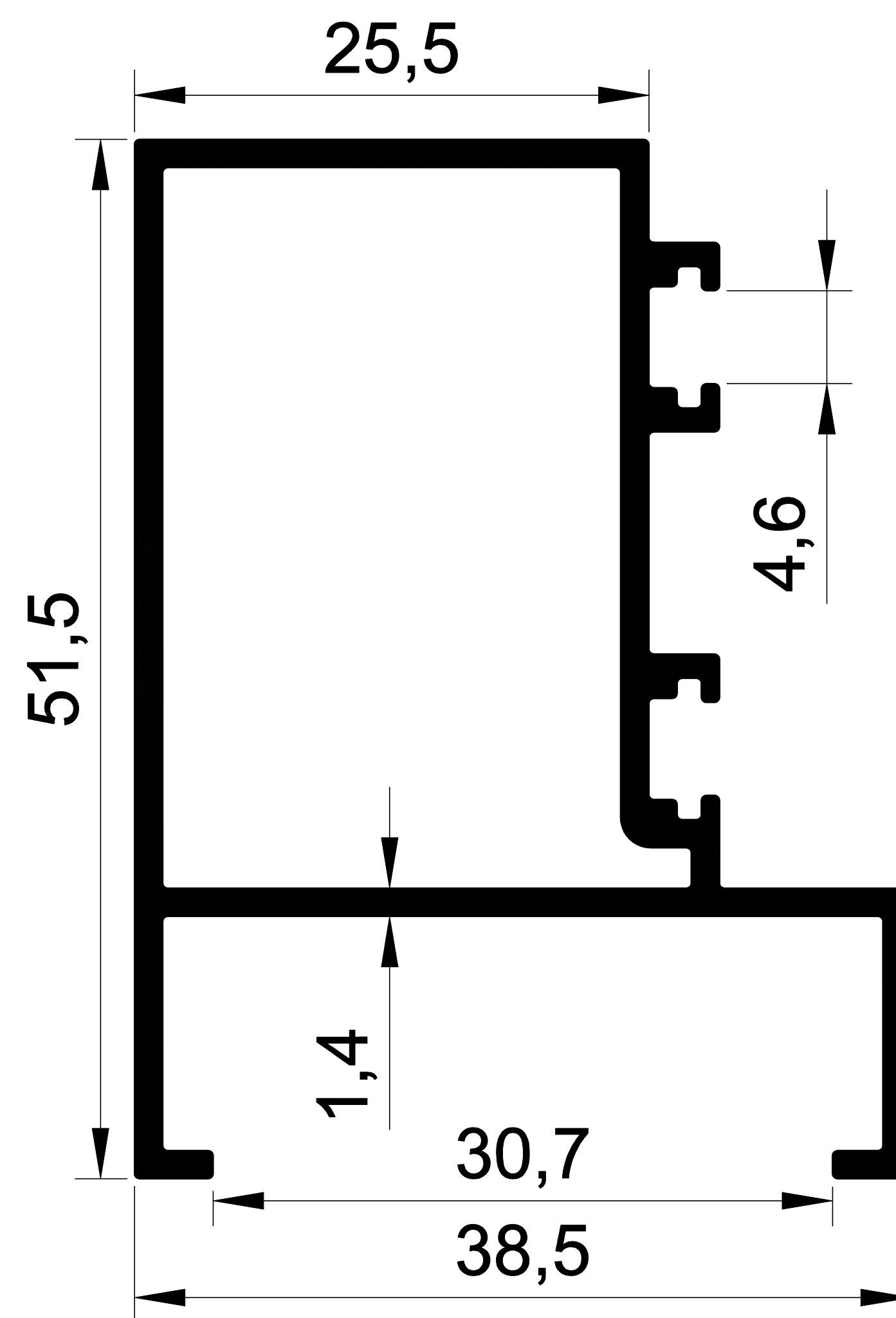
EKOL 1363 0,704 gr/m. ISI YALITIM KANAT 90° DÖNÜŞ
