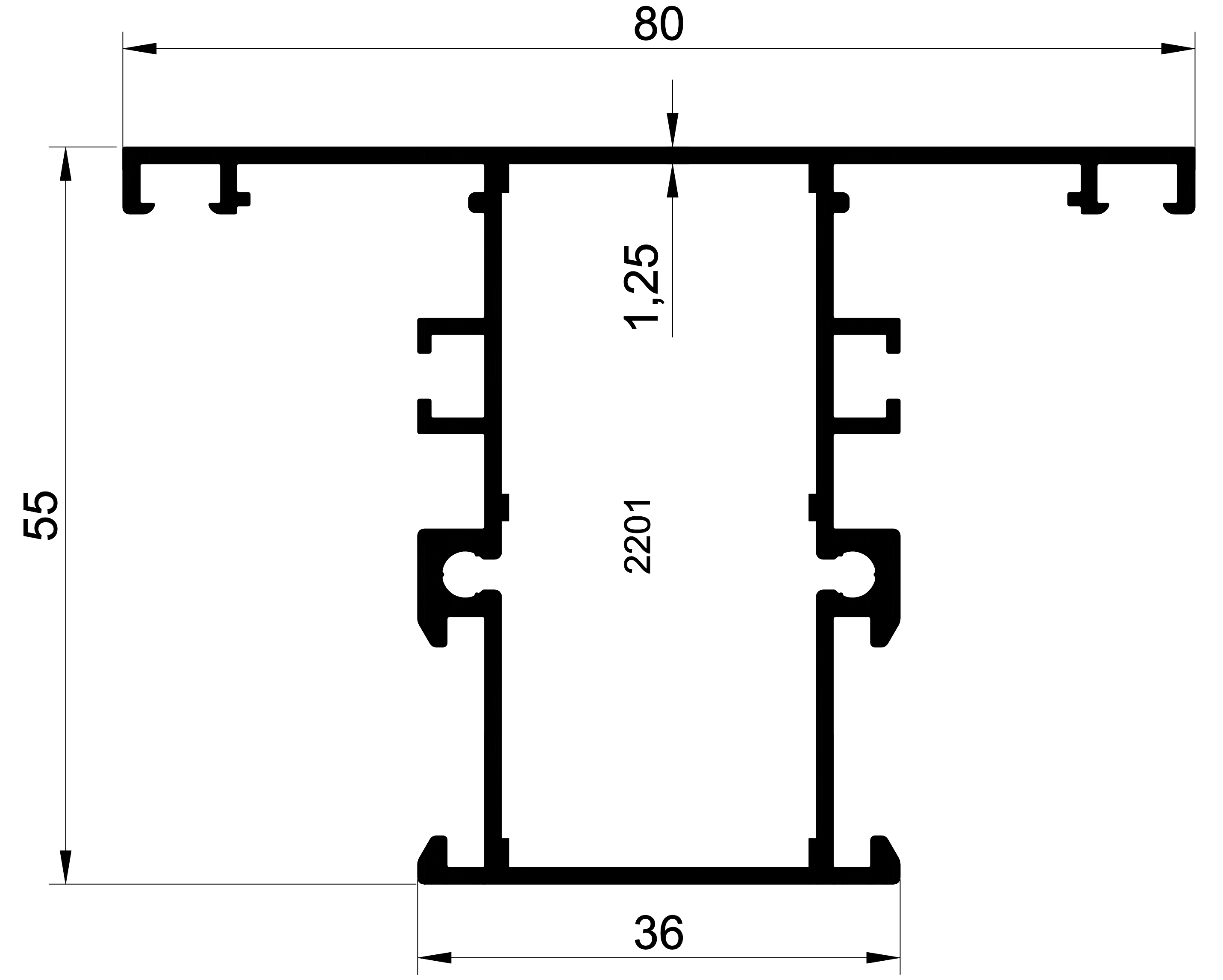
EK-55- 2201 1,073 gr/m SİSTEM 55 YALITIMSIZ ORTA
