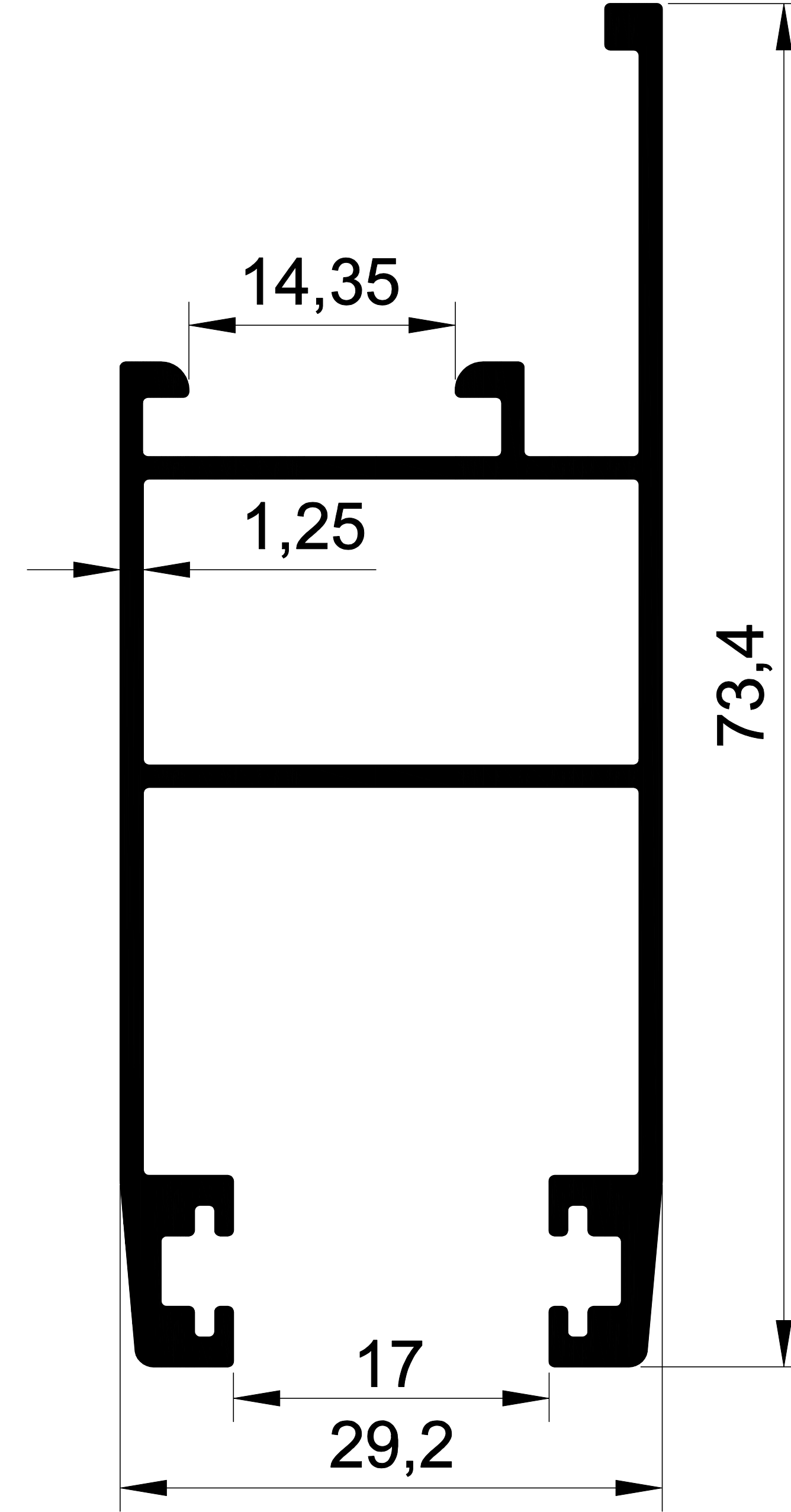
EKOL 1382 0,803 gr/m. 2000 SERİ SÜRME KANAT
