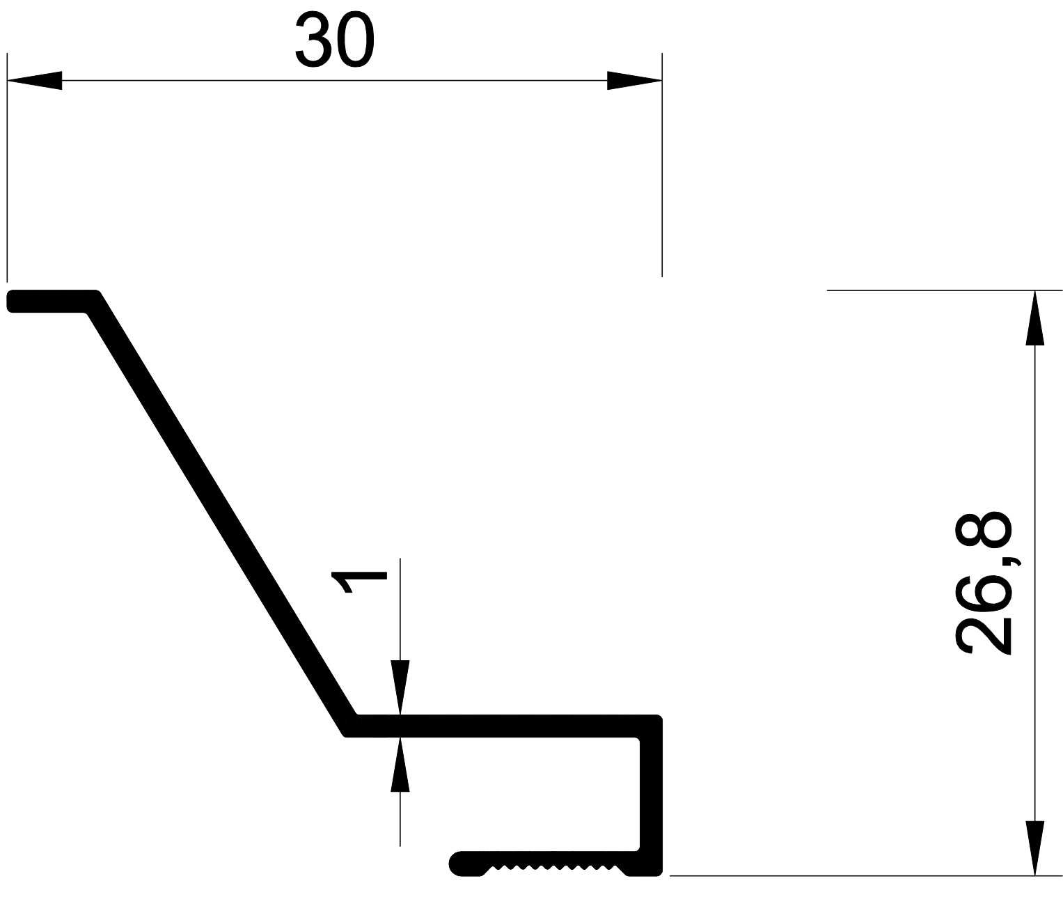
EKOL 1174 0,146 gr/m. DAMLALKI PROF.
