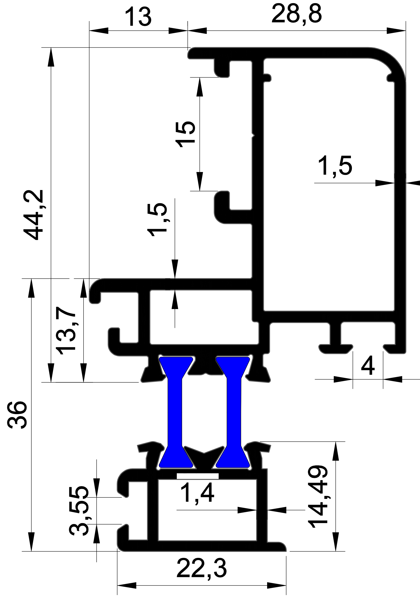
EKOL 1445 0,298 gr/m. CEPHE KASET PROFİLİ-2
