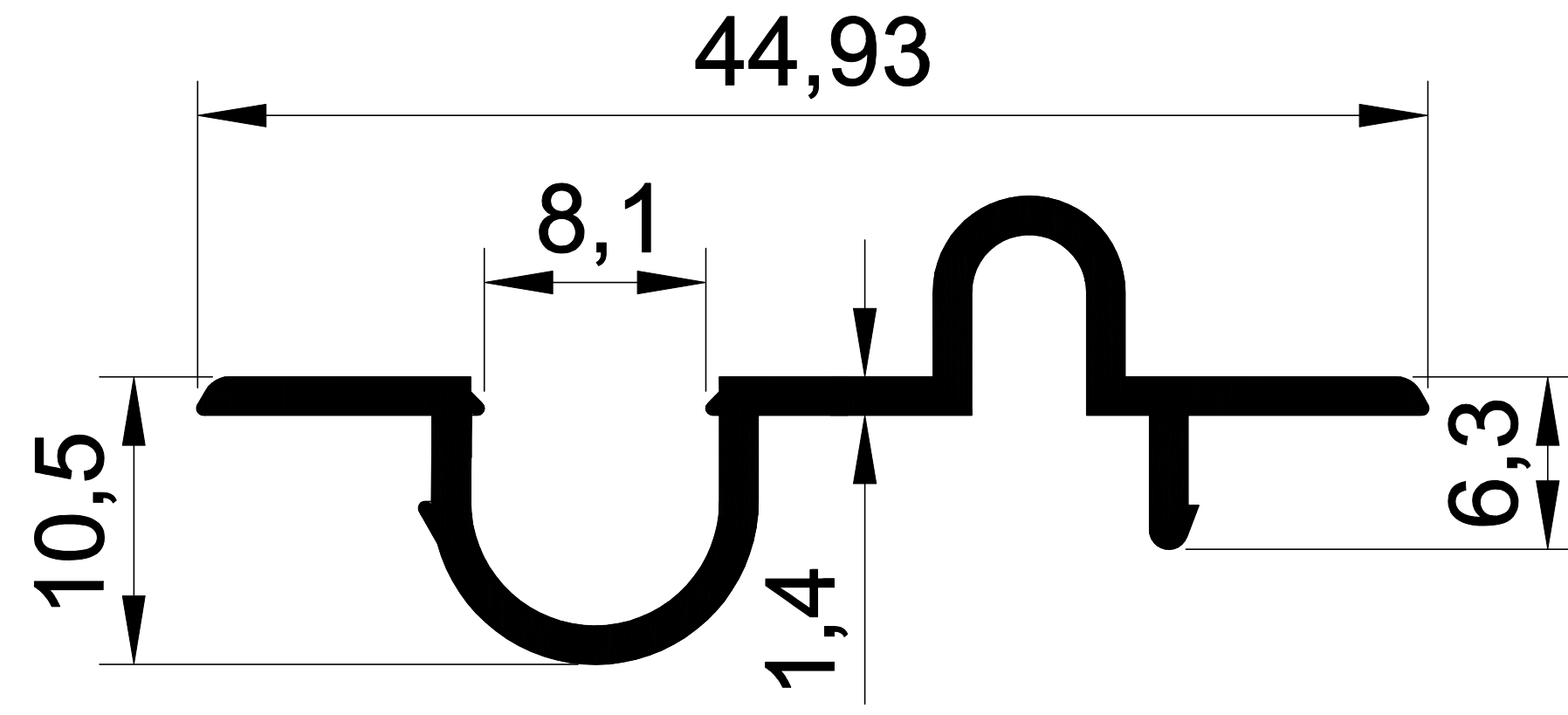
EKOL 1377 0,283 gr/m. 100'LÜK TUBA S
