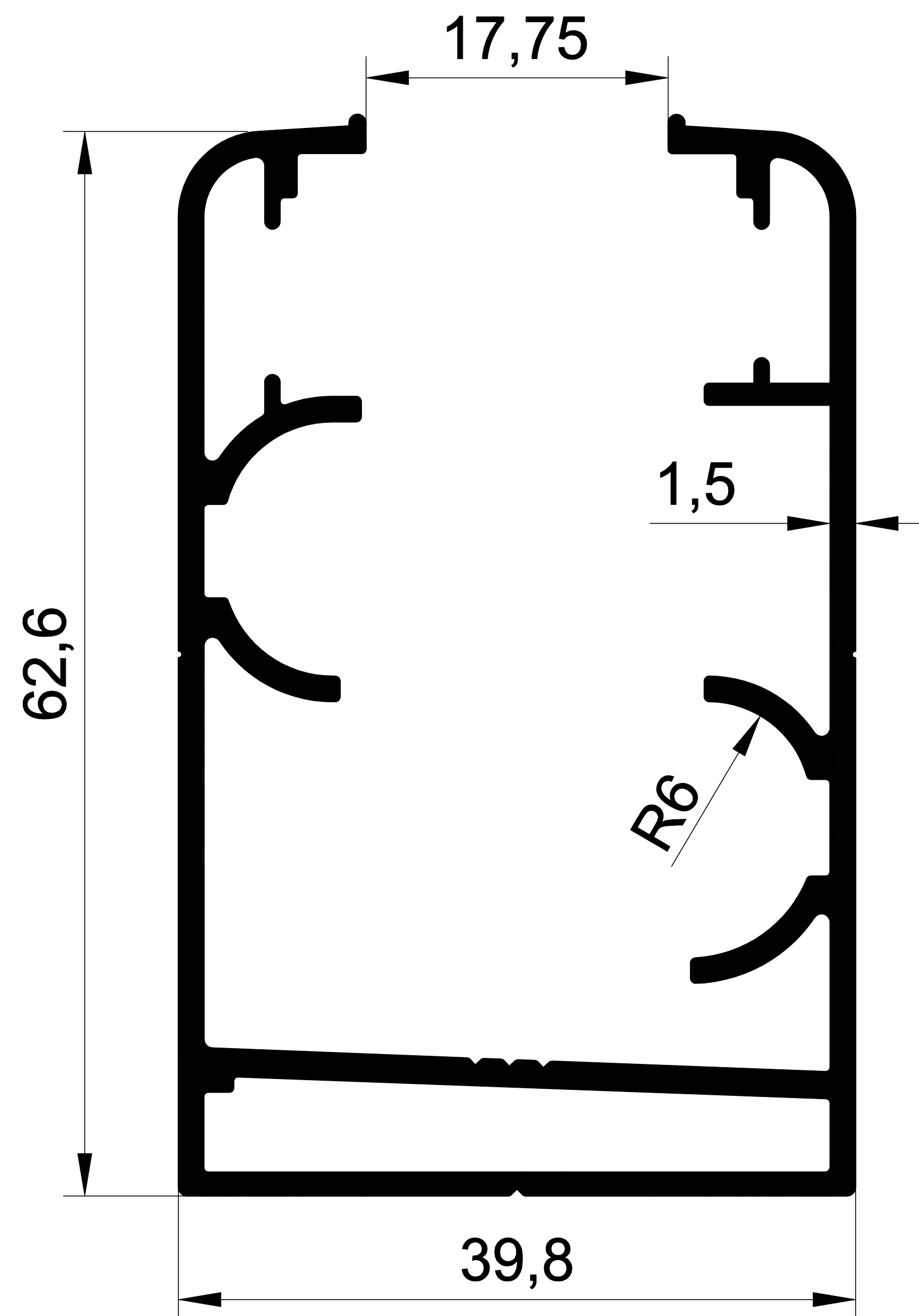
EKOL 1250-B 1,120 gr/m. GOLD KASA-1,5 mm
