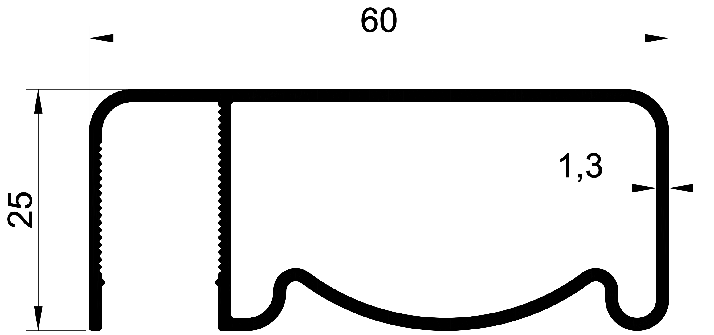
EKOL 1134 0,622 gr/m. 25X60 YANDAN CAMLI
