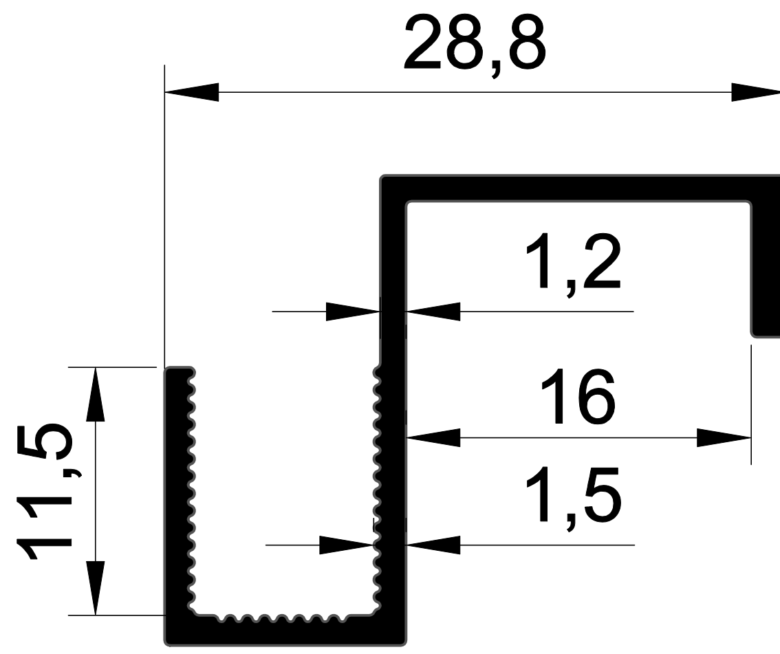
EKOL 1448 0.236 gr/m. C.B KOL PROFİLİ-1
