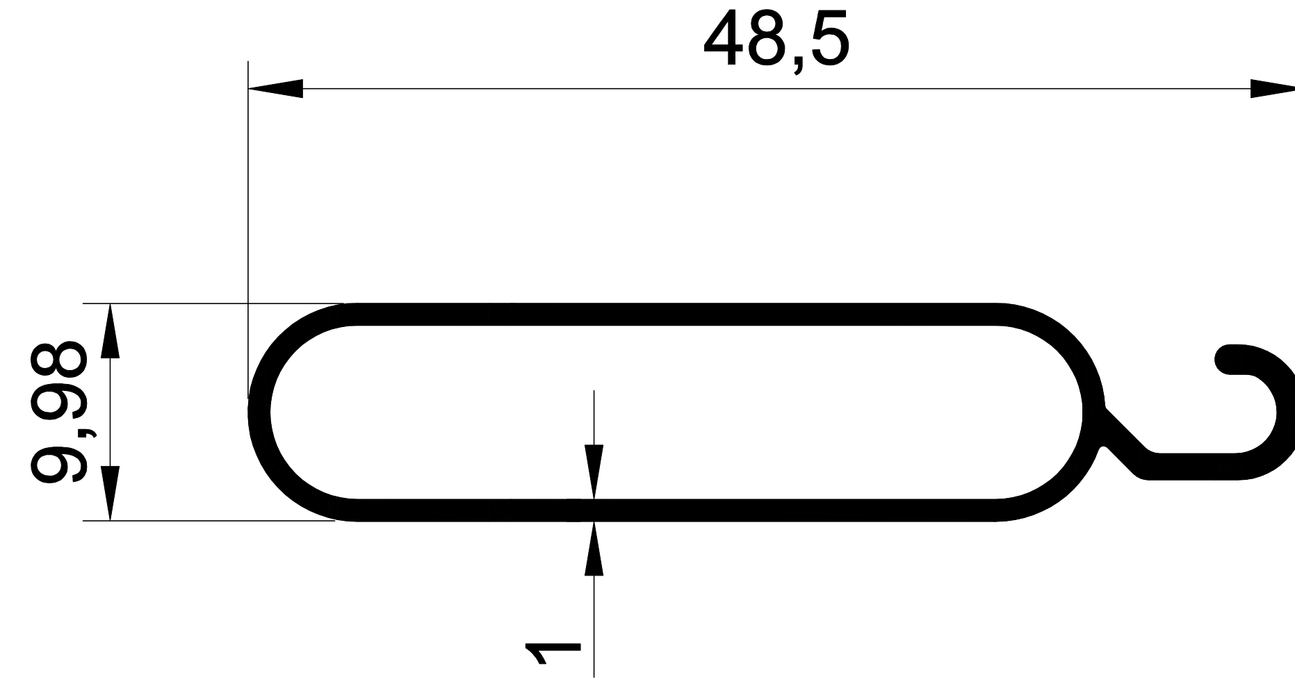
EKOL 1181 0,287 gr/m. PANJUR ALT PARÇA
