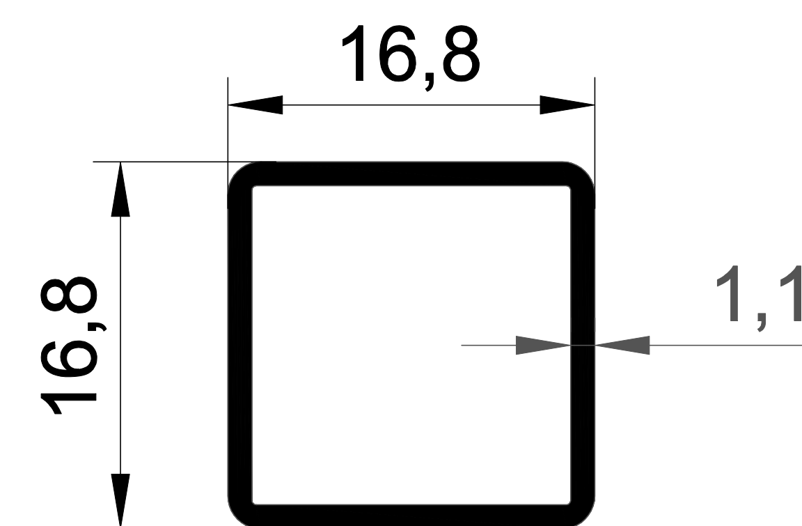
EKOL 1047 0,181 gr/m.
