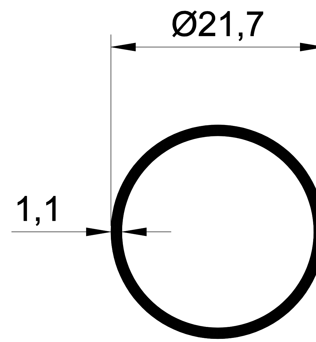
EKOL 1056 0,192gr/m.
