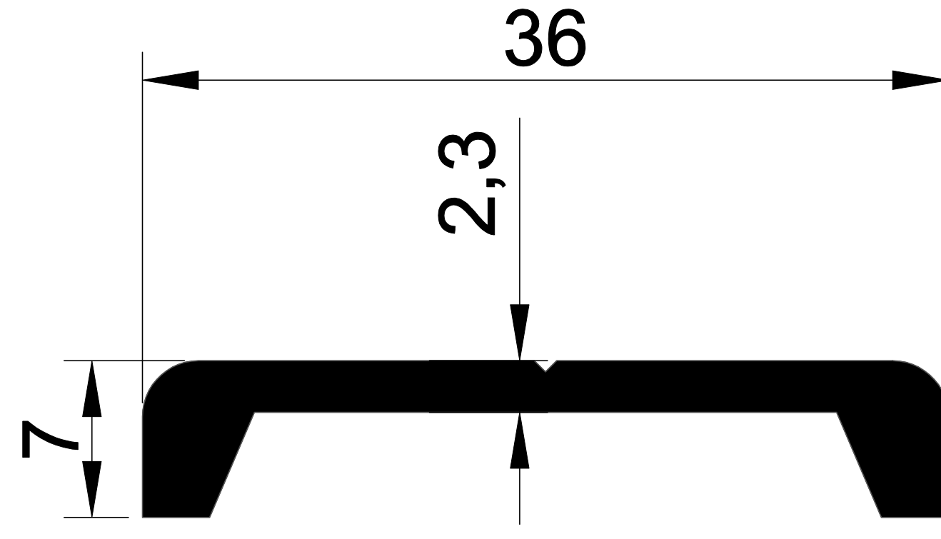
EKOL 1239 0,320 gr/m.
