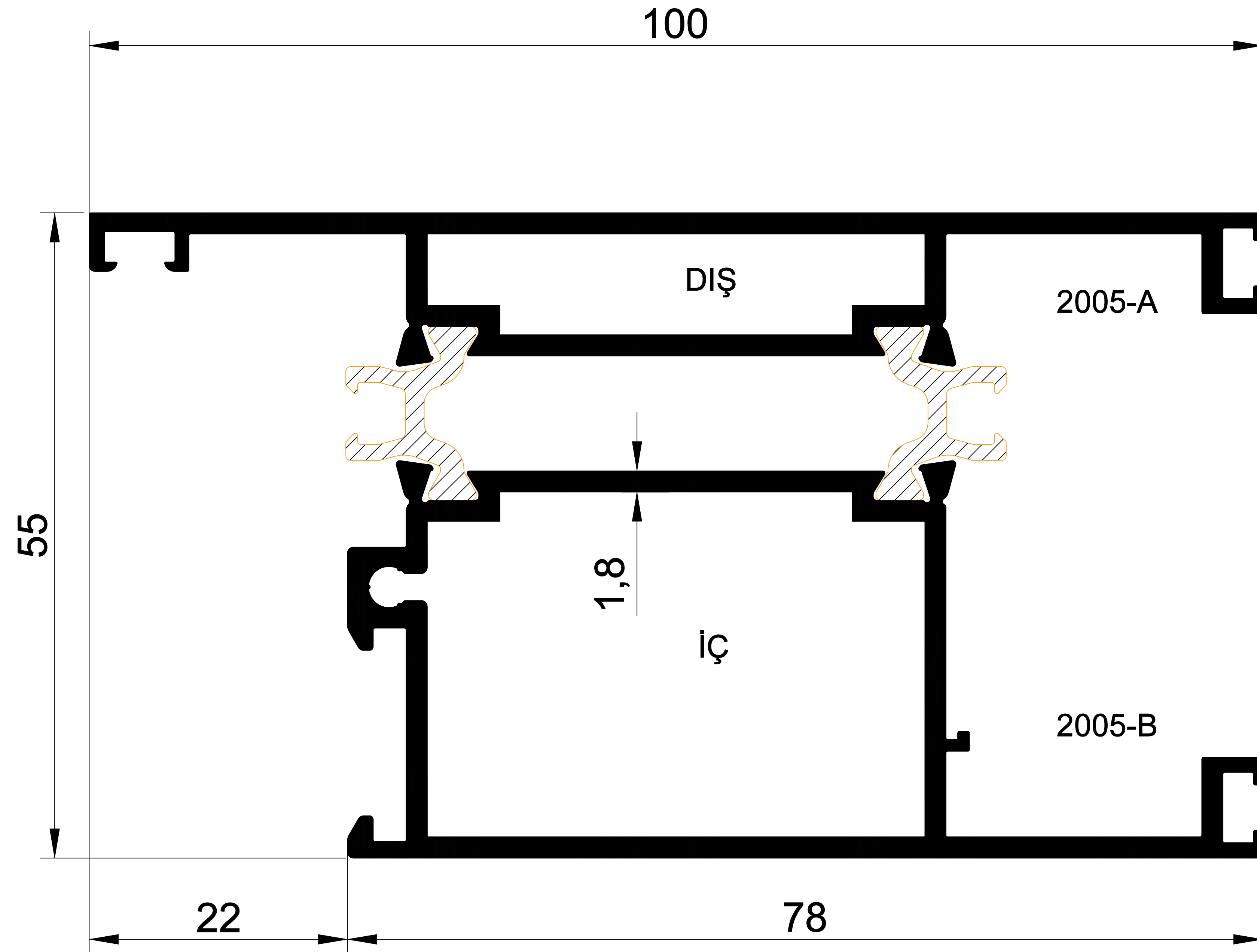
EKL-55- 2005 1,964 gr/m SİSTEM 55 ISI YALITIM ETEK
