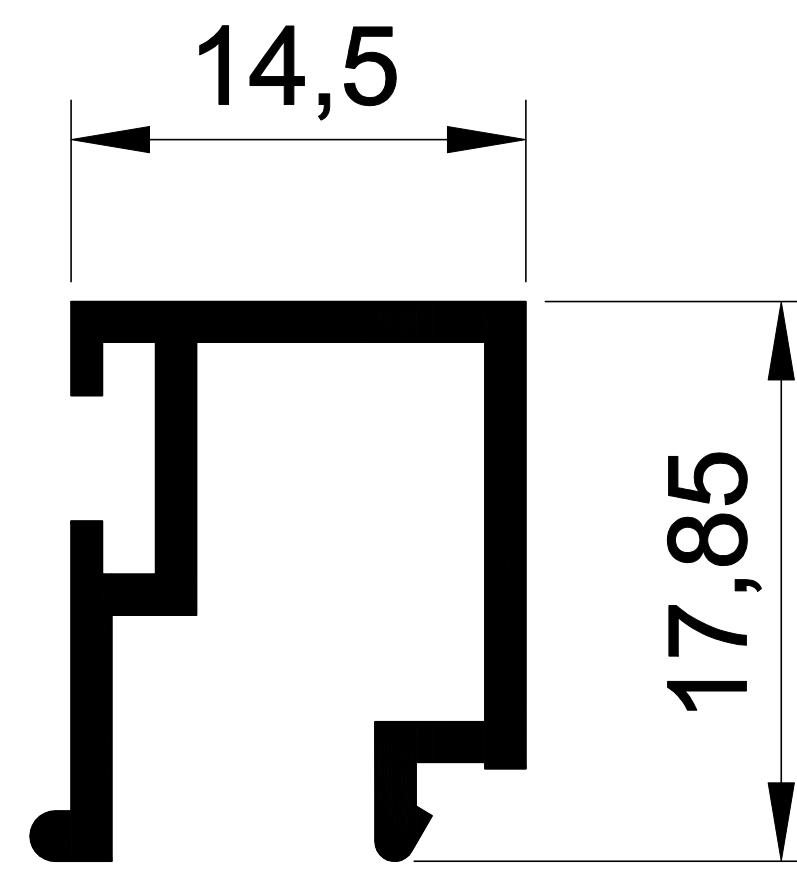
EKOL 1189 0,206 gr/m TEK CAM ÇITASI
