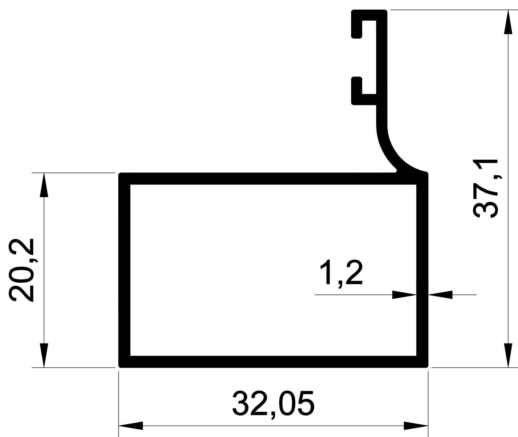
EKOL 1153 0,404 gr/m. FIRTINA DIKME
