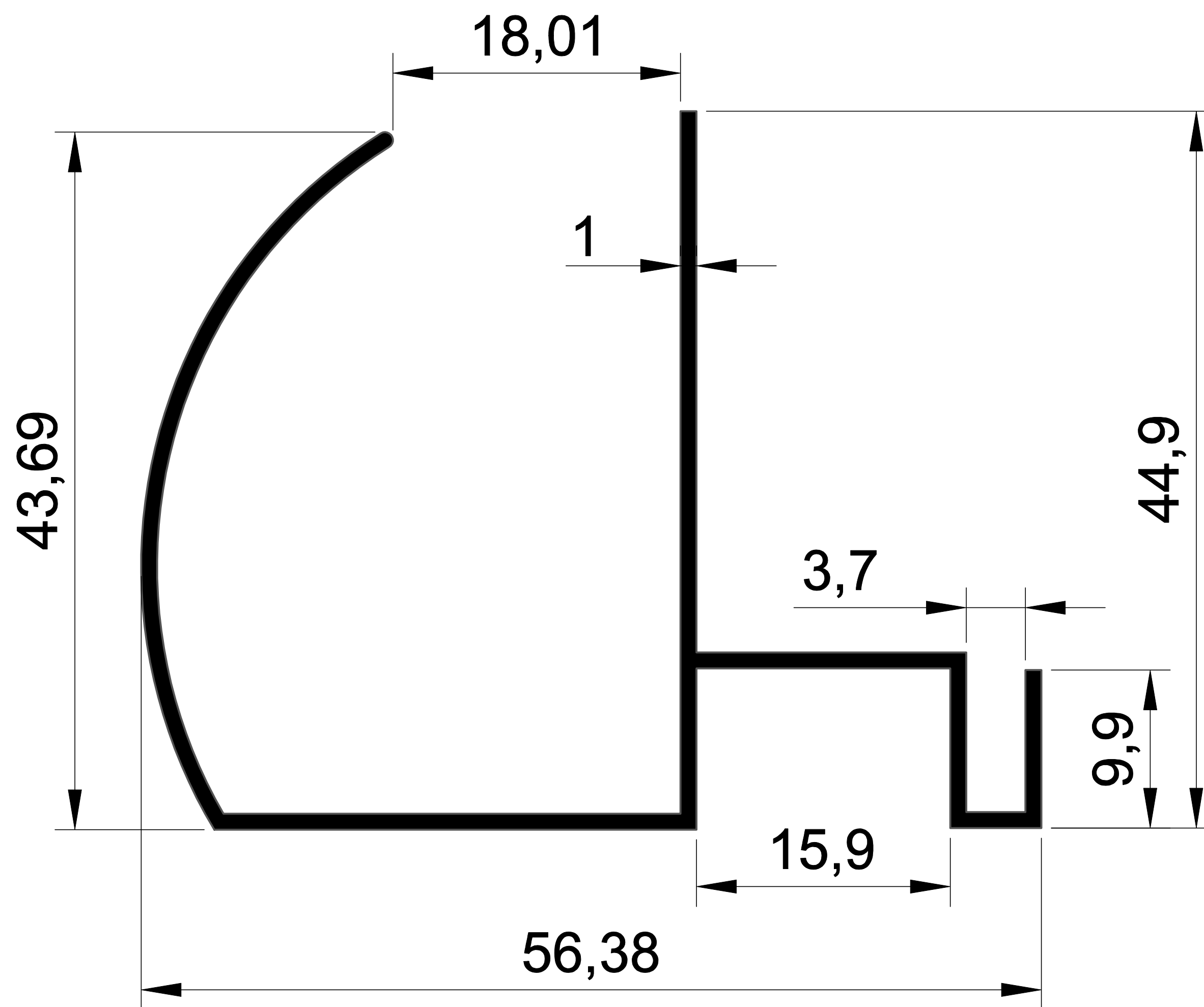
EKOL 1453 0.430 gr/m. KENAR PROFİLİ
