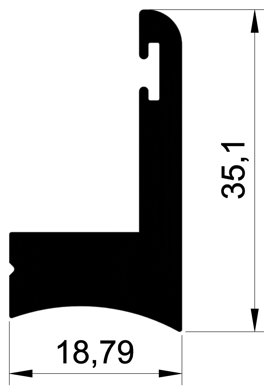
EKOL 1127 0,715 gr/m.
