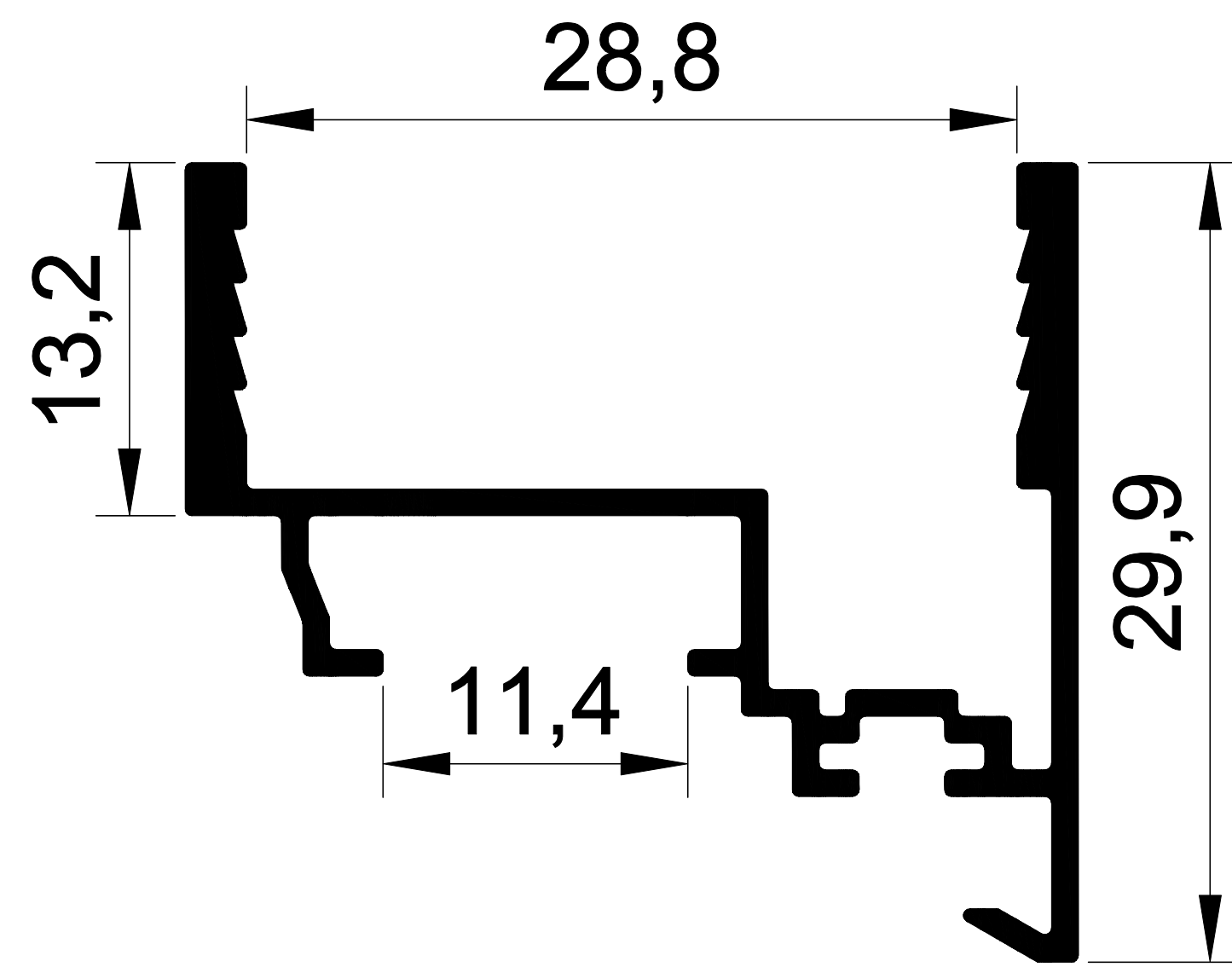
EKOL 1436 0.358 gr/m. ISI YALITIM KATLANIR CAM BALKON DÖNÜŞ
