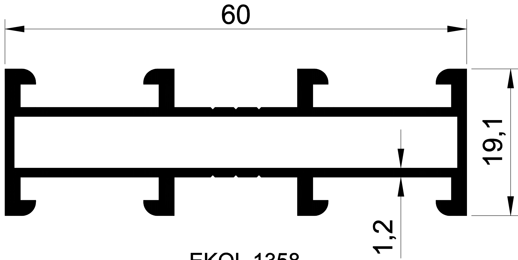
EKOL 1358 0,721 gr/m. C-60 DAR KASA
