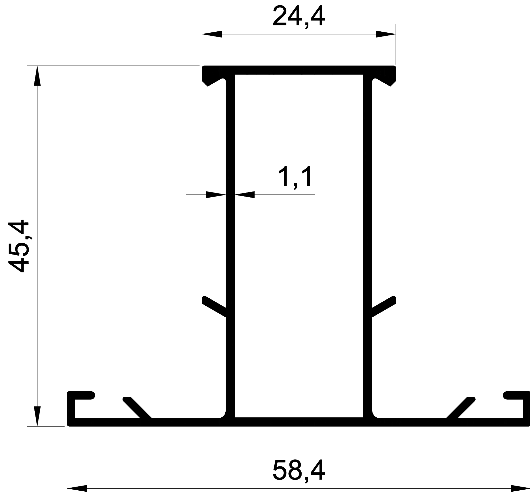
EKOL 1102 0,547 gr/m. ALDOKS DAR ORTA
