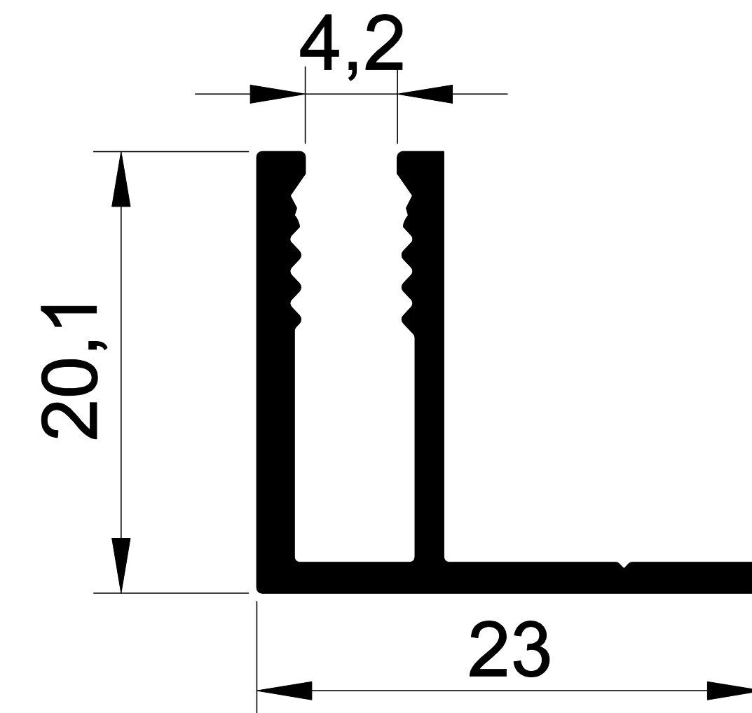
EKOL 1208 0,252 gr/m. KOMPAZİT - F
