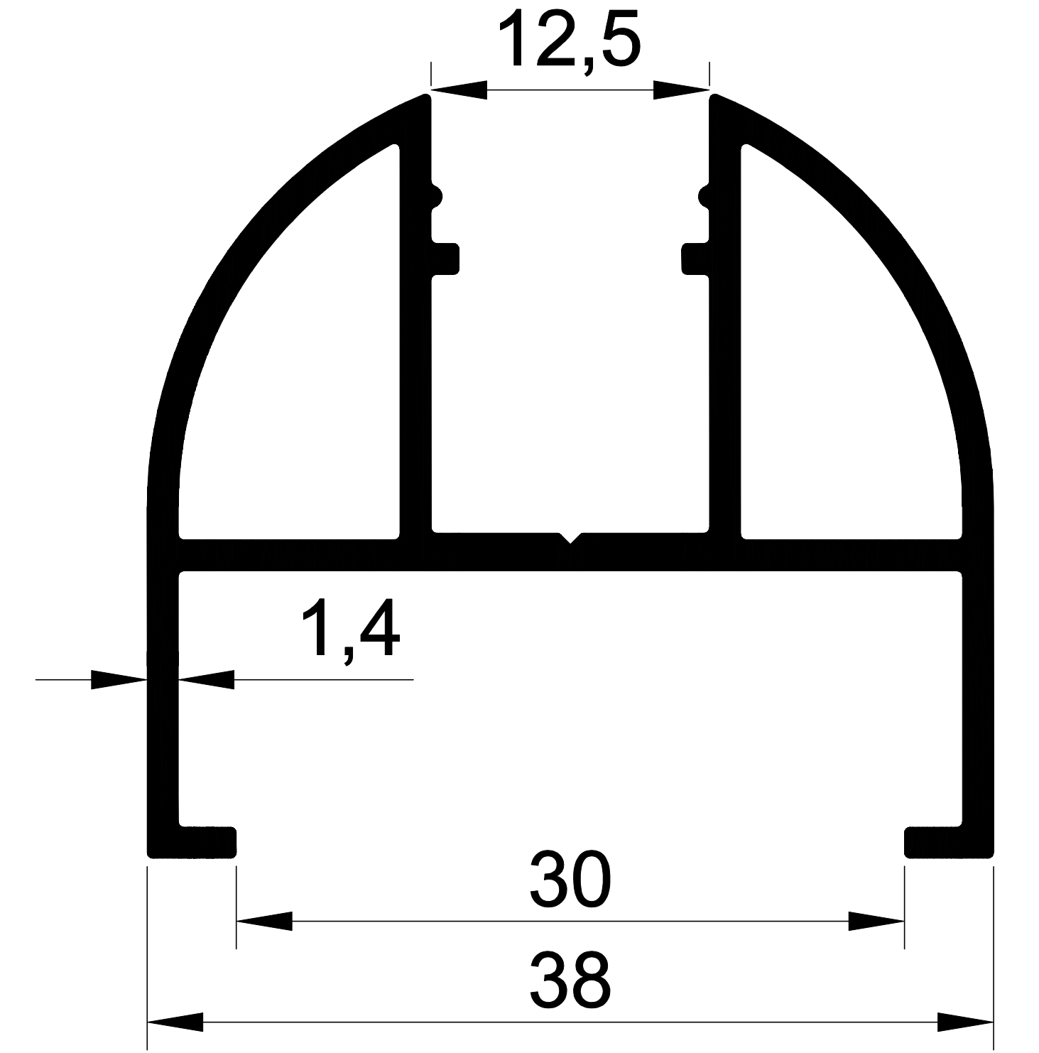
EKOL 1365 0,607 gr/m. ISI YALITIM KÖŞE DÖNÜŞ
