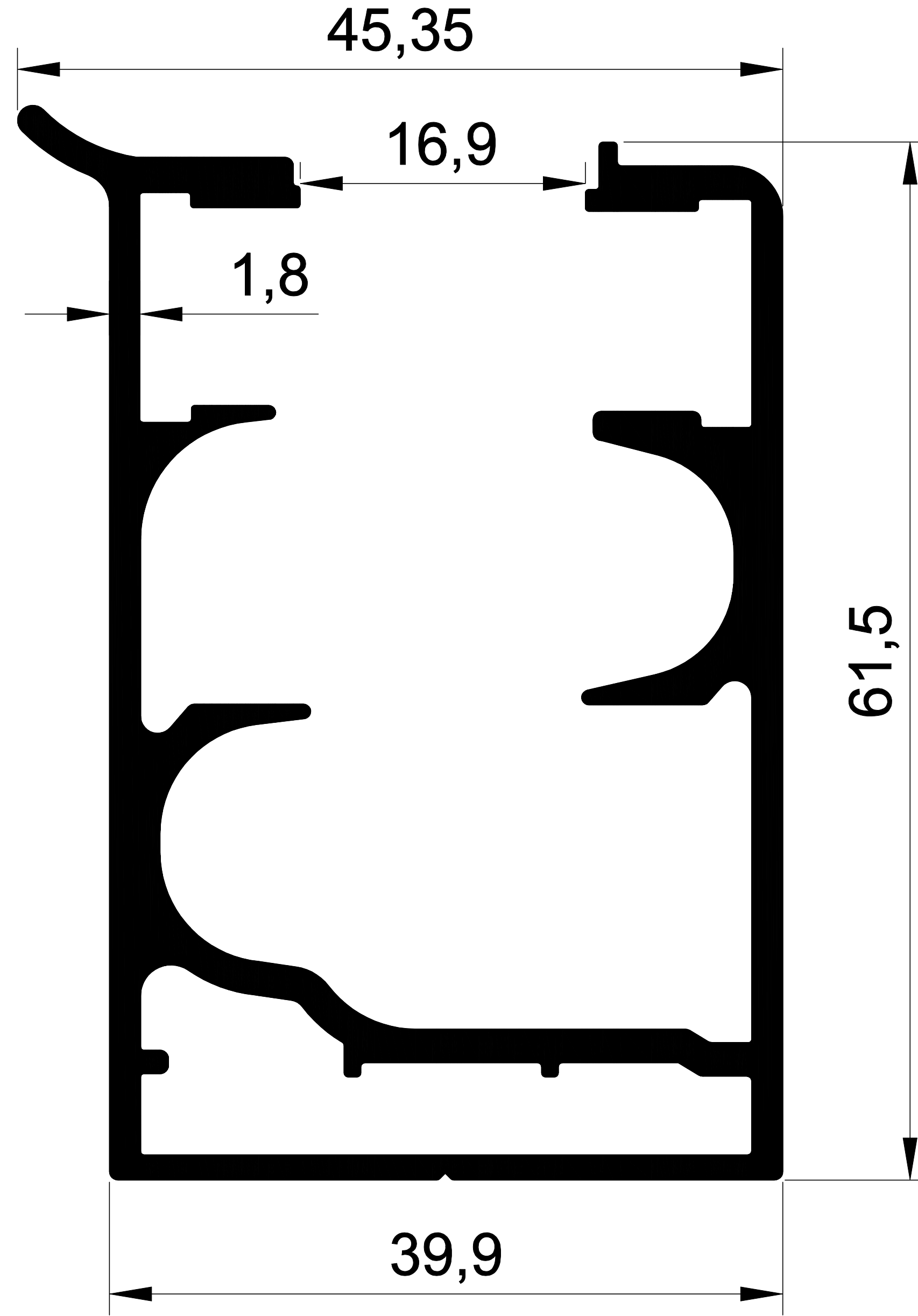
EKOL 1290 1,428 gr/m. ISI YALITIM ÜSTTEN DAMLALIKLI KASA
