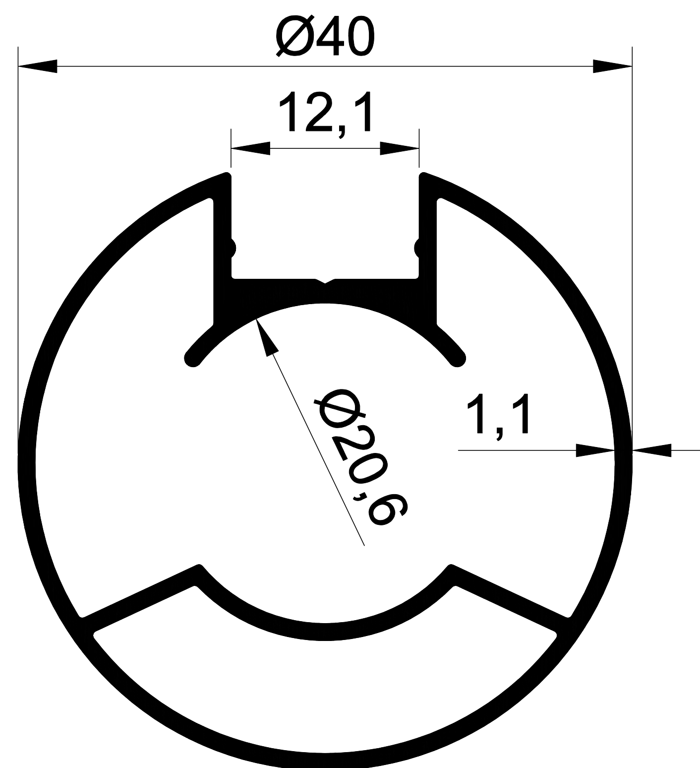
EKOL 1337 0,569 gr/m.
