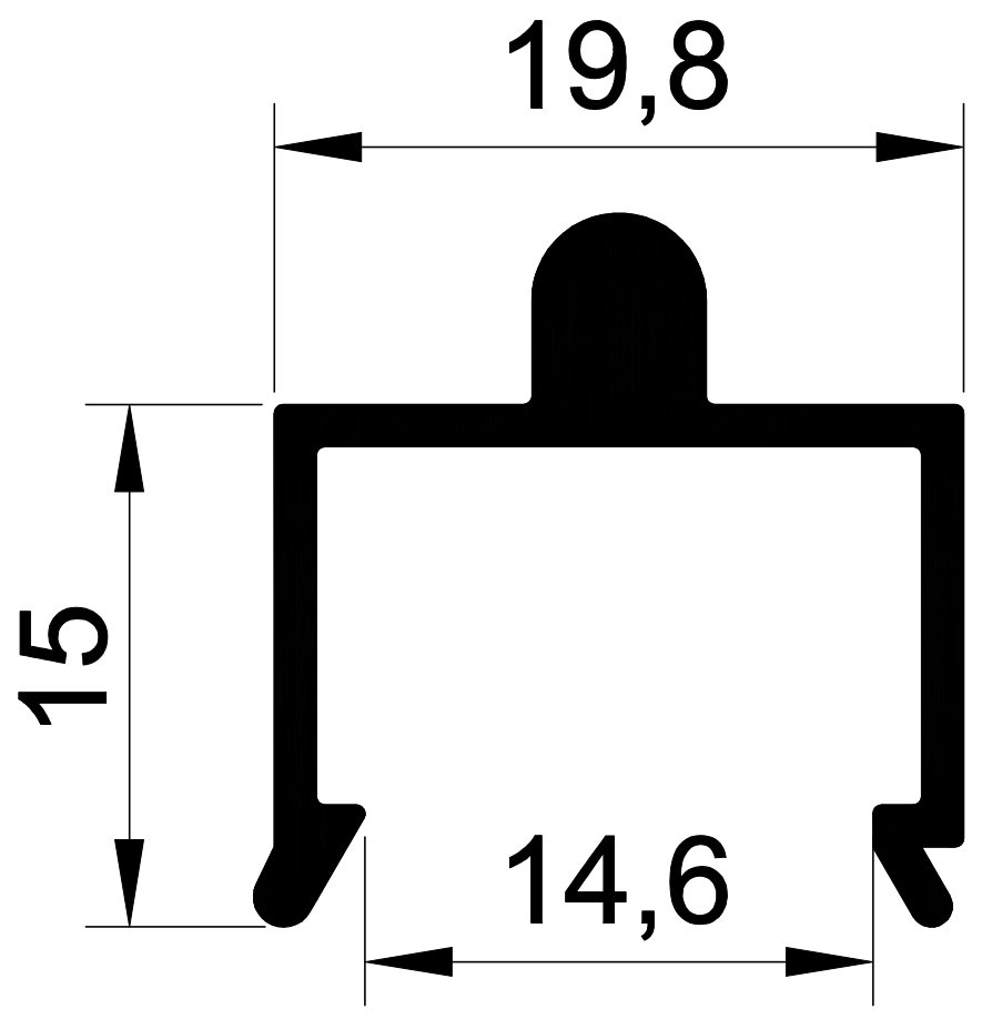
EKOL 1376 0,234 gr/m. 100'LÜK TUBA RAY
