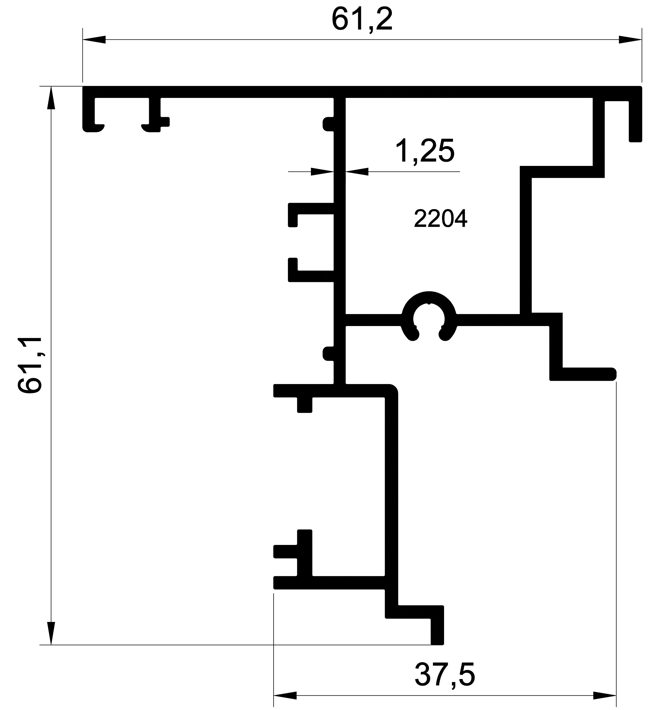
EK-55- 2204 0,932 gr/m
