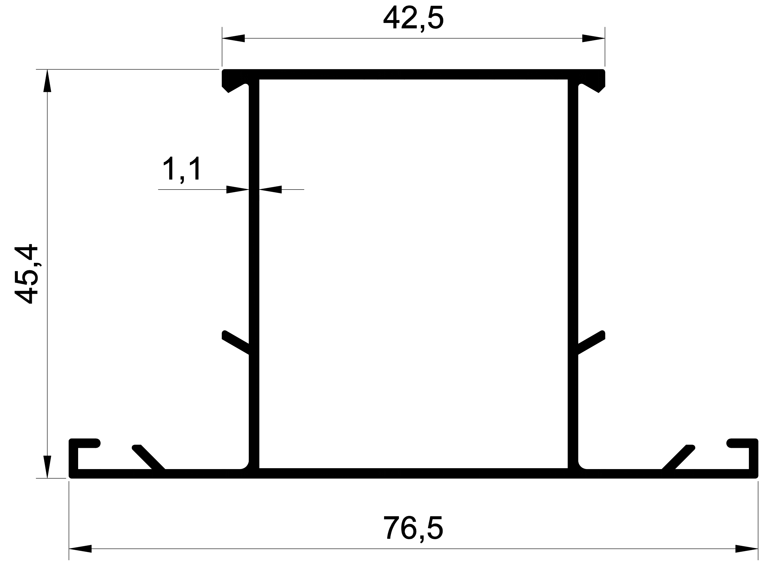
EKOL 1105 0,645 gr/m. ALDOKS GENİŞ ORTA
