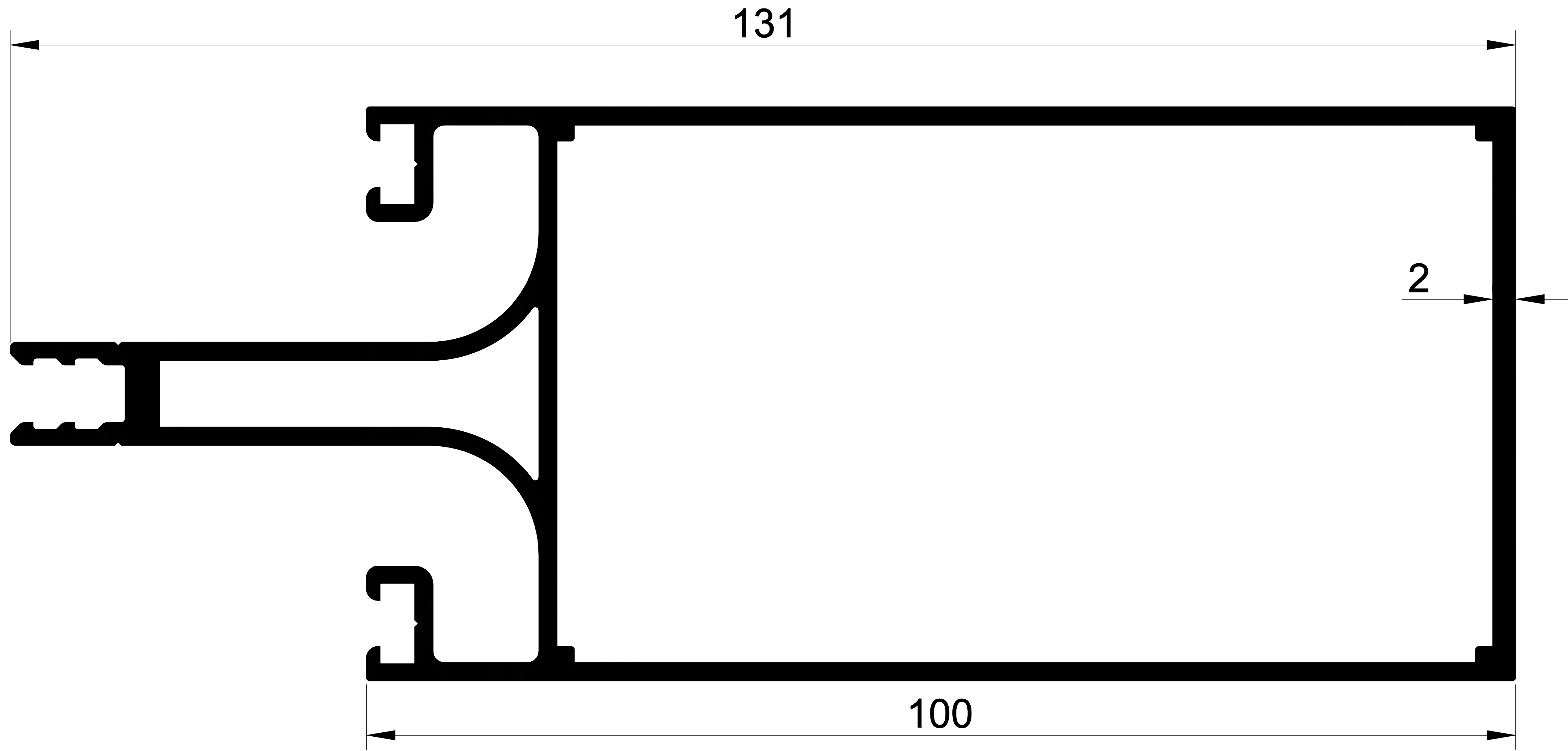
EKOL 1391 1,940 gr/m. 100'LÜK CEPHE PROFİLİ UZUN GAGA
