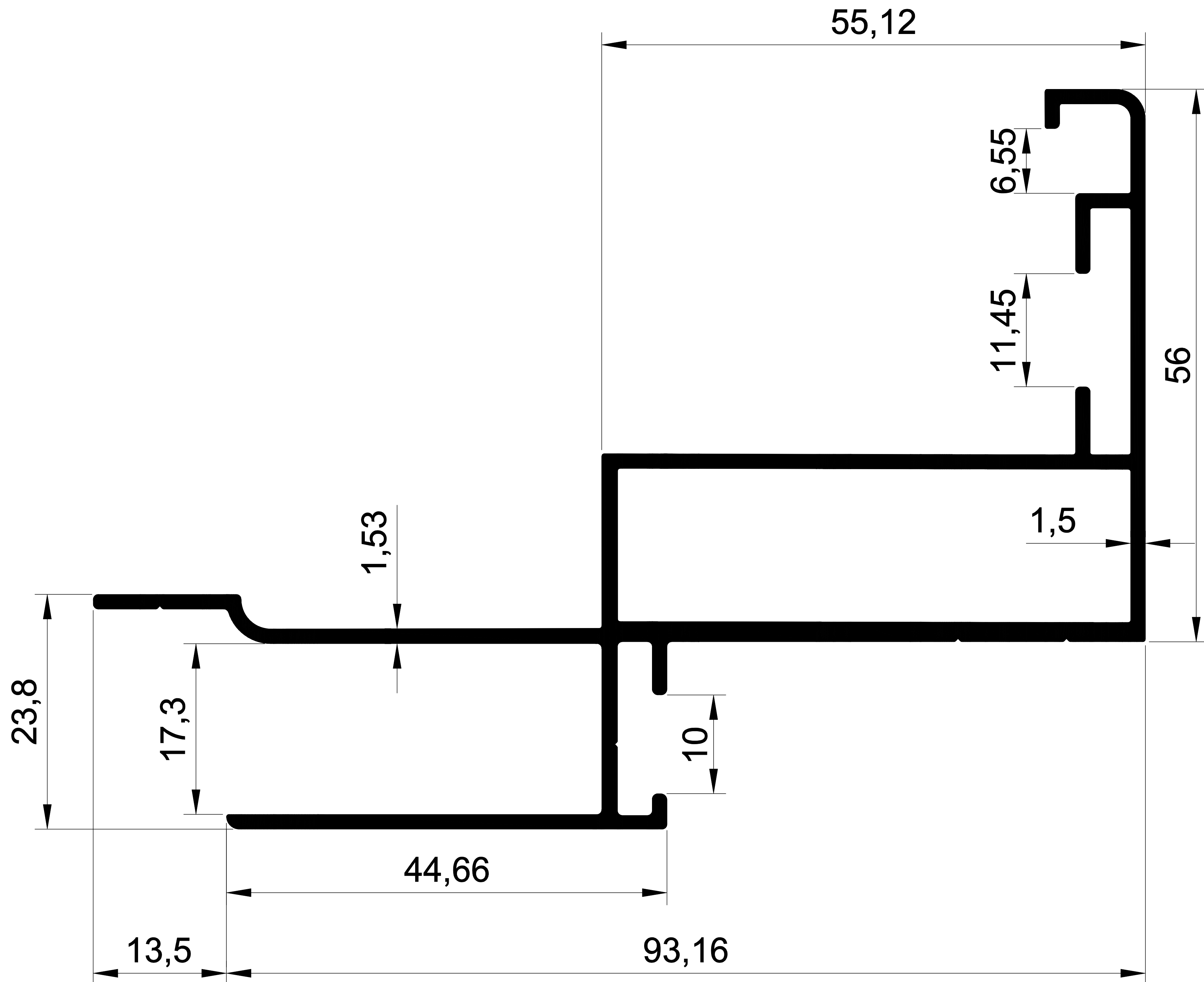
EKOL 1421 1,430 gr/m.
