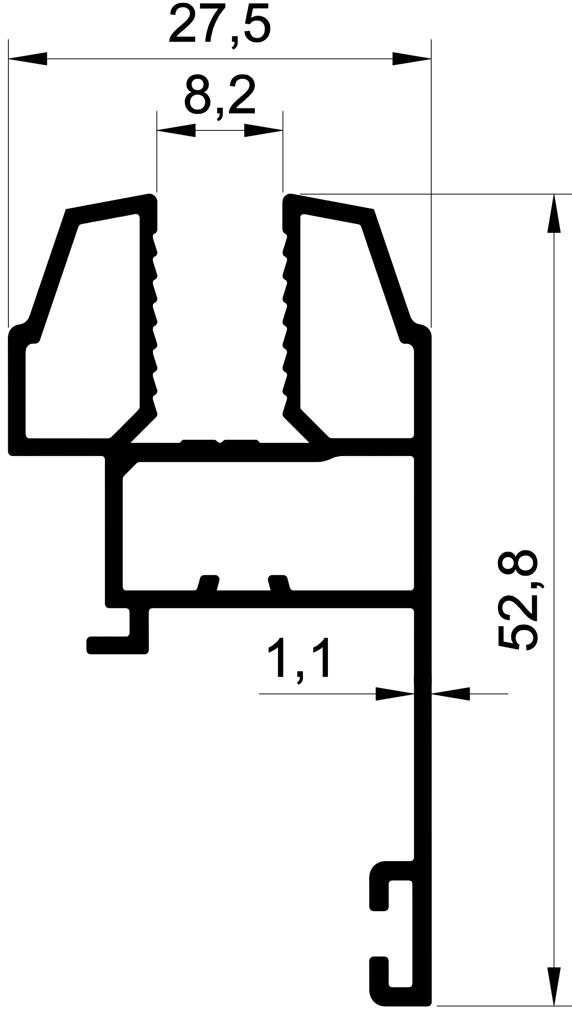
EKOL 1379 0,549 gr/m. 53'LÜK CAM BALKON KİLİT
