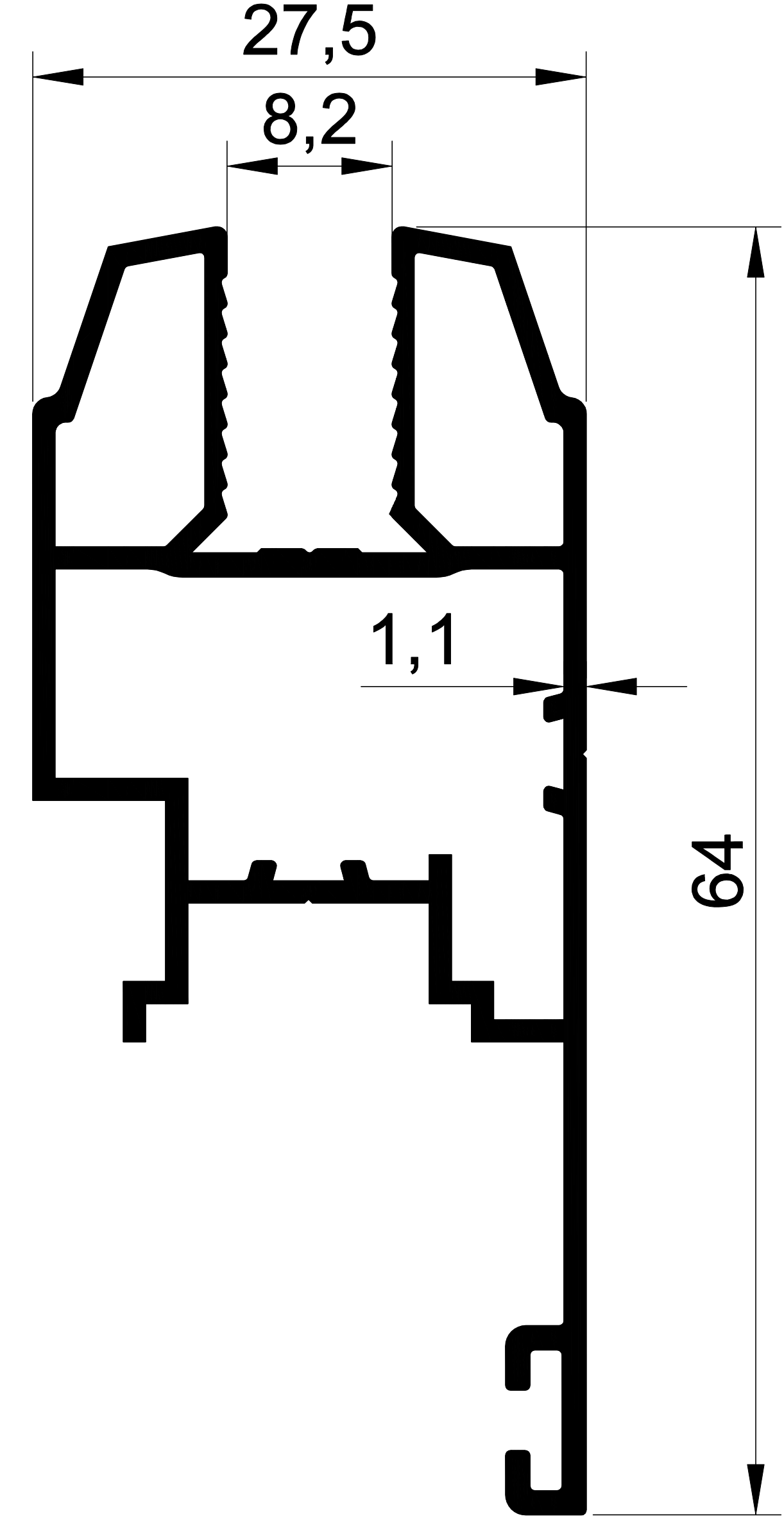
EKOL 1380 0,663 gr/m. 64'LÜK CAM BALKON KİLİT
