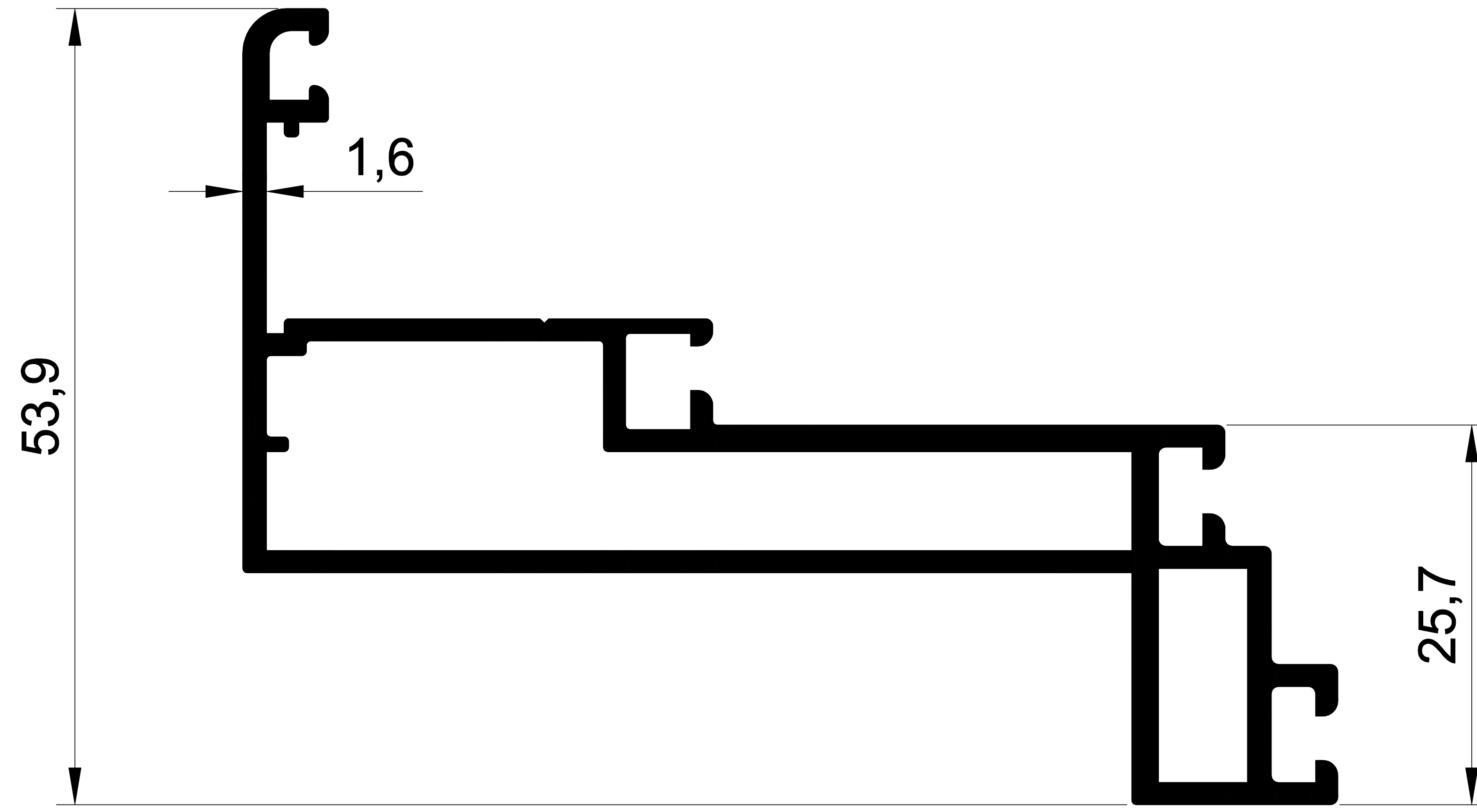
EKOL 1392 1,343 gr/m. CEPHE KANAT KASASI
