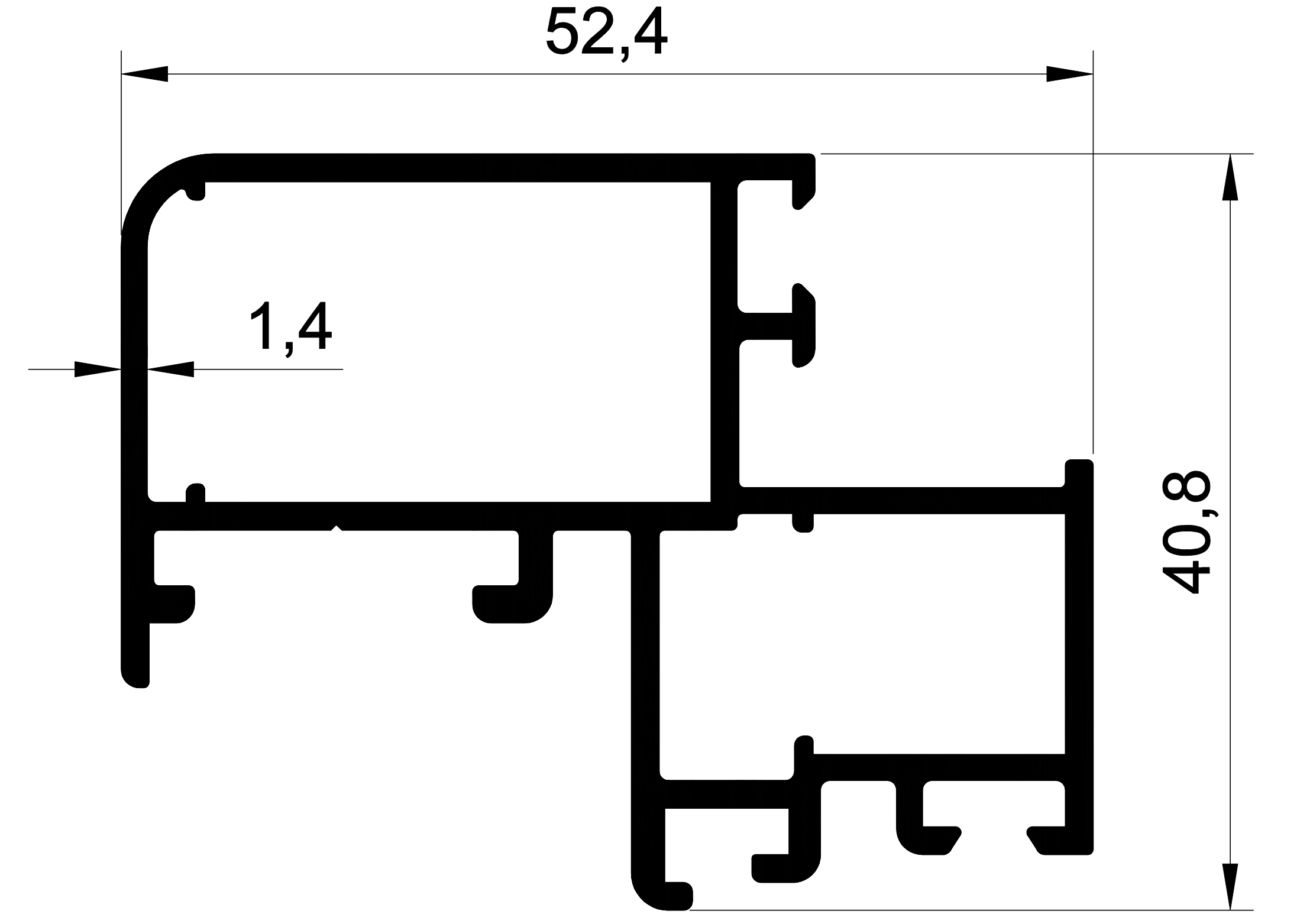
EKOL 1393 0,750 gr/m. CEPHE KASET
