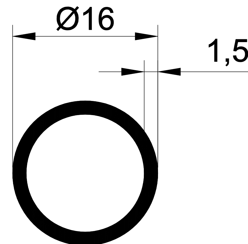
EKOL 1077 0,184 gr/m.
