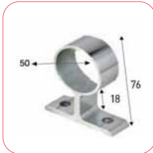
• 3134 50'lik Boru Duvar Bağlantısı
