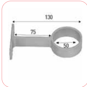
• 3134-B 50'lik Boru Duvar Bağlantısı Tırnaksız Uzun
