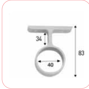
• 3131-B 40'lik Dikme Duvar Bağlantısı Tırnaksız
