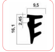
• 2449 Isı Yalıtım İç Cam Fitol
