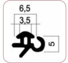
• 2451 Isı Yalıtım Cam Fitol
