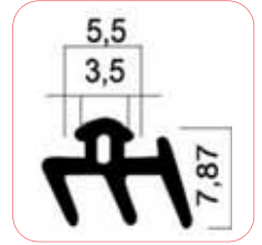
• 2450 Isı Yalıtım İç Cam Fitol
