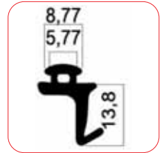
• 2452 Isı Yalıtım Orta Fitol
