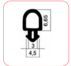
• 2453 Isı Yalıtım Kasa Fitol
