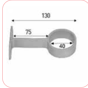
• 3131-C 40'lik Dikme Duvar Bağlantısı Tırnaksız Uzun
